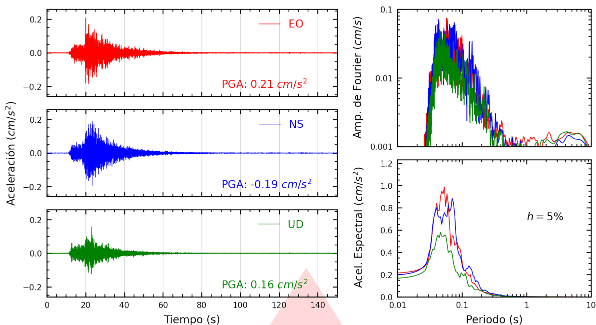
Figura A.1: Registros tiempo-historia, espectros de Fourier y de respuesta en las direcciones EO, NS y vertical de la estación UNSA2. Sismo de Camaná, Camaná - Arequipa del 2026-08-21, 01:45:00 (Hora local)
