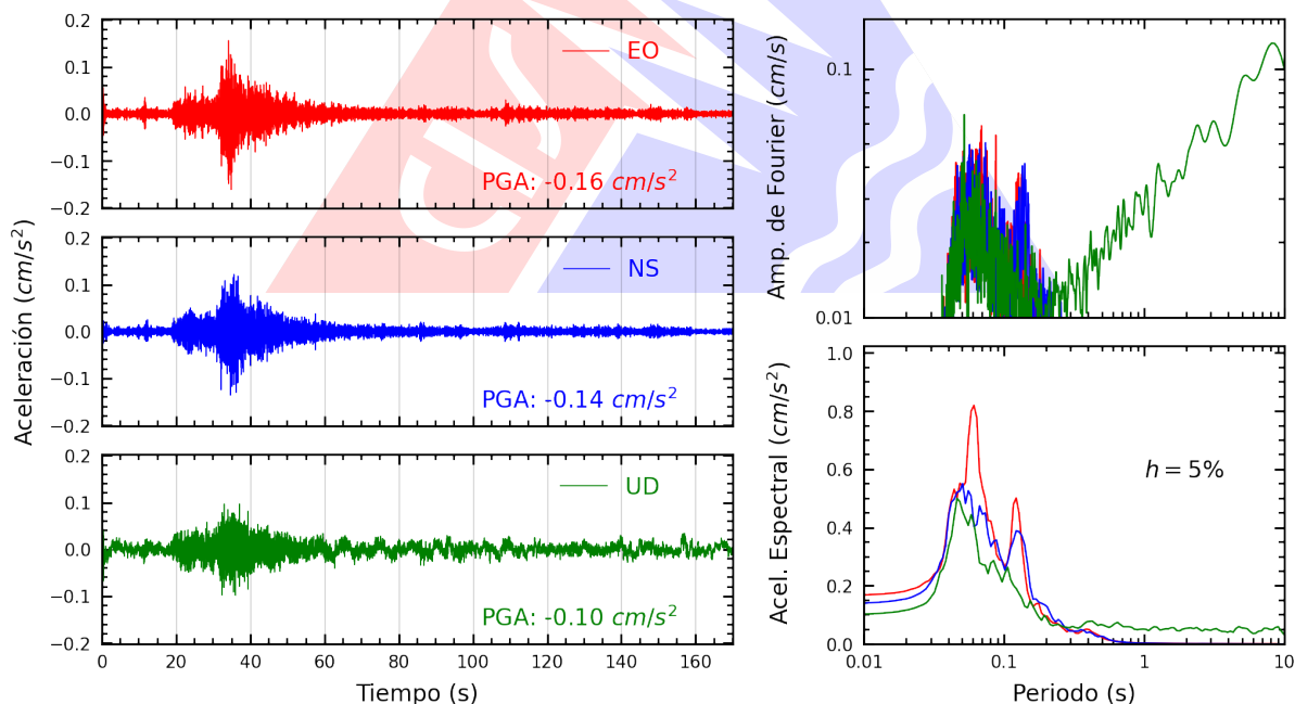
Figura A.2: Registros tiempo-historia, espectros de Fourier y de respuesta en las direcciones EO, NS y vertical de la estación SCARQ. Sismo de Camaná, Camaná - Arequipa del 2026-08-21, 01:45:00 (Hora local)
