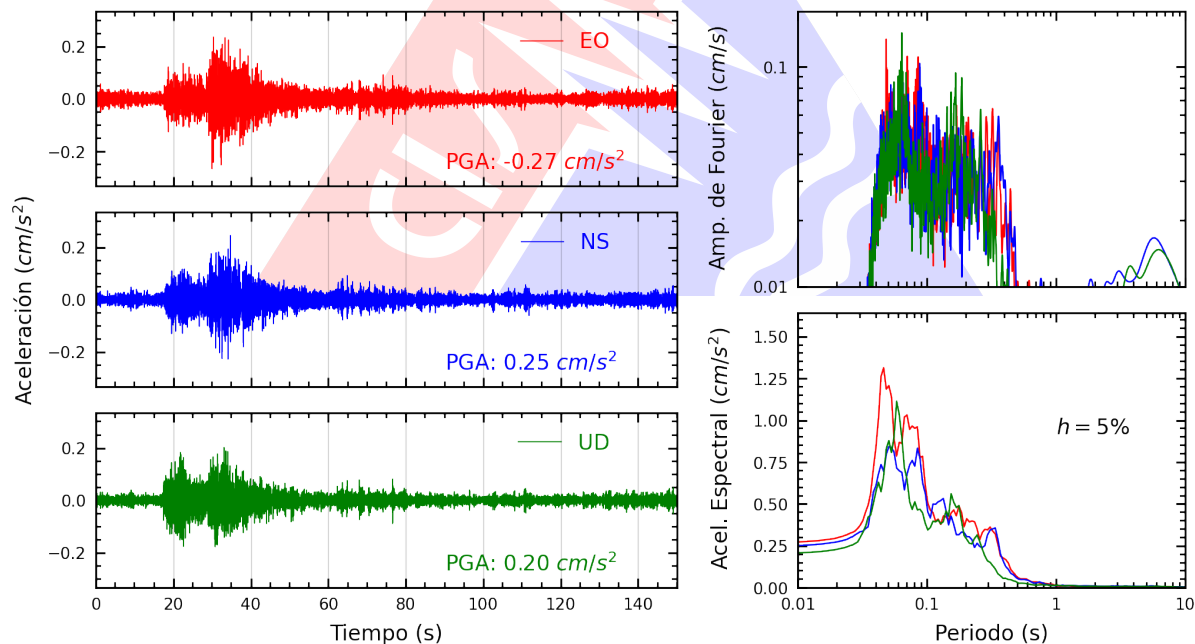
Figura A.2: Registros tiempo-historia, espectros de Fourier y de respuesta en las direcciones EO, NS y vertical de la estación CREY. Sismo de Ilo, Ilo - Moquegua del 2026-08-21, 15:39:40 (Hora local)
