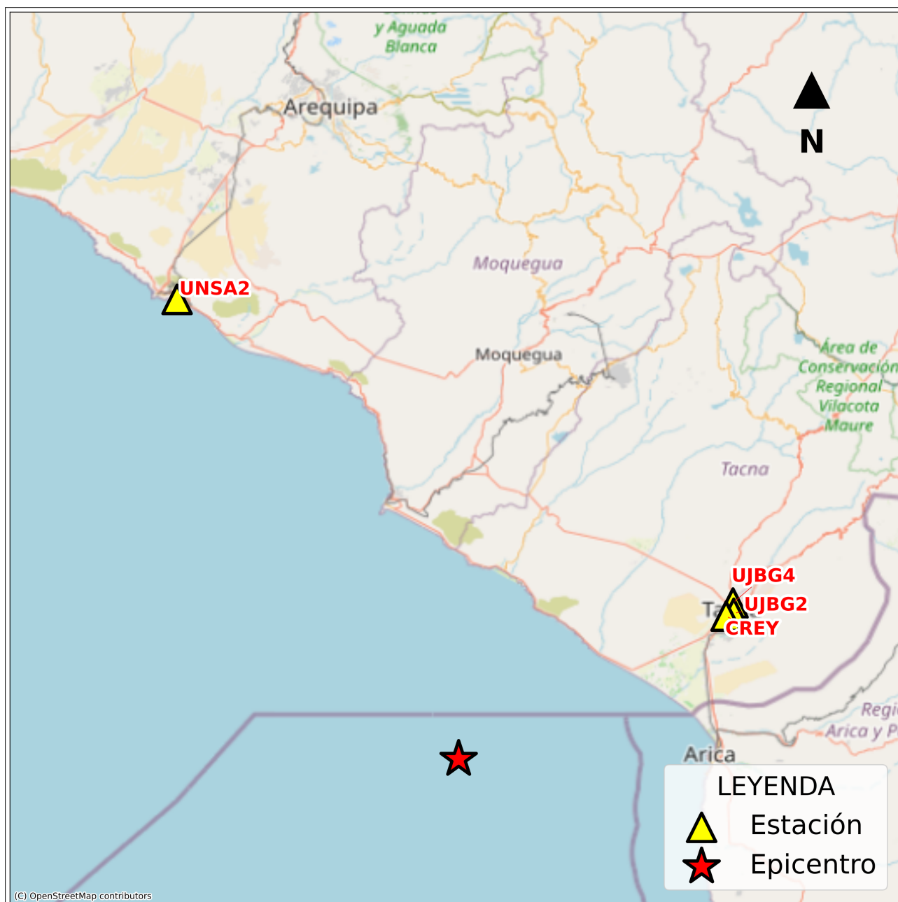
Figura 2: Mapa de ubicación de la(s) estación(es) acelerográfica(s) correspondiente(s) al Sismo de Ilo, Ilo - Moquegua del 21 de agosto de 2026 a las 15:39:40 (hora local)
