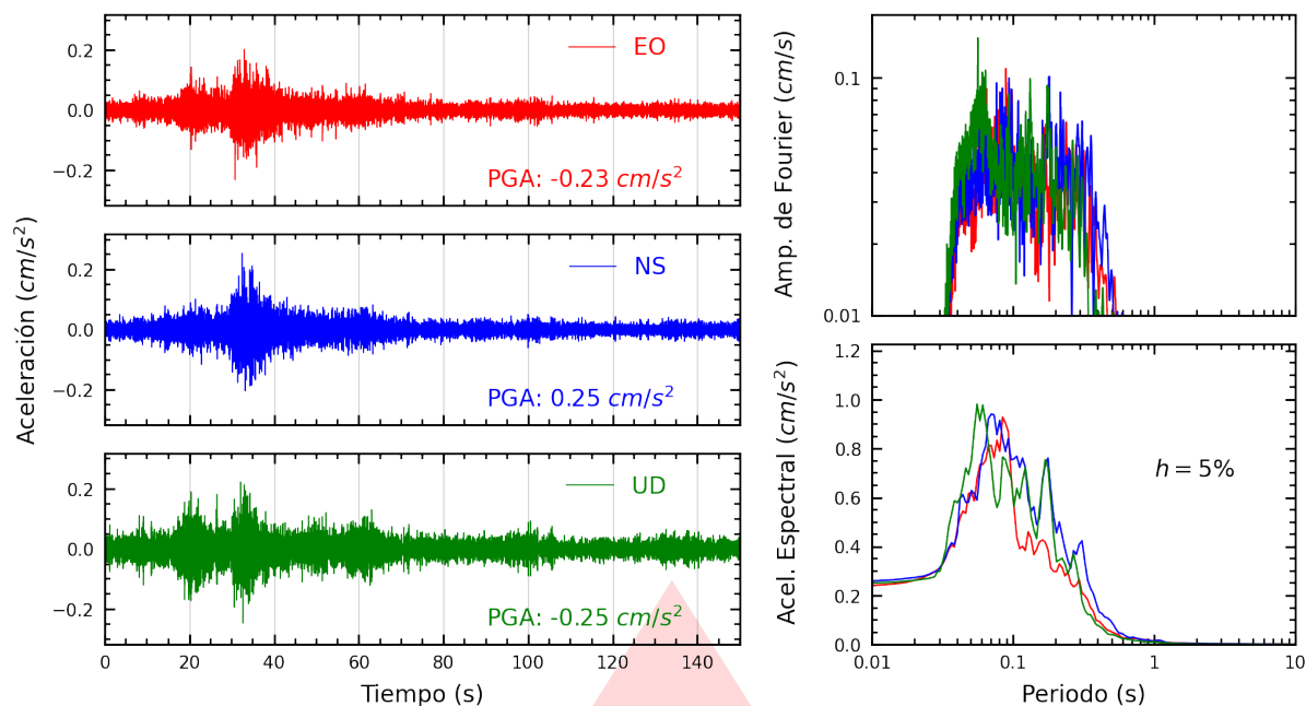
Figura A.3: Registros tiempo-historia, espectros de Fourier y de respuesta en las direcciones EO, NS y vertical de la estación UJBG2. Sismo de Ilo, Ilo - Moquegua del 2026-08-21, 15:39:40 (Hora local)
