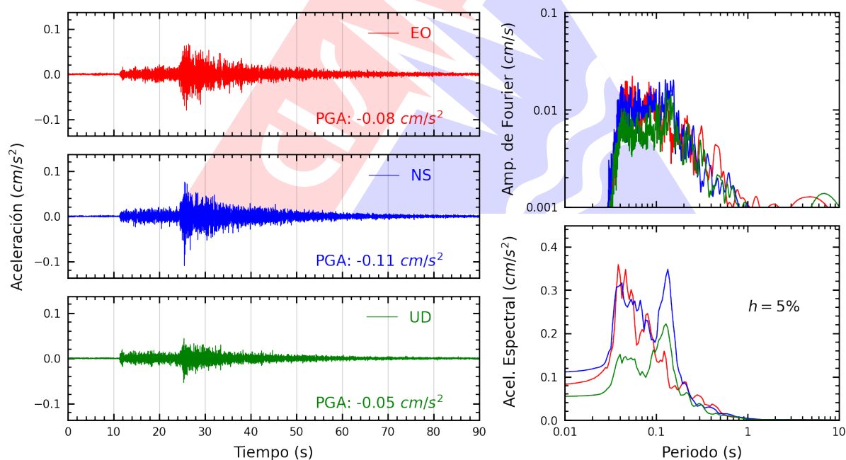
Figura A.4: Registros tiempo-historia, espectros de Fourier y de respuesta en las direcciones EO, NS y vertical de la estación UNSA2. Sismo de Ilo, Ilo - Moquegua del 2026-08-21, 18:23:52 (Hora local)
