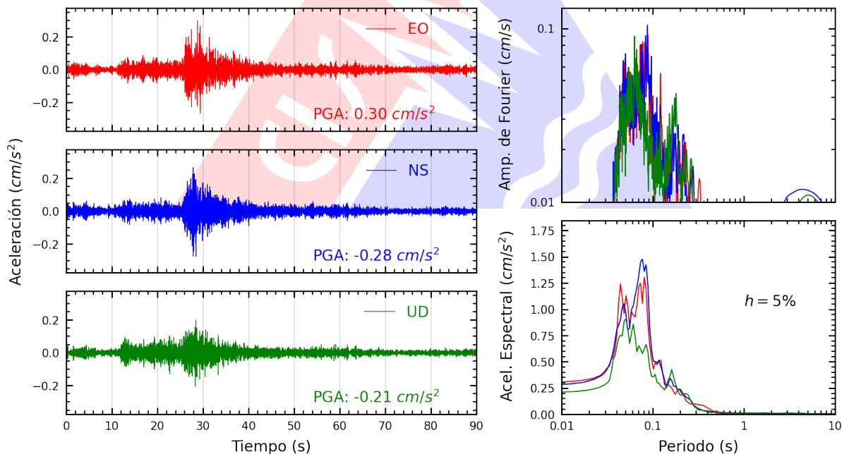
Figura A.2: Registros tiempo-historia, espectros de Fourier y de respuesta en las direcciones EO, NS y vertical de la estación CREY. Sismo de Ilo, Ilo - Moquegua del 2026-08-21, 18:23:52 (Hora local)
