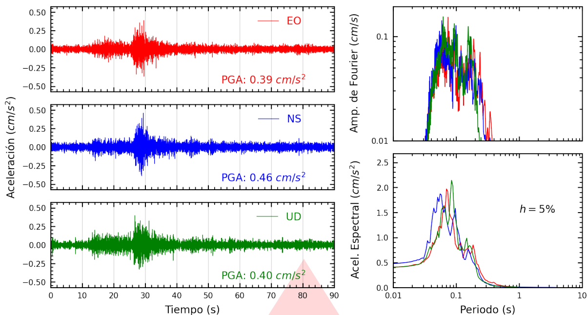
Figura A.1: Registros tiempo-historia, espectros de Fourier y de respuesta en las direcciones EO, NS y vertical de la estación UJBG4. Sismo de Ilo, Ilo - Moquegua del 2026-08-21, 18:23:52 (Hora local)
