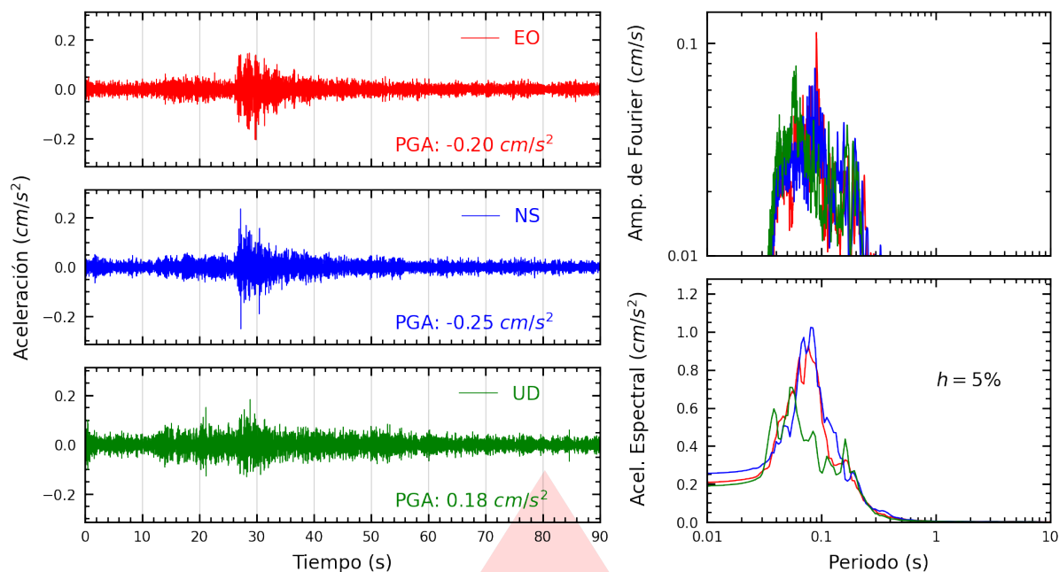
Figura A.3: Registros tiempo-historia, espectros de Fourier y de respuesta en las direcciones EO, NS y vertical de la estación UJBG2. Sismo de Ilo, Ilo - Moquegua del 2026-08-21, 18:23:52 (Hora local)
