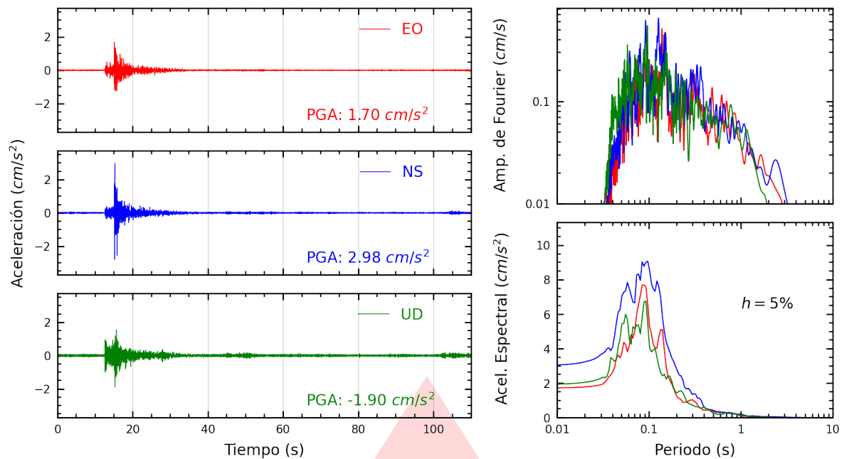
Figura A.1: Registros tiempo-historia, espectros de Fourier y de respuesta en las direcciones EO, NS y vertical de la estación SCHYO. Sismo de Chupaca, Chupaca - Junín del 2026-08-24, 14:40:18 (Hora local)
