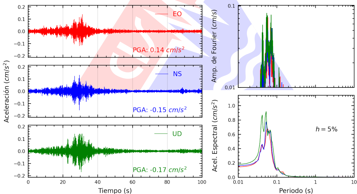
Figura A.2: Registros tiempo-historia, espectros de Fourier y de respuesta en las direcciones EO, NS y vertical de la estación ASIA. Sismo de Chupaca, Chupaca - Junín del 2026-08-25, 21:51:19 (Hora local)
