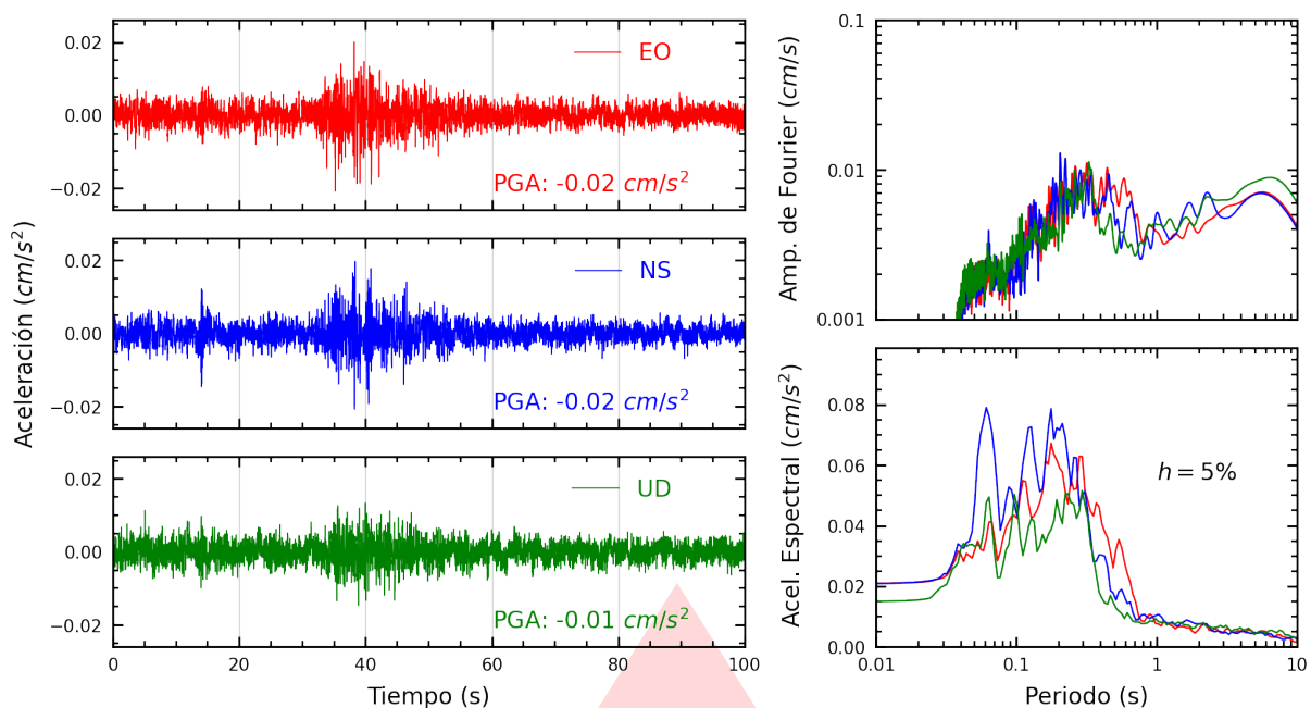
Figura A.3: Registros tiempo-historia, espectros de Fourier y de respuesta en las direcciones EO, NS y vertical de la estación CARAL. Sismo de Chupaca, Chupaca - Junín del 2026-08-25, 21:51:19 (Hora local)
