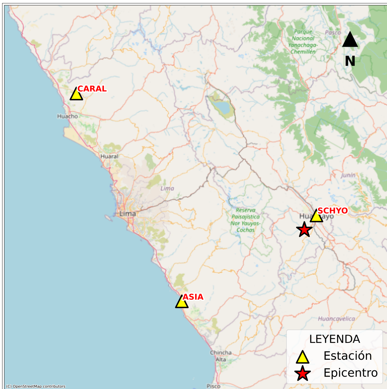
Figura 2: Mapa de ubicación de la(s) estación(es) acelerográfica(s) correspondiente(s) al Sismo de Chupaca, Chupaca - Junín del 25 de agosto de 2026 a las 21:51:19 (hora local)
