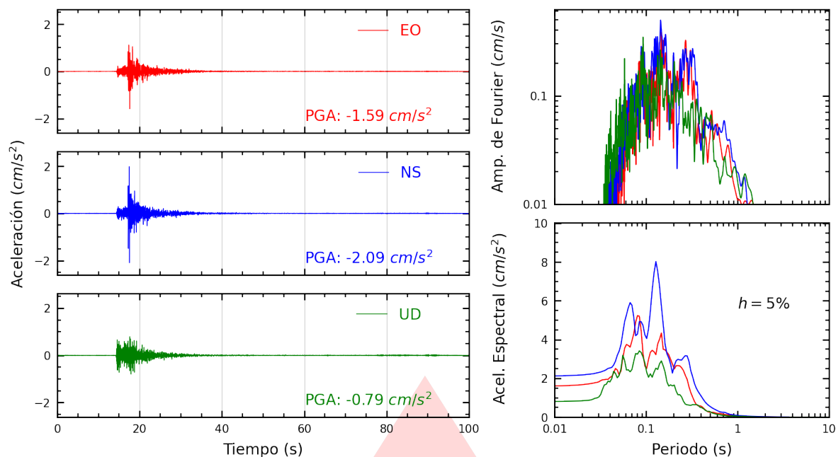
Figura A.1: Registros tiempo-historia, espectros de Fourier y de respuesta en las direcciones EO, NS y vertical de la estación SCHYO. Sismo de Chupaca, Chupaca - Junín del 2026-08-26, 02:40:09 (Hora local)
