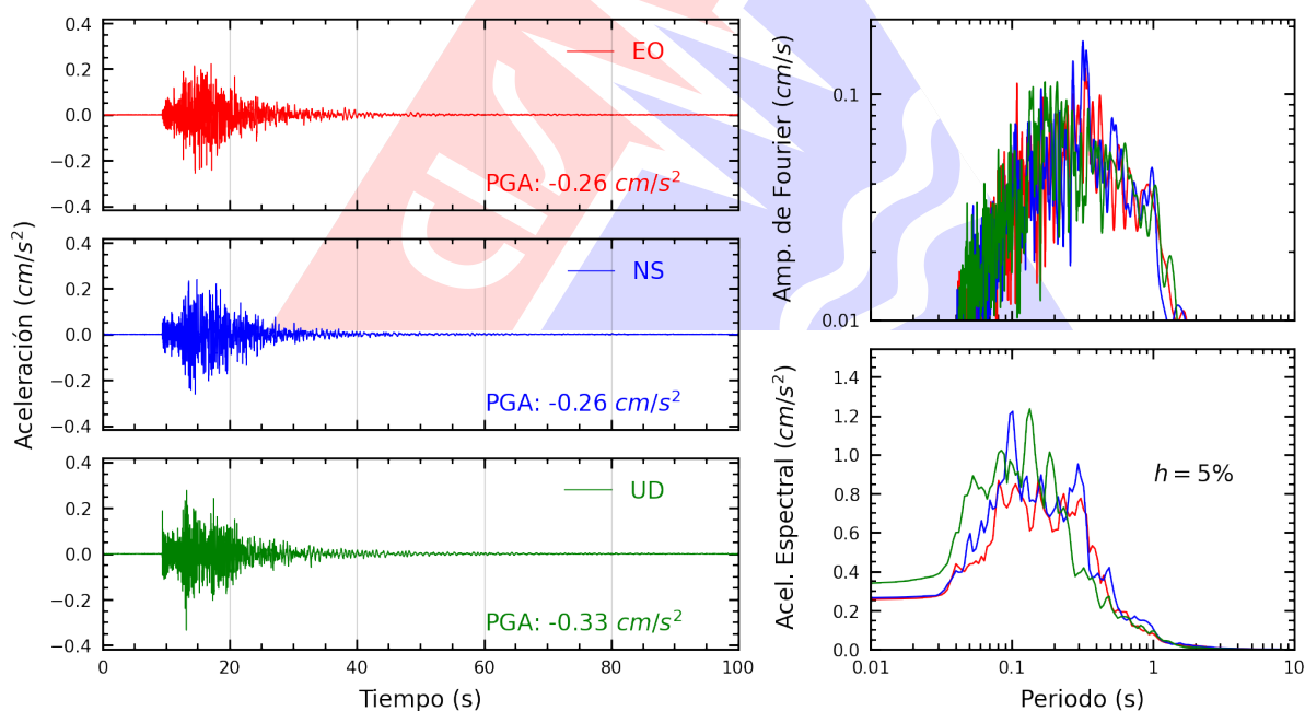
Figura A.2: Registros tiempo-historia, espectros de Fourier y de respuesta en las direcciones EO, NS y vertical de la estación UNCP. Sismo de Chupaca, Chupaca - Junín del 2026-08-26, 02:40:09 (Hora local)
