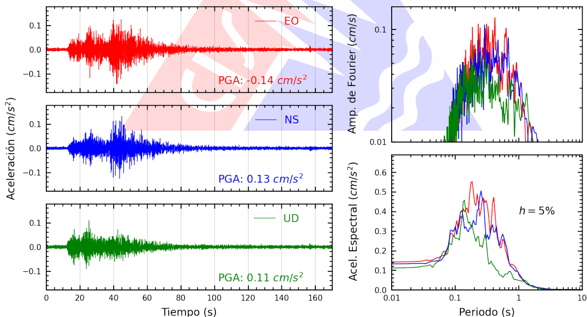
Figura A.2: Registros tiempo-historia, espectros de Fourier y de respuesta en las direcciones EO, NS y vertical de la estación UNC. Sismo de Pimentel, Chiclayo - Lambayeque del 2026-08-26, 23:04:18 (Hora local)
