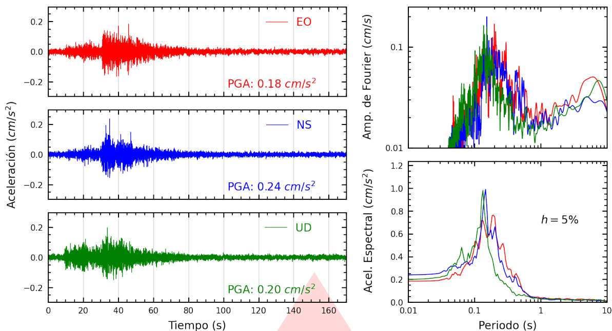
Figura A.1: Registros tiempo-historia, espectros de Fourier y de respuesta en las direcciones EO, NS y vertical de la estación UPAOT. Sismo de Pimentel, Chiclayo - Lambayeque del 2026-08-26, 23:04:18 (Hora local)
