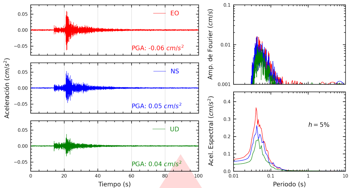
Figura A.1: Registros tiempo-historia, espectros de Fourier y de respuesta en las direcciones EO, NS y vertical de la estación UNSA2. Sismo de Vitor, Arequipa - Arequipa del 2026-08-27, 23:55:03 (Hora local)
