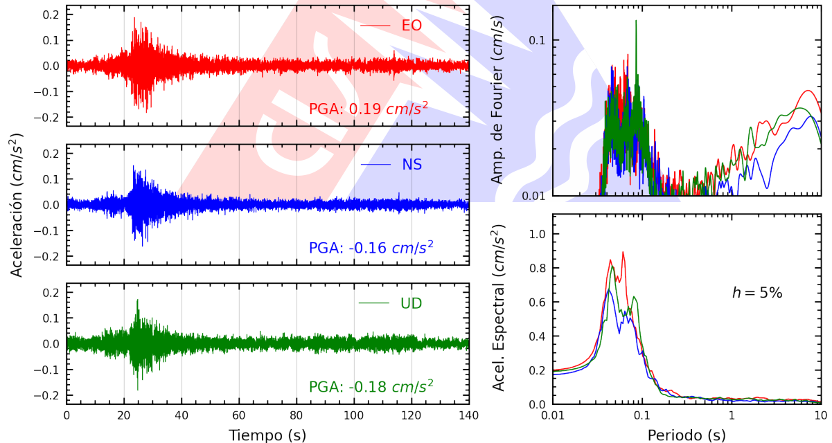
Figura A.2: Registros tiempo-historia, espectros de Fourier y de respuesta en las direcciones EO, NS y vertical de la estación AMORE. Sismo de Chilca, Cañete - Lima del 2026-08-28, 08:19:54 (Hora local)
