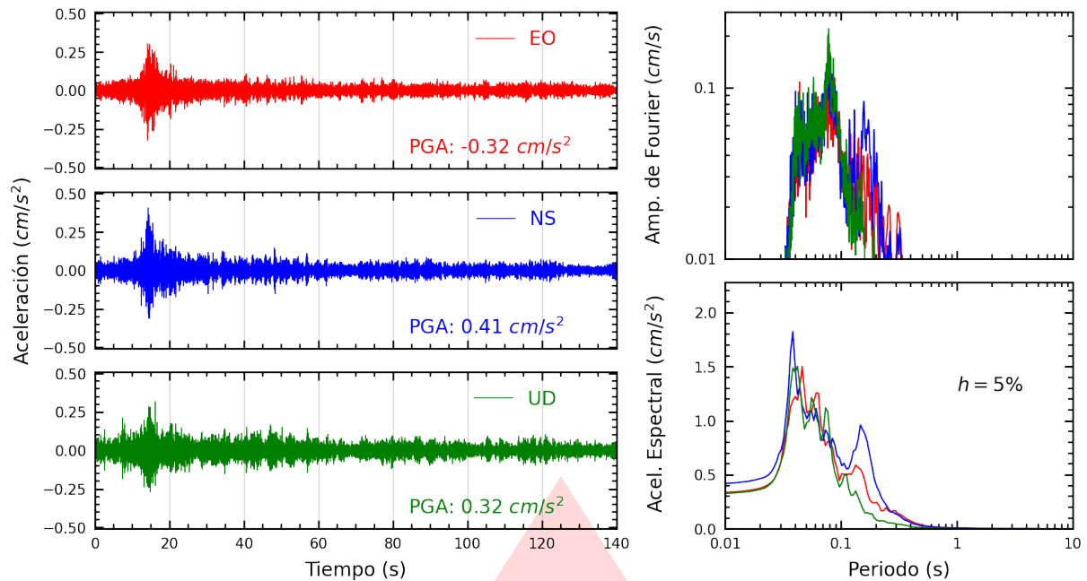
Figura A.1: Registros tiempo-historia, espectros de Fourier y de respuesta en las direcciones EO, NS y vertical de la estación ASIA. Sismo de Chilca, Cañete - Lima del 2026-08-28, 08:19:54 (Hora local)
