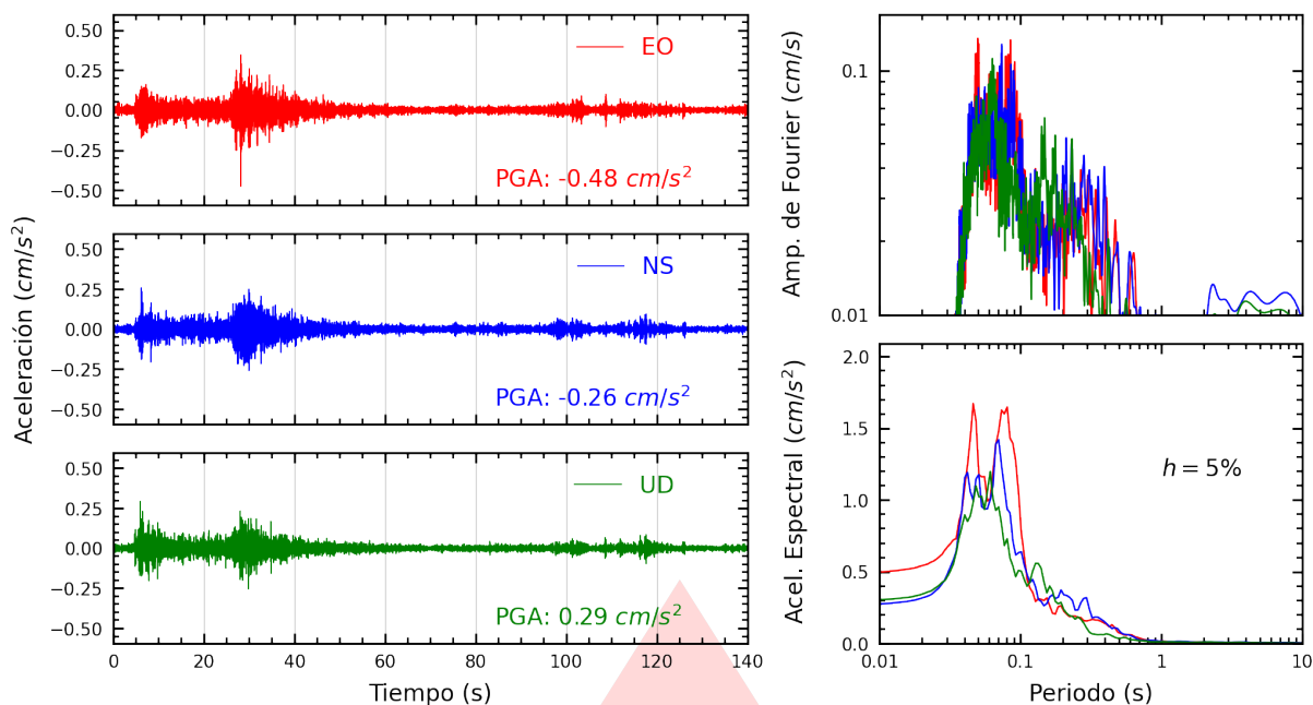
Figura A.1: Registros tiempo-historia, espectros de Fourier y de respuesta en las direcciones EO, NS y vertical de la estación CREY. Sismo de Tacna, Tacna - Tacna del 2026-08-28, 12:53:26 (Hora local)
