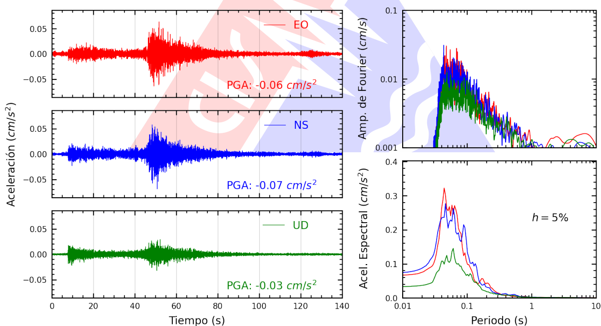
Figura A.4: Registros tiempo-historia, espectros de Fourier y de respuesta en las direcciones EO, NS y vertical de la estación UNSA2. Sismo de Tacna, Tacna - Tacna del 2026-08-28, 12:53:26 (Hora local)
