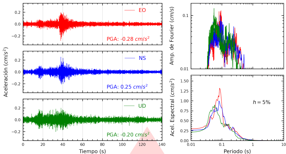
Figura A.3: Registros tiempo-historia, espectros de Fourier y de respuesta en las direcciones EO, NS y vertical de la estación UJBG2. Sismo de Tacna, Tacna - Tacna del 2026-08-28, 12:53:26 (Hora local)
