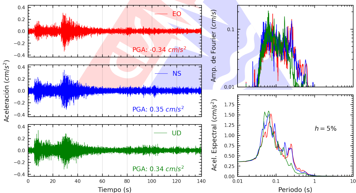
Figura A.2: Registros tiempo-historia, espectros de Fourier y de respuesta en las direcciones EO, NS y vertical de la estación UJBG4. Sismo de Tacna, Tacna - Tacna del 2026-08-28, 12:53:26 (Hora local)
