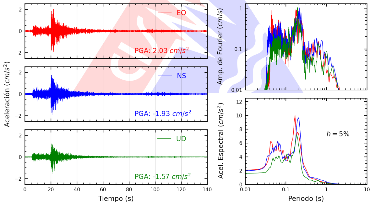
Figura A.4: Registros tiempo-historia, espectros de Fourier y de respuesta en las direcciones EO, NS y vertical de la estación UPTAC. Sismo de Tacna, Tacna - Tacna del 2026-08-28, 15:44:37 (Hora local)
