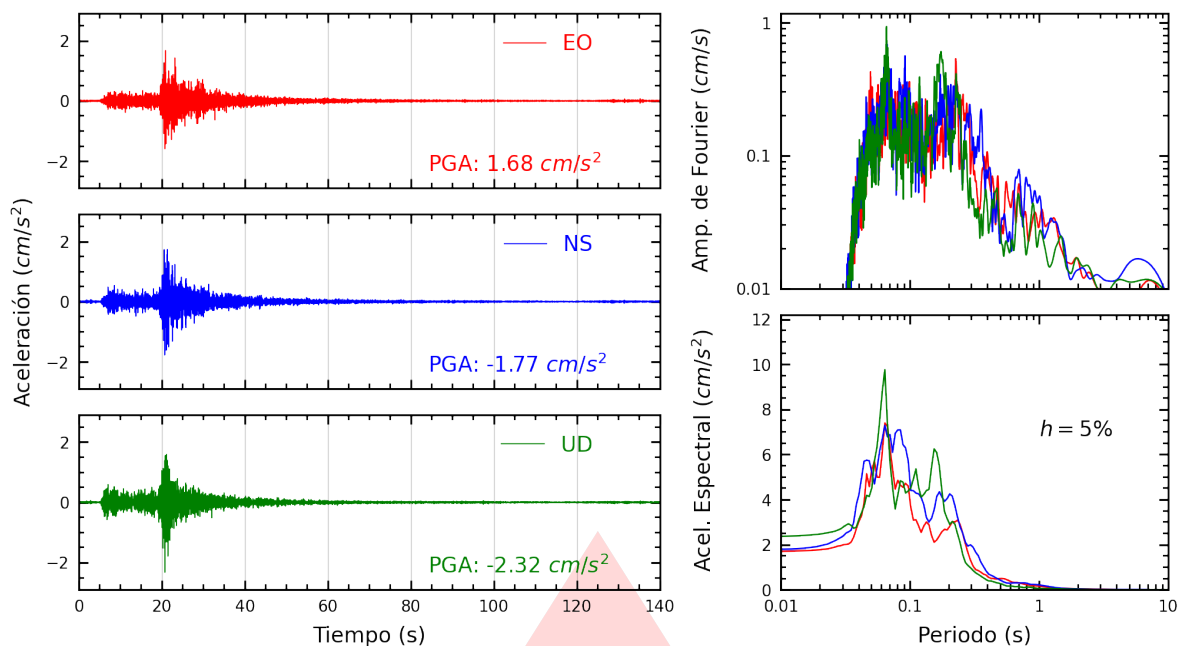
Figura A.3: Registros tiempo-historia, espectros de Fourier y de respuesta en las direcciones EO, NS y vertical de la estación CREY. Sismo de Tacna, Tacna - Tacna del 2026-08-28, 15:44:37 (Hora local)
