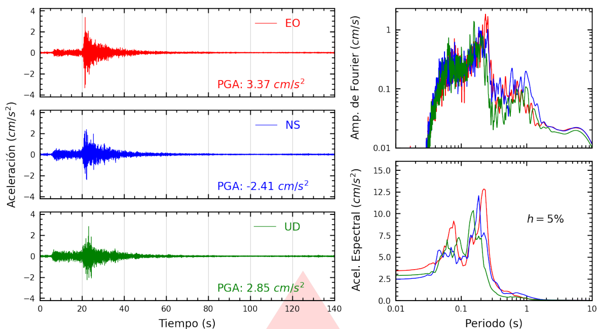
Figura A.1: Registros tiempo-historia, espectros de Fourier y de respuesta en las direcciones EO, NS y vertical de la estación UJBG4. Sismo de Tacna, Tacna - Tacna del 2026-08-28, 15:44:37 (Hora local)
