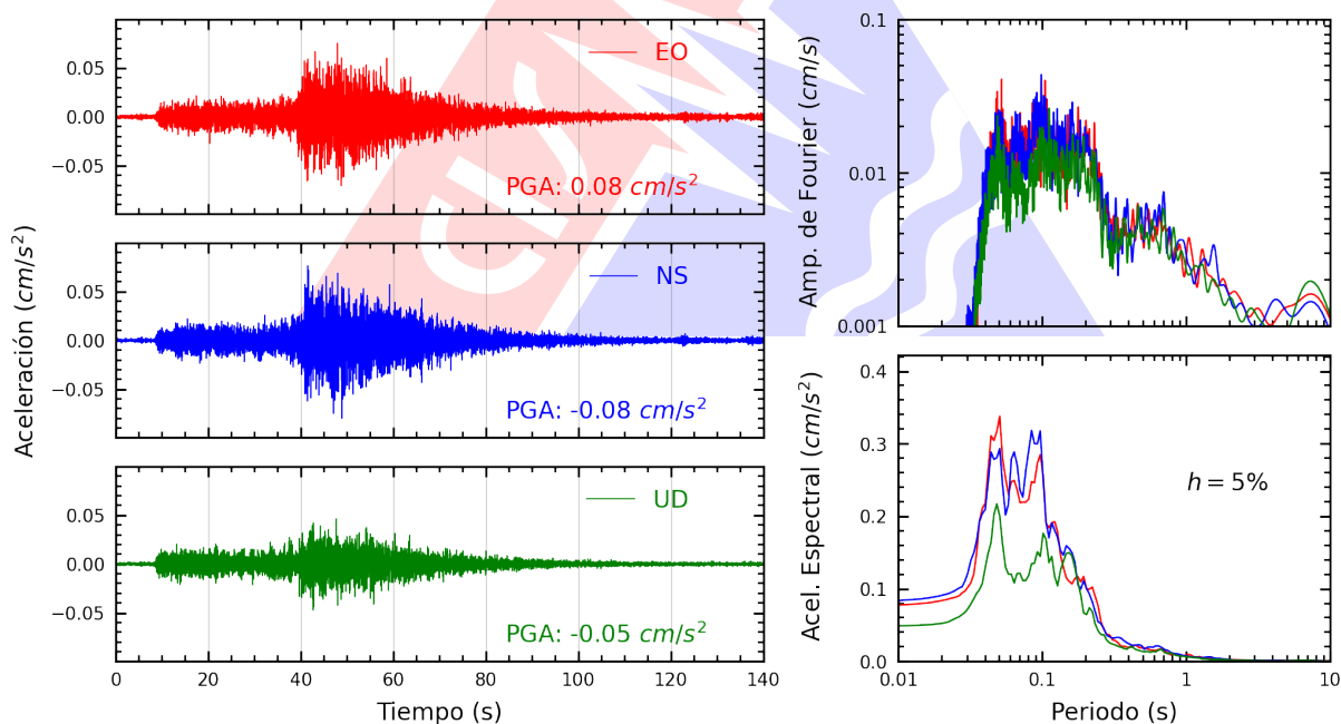
Figura A.6: Registros tiempo-historia, espectros de Fourier y de respuesta en las direcciones EO, NS y vertical de la estación UNSA2. Sismo de Tacna, Tacna - Tacna del 2026-08-28, 15:44:37 (Hora local)
