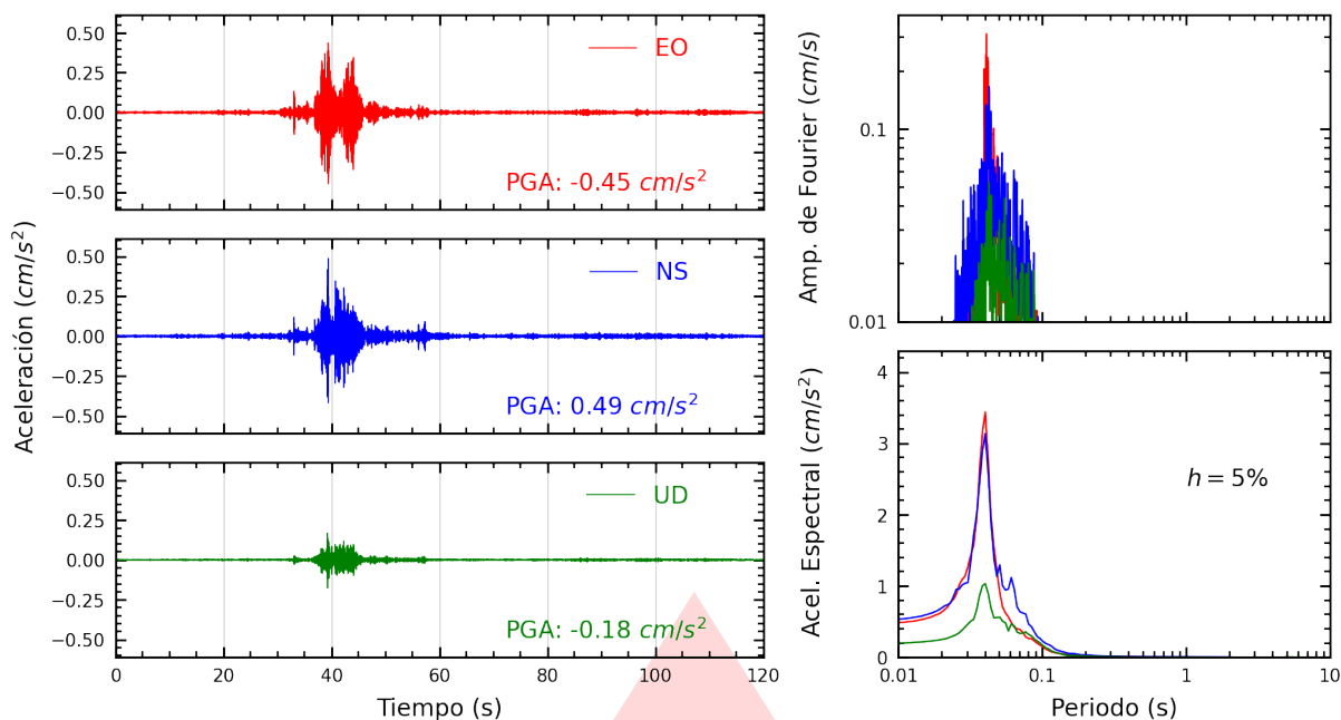
Figura A.1: Registros tiempo-historia, espectros de Fourier y de respuesta en las direcciones EO, NS y vertical de la estación UNAM. Sismo de Tuti, Caylloma - Arequipa del 2026-08-29, 15:46:06 (Hora local)
