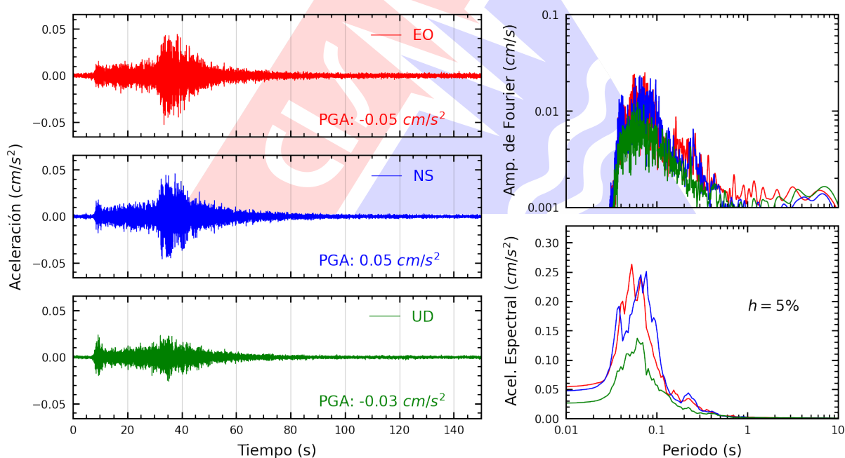
Figura A.2: Registros tiempo-historia, espectros de Fourier y de respuesta en las direcciones EO, NS y vertical de la estación UNSA2. Sismo de Tuti, Caylloma - Arequipa del 2026-08-29, 15:46:06 (Hora local)
