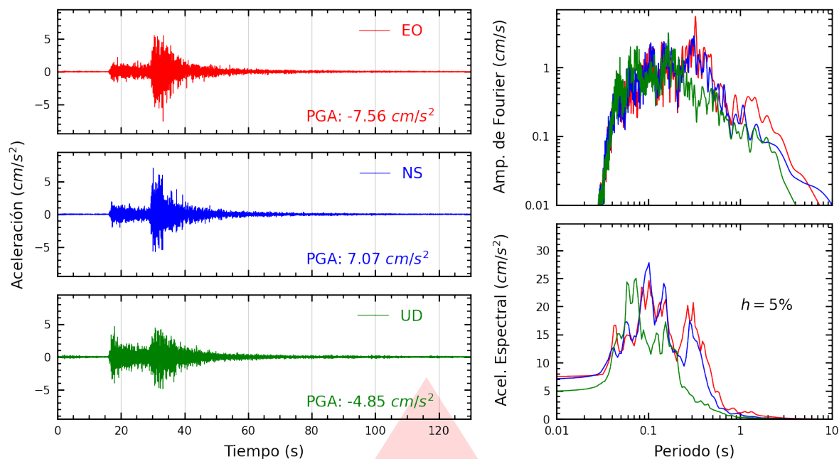
Figura A.3: Registros tiempo-historia, espectros de Fourier y de respuesta en las direcciones EO, NS y vertical de la estación SCTAC. Sismo de Tacna, Tacna - Tacna del 2026-08-30, 11:04:09 (Hora local)
