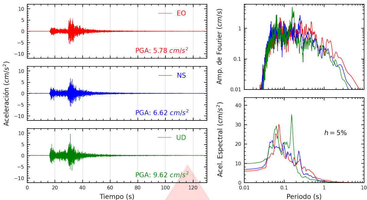
Figura A.1: Registros tiempo-historia, espectros de Fourier y de respuesta en las direcciones EO, NS y vertical de la estación UJBG4. Sismo de Tacna, Tacna - Tacna del 2026-08-30, 11:04:09 (Hora local)
