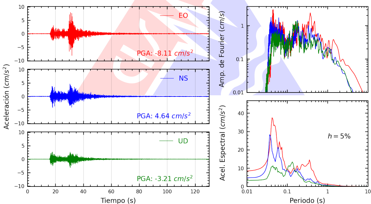
Figura A.2: Registros tiempo-historia, espectros de Fourier y de respuesta en las direcciones EO, NS y vertical de la estación UPTAC. Sismo de Tacna, Tacna - Tacna del 2026-08-30, 11:04:09 (Hora local)
