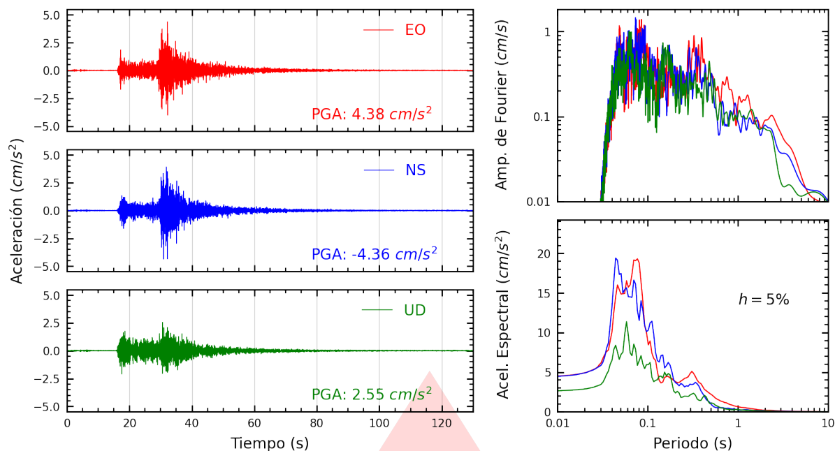
Figura A.5: Registros tiempo-historia, espectros de Fourier y de respuesta en las direcciones EO, NS y vertical de la estación CREY. Sismo de Tacna, Tacna - Tacna del 2026-08-30, 11:04:09 (Hora local)
