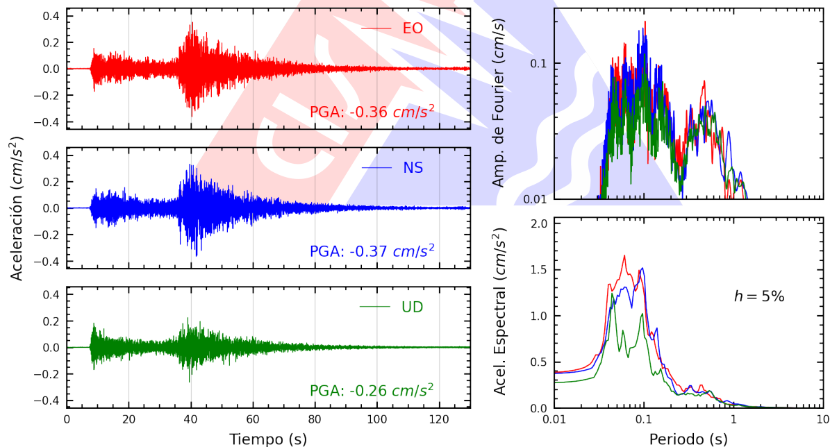
Figura A.6: Registros tiempo-historia, espectros de Fourier y de respuesta en las direcciones EO, NS y vertical de la estación UNSA2. Sismo de Tacna, Tacna - Tacna del 2026-08-30, 11:04:09 (Hora local)
