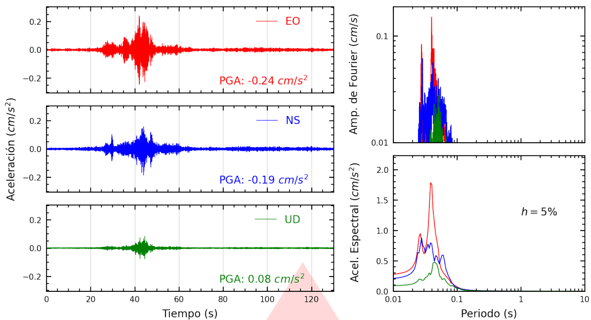
Figura A.7: Registros tiempo-historia, espectros de Fourier y de respuesta en las direcciones EO, NS y vertical de la estación UNAM. Sismo de Tacna, Tacna - Tacna del 2026-08-30, 11:04:09 (Hora local)
