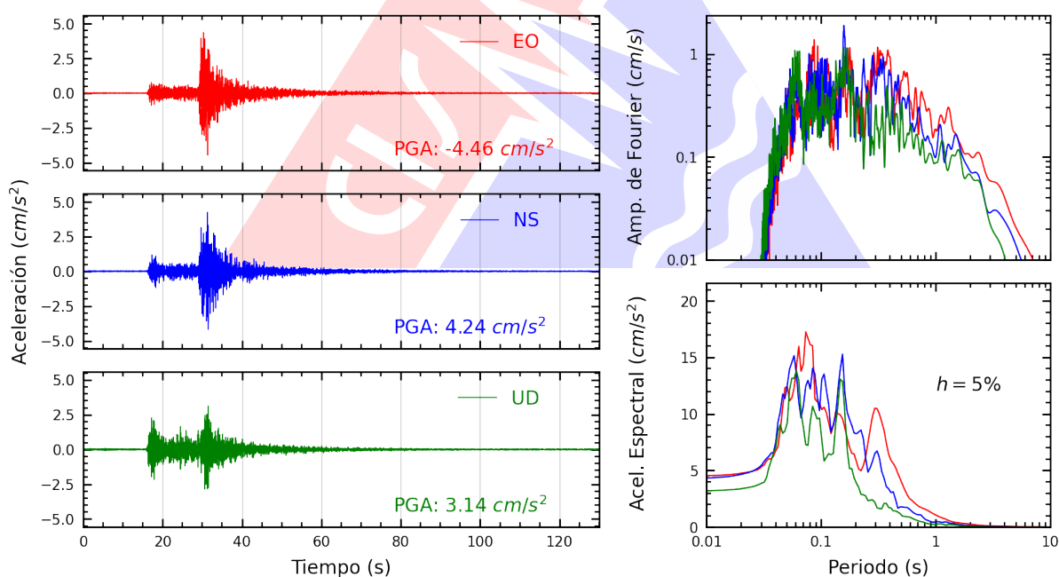
Figura A.4: Registros tiempo-historia, espectros de Fourier y de respuesta en las direcciones EO, NS y vertical de la estación UJBG2. Sismo de Tacna, Tacna - Tacna del 2026-08-30, 11:04:09 (Hora local)
