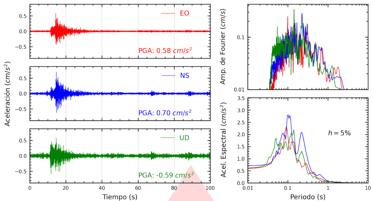
Figura A.1: Registros tiempo-historia, espectros de Fourier y de respuesta en las direcciones EO, NS y vertical de la estación SCHYO. Sismo de Chupaca, Chupaca - Junín del 2026-08-30, 12:42:28 (Hora local)
