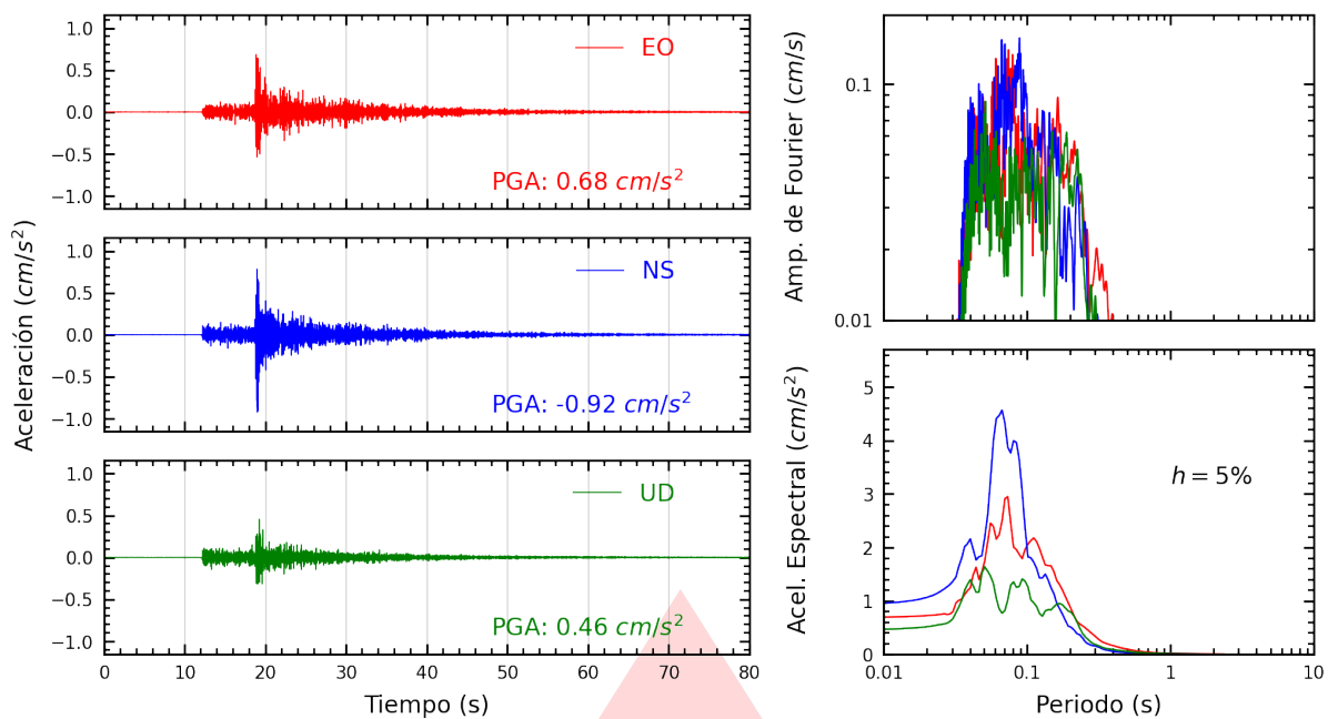
Figura A.1: Registros tiempo-historia, espectros de Fourier y de respuesta en las direcciones EO, NS y vertical de la estación UNSA2. Sismo de Quilca, Camaná - Arequipa del 2026-08-31, 00:48:31 (Hora local)
