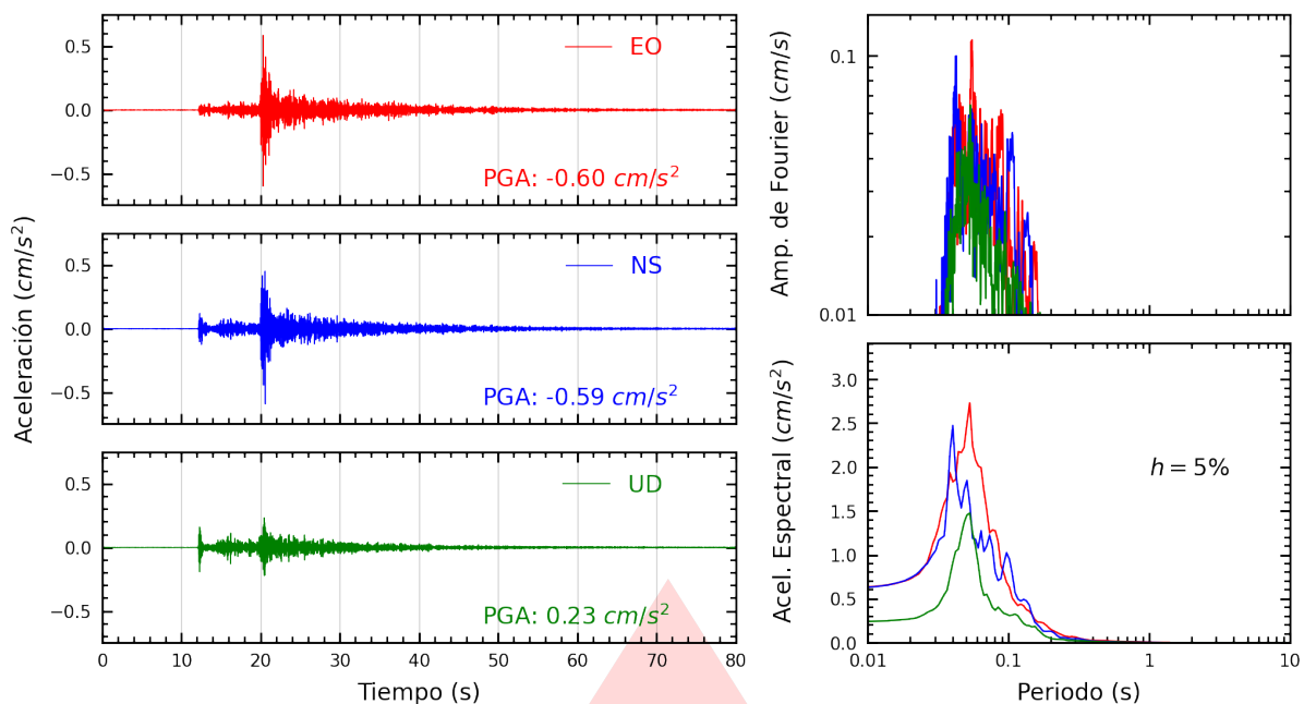
Figura A.1: Registros tiempo-historia, espectros de Fourier y de respuesta en las direcciones EO, NS y vertical de la estación UNSA2. Sismo de La Capilla, General Sánchez Cerro - Moquegua del 2026-08-31, 03:22:31 (Hora local)
