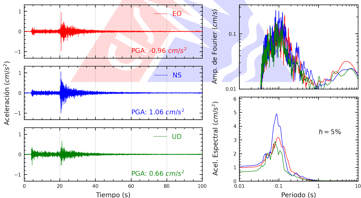
Figura A.12: Registros tiempo-historia, espectros de Fourier y de respuesta en las direcciones EO, NS y vertical de la estación SERVI. Sismo de Canta, Canta - Lima del 2026-08-31, 05:36:50 (Hora local)
