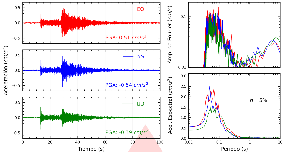
Figura A.25: Registros tiempo-historia, espectros de Fourier y de respuesta en las direcciones EO, NS y vertical de la estación UCSS. Sismo de Canta, Canta - Lima del 2026-08-31, 05:36:50 (Hora local)
