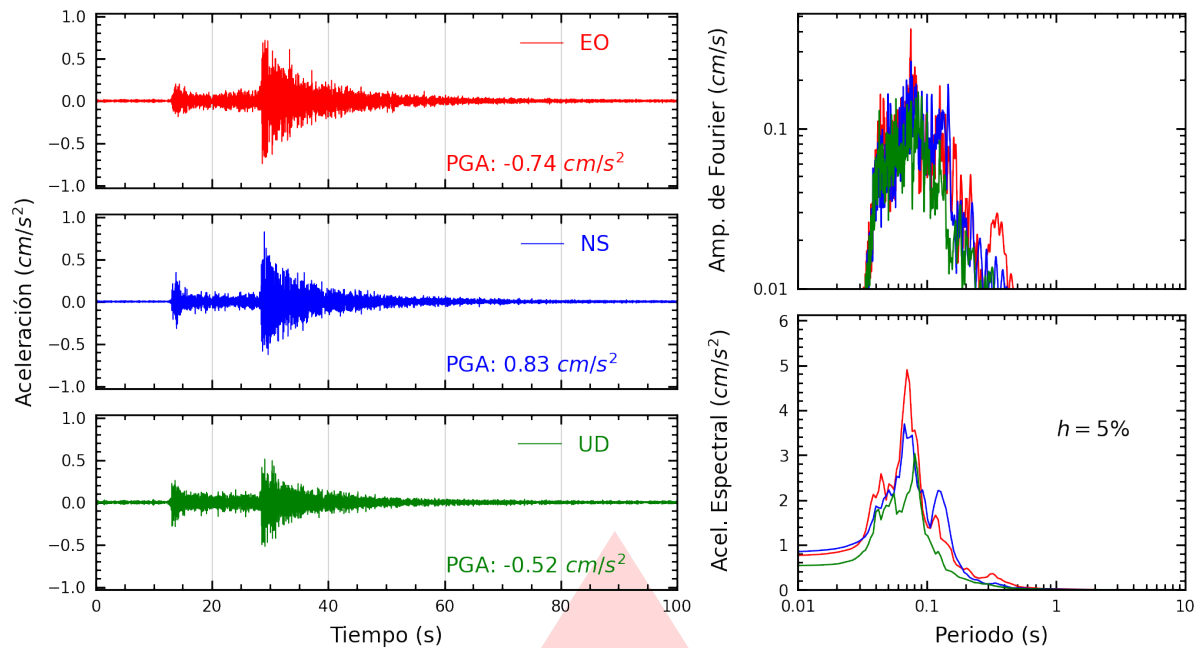
Figura A.15: Registros tiempo-historia, espectros de Fourier y de respuesta en las direcciones EO, NS y vertical de la estación ATARJ. Sismo de Canta, Canta - Lima del 2026-08-31, 05:36:50 (Hora local)
