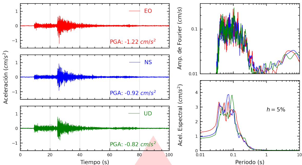
Figura A.9: Registros tiempo-historia, espectros de Fourier y de respuesta en las direcciones EO, NS y vertical de la estación USMP. Sismo de Canta, Canta - Lima del 2026-08-31, 05:36:50 (Hora local)
