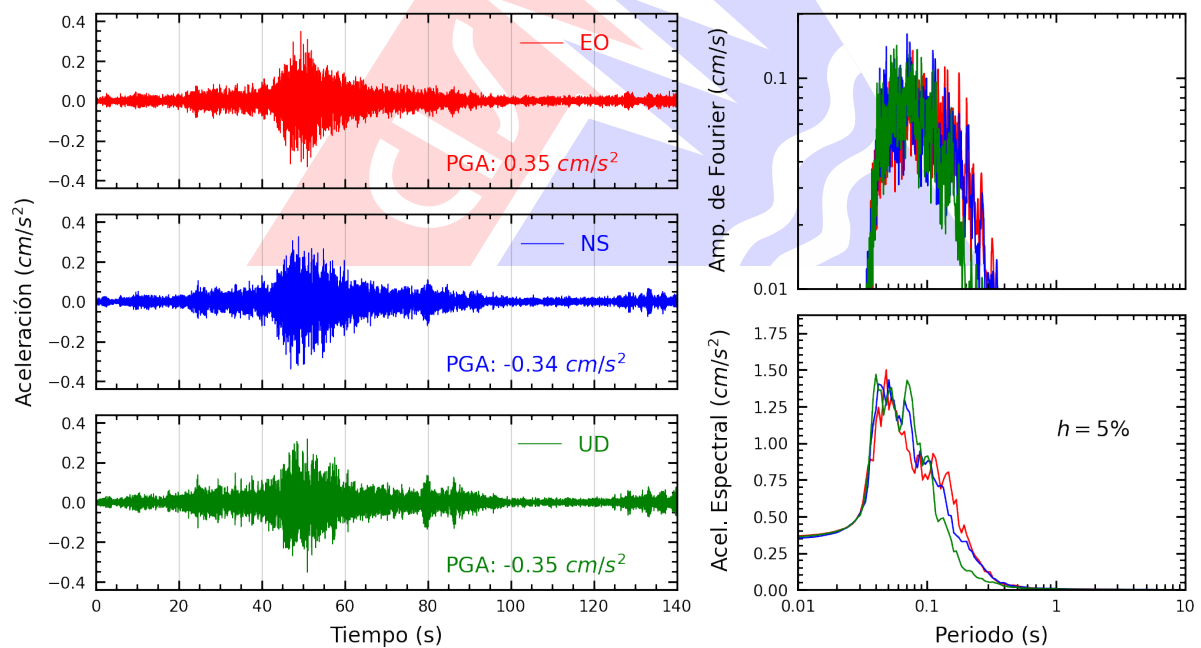
Figura A.30: Registros tiempo-historia, espectros de Fourier y de respuesta en las direcciones EO, NS y vertical de la estación ASIA. Sismo de Canta, Canta - Lima del 2026-08-31, 05:36:50 (Hora local)
