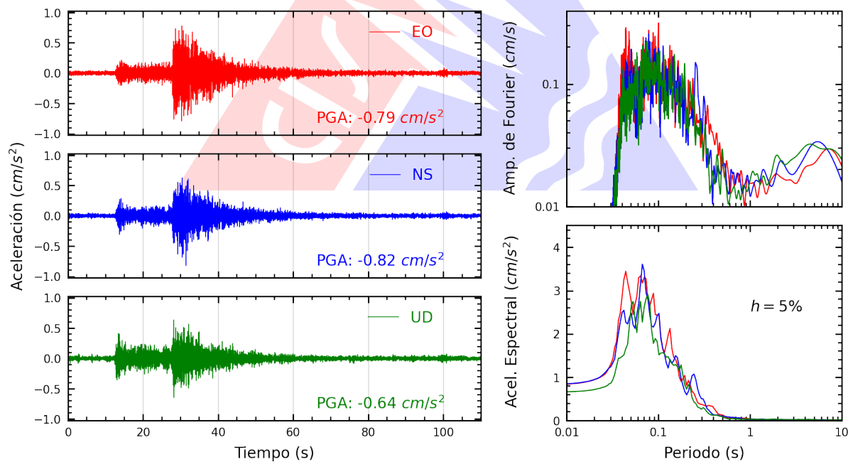
Figura A.16: Registros tiempo-historia, espectros de Fourier y de respuesta en las direcciones EO, NS y vertical de la estación UCVAT. Sismo de Canta, Canta - Lima del 2026-08-31, 05:36:50 (Hora local)
