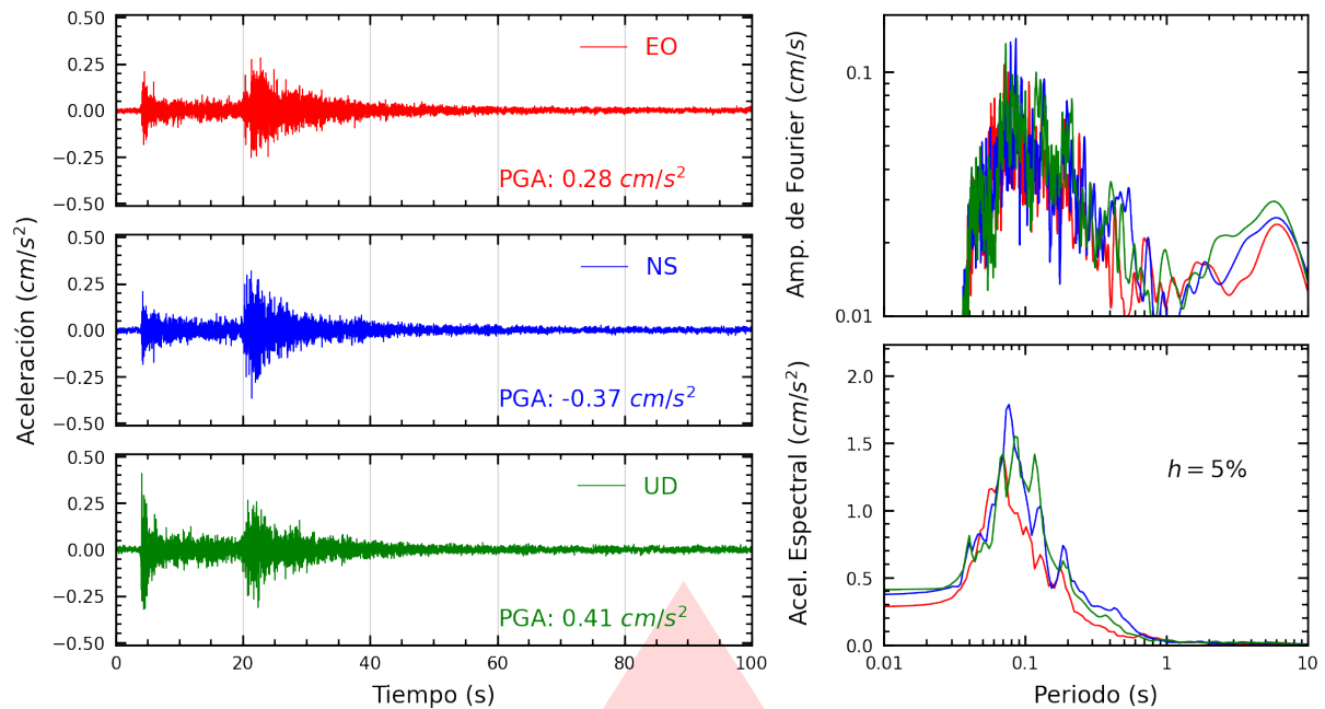
Figura A.29: Registros tiempo-historia, espectros de Fourier y de respuesta en las direcciones EO, NS y vertical de la estación UNFV. Sismo de Canta, Canta - Lima del 2026-08-31, 05:36:50 (Hora local)
