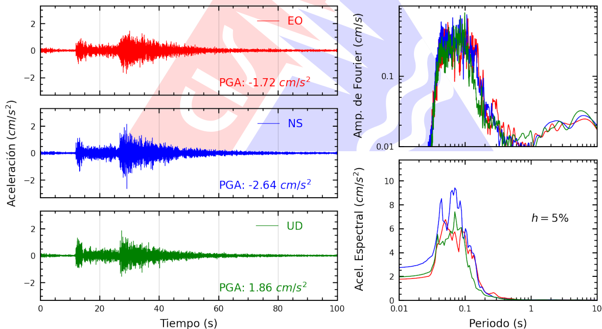
Figura A.2: Registros tiempo-historia, espectros de Fourier y de respuesta en las direcciones EO, NS y vertical de la estación SROSA. Sismo de Canta, Canta - Lima del 2026-08-31, 05:36:50 (Hora local)
