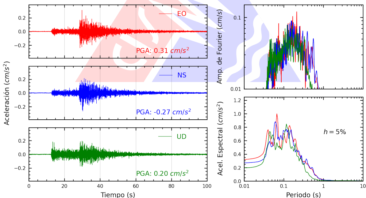
Figura A.32: Registros tiempo-historia, espectros de Fourier y de respuesta en las direcciones EO, NS y vertical de la estación CARAL. Sismo de Canta, Canta - Lima del 2026-08-31, 05:36:50 (Hora local)
