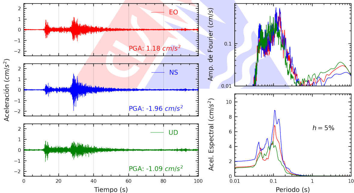
Figura A.6: Registros tiempo-historia, espectros de Fourier y de respuesta en las direcciones EO, NS y vertical de la estación CARAB. Sismo de Canta, Canta - Lima del 2026-08-31, 05:36:50 (Hora local)
