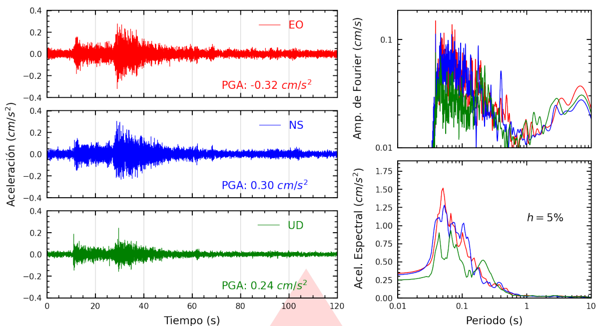
Figura A.31: Registros tiempo-historia, espectros de Fourier y de respuesta en las direcciones EO, NS y vertical de la estación UPCVI. Sismo de Canta, Canta - Lima del 2026-08-31, 05:36:50 (Hora local)
