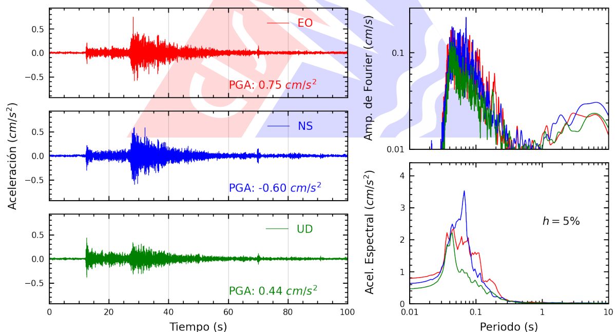
Figura A.20: Registros tiempo-historia, espectros de Fourier y de respuesta en las direcciones EO, NS y vertical de la estación SJLCE. Sismo de Canta, Canta - Lima del 2026-08-31, 05:36:50 (Hora local)
