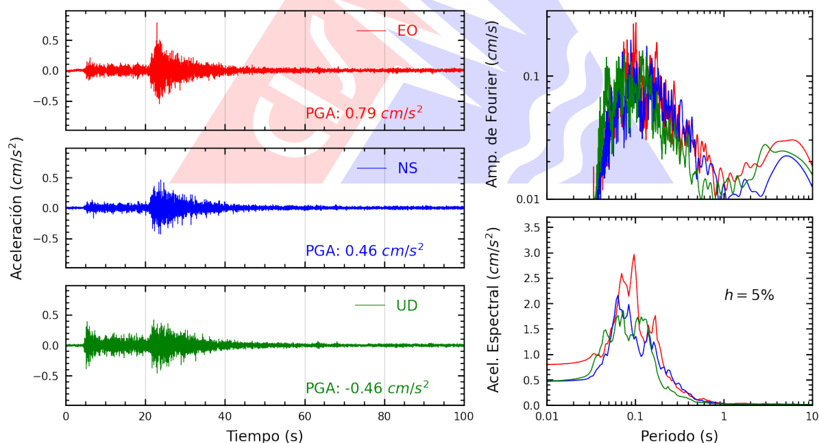
Figura A.18: Registros tiempo-historia, espectros de Fourier y de respuesta en las direcciones EO, NS y vertical de la estación USILP. Sismo de Canta, Canta - Lima del 2026-08-31, 05:36:50 (Hora local)
