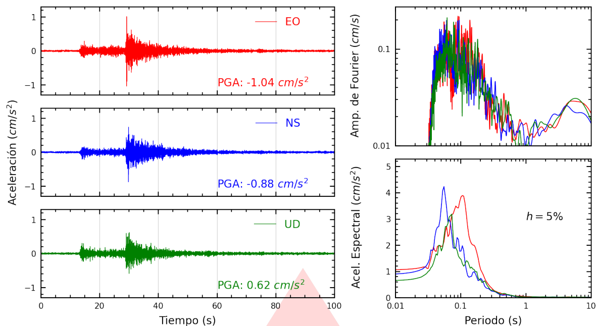
Figura A.13: Registros tiempo-historia, espectros de Fourier y de respuesta en las direcciones EO, NS y vertical de la estación IMCA. Sismo de Canta, Canta - Lima del 2026-08-31, 05:36:50 (Hora local)
