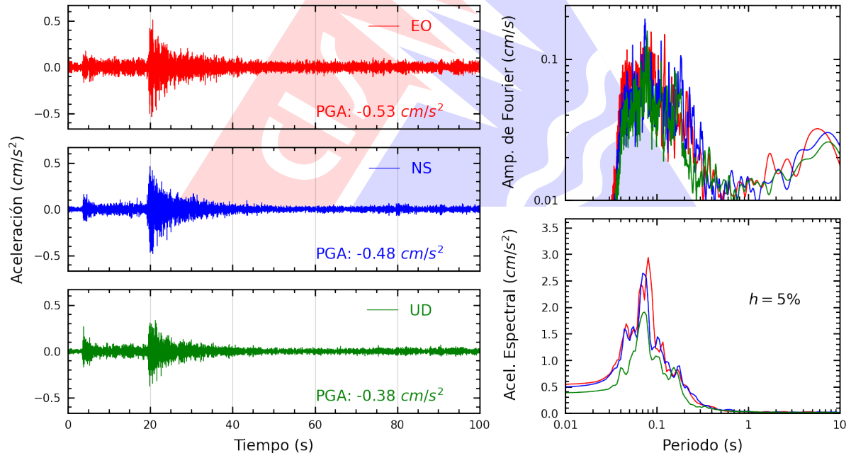
Figura A.26: Registros tiempo-historia, espectros de Fourier y de respuesta en las direcciones EO, NS y vertical de la estación INICT. Sismo de Canta, Canta - Lima del 2026-08-31, 05:36:50 (Hora local)
