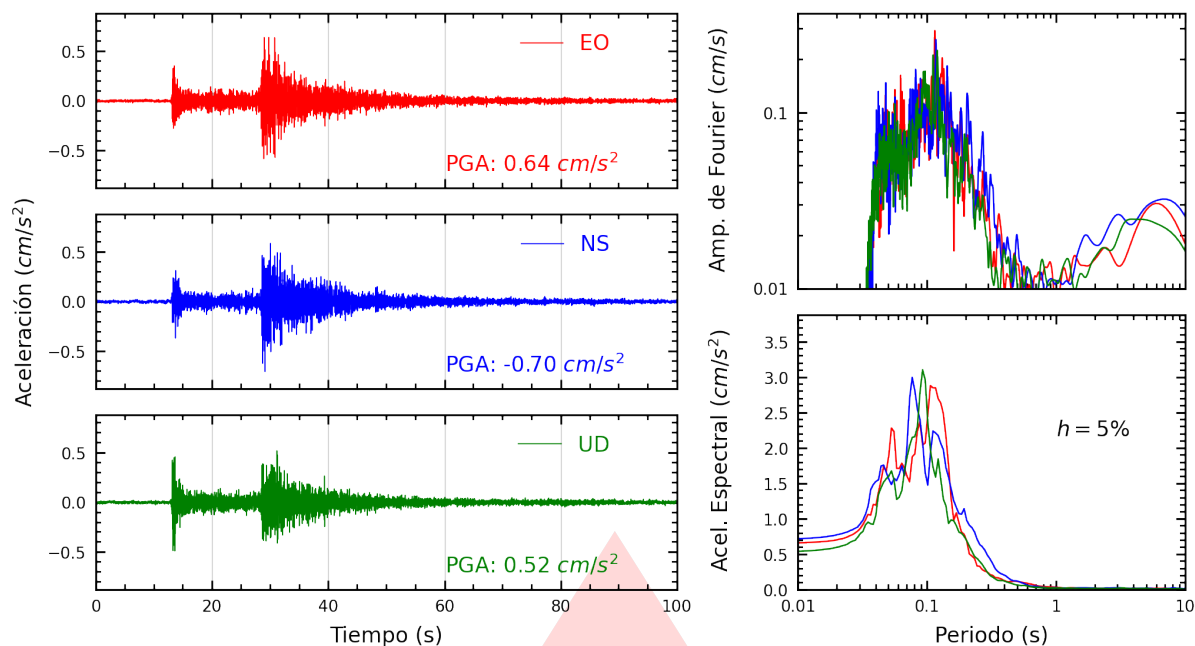
Figura A.21: Registros tiempo-historia, espectros de Fourier y de respuesta en las direcciones EO, NS y vertical de la estación JALVA. Sismo de Canta, Canta - Lima del 2026-08-31, 05:36:50 (Hora local)
