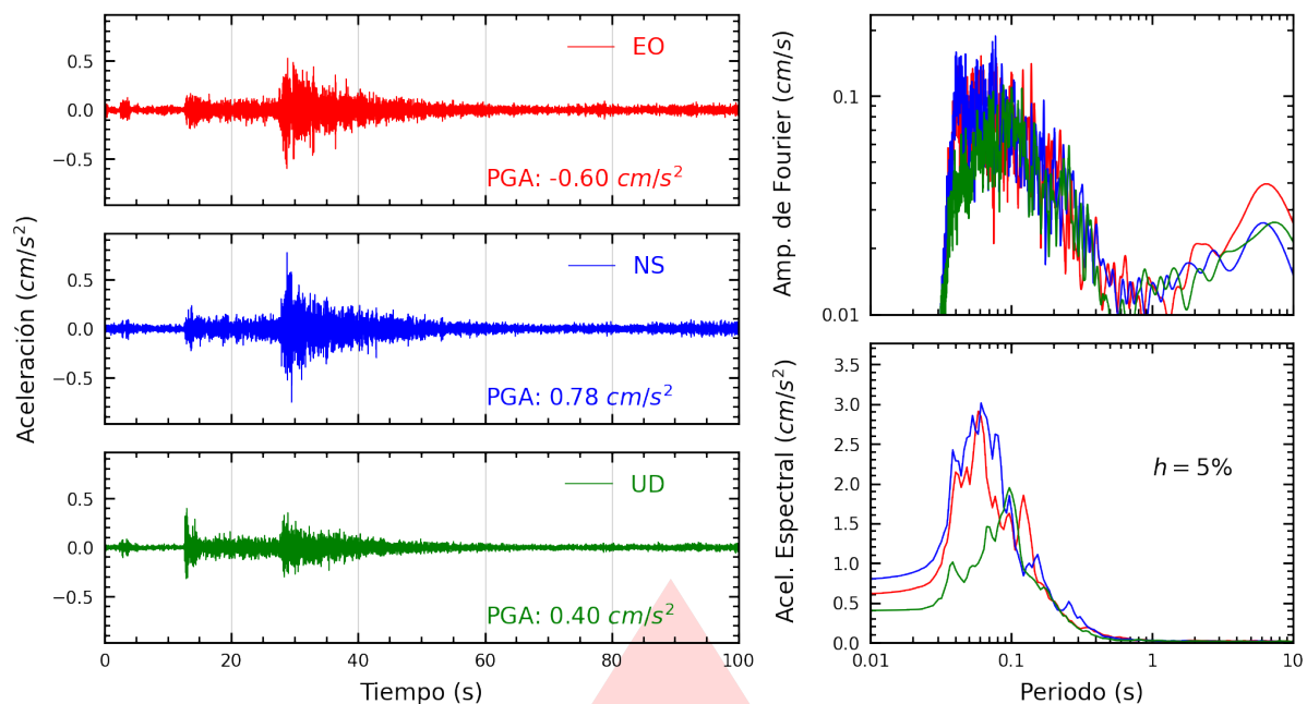
Figura A.19: Registros tiempo-historia, espectros de Fourier y de respuesta en las direcciones EO, NS y vertical de la estación COMAS. Sismo de Canta, Canta - Lima del 2026-08-31, 05:36:50 (Hora local)
