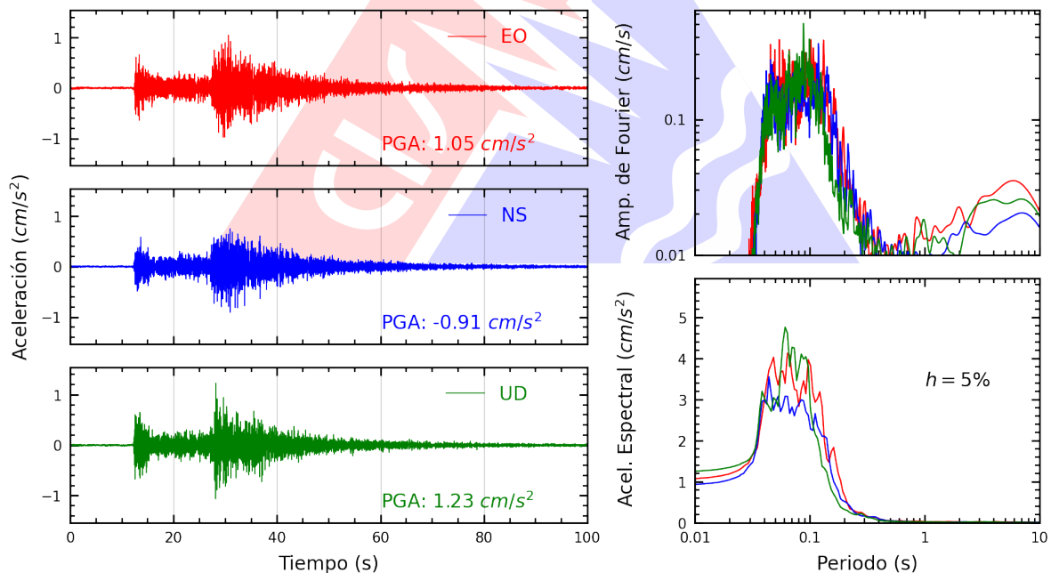
Figura A.8: Registros tiempo-historia, espectros de Fourier y de respuesta en las direcciones EO, NS y vertical de la estación AMORE. Sismo de Canta, Canta - Lima del 2026-08-31, 05:36:50 (Hora local)
