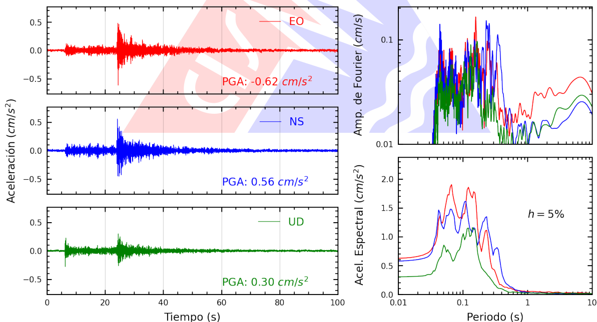
Figura A.24: Registros tiempo-historia, espectros de Fourier y de respuesta en las direcciones EO, NS y vertical de la estación UNAB. Sismo de Canta, Canta - Lima del 2026-08-31, 05:36:50 (Hora local)
