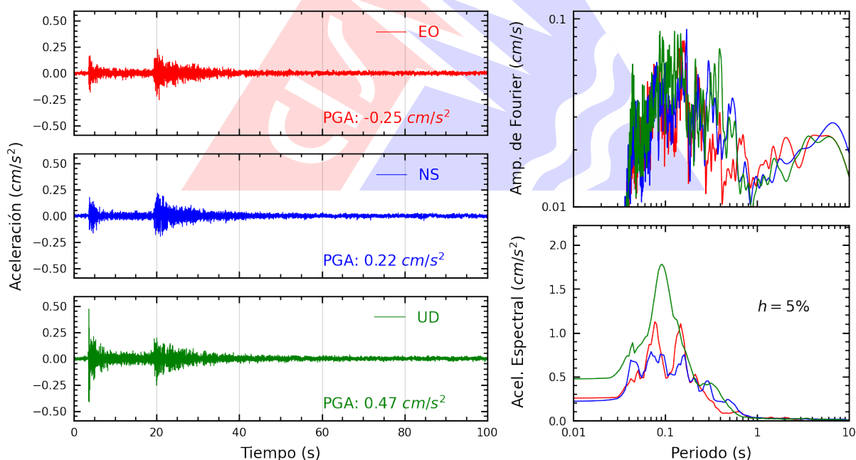
Figura A.28: Registros tiempo-historia, espectros de Fourier y de respuesta en las direcciones EO, NS y vertical de la estación BONDY. Sismo de Canta, Canta - Lima del 2026-08-31, 05:36:50 (Hora local)
