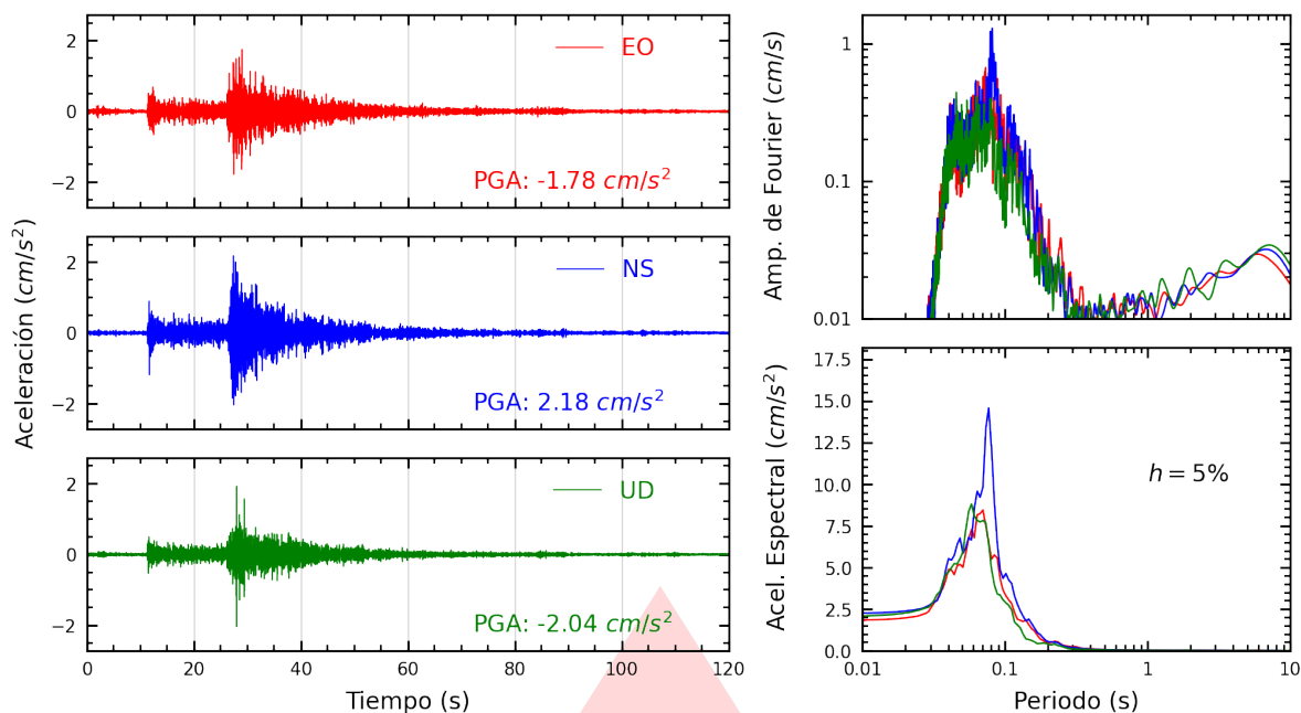
Figura A.3: Registros tiempo-historia, espectros de Fourier y de respuesta en las direcciones EO, NS y vertical de la estación JOSEO. Sismo de Canta, Canta - Lima del 2026-08-31, 05:36:50 (Hora local)
