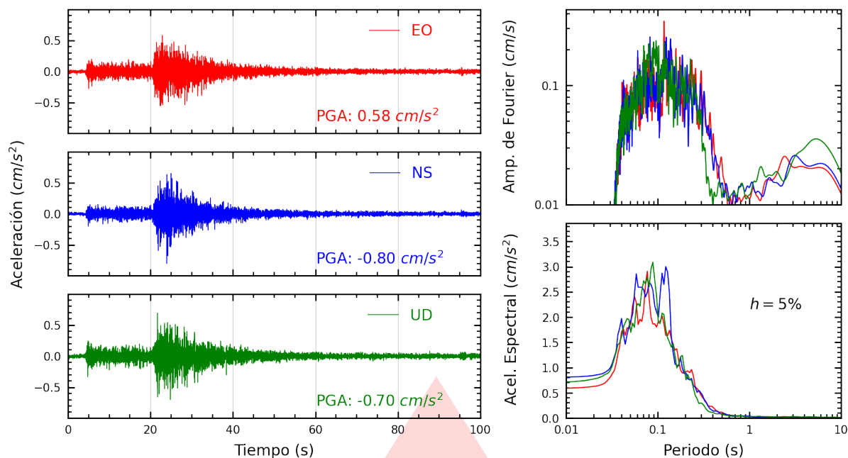
Figura A.17: Registros tiempo-historia, espectros de Fourier y de respuesta en las direcciones EO, NS y vertical de la estación SOVES. Sismo de Canta, Canta - Lima del 2026-08-31, 05:36:50 (Hora local)
