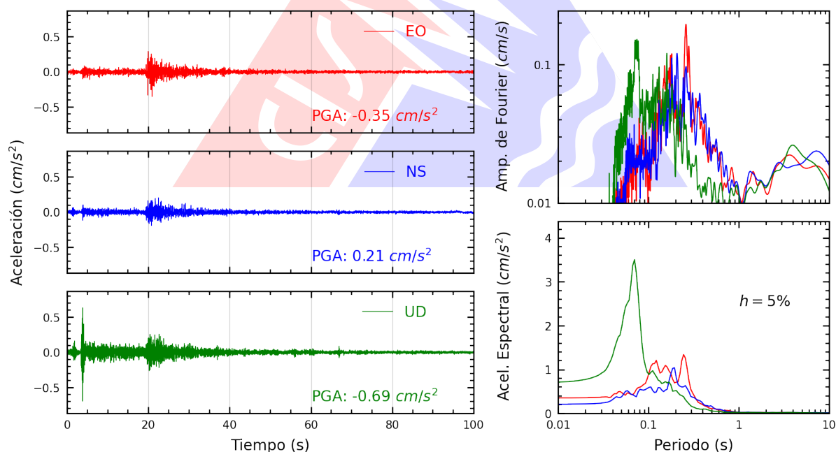
Figura A.22: Registros tiempo-historia, espectros de Fourier y de respuesta en las direcciones EO, NS y vertical de la estación ACAPU. Sismo de Canta, Canta - Lima del 2026-08-31, 05:36:50 (Hora local)
