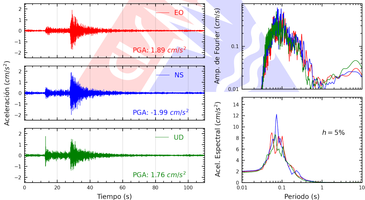
Figura A.4: Registros tiempo-historia, espectros de Fourier y de respuesta en las direcciones EO, NS y vertical de la estación SJLSC. Sismo de Canta, Canta - Lima del 2026-08-31, 05:36:50 (Hora local)
