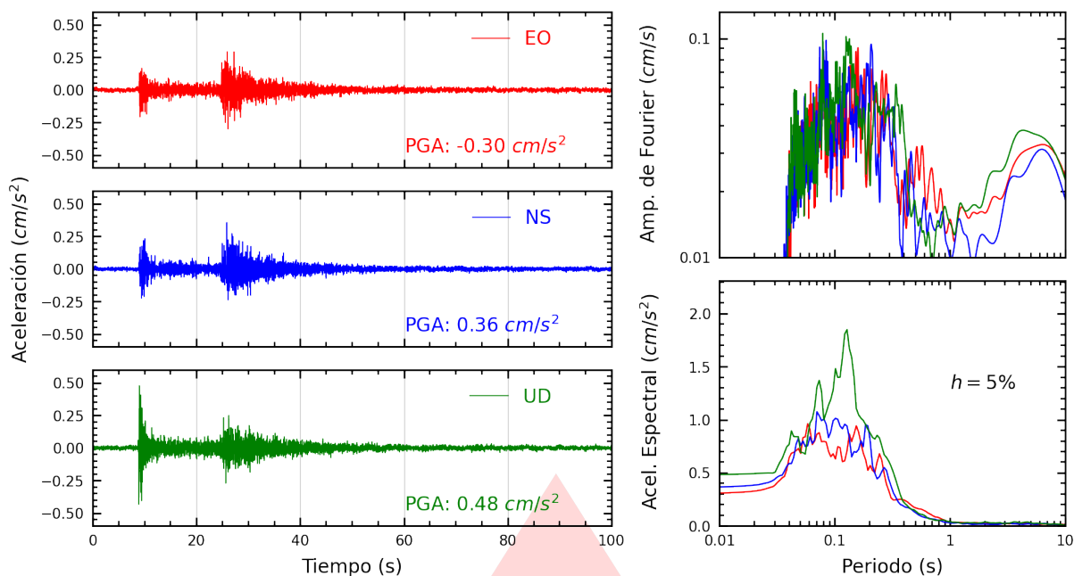
Figura A.27: Registros tiempo-historia, espectros de Fourier y de respuesta en las direcciones EO, NS y vertical de la estación UNMSM. Sismo de Canta, Canta - Lima del 2026-08-31, 05:36:50 (Hora local)
