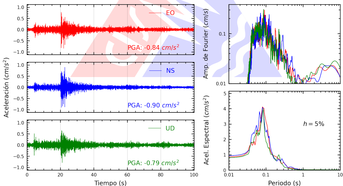
Figura A.14: Registros tiempo-historia, espectros de Fourier y de respuesta en las direcciones EO, NS y vertical de la estación URPPE. Sismo de Canta, Canta - Lima del 2026-08-31, 05:36:50 (Hora local)
