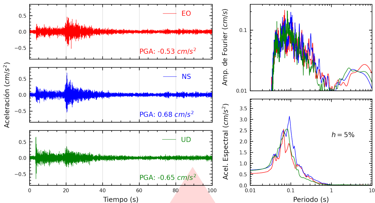
Figura A.23: Registros tiempo-historia, espectros de Fourier y de respuesta en las direcciones EO, NS y vertical de la estación MADRE. Sismo de Canta, Canta - Lima del 2026-08-31, 05:36:50 (Hora local)
