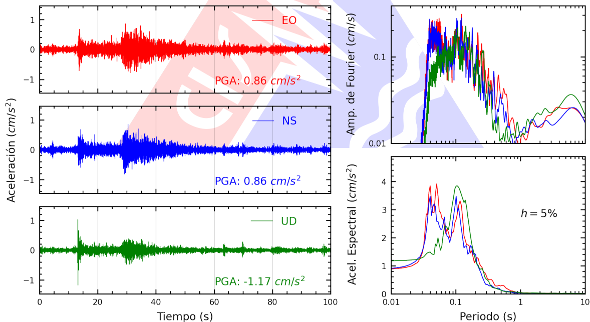
Figura A.10: Registros tiempo-historia, espectros de Fourier y de respuesta en las direcciones EO, NS y vertical de la estación OLIVO. Sismo de Canta, Canta - Lima del 2026-08-31, 05:36:50 (Hora local)
