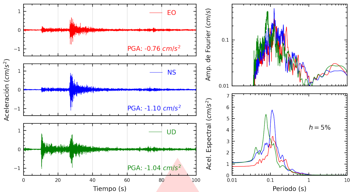
Figura A.11: Registros tiempo-historia, espectros de Fourier y de respuesta en las direcciones EO, NS y vertical de la estación SOCHO. Sismo de Canta, Canta - Lima del 2026-08-31, 05:36:50 (Hora local)
