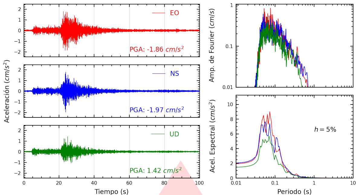
Figura A.5: Registros tiempo-historia, espectros de Fourier y de respuesta en las direcciones EO, NS y vertical de la estación UNTEL. Sismo de Canta, Canta - Lima del 2026-08-31, 05:36:50 (Hora local)
