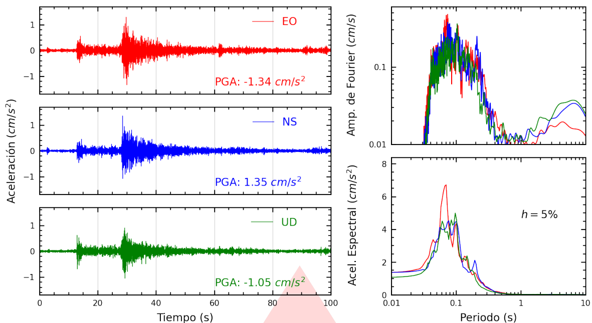
Figura A.7: Registros tiempo-historia, espectros de Fourier y de respuesta en las direcciones EO, NS y vertical de la estación INDEP. Sismo de Canta, Canta - Lima del 2026-08-31, 05:36:50 (Hora local)
