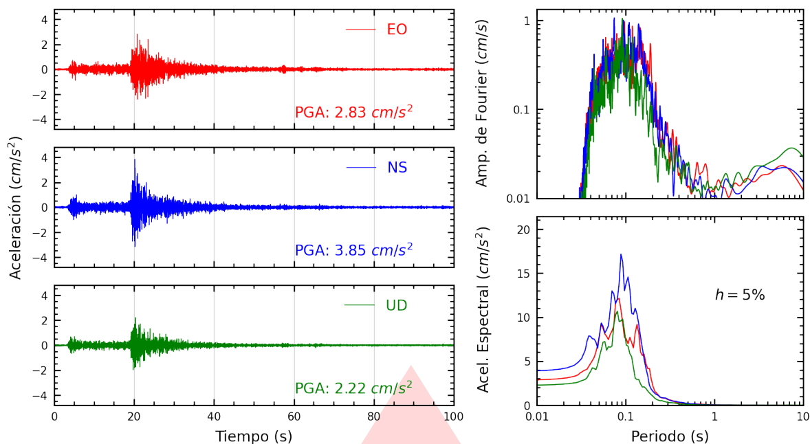
Figura A.1: Registros tiempo-historia, espectros de Fourier y de respuesta en las direcciones EO, NS y vertical de la estación USILM. Sismo de Canta, Canta - Lima del 2026-08-31, 05:36:50 (Hora local)
