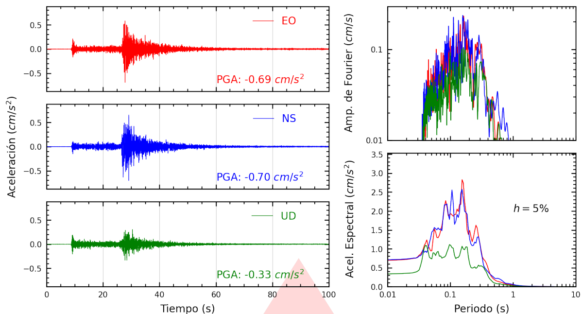
Figura A.1: Registros tiempo-historia, espectros de Fourier y de respuesta en las direcciones EO, NS y vertical de la estación UNSA2. Sismo de Chuquibamba, Condesuyos - Arequipa del 2026-08-31, 09:07:43 (Hora local)
