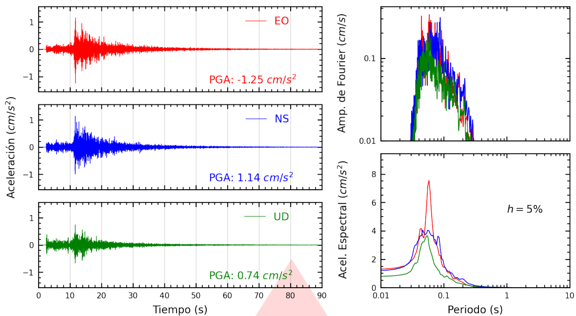
Figura A.1: Registros tiempo-historia, espectros de Fourier y de respuesta en las direcciones EO, NS y vertical de la estación UNSA2. Sismo de Quilca, Camaná - Arequipa del 2026-08-31, 09:55:10 (Hora local)
