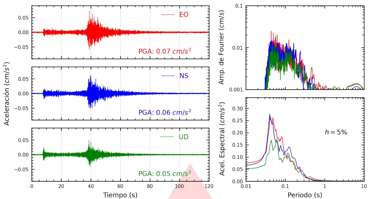
Figura A.1: Registros tiempo-historia, espectros de Fourier y de respuesta en las direcciones EO, NS y vertical de la estación UNSA2. Sismo de Ilave, El Collao - Puno del 2026-08-17, 19:51:46 (Hora local)
