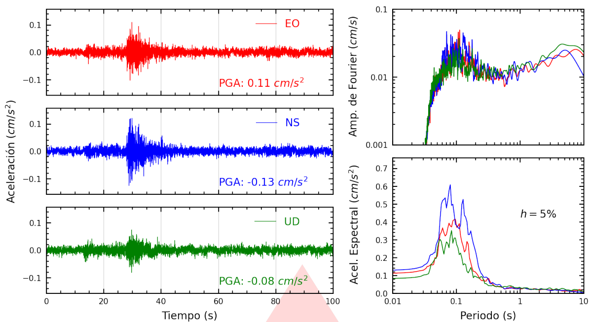
Figura A.1: Registros tiempo-historia, espectros de Fourier y de respuesta en las direcciones EO, NS y vertical de la estación UNTRM. Sismo de Jaén, Jaén - Cajamarca del 2026-09-01, 19:39:11 (Hora local)
