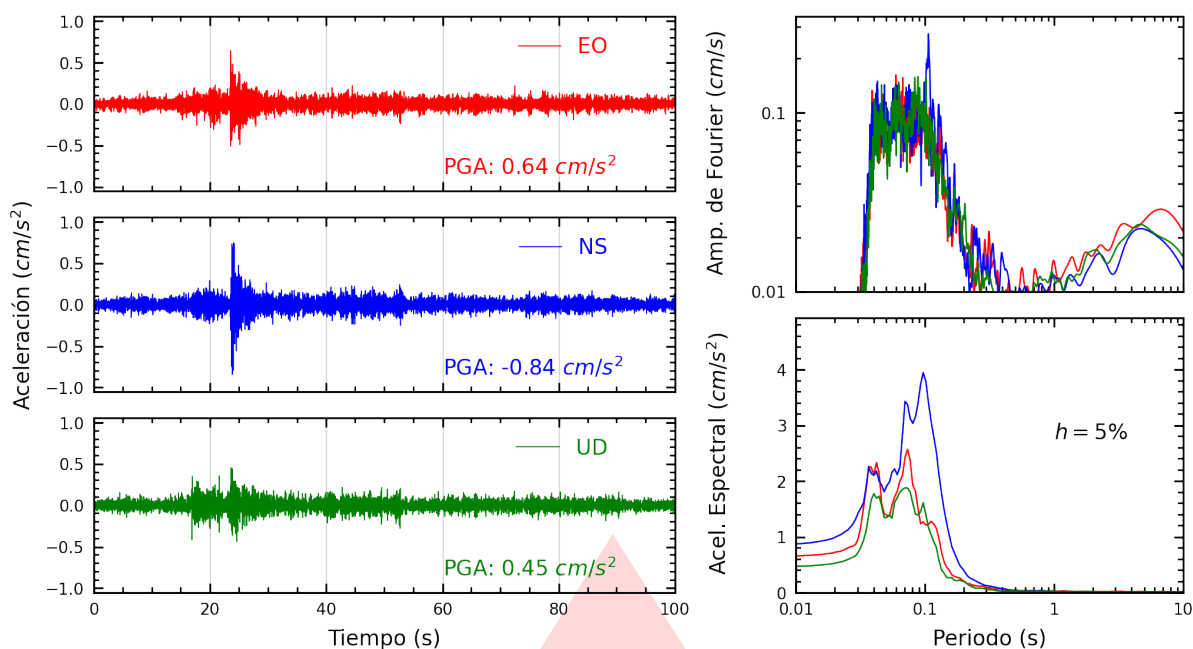
Figura A.15: Registros tiempo-historia, espectros de Fourier y de respuesta en las direcciones EO, NS y vertical de la estación MADRE. Sismo de Callao, Provincia Constitucional del Callao del 2026-09-03, 06:32:46 (Hora local)
