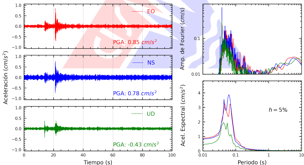
Figura A.14: Registros tiempo-historia, espectros de Fourier y de respuesta en las direcciones EO, NS y vertical de la estación UPCVI. Sismo de Callao, Provincia Constitucional del Callao del 2026-09-03, 06:32:46 (Hora local)
