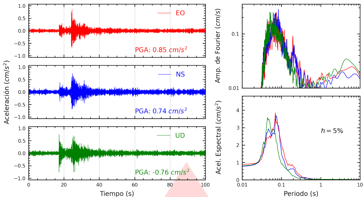
Figura A.13: Registros tiempo-historia, espectros de Fourier y de respuesta en las direcciones EO, NS y vertical de la estación SJLSC. Sismo de Callao, Provincia Constitucional del Callao del 2026-09-03, 06:32:46 (Hora local)
