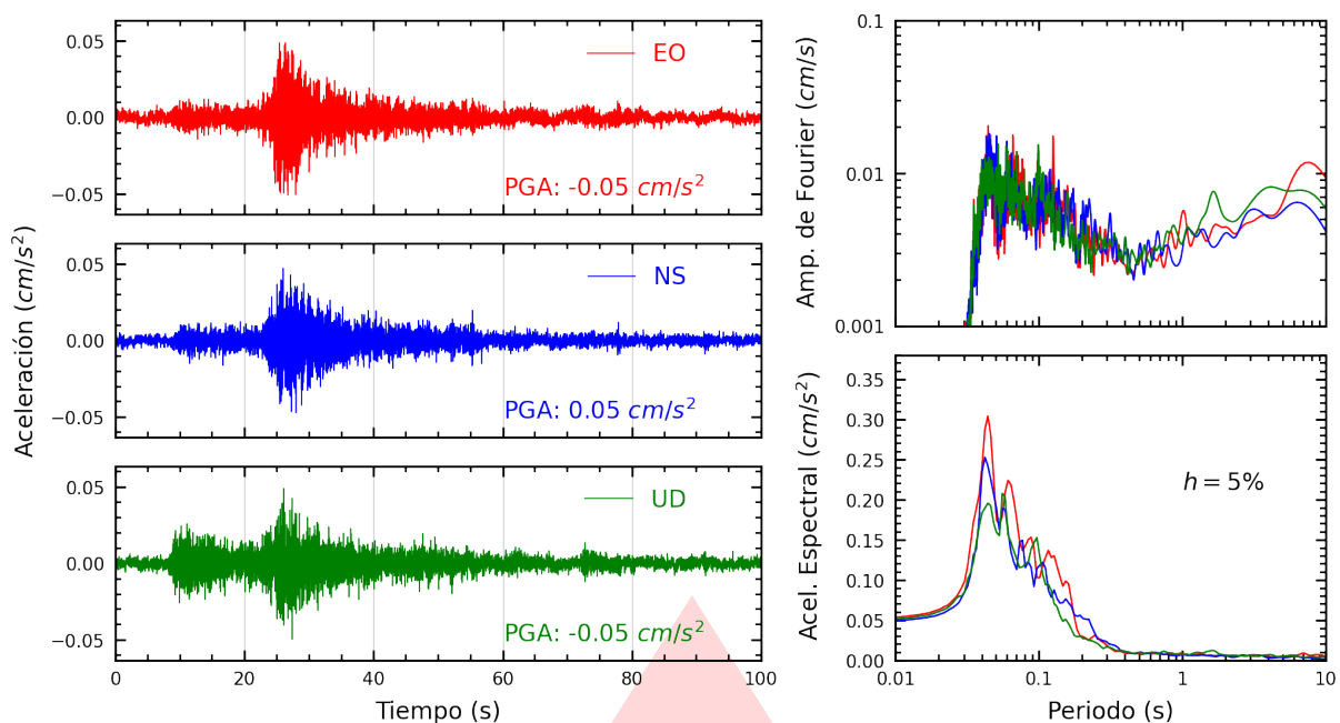
Figura A.31: Registros tiempo-historia, espectros de Fourier y de respuesta en las direcciones EO, NS y vertical de la estación CARAL. Sismo de Callao, Provincia Constitucional del Callao del 2026-09-03, 06:32:46 (Hora local)
