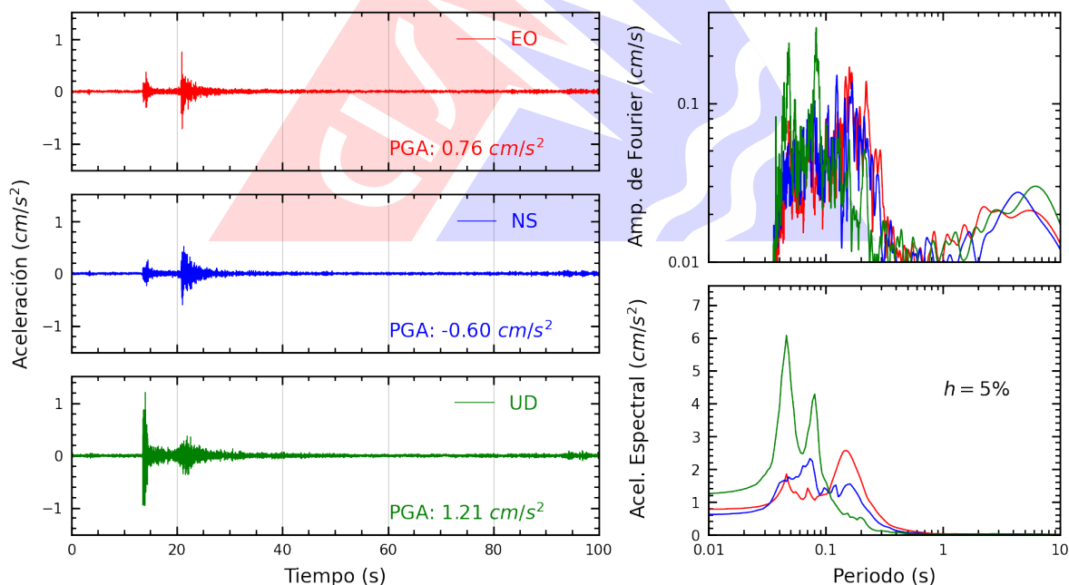
Figura A.10: Registros tiempo-historia, espectros de Fourier y de respuesta en las direcciones EO, NS y vertical de la estación SOCHO. Sismo de Callao, Provincia Constitucional del Callao del 2026-09-03, 06:32:46 (Hora local)
