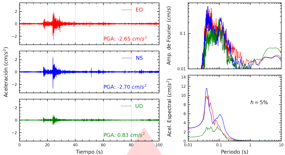
Figura A.3: Registros tiempo-historia, espectros de Fourier y de respuesta en las direcciones EO, NS y vertical de la estación OLIVO. Sismo de Callao, Provincia Constitucional del Callao del 2026-09-03, 06:32:46 (Hora local)
