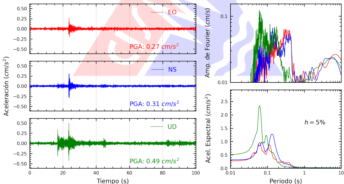
Figura A.20: Registros tiempo-historia, espectros de Fourier y de respuesta en las direcciones EO, NS y vertical de la estación ACAPU. Sismo de Callao, Provincia Constitucional del Callao del 2026-09-03, 06:32:46 (Hora local)
