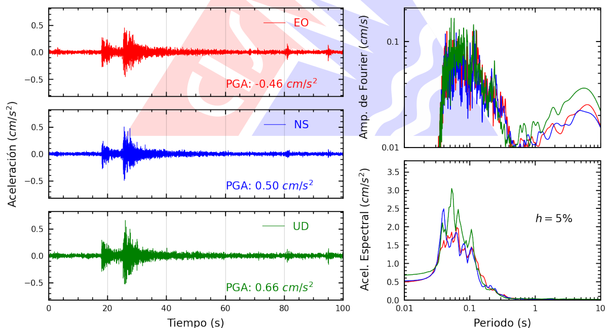
Figura A.18: Registros tiempo-historia, espectros de Fourier y de respuesta en las direcciones EO, NS y vertical de la estación SOVES. Sismo de Callao, Provincia Constitucional del Callao del 2026-09-03, 06:32:46 (Hora local)
