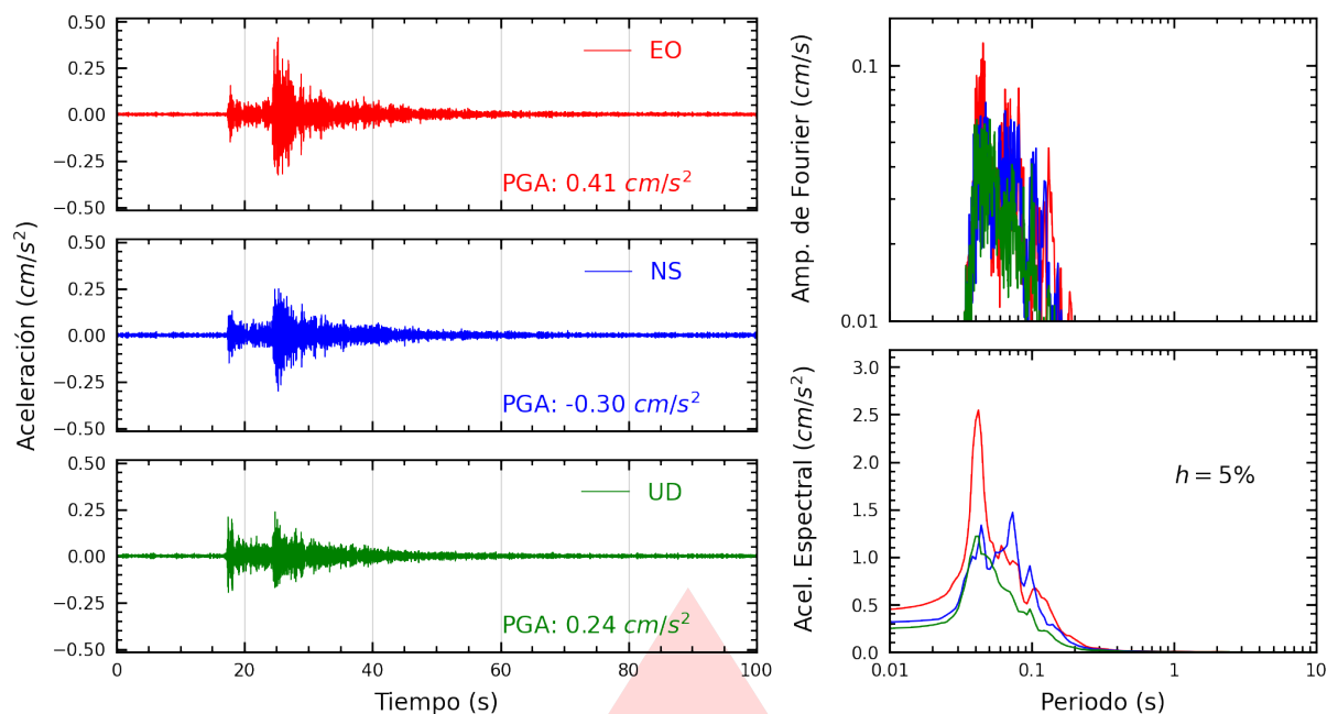
Figura A.23: Registros tiempo-historia, espectros de Fourier y de respuesta en las direcciones EO, NS y vertical de la estación ATARJ. Sismo de Callao, Provincia Constitucional del Callao del 2026-09-03, 06:32:46 (Hora local)
