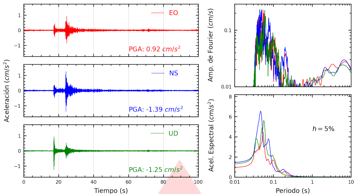
Figura A.7: Registros tiempo-historia, espectros de Fourier y de respuesta en las direcciones EO, NS y vertical de la estación COMAS. Sismo de Callao, Provincia Constitucional del Callao del 2026-09-03, 06:32:46 (Hora local)
