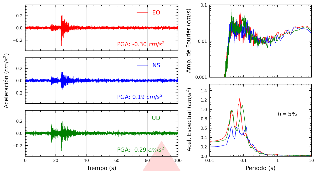
Figura A.27: Registros tiempo-historia, espectros de Fourier y de respuesta en las direcciones EO, NS y vertical de la estación BONDY. Sismo de Callao, Provincia Constitucional del Callao del 2026-09-03, 06:32:46 (Hora local)
