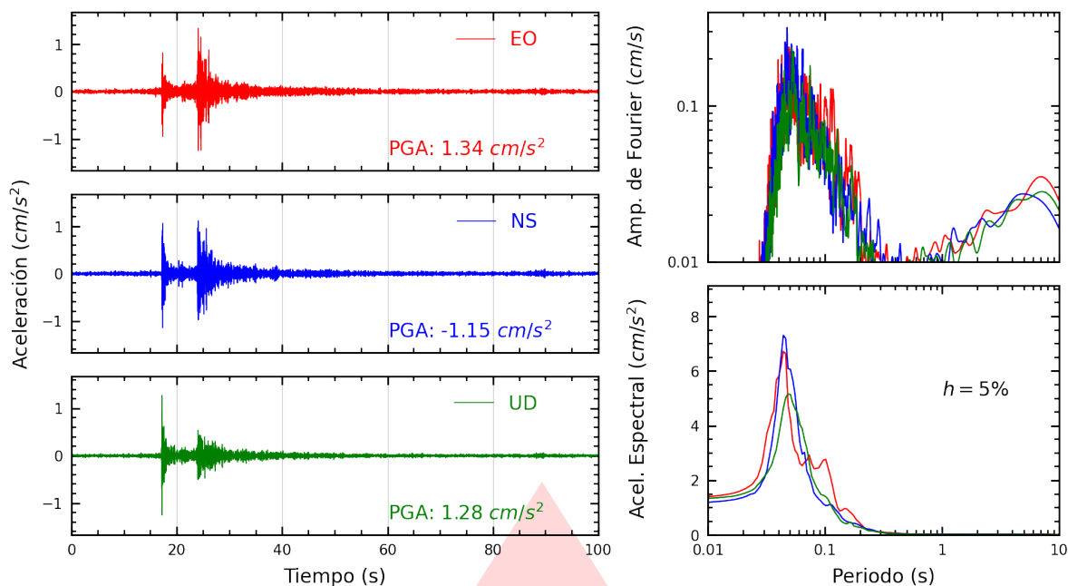
Figura A.9: Registros tiempo-historia, espectros de Fourier y de respuesta en las direcciones EO, NS y vertical de la estación FICPE. Sismo de Callao, Provincia Constitucional del Callao del 2026-09-03, 06:32:46 (Hora local)
