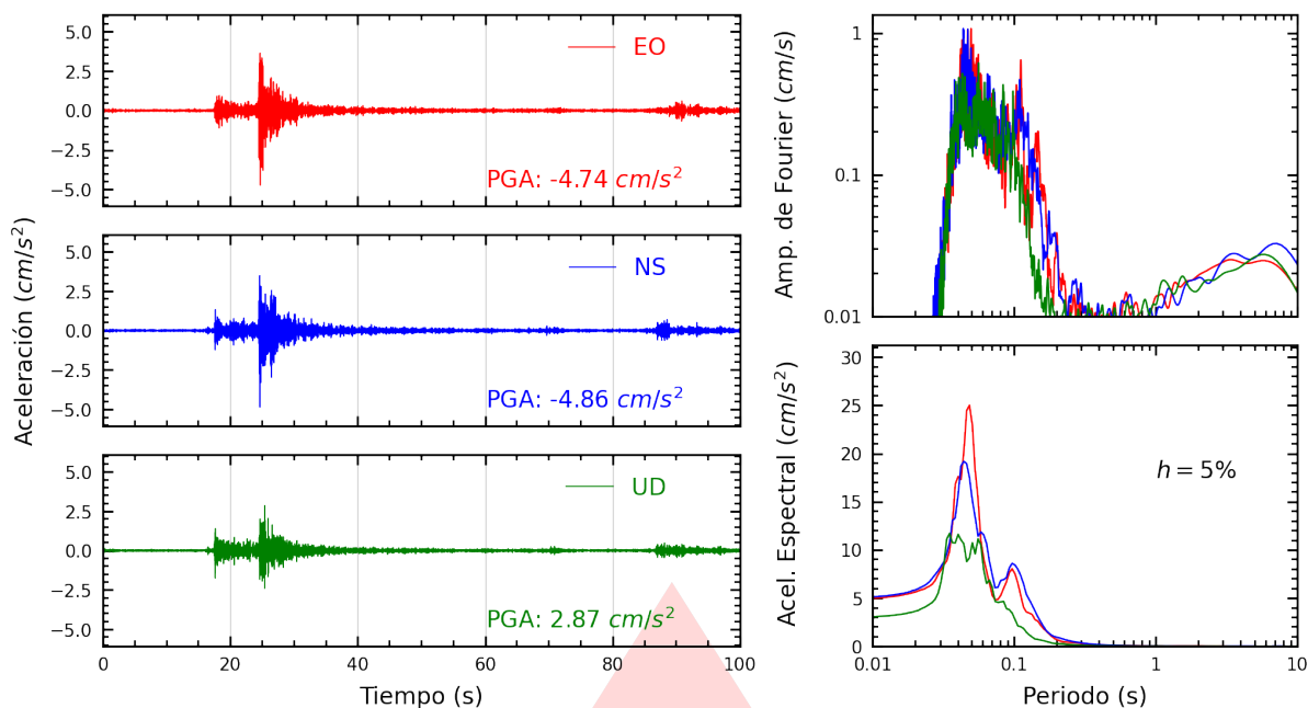
Figura A.1: Registros tiempo-historia, espectros de Fourier y de respuesta en las direcciones EO, NS y vertical de la estación SROSA. Sismo de Callao, Provincia Constitucional del Callao del 2026-09-03, 06:32:46 (Hora local)
