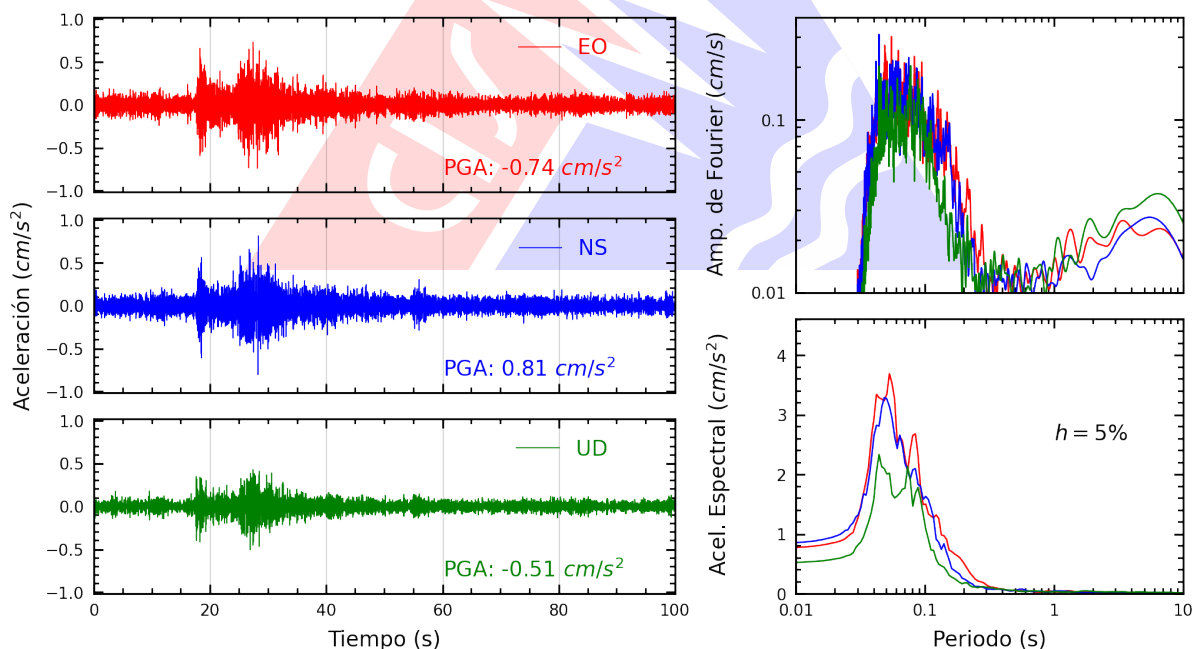
Figura A.16: Registros tiempo-historia, espectros de Fourier y de respuesta en las direcciones EO, NS y vertical de la estación USILM. Sismo de Callao, Provincia Constitucional del Callao del 2026-09-03, 06:32:46 (Hora local)
