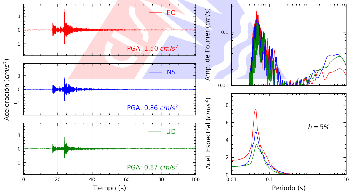
Figura A.6: Registros tiempo-historia, espectros de Fourier y de respuesta en las direcciones EO, NS y vertical de la estación UCSS. Sismo de Callao, Provincia Constitucional del Callao del 2026-09-03, 06:32:46 (Hora local)
