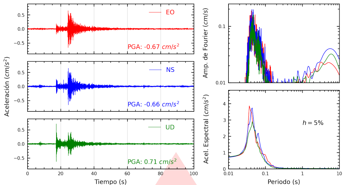
Figura A.17: Registros tiempo-historia, espectros de Fourier y de respuesta en las direcciones EO, NS y vertical de la estación SJLCE. Sismo de Callao, Provincia Constitucional del Callao del 2026-09-03, 06:32:46 (Hora local)
