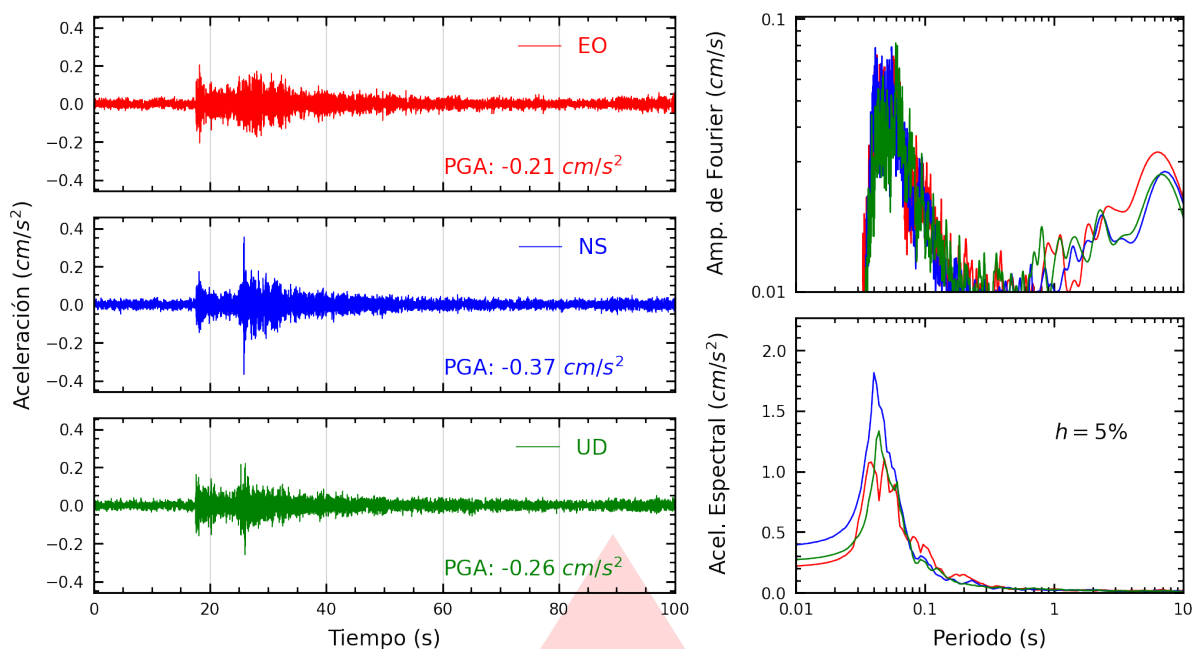
Figura A.25: Registros tiempo-historia, espectros de Fourier y de respuesta en las direcciones EO, NS y vertical de la estación IMCA. Sismo de Callao, Provincia Constitucional del Callao del 2026-09-03, 06:32:46 (Hora local)
