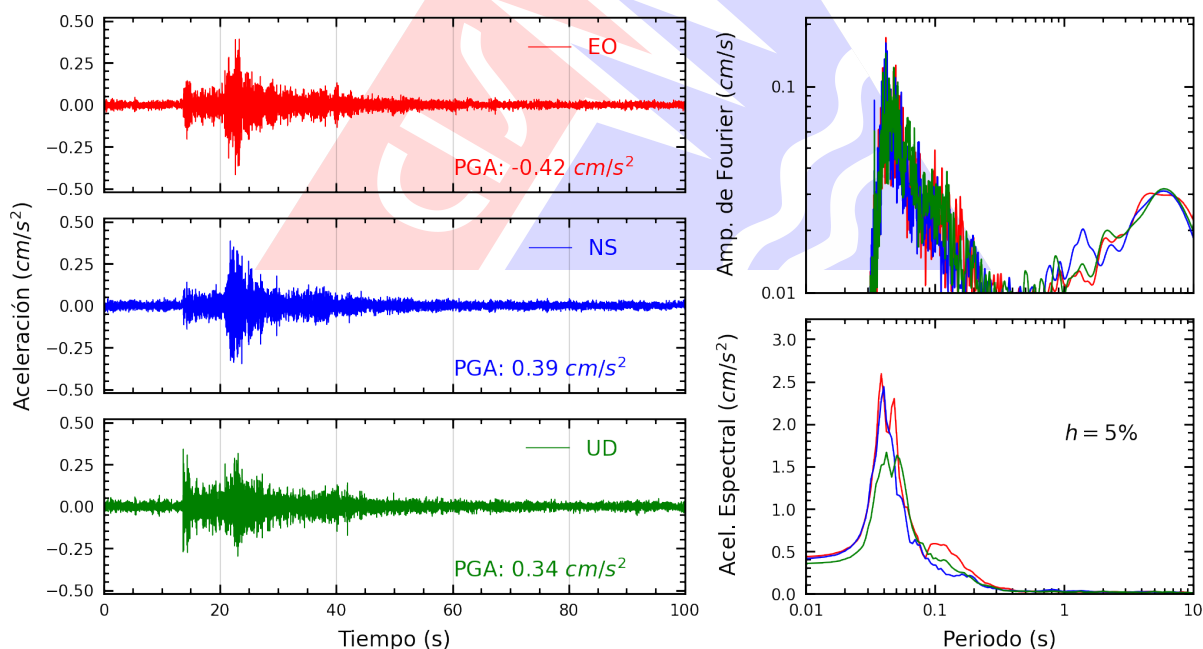
Figura A.22: Registros tiempo-historia, espectros de Fourier y de respuesta en las direcciones EO, NS y vertical de la estación USMP. Sismo de Callao, Provincia Constitucional del Callao del 2026-09-03, 06:32:46 (Hora local)
