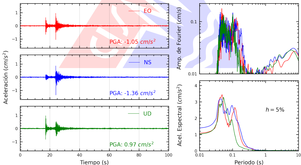
Figura A.8: Registros tiempo-historia, espectros de Fourier y de respuesta en las direcciones EO, NS y vertical de la estación JALVA. Sismo de Callao, Provincia Constitucional del Callao del 2026-09-03, 06:32:46 (Hora local)
