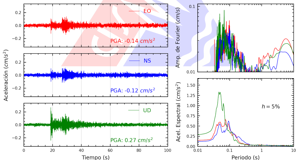
Figura A.28: Registros tiempo-historia, espectros de Fourier y de respuesta en las direcciones EO, NS y vertical de la estación USILP. Sismo de Callao, Provincia Constitucional del Callao del 2026-09-03, 06:32:46 (Hora local)
