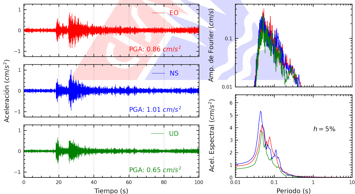
Figura A.12: Registros tiempo-historia, espectros de Fourier y de respuesta en las direcciones EO, NS y vertical de la estación UNTEL. Sismo de Callao, Provincia Constitucional del Callao del 2026-09-03, 06:32:46 (Hora local)
