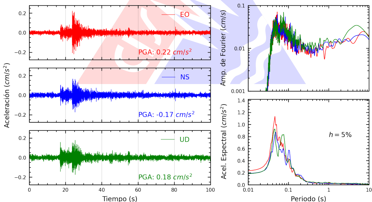
Figura A.30: Registros tiempo-historia, espectros de Fourier y de respuesta en las direcciones EO, NS y vertical de la estación UNFV. Sismo de Callao, Provincia Constitucional del Callao del 2026-09-03, 06:32:46 (Hora local)
