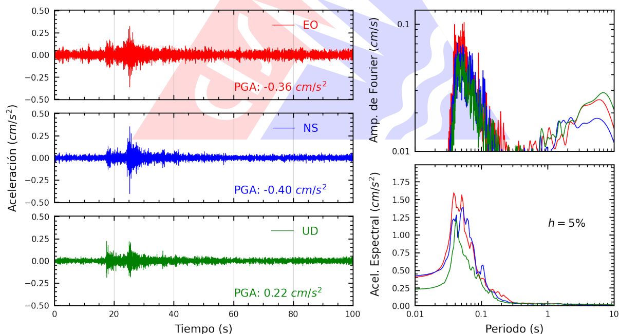
Figura A.24: Registros tiempo-historia, espectros de Fourier y de respuesta en las direcciones EO, NS y vertical de la estación INICT. Sismo de Callao, Provincia Constitucional del Callao del 2026-09-03, 06:32:46 (Hora local)
