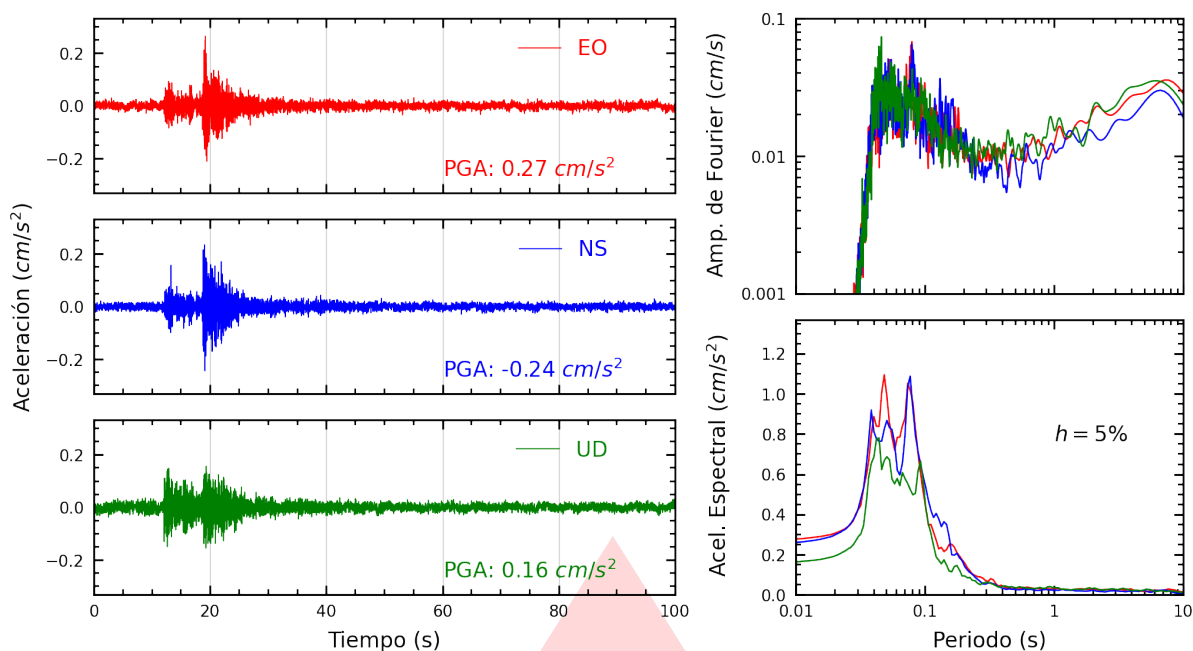
Figura A.29: Registros tiempo-historia, espectros de Fourier y de respuesta en las direcciones EO, NS y vertical de la estación UNMSM. Sismo de Callao, Provincia Constitucional del Callao del 2026-09-03, 06:32:46 (Hora local)
