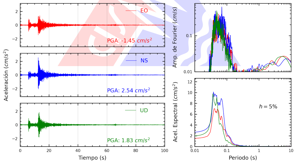
Figura A.4: Registros tiempo-historia, espectros de Fourier y de respuesta en las direcciones EO, NS y vertical de la estación JOSEO. Sismo de Callao, Provincia Constitucional del Callao del 2026-09-03, 06:32:46 (Hora local)
