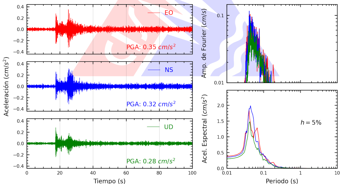
Figura A.26: Registros tiempo-historia, espectros de Fourier y de respuesta en las direcciones EO, NS y vertical de la estación BORJA. Sismo de Callao, Provincia Constitucional del Callao del 2026-09-03, 06:32:46 (Hora local)
