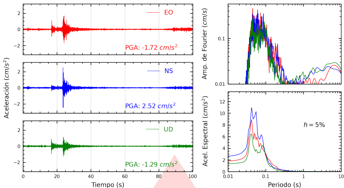
Figura A.5: Registros tiempo-historia, espectros de Fourier y de respuesta en las direcciones EO, NS y vertical de la estación INDEP. Sismo de Callao, Provincia Constitucional del Callao del 2026-09-03, 06:32:46 (Hora local)
