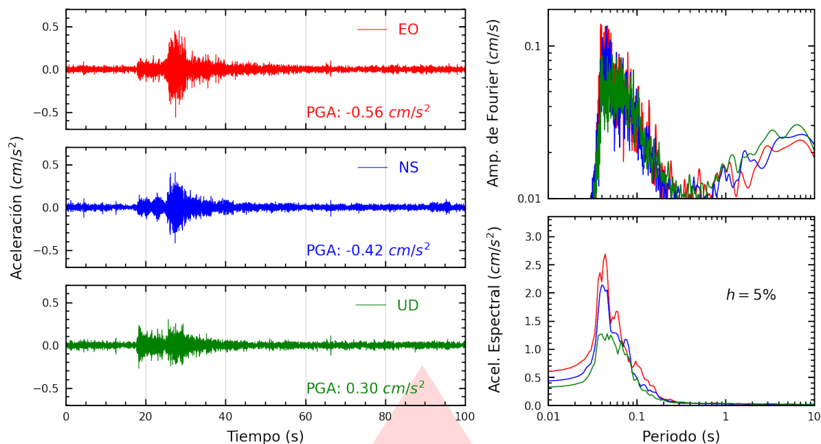
Figura A.19: Registros tiempo-historia, espectros de Fourier y de respuesta en las direcciones EO, NS y vertical de la estación UCVAT. Sismo de Callao, Provincia Constitucional del Callao del 2026-09-03, 06:32:46 (Hora local)
