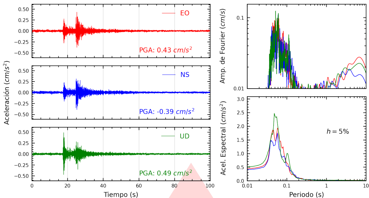
Figura A.21: Registros tiempo-historia, espectros de Fourier y de respuesta en las direcciones EO, NS y vertical de la estación SERVI. Sismo de Callao, Provincia Constitucional del Callao del 2026-09-03, 06:32:46 (Hora local)
