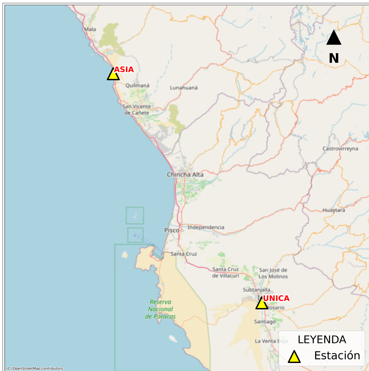
Figura 2: Mapa de ubicación de la(s) estación(es) acelerográfica(s) correspondiente(s) al Sismo de Ica, Ica - Ica del 03 de setiembre de 2026 a las 08:54:19 (hora local)
