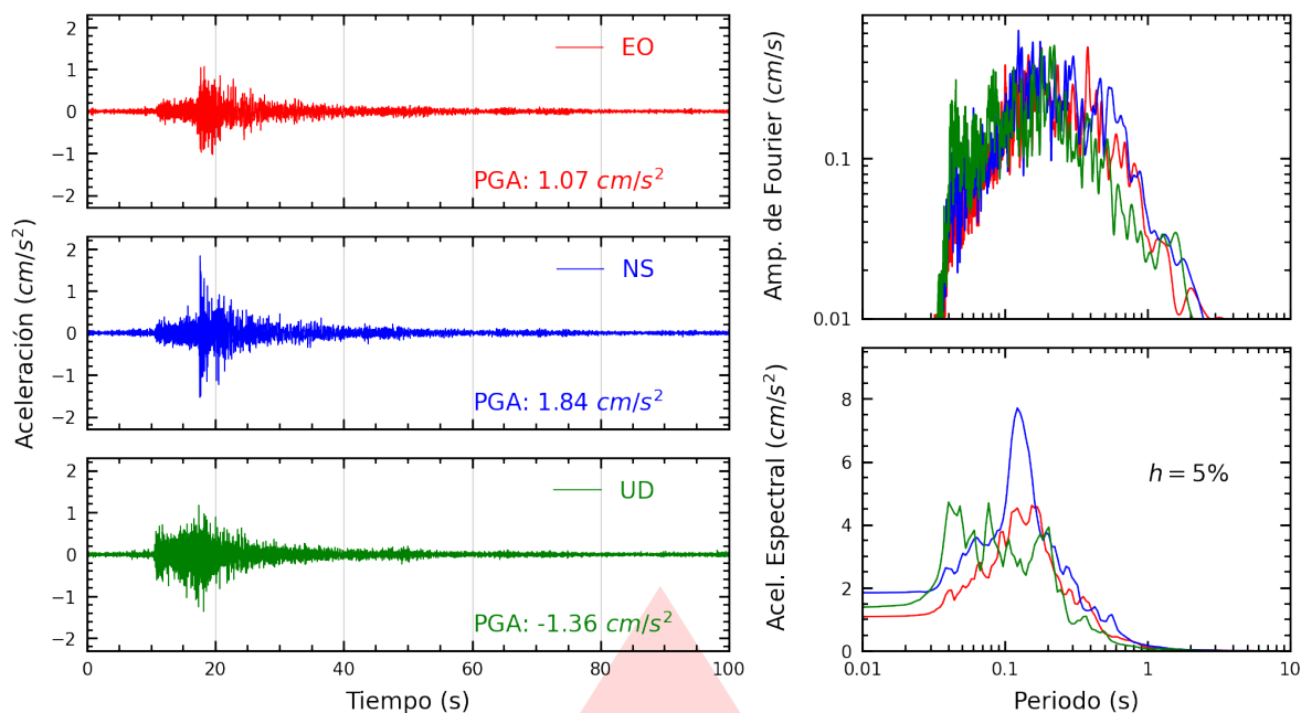
Figura A.1: Registros tiempo-historia, espectros de Fourier y de respuesta en las direcciones EO, NS y vertical de la estación UNICA. Sismo de Ica, Ica - Ica del 2026-09-03, 08:54:19 (Hora local)
