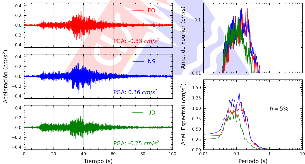
Figura A.2: Registros tiempo-historia, espectros de Fourier y de respuesta en las direcciones EO, NS y vertical de la estación ASIA. Sismo de Ica, Ica - Ica del 2026-09-03, 08:54:19 (Hora local)
