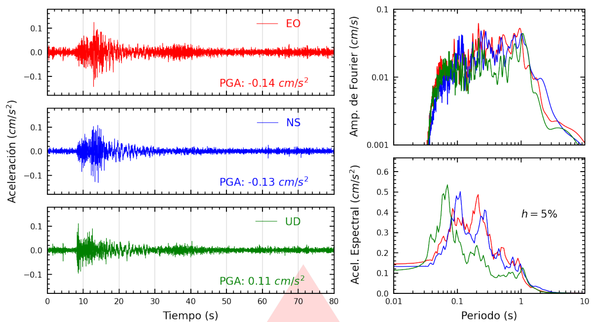
Figura A.1: Registros tiempo-historia, espectros de Fourier y de respuesta en las direcciones EO, NS y vertical de la estación UNC. Sismo de Contumazá, Contumazá - Cajamarca del 2026-09-03, 12:14:11 (Hora local)
