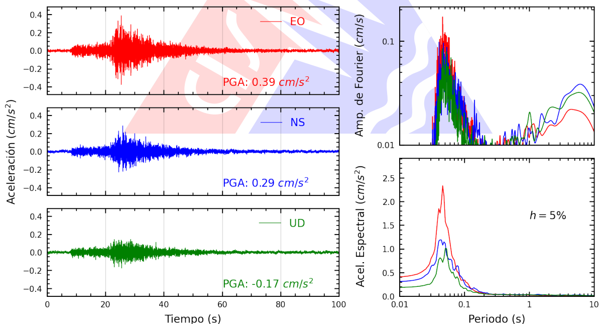
Figura A.12: Registros tiempo-historia, espectros de Fourier y de respuesta en las direcciones EO, NS y vertical de la estación UCSS. Sismo de Cañete, Cañete - Lima del 2026-09-04, 05:18:37 (Hora local)
