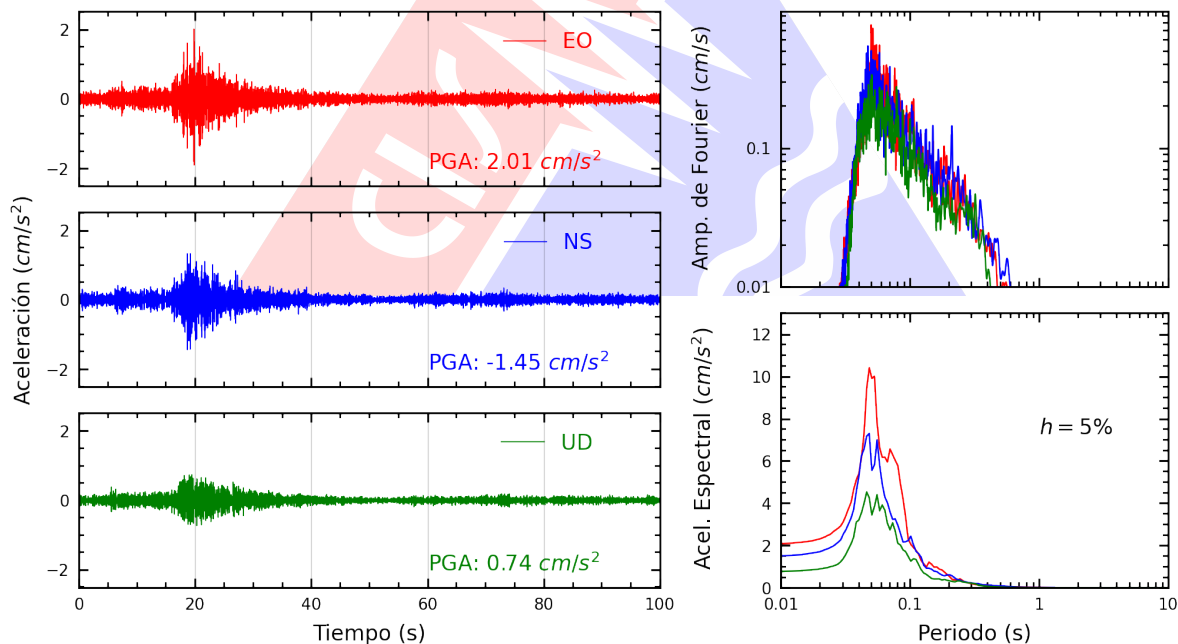
Figura A.2: Registros tiempo-historia, espectros de Fourier y de respuesta en las direcciones EO, NS y vertical de la estación UNTEL. Sismo de Cañete, Cañete - Lima del 2026-09-04, 05:18:37 (Hora local)
