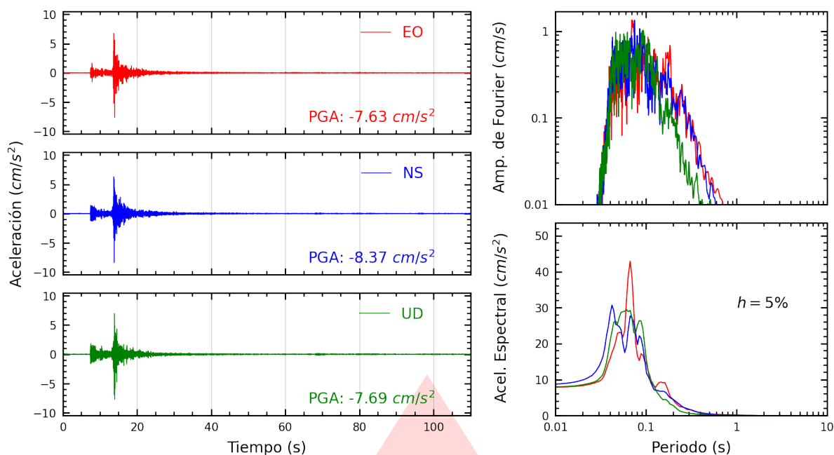
Figura A.1: Registros tiempo-historia, espectros de Fourier y de respuesta en las direcciones EO, NS y vertical de la estación ASIA. Sismo de Cañete, Cañete - Lima del 2026-09-04, 05:18:37 (Hora local)
