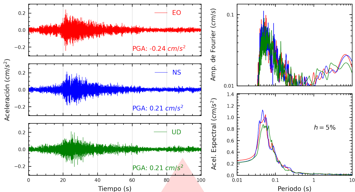
Figura A.19: Registros tiempo-historia, espectros de Fourier y de respuesta en las direcciones EO, NS y vertical de la estación IMCA. Sismo de Cañete, Cañete - Lima del 2026-09-04, 05:18:37 (Hora local)
