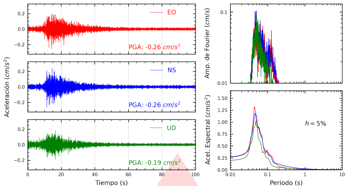
Figura A.17: Registros tiempo-historia, espectros de Fourier y de respuesta en las direcciones EO, NS y vertical de la estación ATARJ. Sismo de Cañete, Cañete - Lima del 2026-09-04, 05:18:37 (Hora local)
