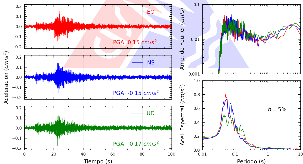
Figura A.22: Registros tiempo-historia, espectros de Fourier y de respuesta en las direcciones EO, NS y vertical de la estación UNFV. Sismo de Cañete, Cañete - Lima del 2026-09-04, 05:18:37 (Hora local)
