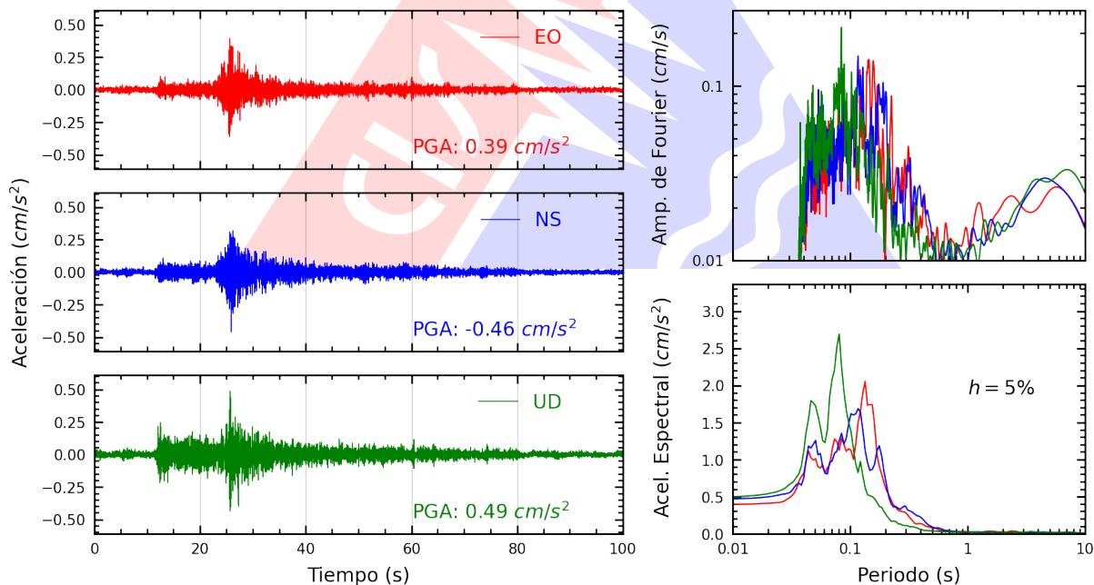
Figura A.10: Registros tiempo-historia, espectros de Fourier y de respuesta en las direcciones EO, NS y vertical de la estación SOCHO. Sismo de Cañete, Cañete - Lima del 2026-09-04, 05:18:37 (Hora local)
