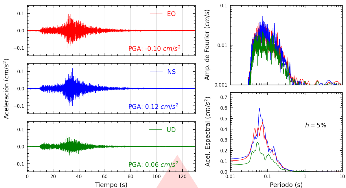
Figura A.1: Registros tiempo-historia, espectros de Fourier y de respuesta en las direcciones EO, NS y vertical de la estación UNSA2. Sismo de Atico, Caravelí - Arequipa del 2026-09-04, 08:08:53 (Hora local)
