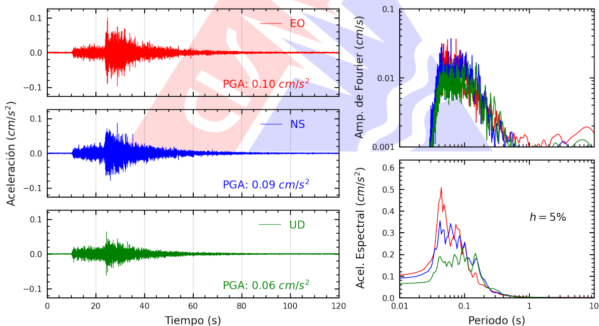
Figura A.2: Registros tiempo-historia, espectros de Fourier y de respuesta en las direcciones EO, NS y vertical de la estación UNSA2. Sismo de Ilo, Ilo - Moquegua del 2026-09-04, 08:28:00 (Hora local)
