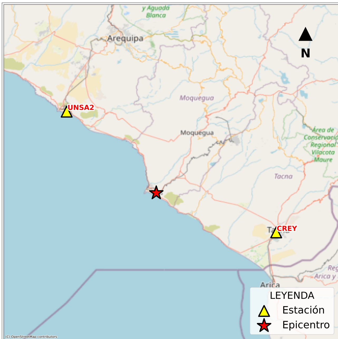
Figura 2: Mapa de ubicación de la(s) estación(es) acelerográfica(s) correspondiente(s) al Sismo de Ilo, Ilo - Moquegua del 04 de setiembre de 2026 a las 08:28:00 (hora local)
