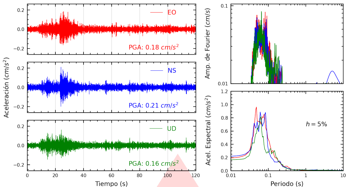
Figura A.1: Registros tiempo-historia, espectros de Fourier y de respuesta en las direcciones EO, NS y vertical de la estación CREY. Sismo de Ilo, Ilo - Moquegua del 2026-09-04, 08:28:00 (Hora local)
