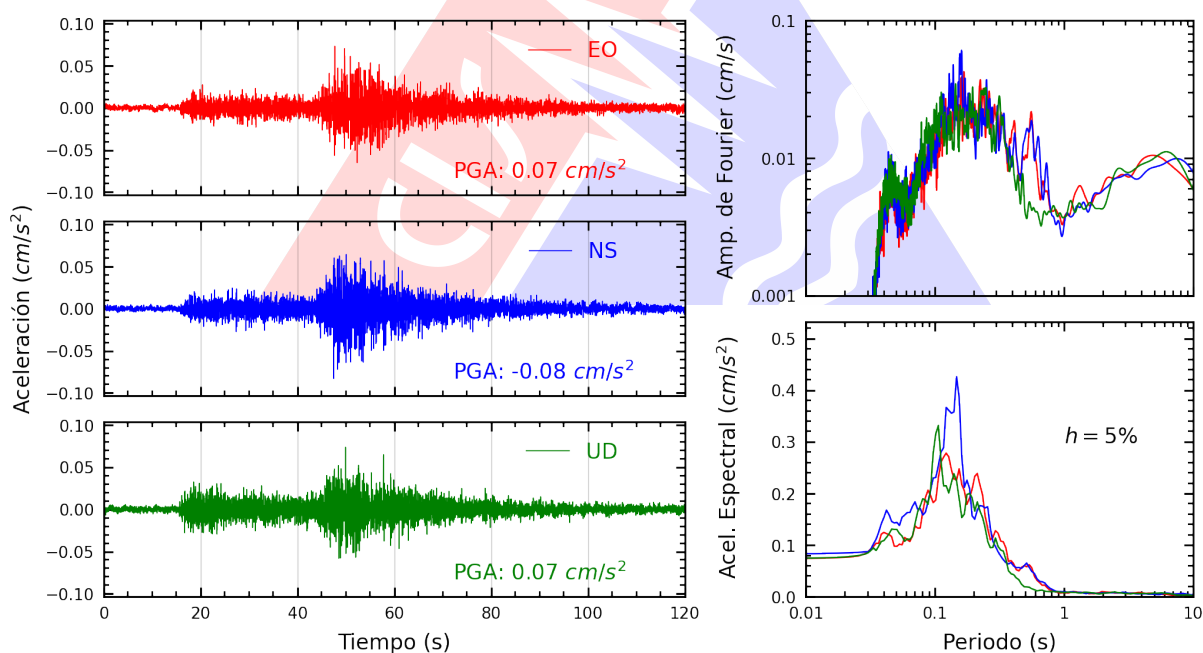
Figura A.2: Registros tiempo-historia, espectros de Fourier y de respuesta en las direcciones EO, NS y vertical de la estación CARAL. Sismo de Chimbote, Santa - Áncash del 2026-09-05, 12:09:14 (Hora local)
