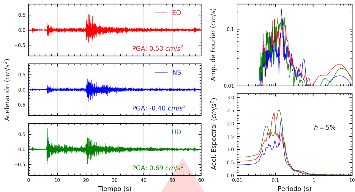
Figura A.1: Registros tiempo-historia, espectros de Fourier y de respuesta en las direcciones EO, NS y vertical de la estación UPAOT. Sismo de Chimbote, Santa - Áncash del 2026-09-05, 12:09:14 (Hora local)
