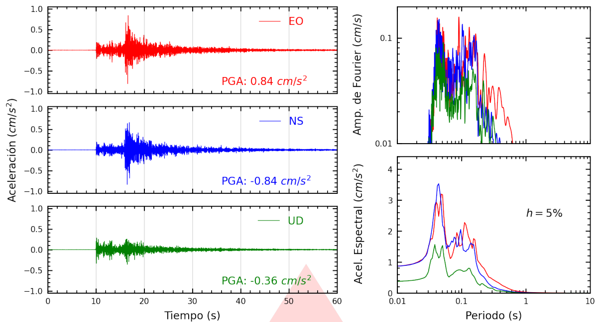
Figura A.1: Registros tiempo-historia, espectros de Fourier y de respuesta en las direcciones EO, NS y vertical de la estación UNSA2. Sismo de Mollendo, Islay - Arequipa del 2026-09-06, 19:54:50 (Hora local)
