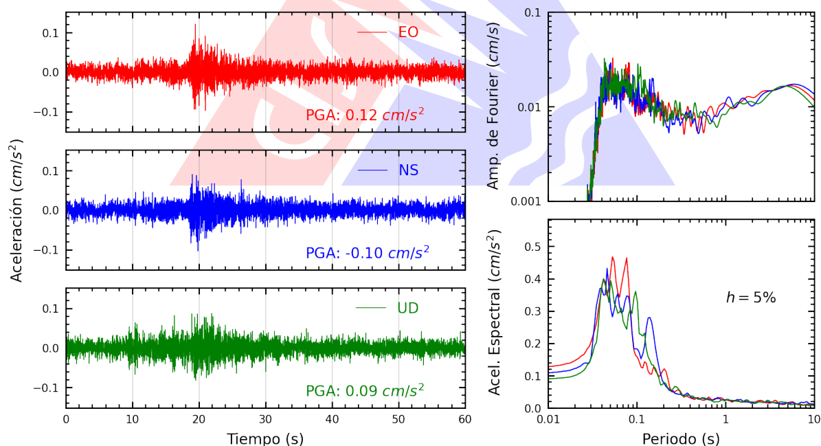
Figura A.22: Registros tiempo-historia, espectros de Fourier y de respuesta en las direcciones EO, NS y vertical de la estación BONDY. Sismo de Chilca, Cañete - Lima del 2026-09-07, 15:57:43 (Hora local)
