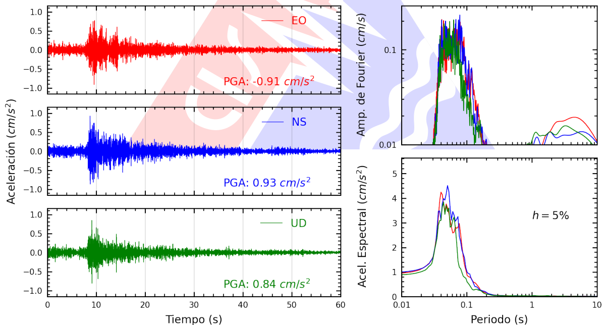
Figura A.6: Registros tiempo-historia, espectros de Fourier y de respuesta en las direcciones EO, NS y vertical de la estación JOSEO. Sismo de Chilca, Cañete - Lima del 2026-09-07, 15:57:43 (Hora local)
