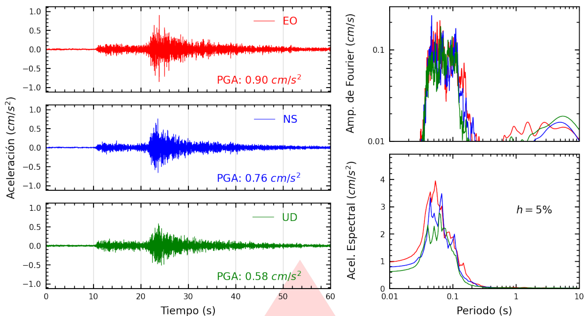
Figura A.7: Registros tiempo-historia, espectros de Fourier y de respuesta en las direcciones EO, NS y vertical de la estación AMORE. Sismo de Chilca, Cañete - Lima del 2026-09-07, 15:57:43 (Hora local)
