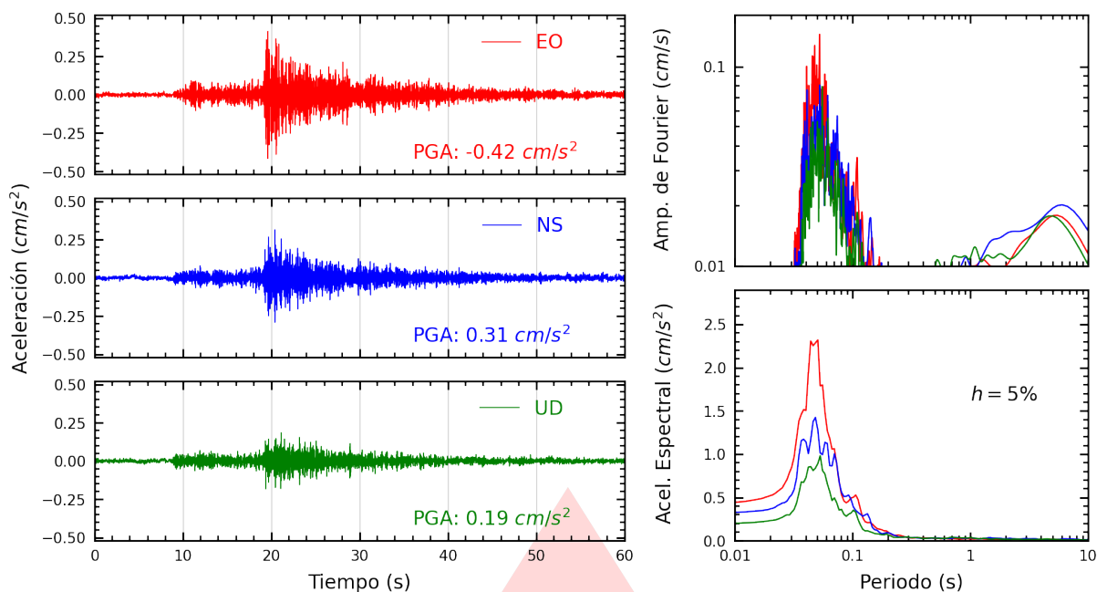
Figura A.15: Registros tiempo-historia, espectros de Fourier y de respuesta en las direcciones EO, NS y vertical de la estación UCSS. Sismo de Chilca, Cañete - Lima del 2026-09-07, 15:57:43 (Hora local)
