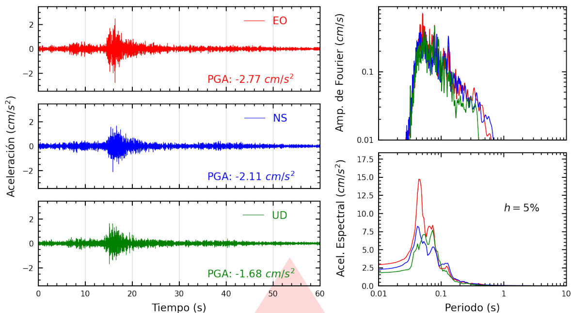
Figura A.1: Registros tiempo-historia, espectros de Fourier y de respuesta en las direcciones EO, NS y vertical de la estación UNTEL. Sismo de Chilca, Cañete - Lima del 2026-09-07, 15:57:43 (Hora local)
