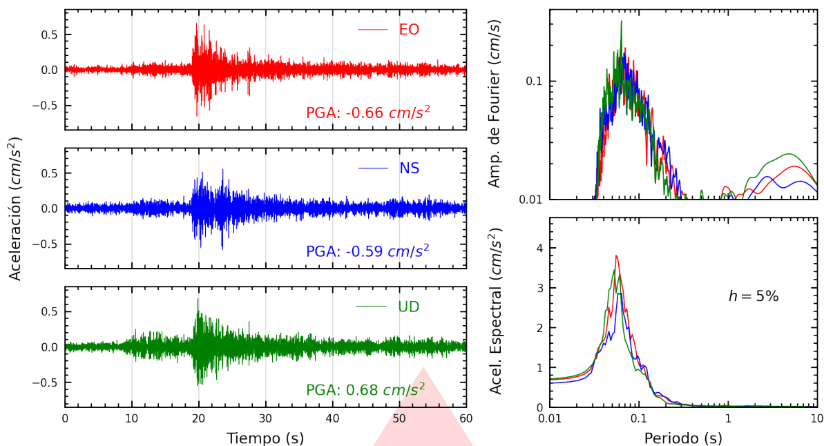
Figura A.11: Registros tiempo-historia, espectros de Fourier y de respuesta en las direcciones EO, NS y vertical de la estación SJLSC. Sismo de Chilca, Cañete - Lima del 2026-09-07, 15:57:43 (Hora local)
