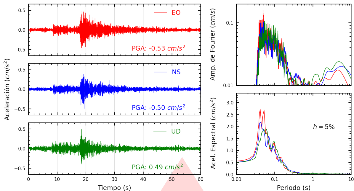
Figura A.13: Registros tiempo-historia, espectros de Fourier y de respuesta en las direcciones EO, NS y vertical de la estación UCVAT. Sismo de Chilca, Cañete - Lima del 2026-09-07, 15:57:43 (Hora local)
