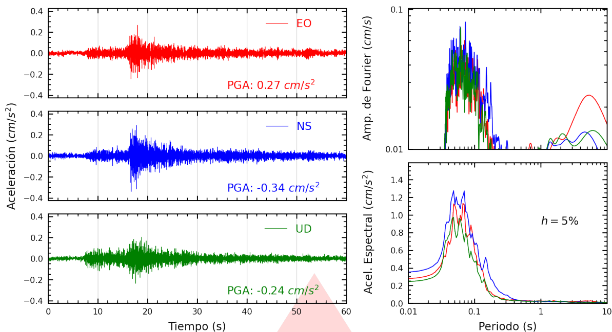
Figura A.17: Registros tiempo-historia, espectros de Fourier y de respuesta en las direcciones EO, NS y vertical de la estación SERVI. Sismo de Chilca, Cañete - Lima del 2026-09-07, 15:57:43 (Hora local)
