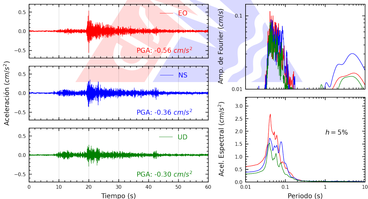
Figura A.12: Registros tiempo-historia, espectros de Fourier y de respuesta en las direcciones EO, NS y vertical de la estación SJLCE. Sismo de Chilca, Cañete - Lima del 2026-09-07, 15:57:43 (Hora local)
