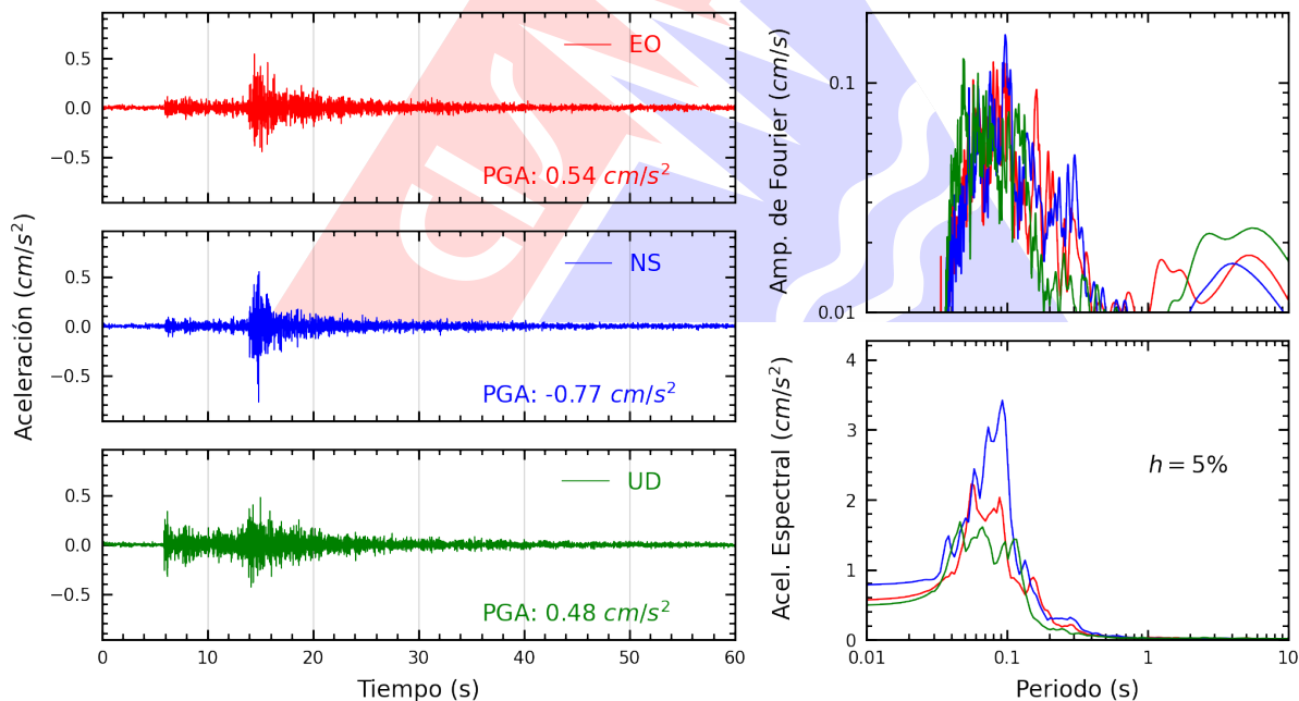
Figura A.8: Registros tiempo-historia, espectros de Fourier y de respuesta en las direcciones EO, NS y vertical de la estación USILP. Sismo de Chilca, Cañete - Lima del 2026-09-07, 15:57:43 (Hora local)
