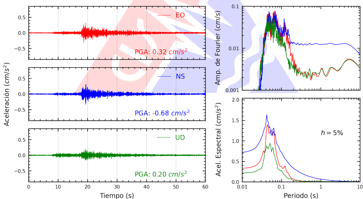
Figura A.10: Registros tiempo-historia, espectros de Fourier y de respuesta en las direcciones EO, NS y vertical de la estación ATARJ. Sismo de Chilca, Cañete - Lima del 2026-09-07, 15:57:43 (Hora local)
