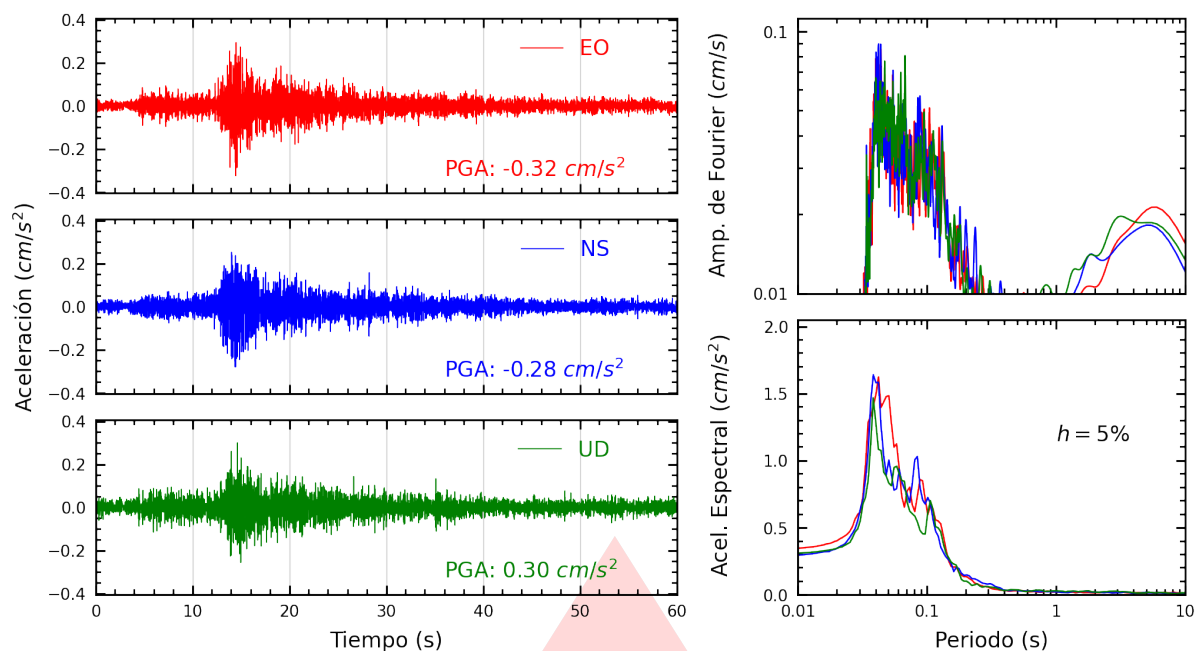
Figura A.19: Registros tiempo-historia, espectros de Fourier y de respuesta en las direcciones EO, NS y vertical de la estación USMP. Sismo de Chilca, Cañete - Lima del 2026-09-07, 15:57:43 (Hora local)
