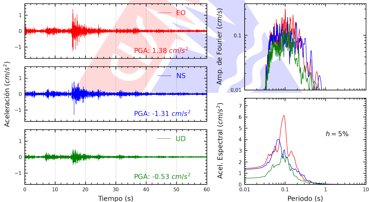
Figura A.4: Registros tiempo-historia, espectros de Fourier y de respuesta en las direcciones EO, NS y vertical de la estación BRISA. Sismo de Chilca, Cañete - Lima del 2026-09-07, 15:57:43 (Hora local)
