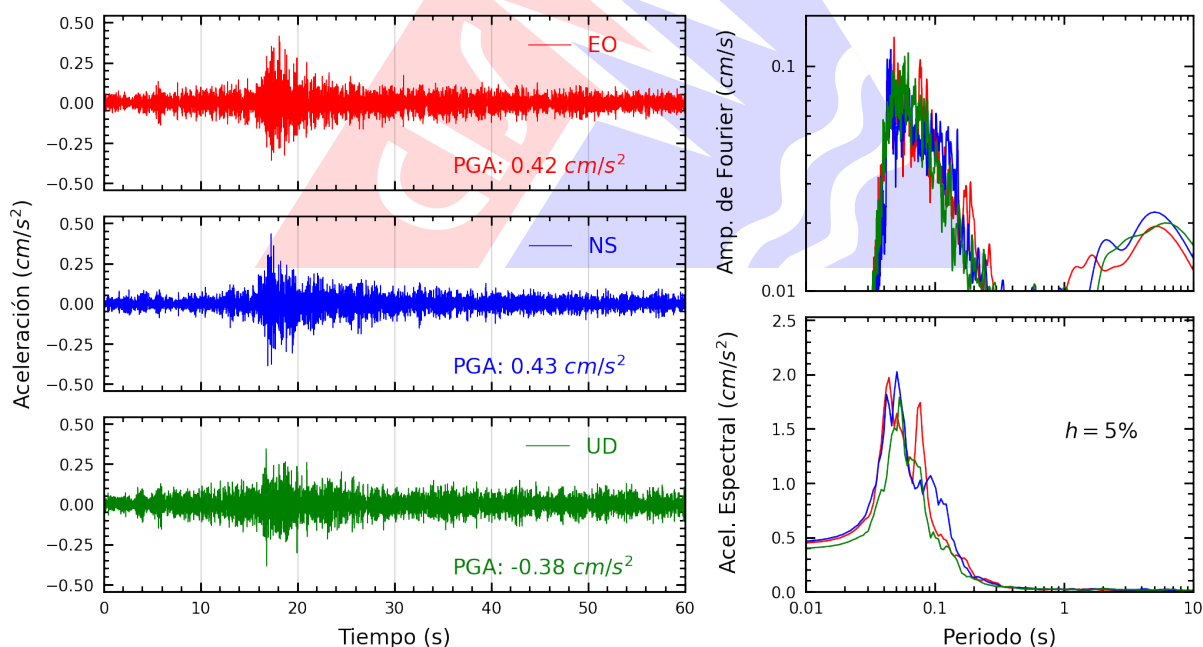
Figura A.14: Registros tiempo-historia, espectros de Fourier y de respuesta en las direcciones EO, NS y vertical de la estación URPPE. Sismo de Chilca, Cañete - Lima del 2026-09-07, 15:57:43 (Hora local)
