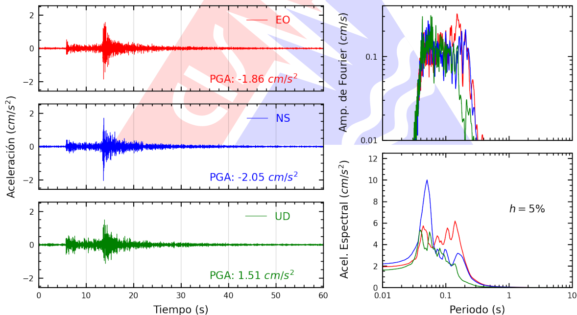
Figura A.2: Registros tiempo-historia, espectros de Fourier y de respuesta en las direcciones EO, NS y vertical de la estación ASIA. Sismo de Chilca, Cañete - Lima del 2026-09-07, 15:57:43 (Hora local)
