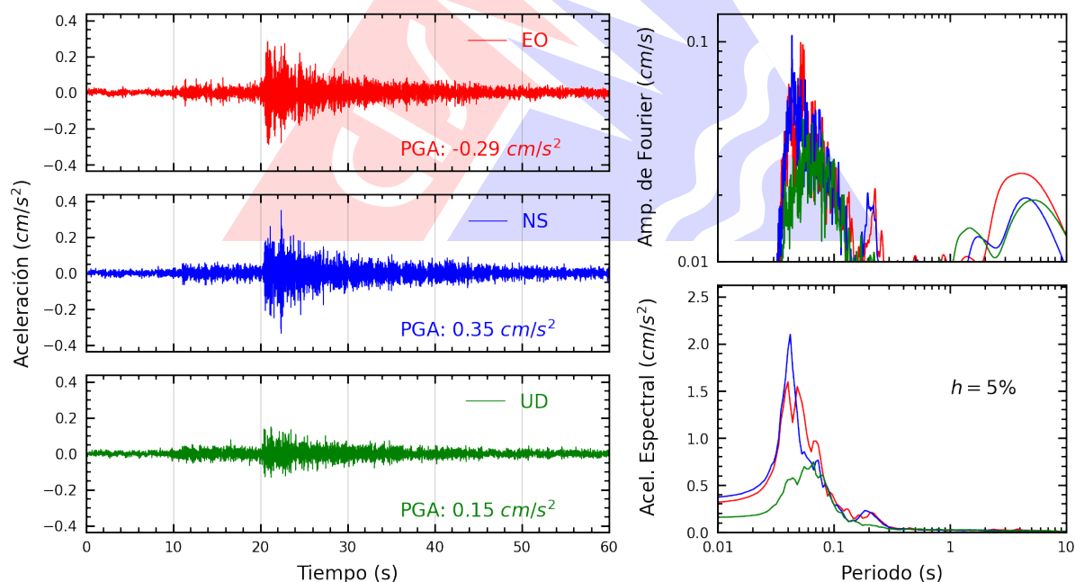
Figura A.16: Registros tiempo-historia, espectros de Fourier y de respuesta en las direcciones EO, NS y vertical de la estación COMAS. Sismo de Chilca, Cañete - Lima del 2026-09-07, 15:57:43 (Hora local)
