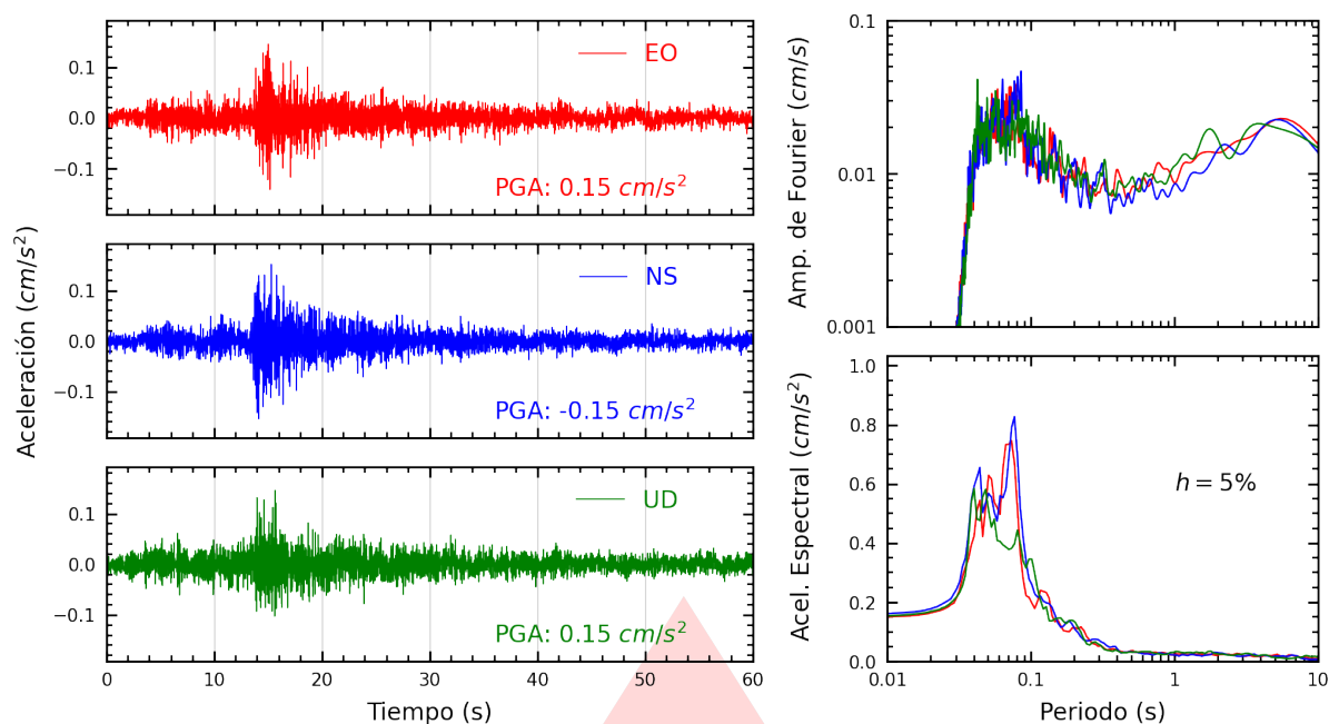
Figura A.21: Registros tiempo-historia, espectros de Fourier y de respuesta en las direcciones EO, NS y vertical de la estación UNMSM. Sismo de Chilca, Cañete - Lima del 2026-09-07, 15:57:43 (Hora local)
