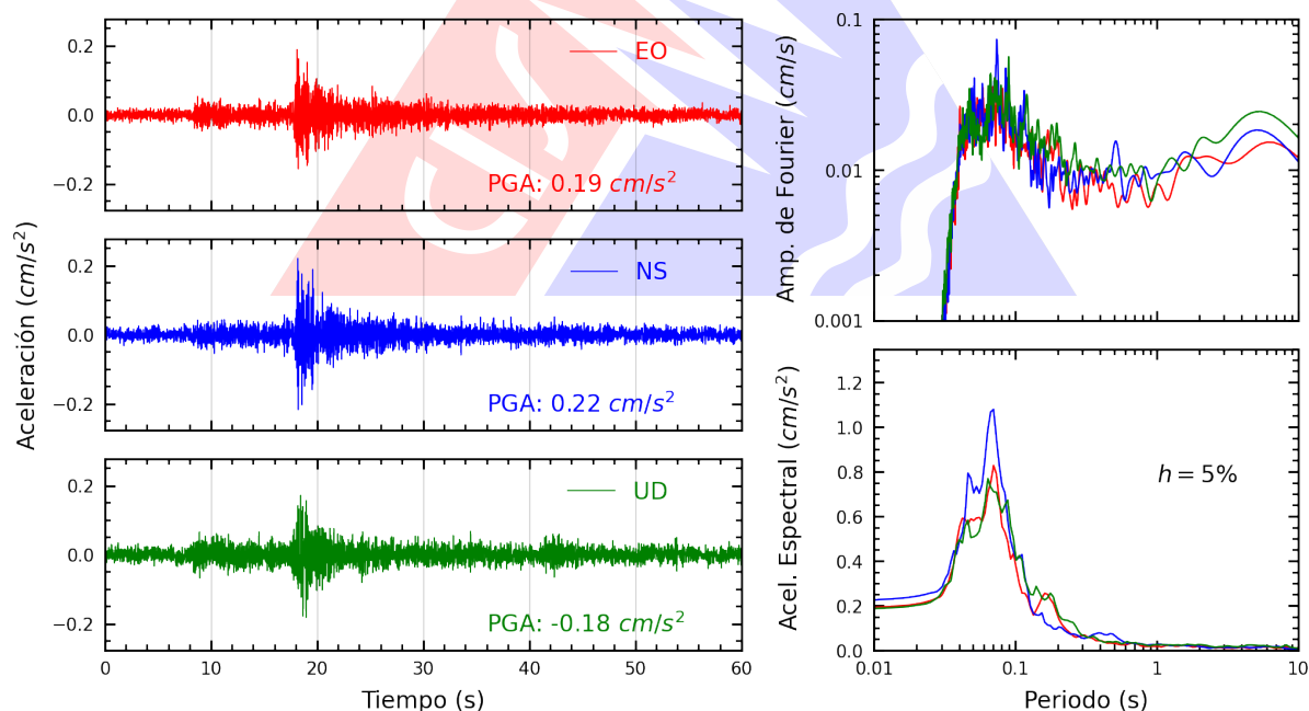
Figura A.20: Registros tiempo-historia, espectros de Fourier y de respuesta en las direcciones EO, NS y vertical de la estación UNFV. Sismo de Chilca, Cañete - Lima del 2026-09-07, 15:57:43 (Hora local)
