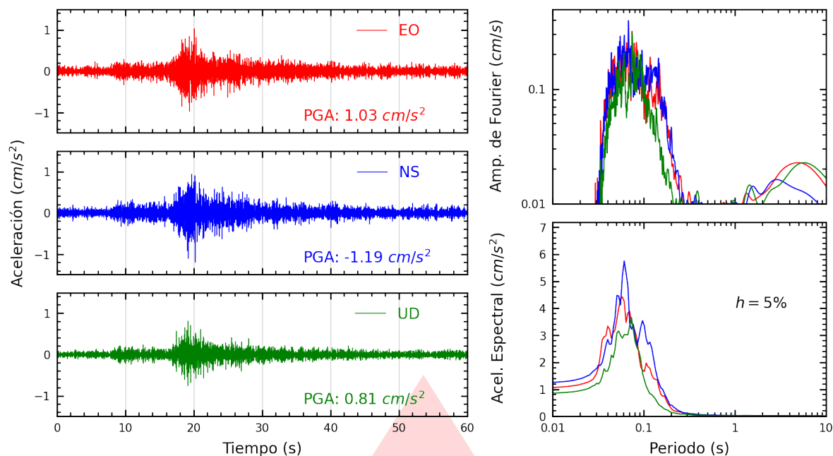
Figura A.5: Registros tiempo-historia, espectros de Fourier y de respuesta en las direcciones EO, NS y vertical de la estación USILM. Sismo de Chilca, Cañete - Lima del 2026-09-07, 15:57:43 (Hora local)
