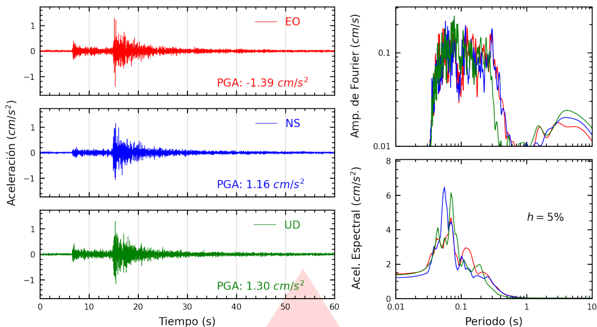
Figura A.3: Registros tiempo-historia, espectros de Fourier y de respuesta en las direcciones EO, NS y vertical de la estación SOVES. Sismo de Chilca, Cañete - Lima del 2026-09-07, 15:57:43 (Hora local)
