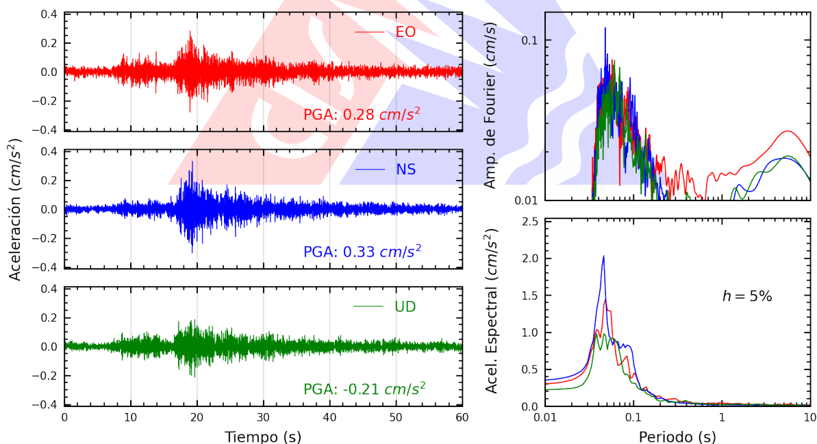
Figura A.18: Registros tiempo-historia, espectros de Fourier y de respuesta en las direcciones EO, NS y vertical de la estación IMCA. Sismo de Chilca, Cañete - Lima del 2026-09-07, 15:57:43 (Hora local)
