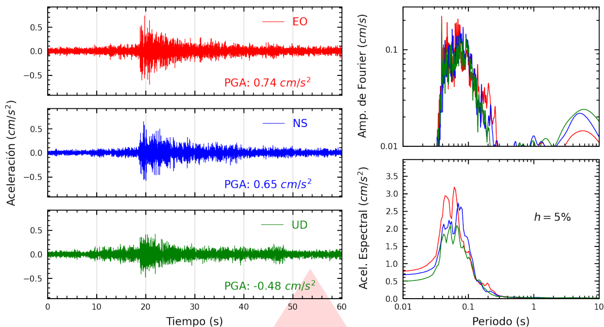
Figura A.9: Registros tiempo-historia, espectros de Fourier y de respuesta en las direcciones EO, NS y vertical de la estación INDEP. Sismo de Chilca, Cañete - Lima del 2026-09-07, 15:57:43 (Hora local)
