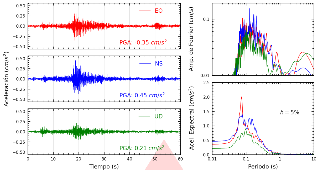
Figura A.1: Registros tiempo-historia, espectros de Fourier y de respuesta en las direcciones EO, NS y vertical de la estación UNTRM. Sismo de Jaén, Jaén - Cajamarca del 2026-09-07, 20:41:17 (Hora local)
