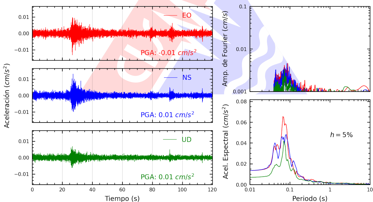
Figura A.2: Registros tiempo-historia, espectros de Fourier y de respuesta en las direcciones EO, NS y vertical de la estación UNSA2. Sismo de Tarata, Tarata - Tacna del 2026-09-10, 01:18:22 (Hora local)
