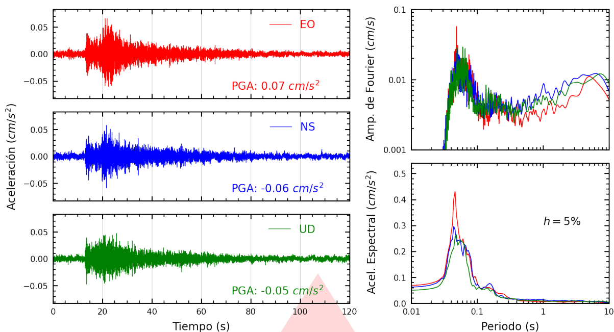
Figura A.1: Registros tiempo-historia, espectros de Fourier y de respuesta en las direcciones EO, NS y vertical de la estación CREY. Sismo de Tarata, Tarata - Tacna del 2026-09-10, 01:18:22 (Hora local)
