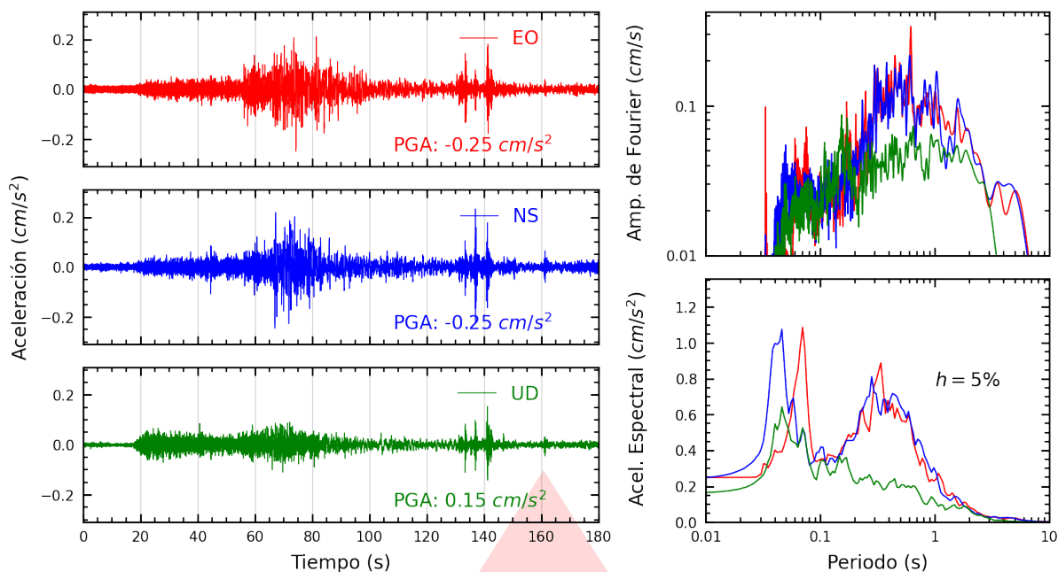
Figura A.1: Registros tiempo-historia, espectros de Fourier y de respuesta en las direcciones EO, NS y vertical de la estación UPAOP. Sismo de Nieva, Condorcanqui - Amazonas del 2026-09-10, 05:39:35 (Hora local)
