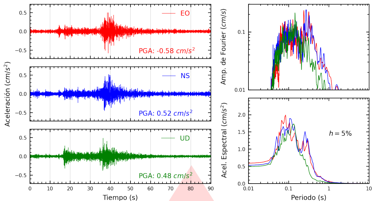
Figura A.1: Registros tiempo-historia, espectros de Fourier y de respuesta en las direcciones EO, NS y vertical de la estación UPAOP. Sismo de Ayabaca, Ayabaca - Piura del 2026-09-10, 14:21:39 (Hora local)
