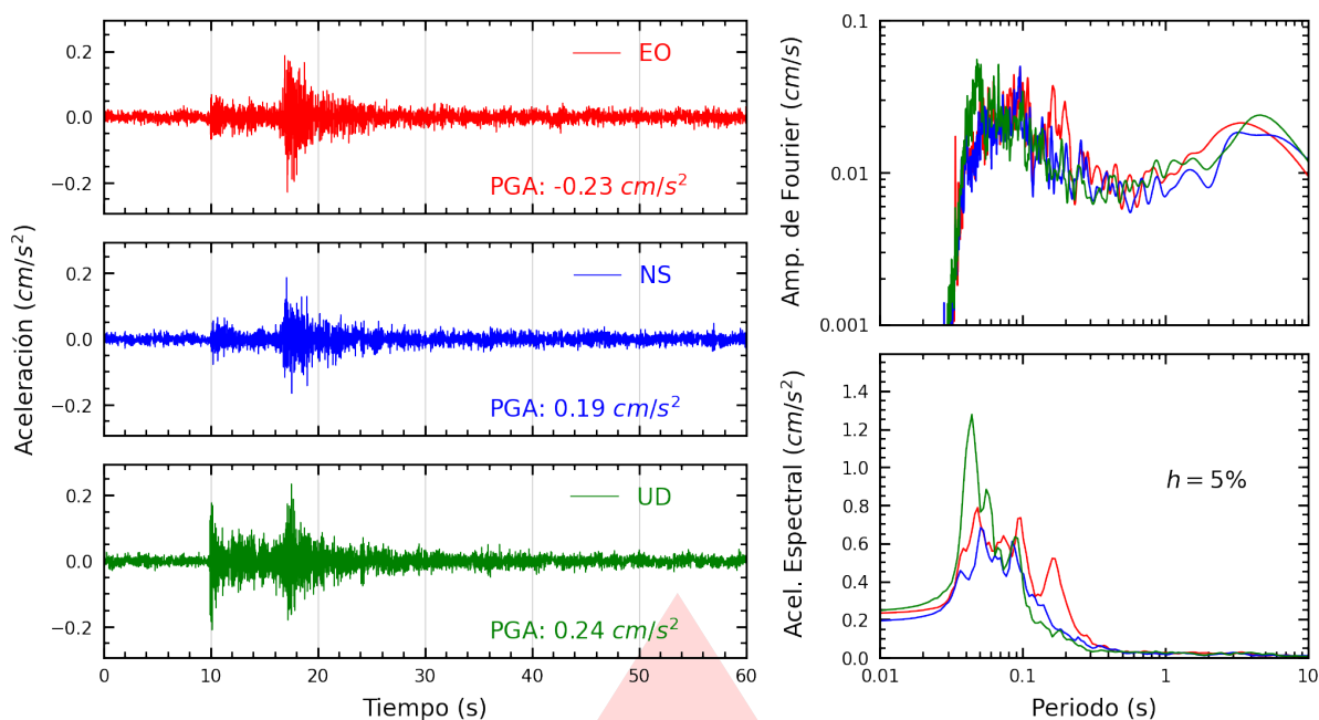
Figura A.9: Registros tiempo-historia, espectros de Fourier y de respuesta en las direcciones EO, NS y vertical de la estación USILP. Sismo de Chilca, Cañete - Lima del 2026-09-11, 17:47:09 (Hora local)
