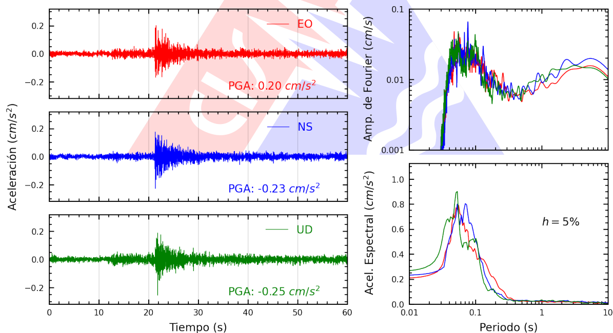
Figura A.8: Registros tiempo-historia, espectros de Fourier y de respuesta en las direcciones EO, NS y vertical de la estación JALVA. Sismo de Chilca, Cañete - Lima del 2026-09-11, 17:47:09 (Hora local)
