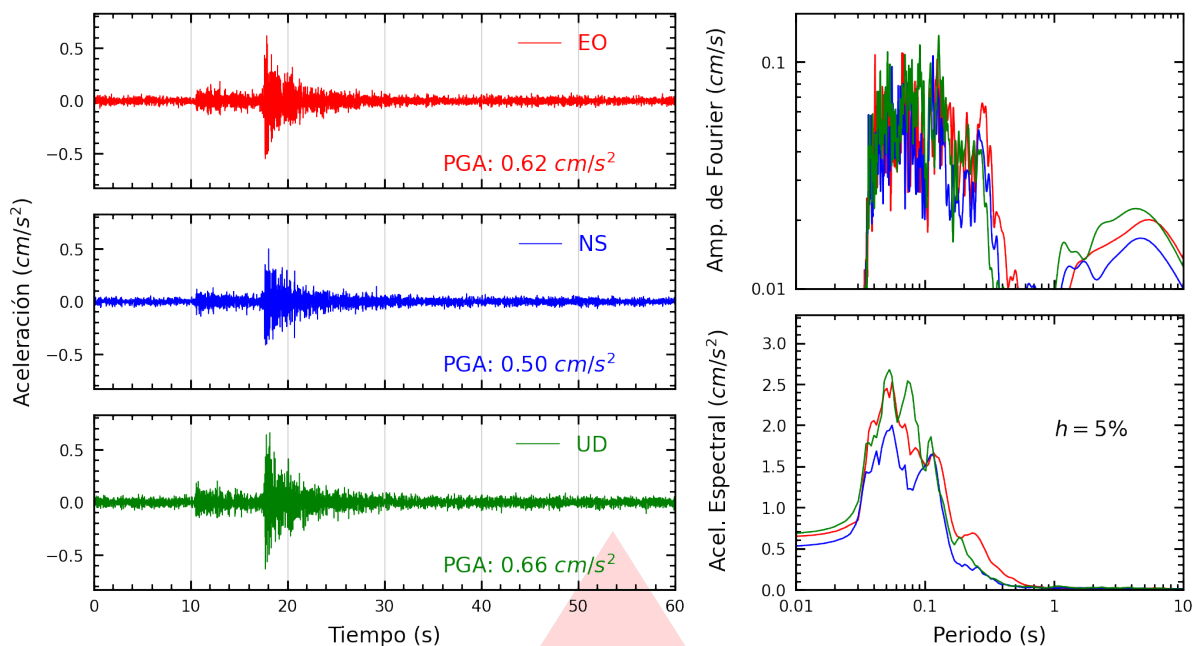
Figura A.5: Registros tiempo-historia, espectros de Fourier y de respuesta en las direcciones EO, NS y vertical de la estación SOVES. Sismo de Chilca, Cañete - Lima del 2026-09-11, 17:47:09 (Hora local)
