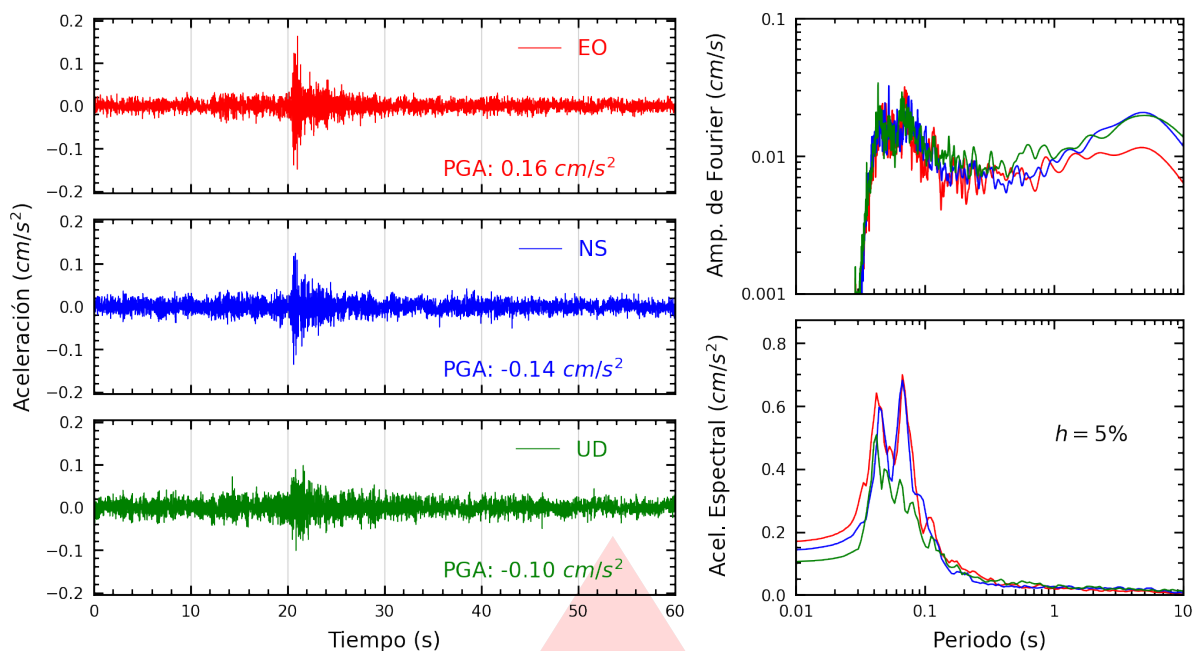
Figura A.13: Registros tiempo-historia, espectros de Fourier y de respuesta en las direcciones EO, NS y vertical de la estación UNFV. Sismo de Chilca, Cañete - Lima del 2026-09-11, 17:47:09 (Hora local)
