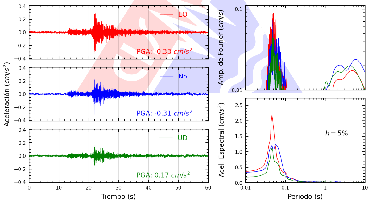
Figura A.6: Registros tiempo-historia, espectros de Fourier y de respuesta en las direcciones EO, NS y vertical de la estación UCSS. Sismo de Chilca, Cañete - Lima del 2026-09-11, 17:47:09 (Hora local)
