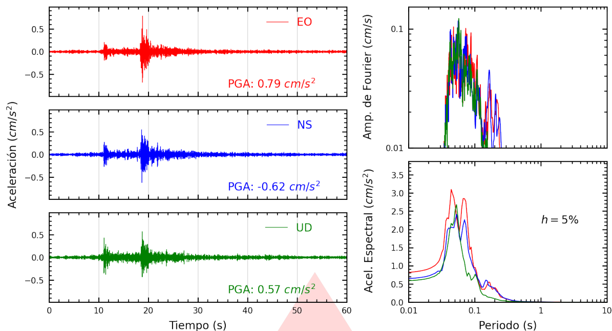
Figura A.3: Registros tiempo-historia, espectros de Fourier y de respuesta en las direcciones EO, NS y vertical de la estación ASIA. Sismo de Chilca, Cañete - Lima del 2026-09-11, 17:47:09 (Hora local)
