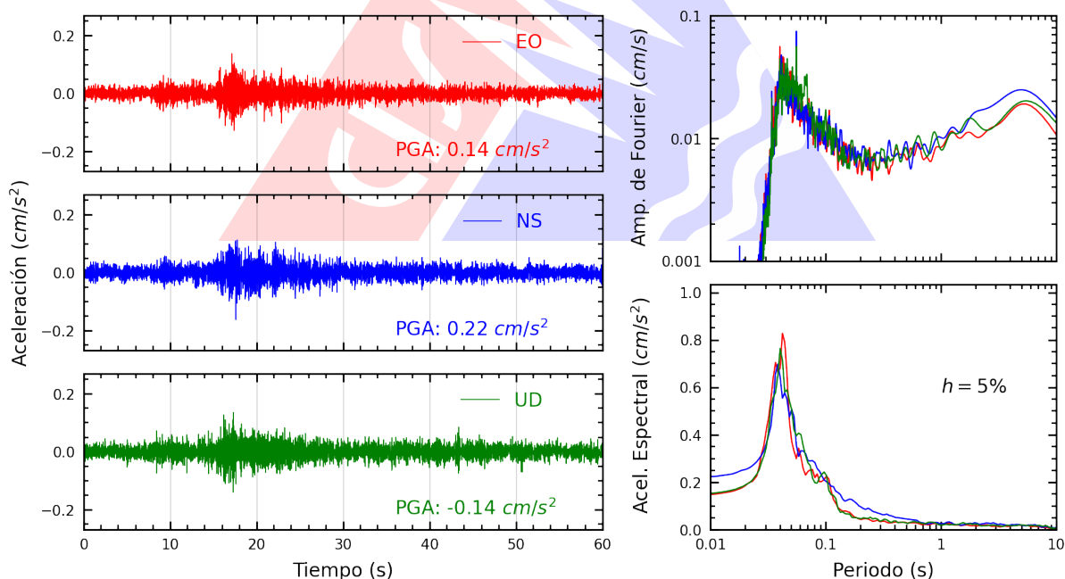
Figura A.12: Registros tiempo-historia, espectros de Fourier y de respuesta en las direcciones EO, NS y vertical de la estación USMP. Sismo de Chilca, Cañete - Lima del 2026-09-11, 17:47:09 (Hora local)
