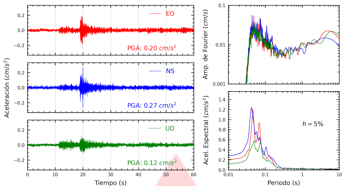
Figura A.7: Registros tiempo-historia, espectros de Fourier y de respuesta en las direcciones EO, NS y vertical de la estación SERVI. Sismo de Chilca, Cañete - Lima del 2026-09-11, 17:47:09 (Hora local)
