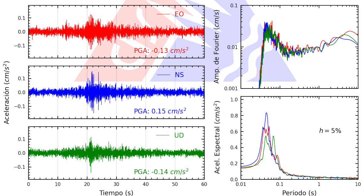
Figura A.14: Registros tiempo-historia, espectros de Fourier y de respuesta en las direcciones EO, NS y vertical de la estación IMCA. Sismo de Chilca, Cañete - Lima del 2026-09-11, 17:47:09 (Hora local)
