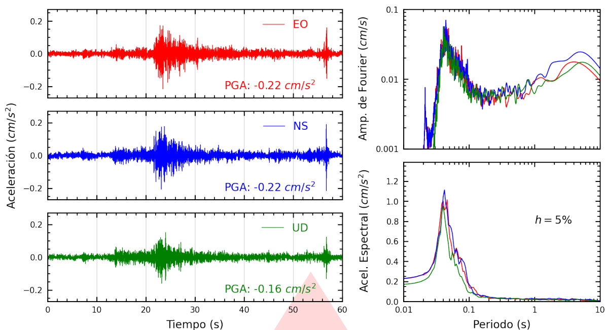
Figura A.11: Registros tiempo-historia, espectros de Fourier y de respuesta en las direcciones EO, NS y vertical de la estación SJLCE. Sismo de Chilca, Cañete - Lima del 2026-09-11, 17:47:09 (Hora local)
