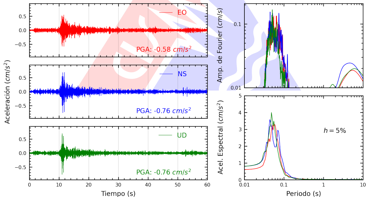
Figura A.4: Registros tiempo-historia, espectros de Fourier y de respuesta en las direcciones EO, NS y vertical de la estación JOSEO. Sismo de Chilca, Cañete - Lima del 2026-09-11, 17:47:09 (Hora local)
