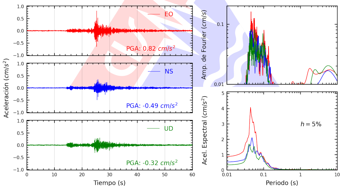
Figura A.2: Registros tiempo-historia, espectros de Fourier y de respuesta en las direcciones EO, NS y vertical de la estación AMORE. Sismo de Chilca, Cañete - Lima del 2026-09-11, 17:47:09 (Hora local)
