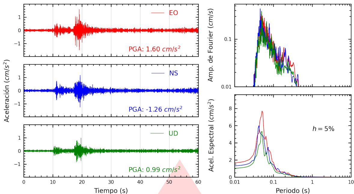
Figura A.1: Registros tiempo-historia, espectros de Fourier y de respuesta en las direcciones EO, NS y vertical de la estación UNTEL. Sismo de Chilca, Cañete - Lima del 2026-09-11, 17:47:09 (Hora local)
