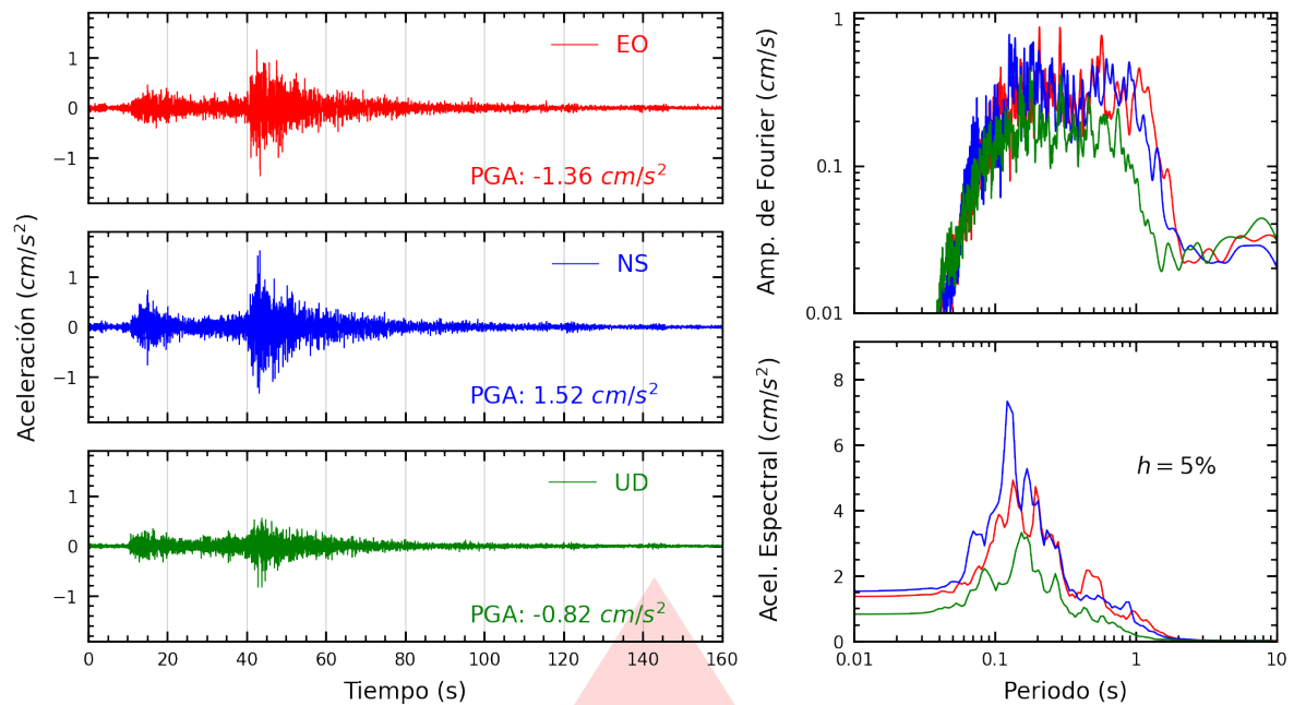
Figura A.1: Registros tiempo-historia, espectros de Fourier y de respuesta en las direcciones EO, NS y vertical de la estación UNTRM. Sismo de Andoas, Datem del Marañón - Loreto del 2026-09-14, 14:16:47 (Hora local)
