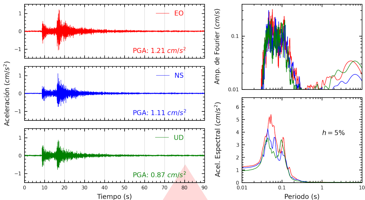
Figura A.3: Registros tiempo-historia, espectros de Fourier y de respuesta en las direcciones EO, NS y vertical de la estación AMORE. Sismo de Ancón, Lima - Lima del 2026-09-15, 10:30:38 (Hora local)
