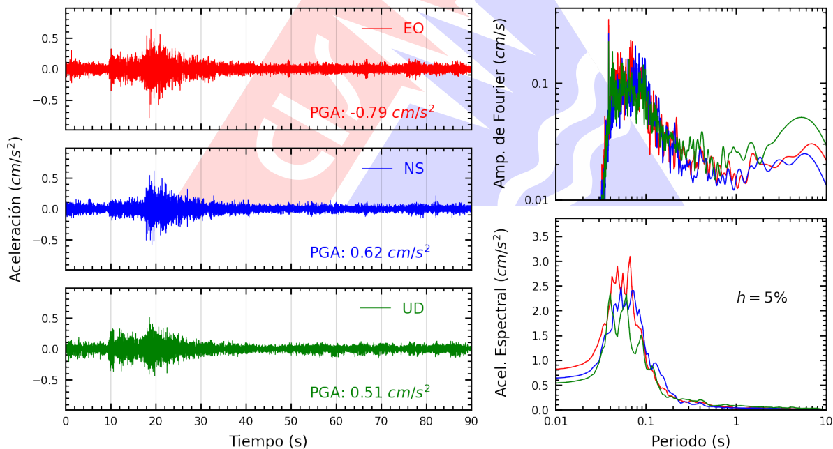
Figura A.4: Registros tiempo-historia, espectros de Fourier y de respuesta en las direcciones EO, NS y vertical de la estación INDEP. Sismo de Ancón, Lima - Lima del 2026-09-15, 10:30:38 (Hora local)
