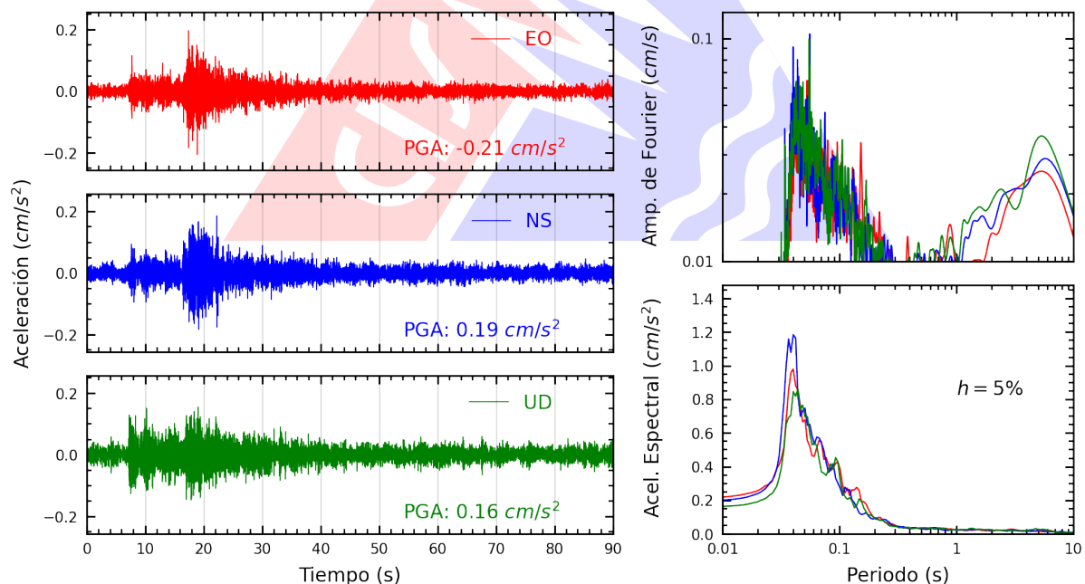
Figura A.12: Registros tiempo-historia, espectros de Fourier y de respuesta en las direcciones EO, NS y vertical de la estación USMP. Sismo de Ancón, Lima - Lima del 2026-09-15, 10:30:38 (Hora local)
