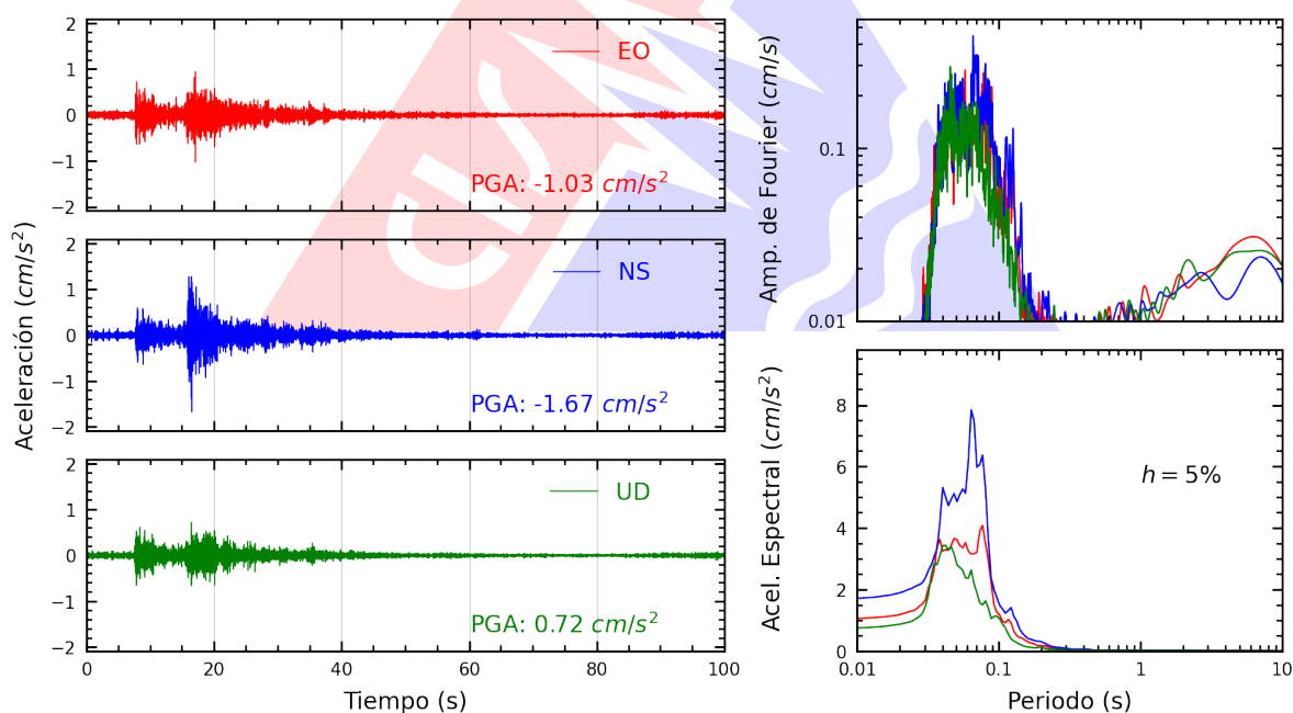
Figura A.2: Registros tiempo-historia, espectros de Fourier y de respuesta en las direcciones EO, NS y vertical de la estación JOSEO. Sismo de Ancón, Lima - Lima del 2026-09-15, 10:30:38 (Hora local)
