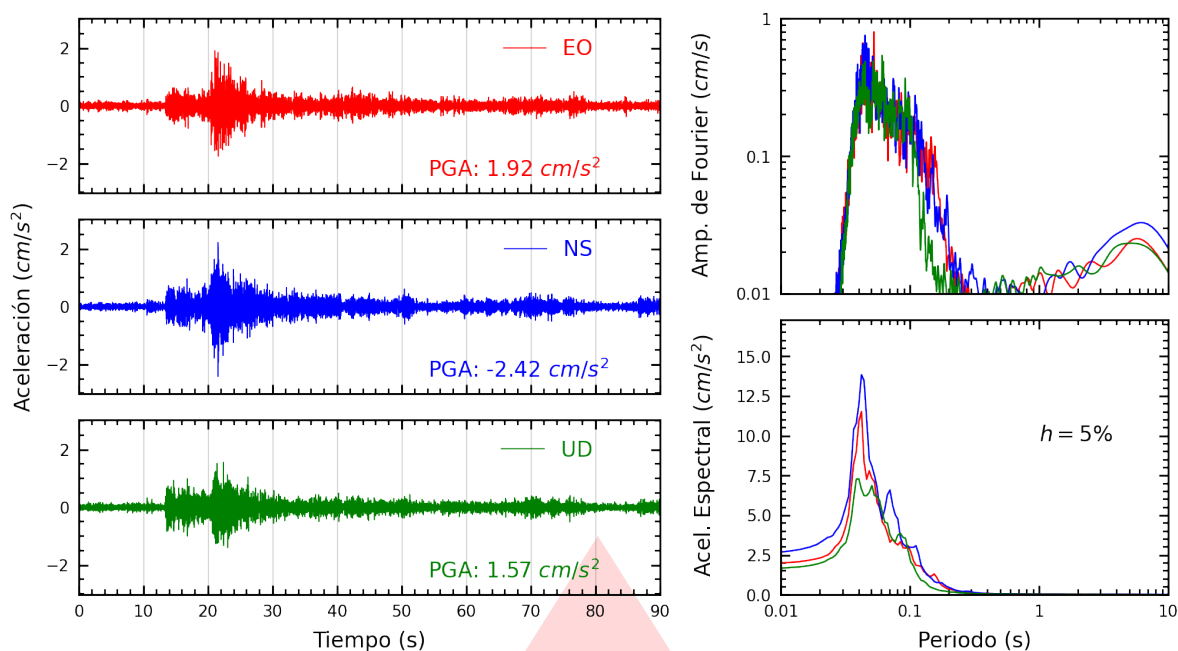
Figura A.1: Registros tiempo-historia, espectros de Fourier y de respuesta en las direcciones EO, NS y vertical de la estación SROSA. Sismo de Ancón, Lima - Lima del 2026-09-15, 10:30:38 (Hora local)
