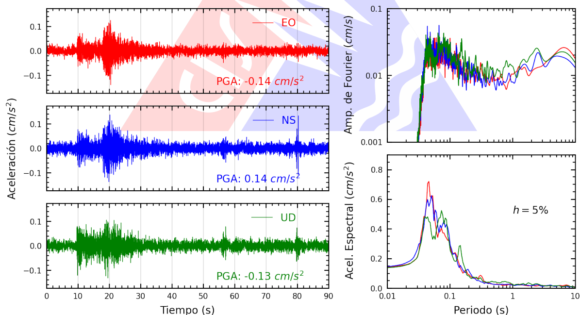
Figura A.14: Registros tiempo-historia, espectros de Fourier y de respuesta en las direcciones EO, NS y vertical de la estación UNFV. Sismo de Ancón, Lima - Lima del 2026-09-15, 10:30:38 (Hora local)
