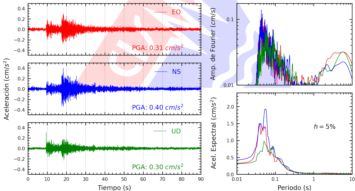
Figura A.6: Registros tiempo-historia, espectros de Fourier y de respuesta en las direcciones EO, NS y vertical de la estación COMAS. Sismo de Ancón, Lima - Lima del 2026-09-15, 10:30:38 (Hora local)
