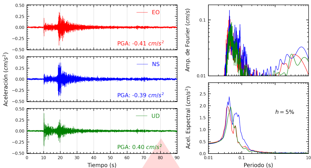
Figura A.5: Registros tiempo-historia, espectros de Fourier y de respuesta en las direcciones EO, NS y vertical de la estación SJLCE. Sismo de Ancón, Lima - Lima del 2026-09-15, 10:30:38 (Hora local)
