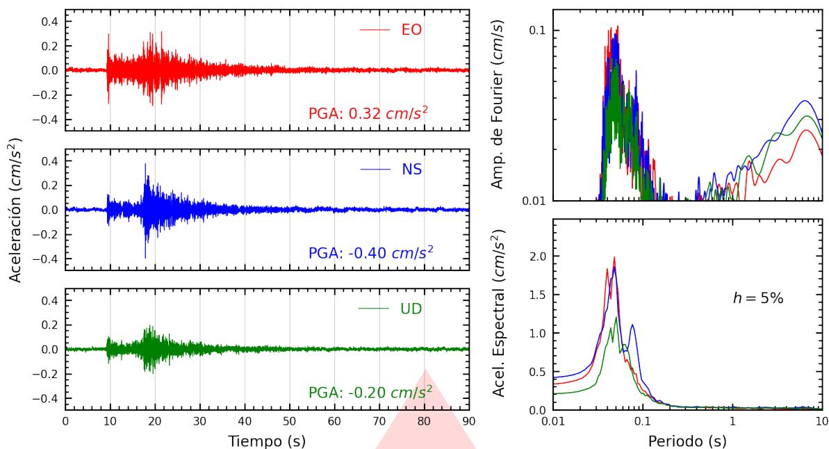
Figura A.7: Registros tiempo-historia, espectros de Fourier y de respuesta en las direcciones EO, NS y vertical de la estación UCSS. Sismo de Ancón, Lima - Lima del 2026-09-15, 10:30:38 (Hora local)
