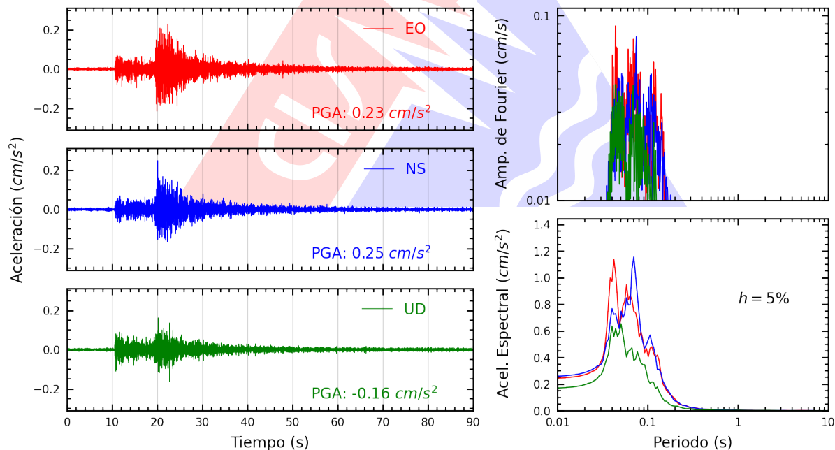
Figura A.10: Registros tiempo-historia, espectros de Fourier y de respuesta en las direcciones EO, NS y vertical de la estación ATARJ. Sismo de Ancón, Lima - Lima del 2026-09-15, 10:30:38 (Hora local)
