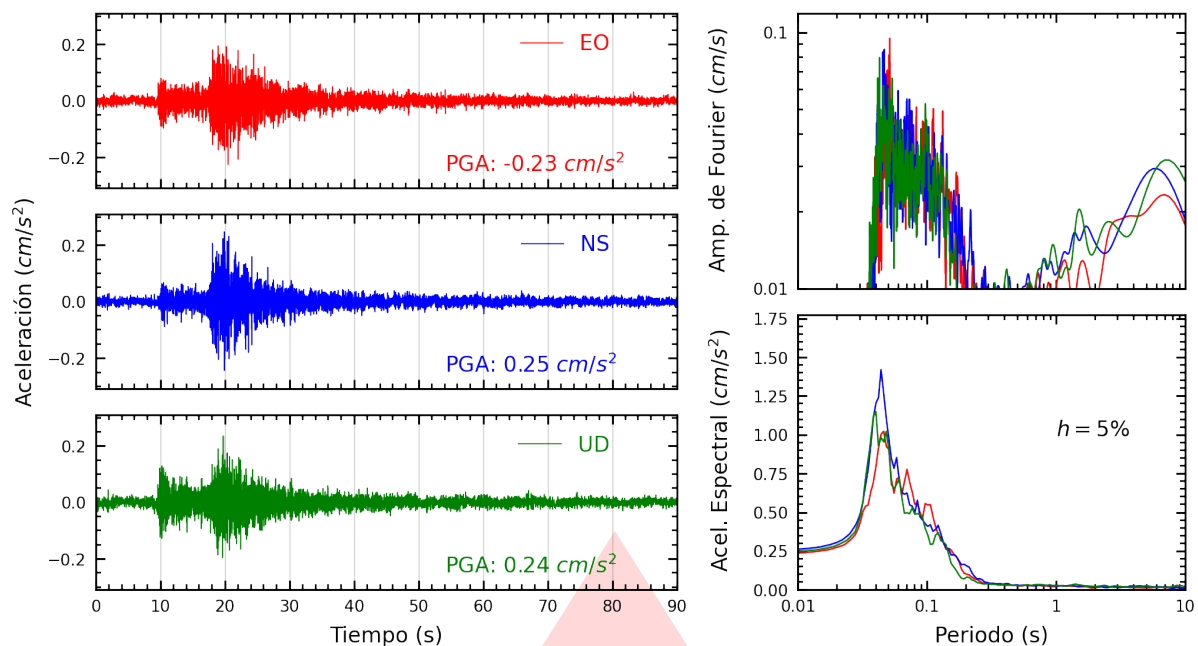
Figura A.11: Registros tiempo-historia, espectros de Fourier y de respuesta en las direcciones EO, NS y vertical de la estación JALVA. Sismo de Ancón, Lima - Lima del 2026-09-15, 10:30:38 (Hora local)
