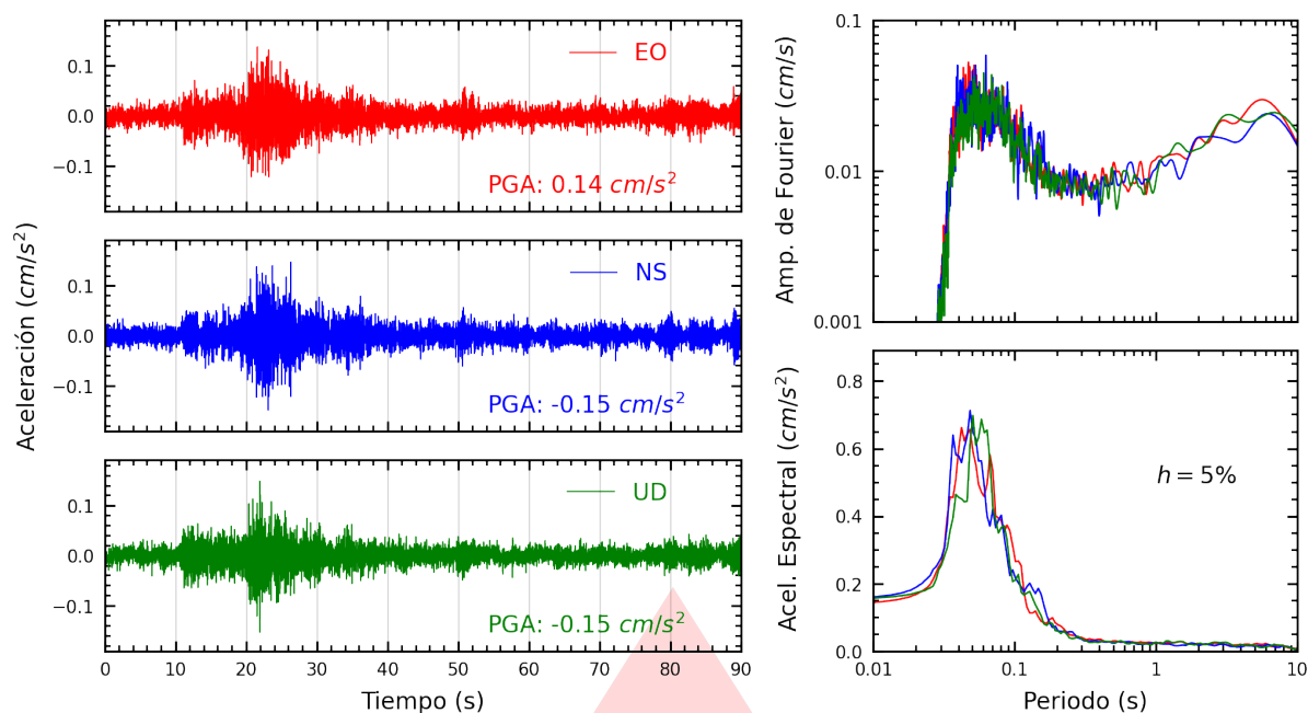
Figura A.13: Registros tiempo-historia, espectros de Fourier y de respuesta en las direcciones EO, NS y vertical de la estación SERVI. Sismo de Ancón, Lima - Lima del 2026-09-15, 10:30:38 (Hora local)
