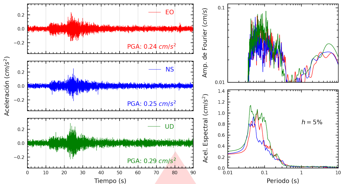
Figura A.9: Registros tiempo-historia, espectros de Fourier y de respuesta en las direcciones EO, NS y vertical de la estación SOVES. Sismo de Ancón, Lima - Lima del 2026-09-15, 10:30:38 (Hora local)
