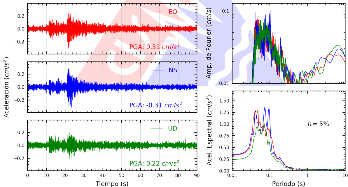
Figura A.8: Registros tiempo-historia, espectros de Fourier y de respuesta en las direcciones EO, NS y vertical de la estación UCVAT. Sismo de Ancón, Lima - Lima del 2026-09-15, 10:30:38 (Hora local)
