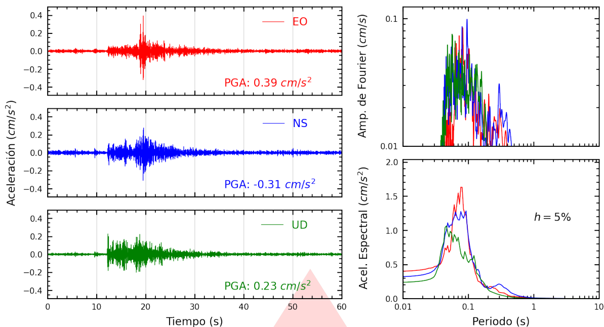
Figura A.1: Registros tiempo-historia, espectros de Fourier y de respuesta en las direcciones EO, NS y vertical de la estación UPAOP. Sismo de Sullana, Sullana - Piura del 2026-09-16, 22:26:53 (Hora local)
