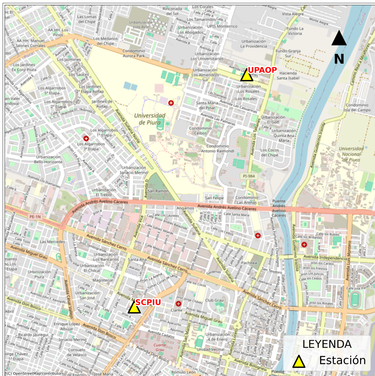
Figura 2: Mapa de ubicación de la(s) estación(es) acelerográfica(s) correspondiente(s) al Sismo de Sullana, Sullana - Piura del 16 de setiembre de 2026 a las 22:26:53 (hora local)
