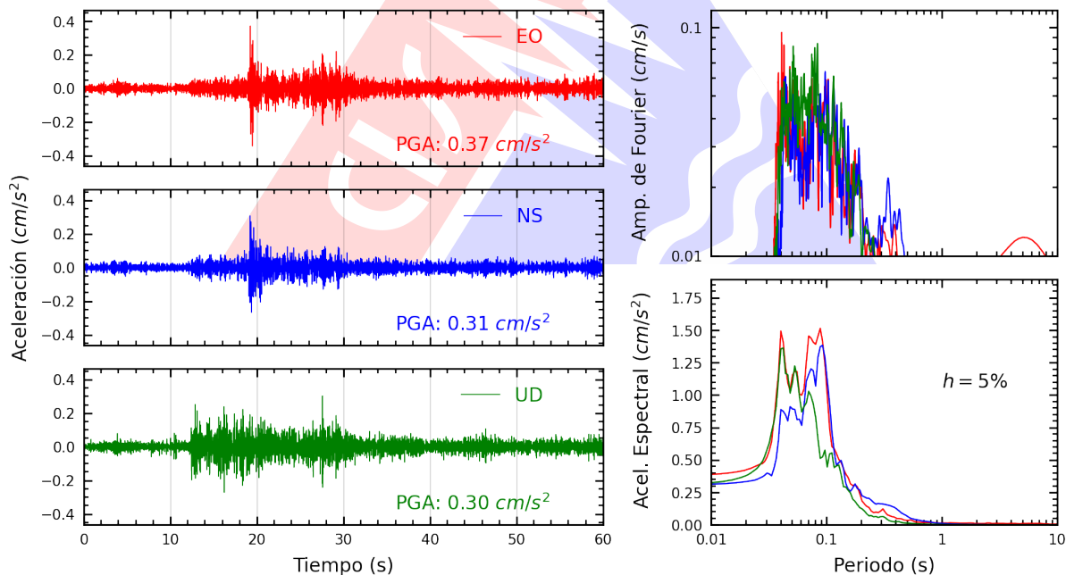
Figura A.2: Registros tiempo-historia, espectros de Fourier y de respuesta en las direcciones EO, NS y vertical de la estación SCPIU. Sismo de Sullana, Sullana - Piura del 2026-09-16, 22:26:53 (Hora local)
