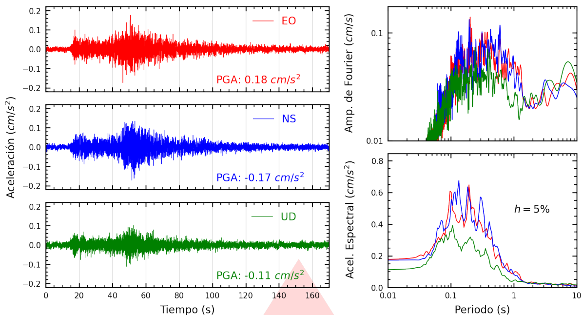
Figura A.5: Registros tiempo-historia, espectros de Fourier y de respuesta en las direcciones EO, NS y vertical de la estación UNTRM. Sismo de Salaverry, Trujillo - La Libertad del 2026-09-20, 22:58:23 (Hora local)
