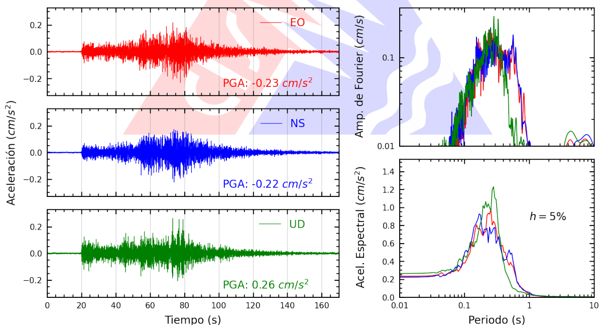
Figura A.4: Registros tiempo-historia, espectros de Fourier y de respuesta en las direcciones EO, NS y vertical de la estación CARAL. Sismo de Salaverry, Trujillo - La Libertad del 2026-09-20, 22:58:23 (Hora local)
