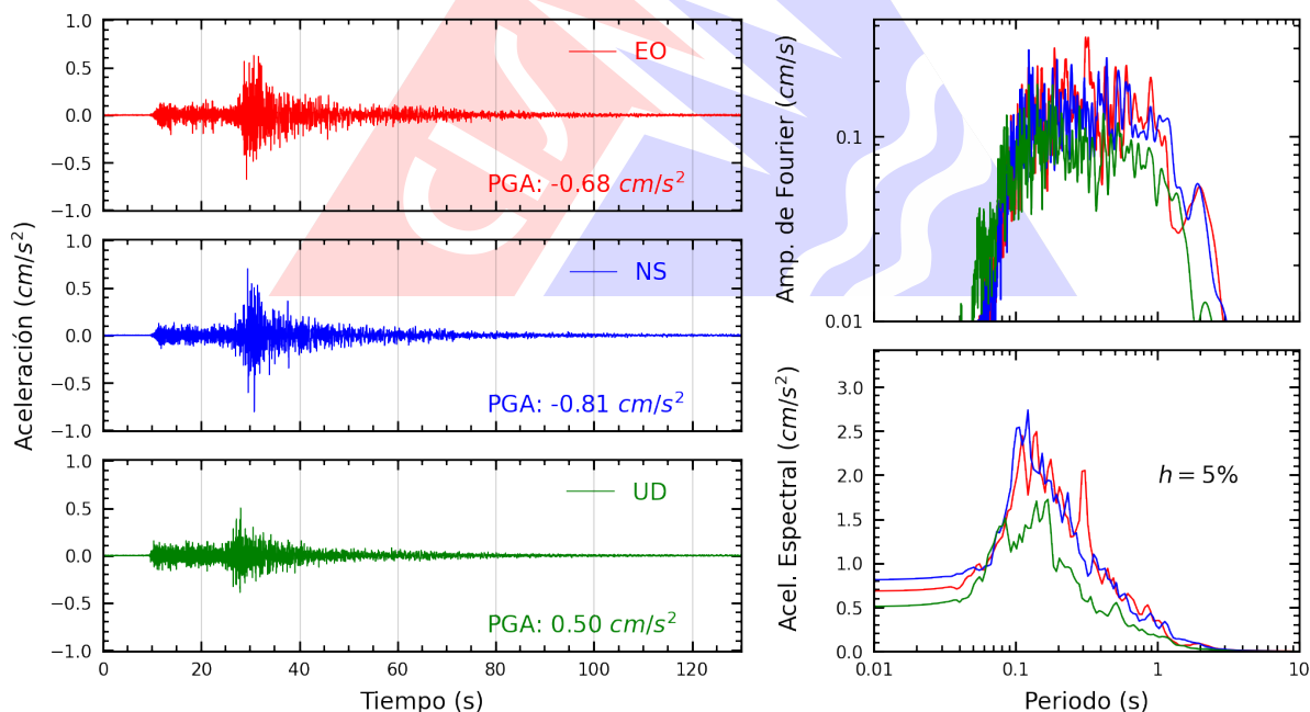
Figura A.2: Registros tiempo-historia, espectros de Fourier y de respuesta en las direcciones EO, NS y vertical de la estación UNC. Sismo de Salaverry, Trujillo - La Libertad del 2026-09-20, 22:58:23 (Hora local)
