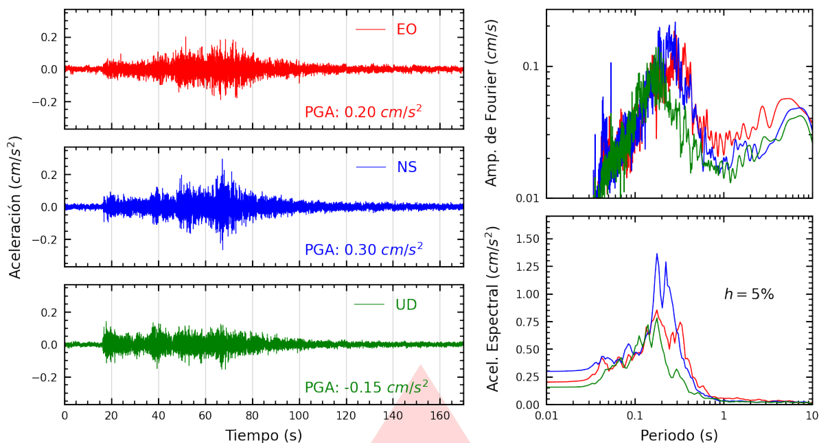
Figura A.3: Registros tiempo-historia, espectros de Fourier y de respuesta en las direcciones EO, NS y vertical de la estación UNAB. Sismo de Salaverry, Trujillo - La Libertad del 2026-09-20, 22:58:23 (Hora local)
