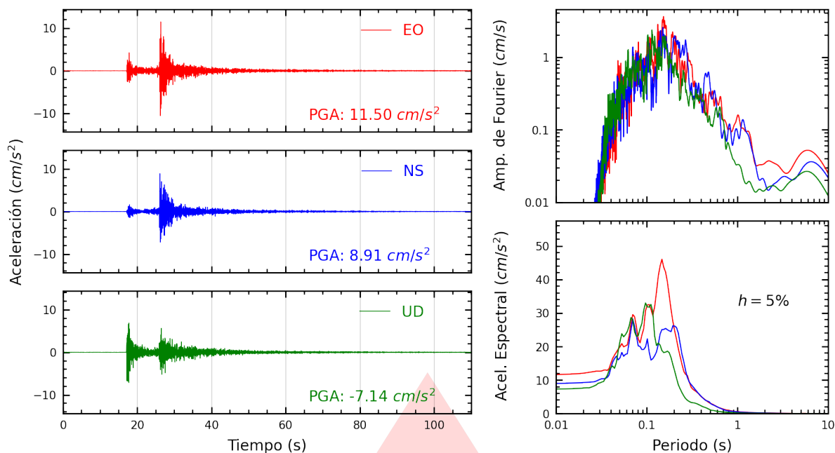
Figura A.1: Registros tiempo-historia, espectros de Fourier y de respuesta en las direcciones EO, NS y vertical de la estación UPAOT. Sismo de Salaverry, Trujillo - La Libertad del 2026-09-20, 22:58:23 (Hora local)
