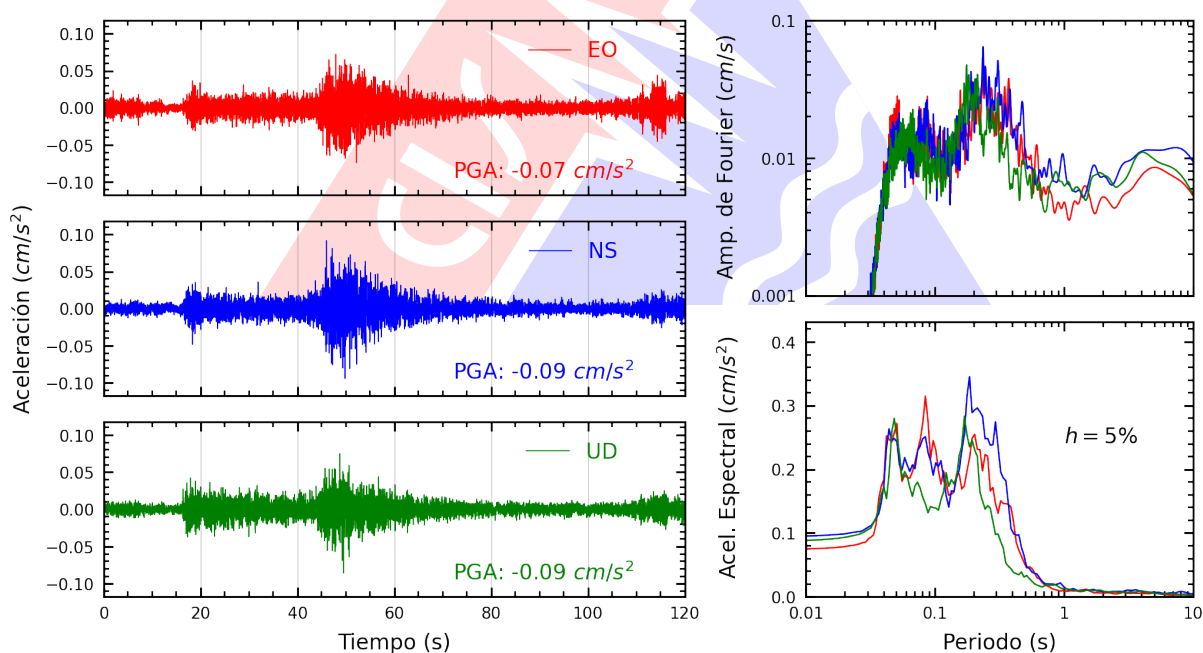
Figura A.2: Registros tiempo-historia, espectros de Fourier y de respuesta en las direcciones EO, NS y vertical de la estación CREY. Sismo de Vitor, Arequipa - Arequipa del 2026-09-22, 04:56:07 (Hora local)
