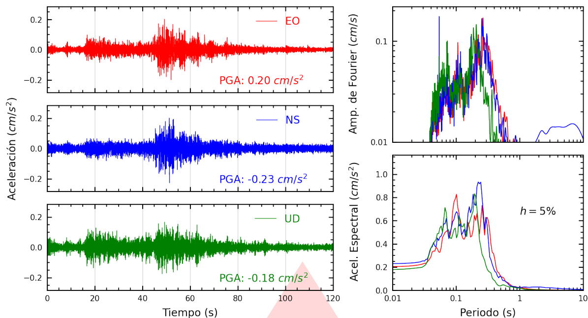
Figura A.1: Registros tiempo-historia, espectros de Fourier y de respuesta en las direcciones EO, NS y vertical de la estación SCTAC. Sismo de Vitor, Arequipa - Arequipa del 2026-09-22, 04:56:07 (Hora local)
