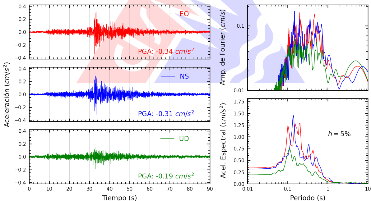
Figura A.2: Registros tiempo-historia, espectros de Fourier y de respuesta en las direcciones EO, NS y vertical de la estación UNTRM. Sismo de San Antonio, San Martín - San Martín del 2026-09-24, 20:50:06 (Hora local)
