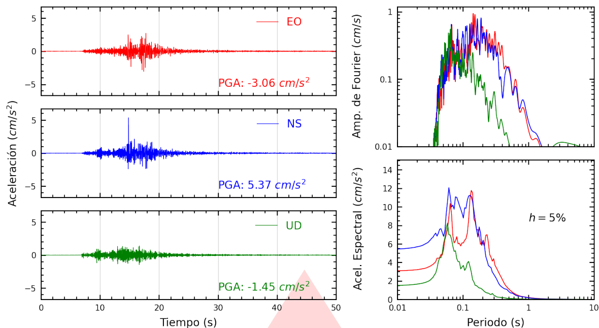
Figura A.1: Registros tiempo-historia, espectros de Fourier y de respuesta en las direcciones EO, NS y vertical de la estación UNAAA. Sismo de San Antonio, San Martín - San Martín del 2026-09-24, 20:50:06 (Hora local)
