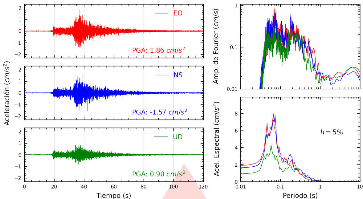
Figura A.33: Registros tiempo-historia, espectros de Fourier y de respuesta en las direcciones EO, NS y vertical de la estación UPCVI. Sismo de Huacho, Huaura - Lima del 2026-09-24, 23:26:28 (Hora local)
