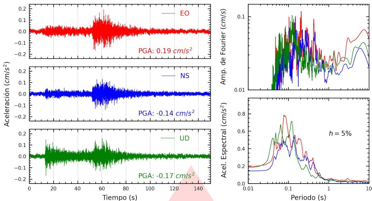
Figura A.43: Registros tiempo-historia, espectros de Fourier y de respuesta en las direcciones EO, NS y vertical de la estación UPAOT. Sismo de Huacho, Huaura - Lima del 2026-09-24, 23:26:28 (Hora local)
