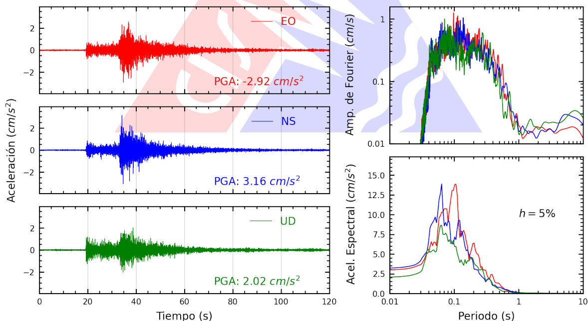
Figura A.18: Registros tiempo-historia, espectros de Fourier y de respuesta en las direcciones EO, NS y vertical de la estación URPE. Sismo de Huacho, Huaura - Lima del 2026-09-24, 23:26:28 (Hora local)
