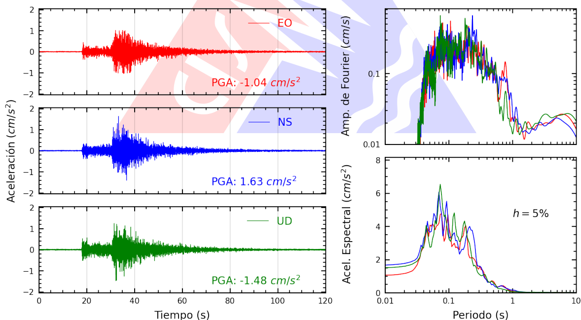
Figura A.34: Registros tiempo-historia, espectros de Fourier y de respuesta en las direcciones EO, NS y vertical de la estación UNFV. Sismo de Huacho, Huaura - Lima del 2026-09-24, 23:26:28 (Hora local)
