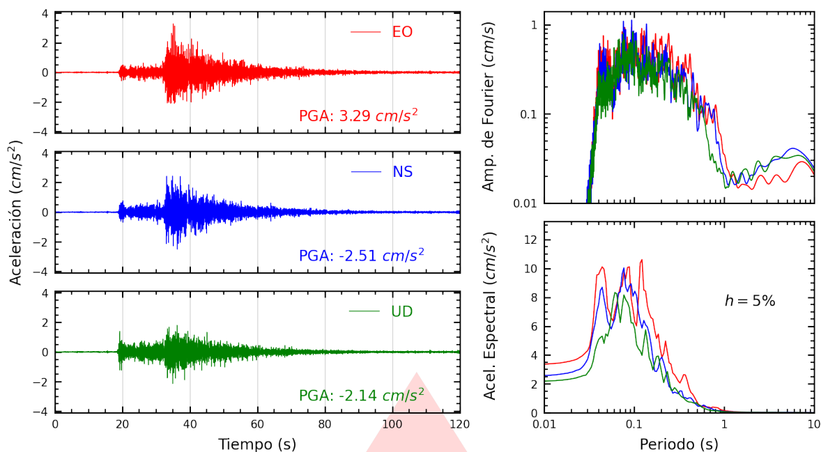
Figura A.17: Registros tiempo-historia, espectros de Fourier y de respuesta en las direcciones EO, NS y vertical de la estación UCVAT. Sismo de Huacho, Huaura - Lima del 2026-09-24, 23:26:28 (Hora local)
