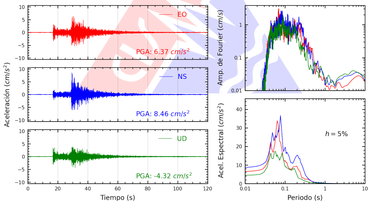
Figura A.4: Registros tiempo-historia, espectros de Fourier y de respuesta en las direcciones EO, NS y vertical de la estación INDEP. Sismo de Huacho, Huaura - Lima del 2026-09-24, 23:26:28 (Hora local)
