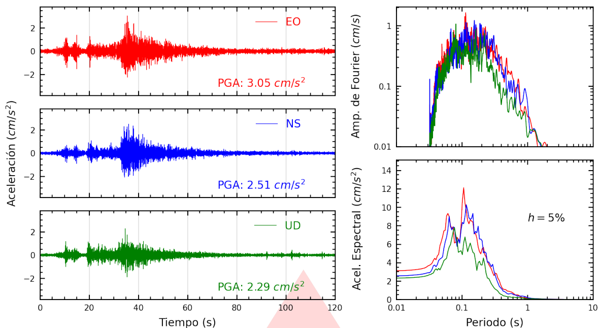
Figura A.21: Registros tiempo-historia, espectros de Fourier y de respuesta en las direcciones EO, NS y vertical de la estación SOBAR. Sismo de Huacho, Huaura - Lima del 2026-09-24, 23:26:28 (Hora local)
