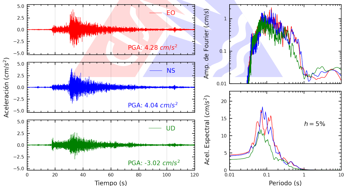
Figura A.12: Registros tiempo-historia, espectros de Fourier y de respuesta en las direcciones EO, NS y vertical de la estación SJLSV. Sismo de Huacho, Huaura - Lima del 2026-09-24, 23:26:28 (Hora local)
