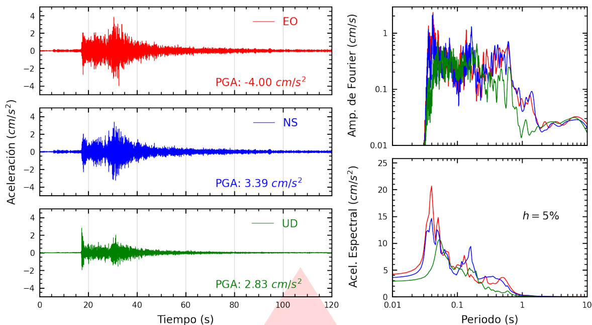
Figura A.13: Registros tiempo-historia, espectros de Fourier y de respuesta en las direcciones EO, NS y vertical de la estación DHNPE. Sismo de Huacho, Huaura - Lima del 2026-09-24, 23:26:28 (Hora local)
