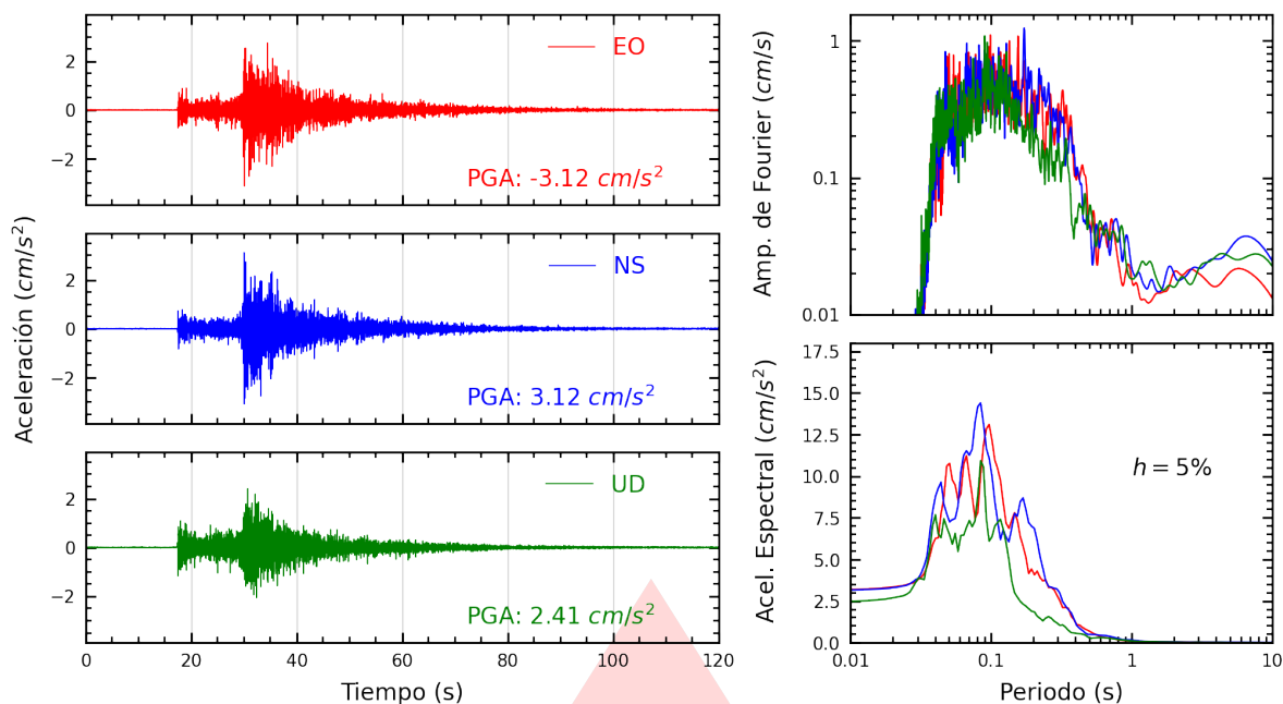
Figura A.19: Registros tiempo-historia, espectros de Fourier y de respuesta en las direcciones EO, NS y vertical de la estación JALVA. Sismo de Huacho, Huaura - Lima del 2026-09-24, 23:26:28 (Hora local)
