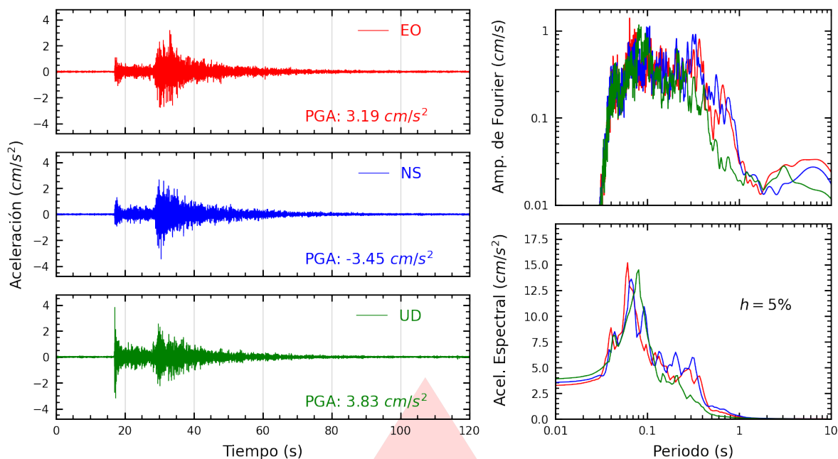
Figura A.15: Registros tiempo-historia, espectros de Fourier y de respuesta en las direcciones EO, NS y vertical de la estación MADRE. Sismo de Huacho, Huaura - Lima del 2026-09-24, 23:26:28 (Hora local)
