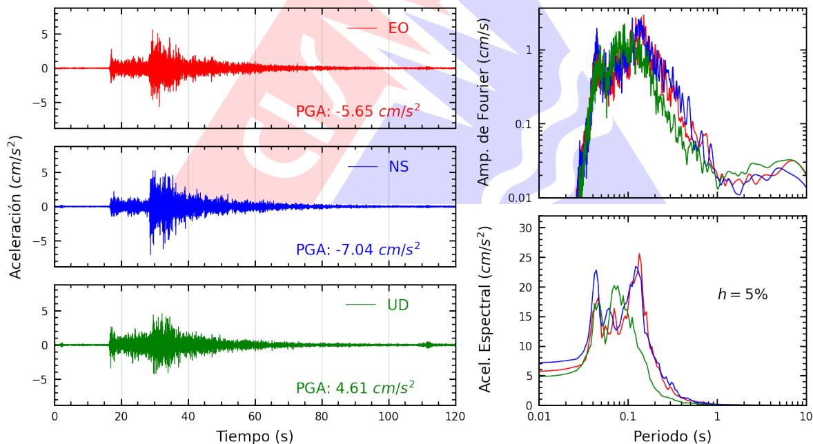
Figura A.6: Registros tiempo-historia, espectros de Fourier y de respuesta en las direcciones EO, NS y vertical de la estación CARAB. Sismo de Huacho, Huaura - Lima del 2026-09-24, 23:26:28 (Hora local)
