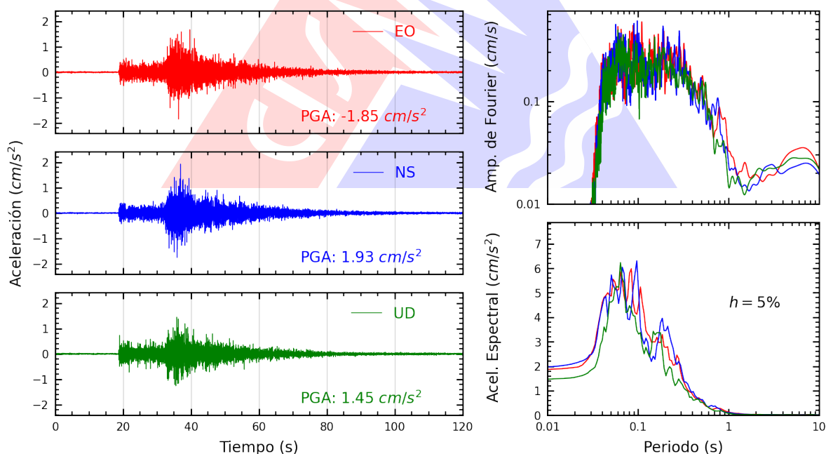
Figura A.32: Registros tiempo-historia, espectros de Fourier y de respuesta en las direcciones EO, NS y vertical de la estación IMCA. Sismo de Huacho, Huaura - Lima del 2026-09-24, 23:26:28 (Hora local)
