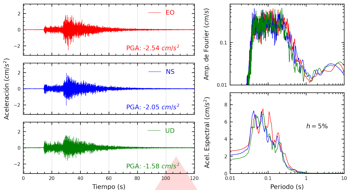
Figura A.27: Registros tiempo-historia, espectros de Fourier y de respuesta en las direcciones EO, NS y vertical de la estación USMP. Sismo de Huacho, Huaura - Lima del 2026-09-24, 23:26:28 (Hora local)
