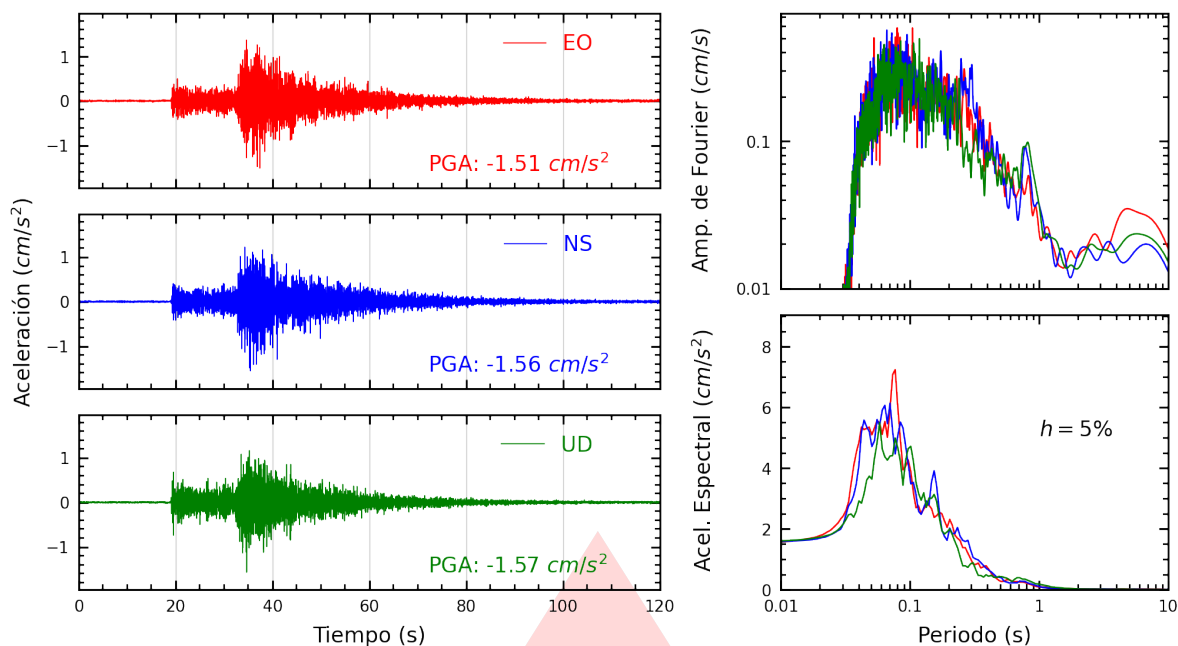
Figura A.37: Registros tiempo-historia, espectros de Fourier y de respuesta en las direcciones EO, NS y vertical de la estación SERVI. Sismo de Huacho, Huaura - Lima del 2026-09-24, 23:26:28 (Hora local)
