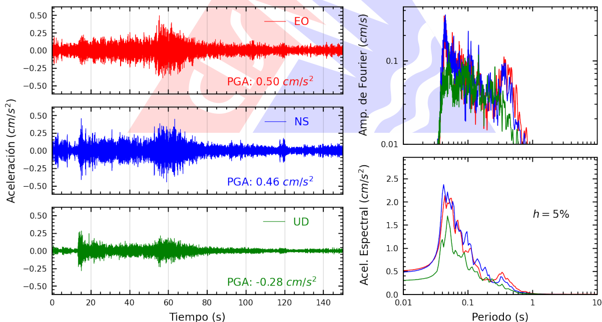
Figura A.42: Registros tiempo-historia, espectros de Fourier y de respuesta en las direcciones EO, NS y vertical de la estación SCTRU. Sismo de Huacho, Huaura - Lima del 2026-09-24, 23:26:28 (Hora local)
