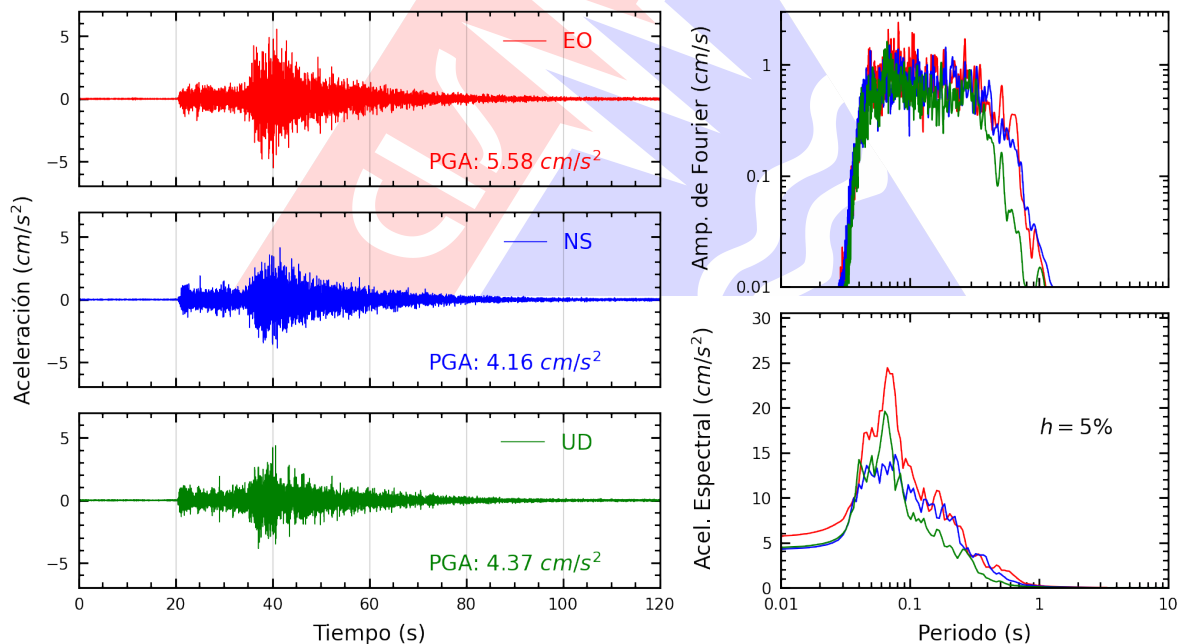
Figura A.8: Registros tiempo-historia, espectros de Fourier y de respuesta en las direcciones EO, NS y vertical de la estación UNTEL. Sismo de Huacho, Huaura - Lima del 2026-09-24, 23:26:28 (Hora local)
