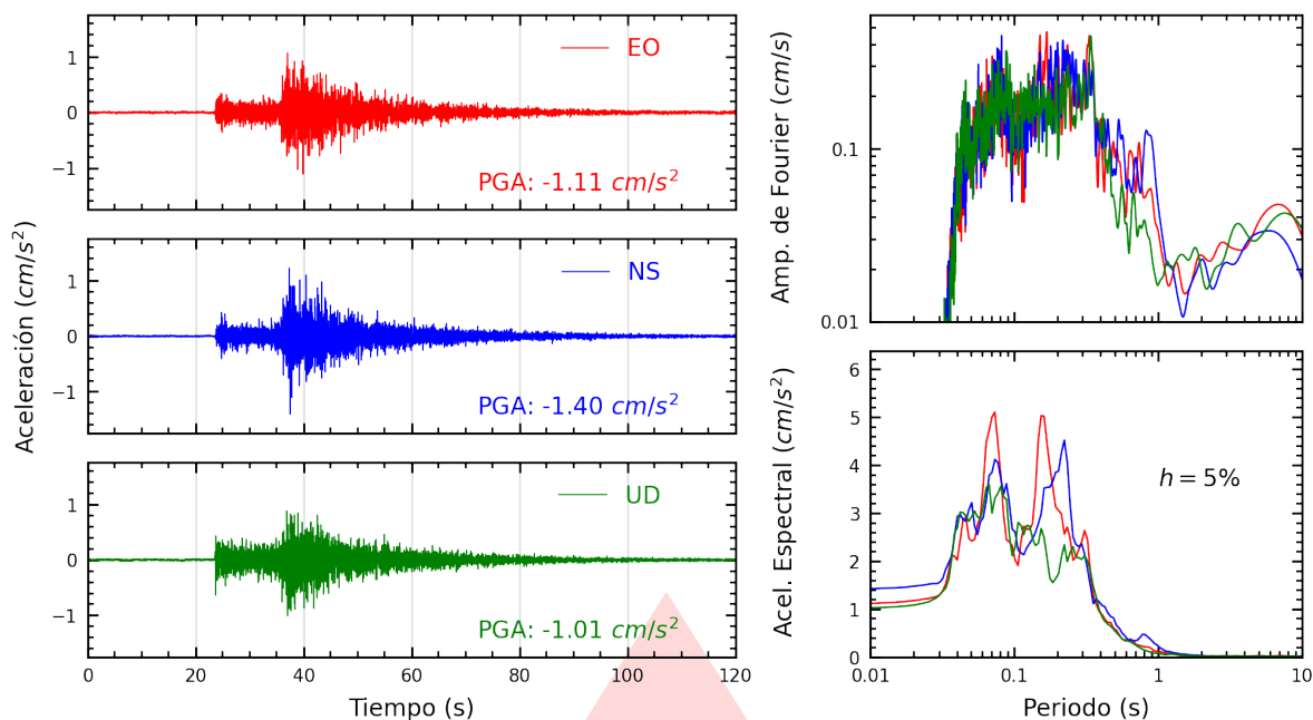
Figura A.39: Registros tiempo-historia, espectros de Fourier y de respuesta en las direcciones EO, NS y vertical de la estación UNMSM. Sismo de Huacho, Huaura - Lima del 2026-09-24, 23:26:28 (Hora local)
