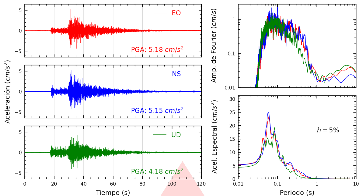
Figura A.9: Registros tiempo-historia, espectros de Fourier y de respuesta en las direcciones EO, NS y vertical de la estación SJLSC. Sismo de Huacho, Huaura - Lima del 2026-09-24, 23:26:28 (Hora local)
