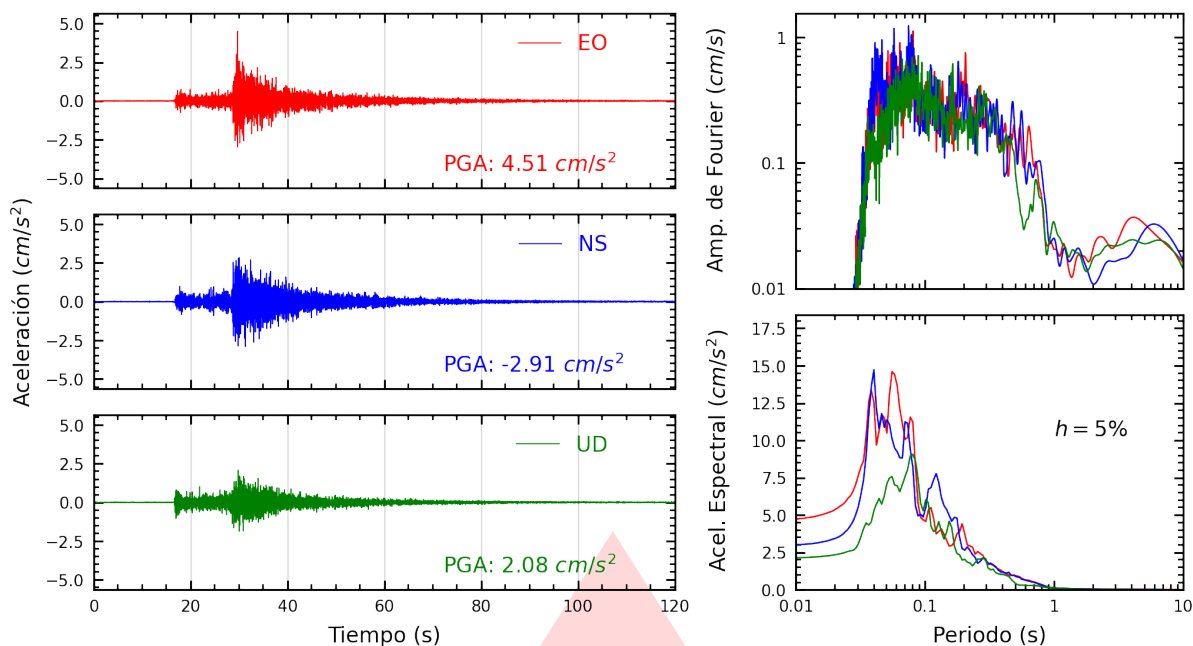
Figura A.11: Registros tiempo-historia, espectros de Fourier y de respuesta en las direcciones EO, NS y vertical de la estación COMAS. Sismo de Huacho, Huaura - Lima del 2026-09-24, 23:26:28 (Hora local)
