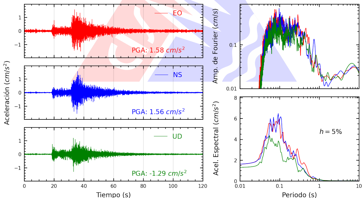
Figura A.36: Registros tiempo-historia, espectros de Fourier y de respuesta en las direcciones EO, NS y vertical de la estación INICT. Sismo de Huacho, Huaura - Lima del 2026-09-24, 23:26:28 (Hora local)
