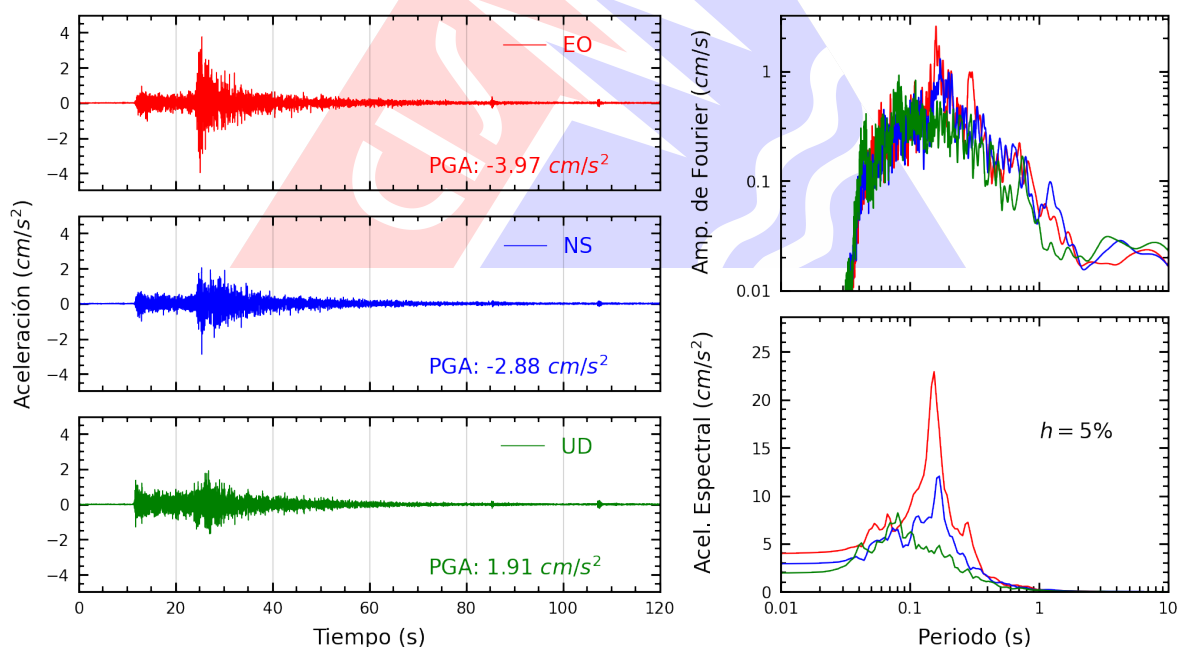
Figura A.14: Registros tiempo-historia, espectros de Fourier y de respuesta en las direcciones EO, NS y vertical de la estación PRADO. Sismo de Huacho, Huaura - Lima del 2026-09-24, 23:26:28 (Hora local)
