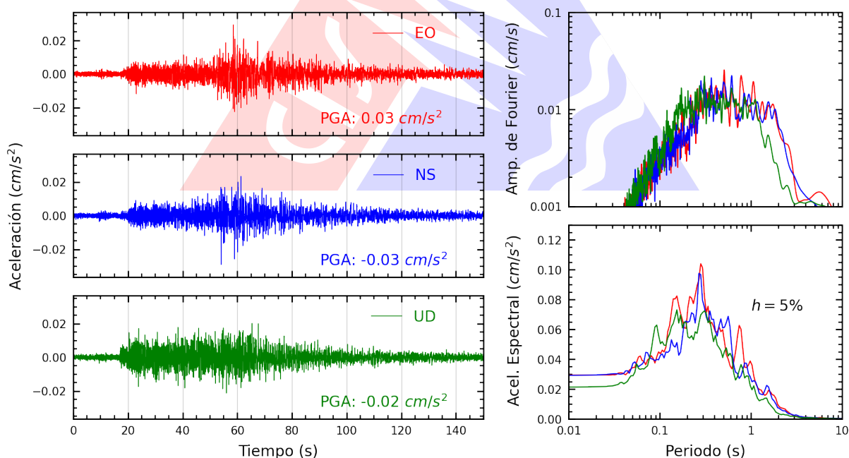
Figura A.46: Registros tiempo-historia, espectros de Fourier y de respuesta en las direcciones EO, NS y vertical de la estación UNCP. Sismo de Huacho, Huaura - Lima del 2026-09-24, 23:26:28 (Hora local)
