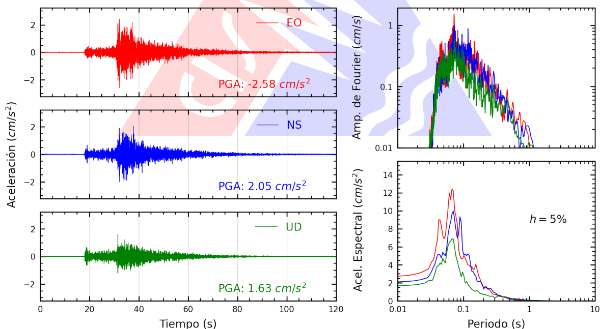
Figura A.26: Registros tiempo-historia, espectros de Fourier y de respuesta en las direcciones EO, NS y vertical de la estación ATARJ. Sismo de Huacho, Huaura - Lima del 2026-09-24, 23:26:28 (Hora local)
