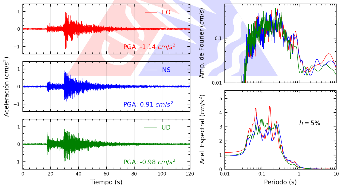
Figura A.40: Registros tiempo-historia, espectros de Fourier y de respuesta en las direcciones EO, NS y vertical de la estación BONDY. Sismo de Huacho, Huaura - Lima del 2026-09-24, 23:26:28 (Hora local)
