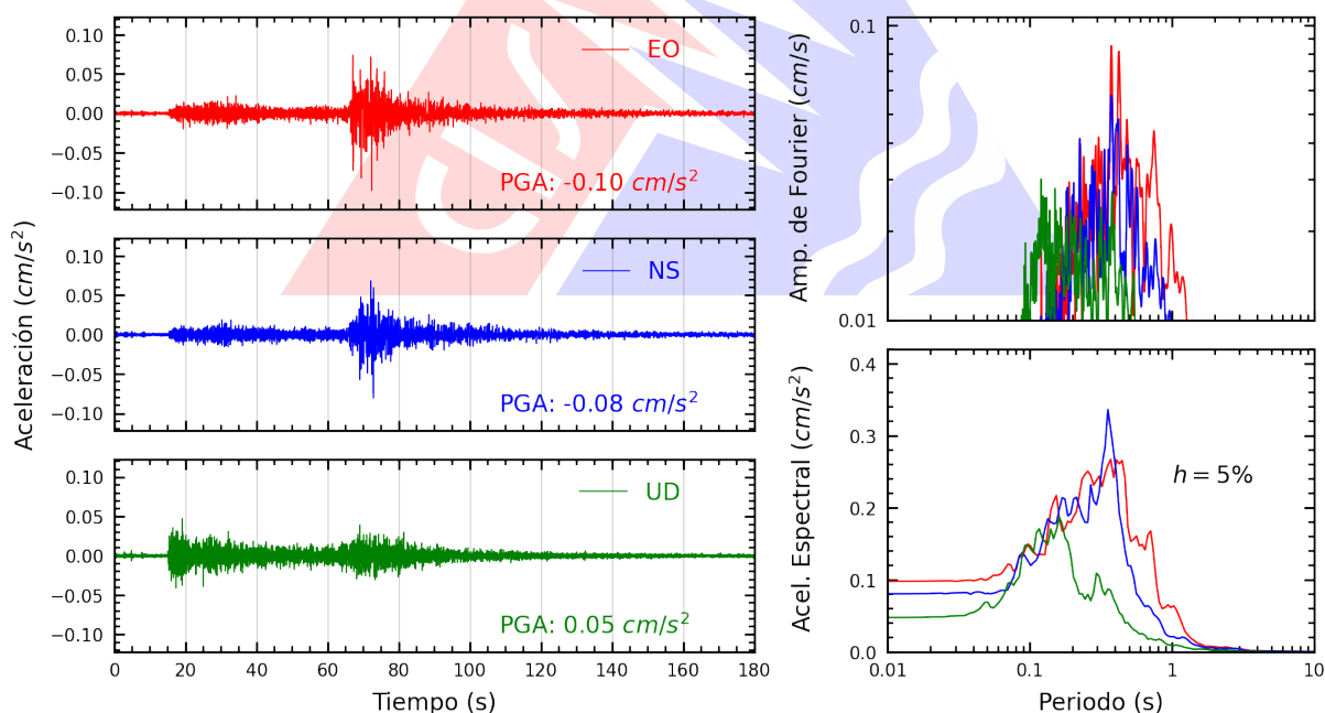
Figura A.44: Registros tiempo-historia, espectros de Fourier y de respuesta en las direcciones EO, NS y vertical de la estación UNIA. Sismo de Huacho, Huaura - Lima del 2026-09-24, 23:26:28 (Hora local)
