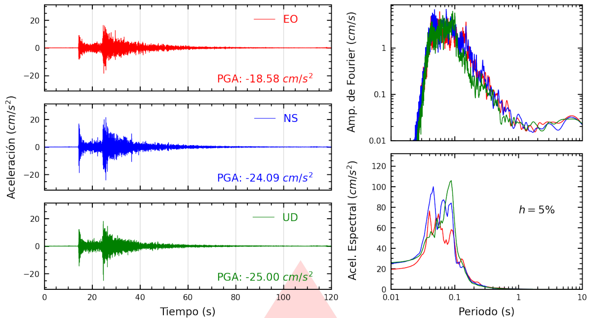
Figura A.1: Registros tiempo-historia, espectros de Fourier y de respuesta en las direcciones EO, NS y vertical de la estación SROSA. Sismo de Huacho, Huaura - Lima del 2026-09-24, 23:26:28 (Hora local)
