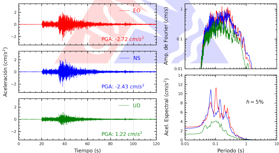
Figura A.24: Registros tiempo-historia, espectros de Fourier y de respuesta en las direcciones EO, NS y vertical de la estación BRISA. Sismo de Huacho, Huaura - Lima del 2026-09-24, 23:26:28 (Hora local)
