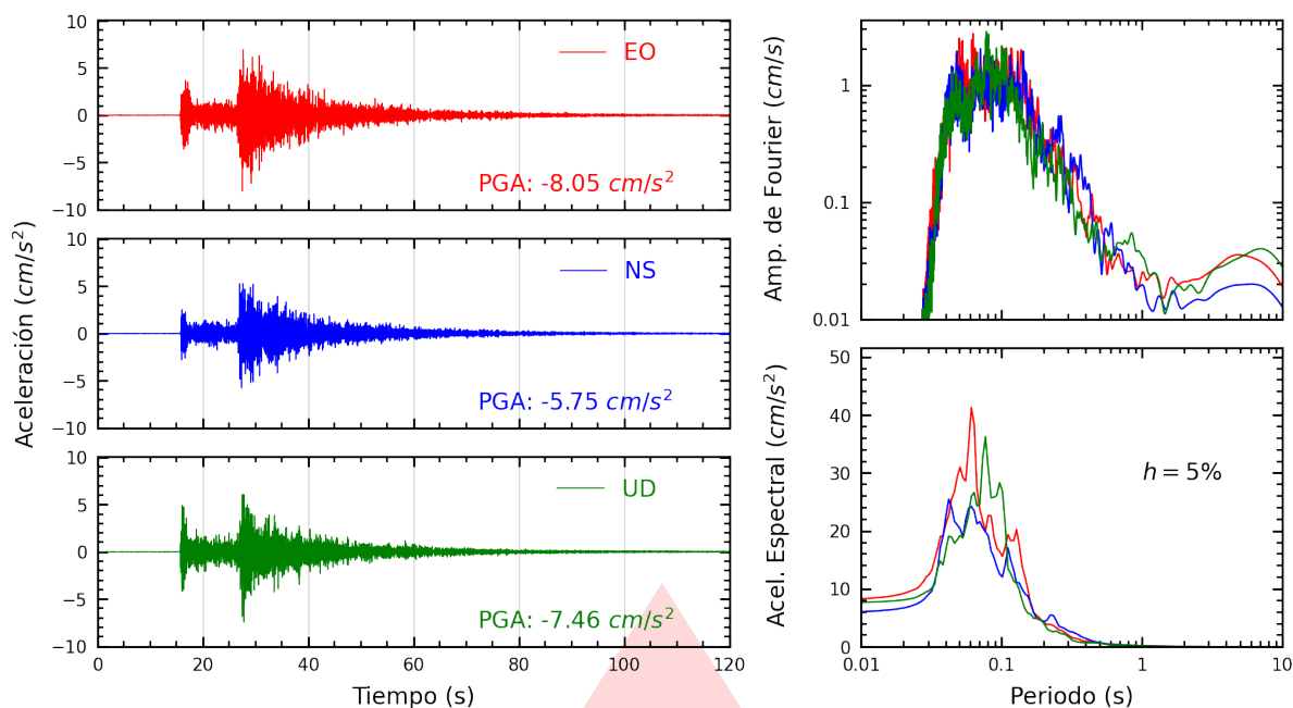
Figura A.5: Registros tiempo-historia, espectros de Fourier y de respuesta en las direcciones EO, NS y vertical de la estación AMORE. Sismo de Huacho, Huaura - Lima del 2026-09-24, 23:26:28 (Hora local)
