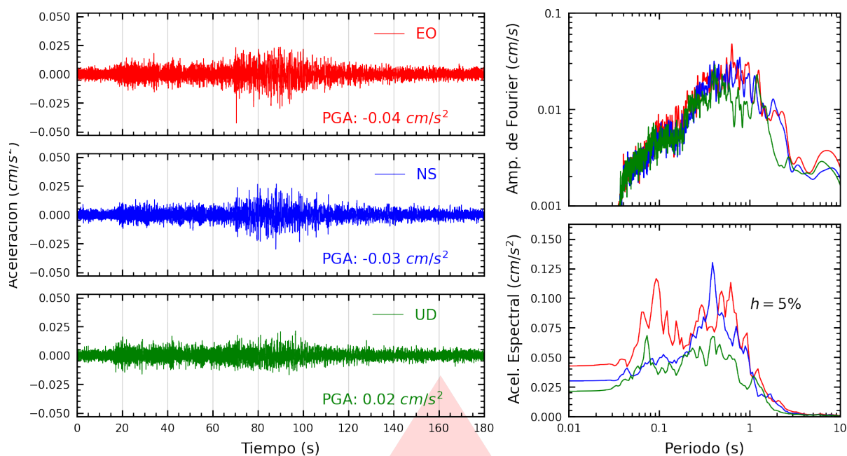
Figura A.45: Registros tiempo-historia, espectros de Fourier y de respuesta en las direcciones EO, NS y vertical de la estación UNC. Sismo de Huacho, Huaura - Lima del 2026-09-24, 23:26:28 (Hora local)
