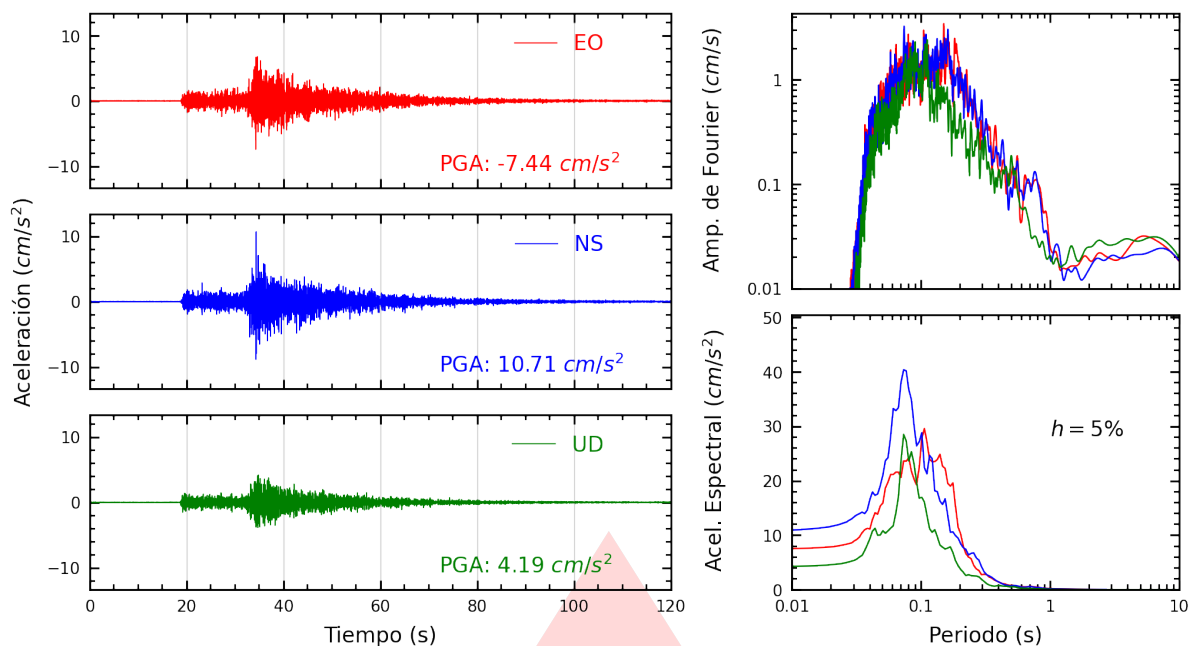
Figura A.3: Registros tiempo-historia, espectros de Fourier y de respuesta en las direcciones EO, NS y vertical de la estación USILM. Sismo de Huacho, Huaura - Lima del 2026-09-24, 23:26:28 (Hora local)
