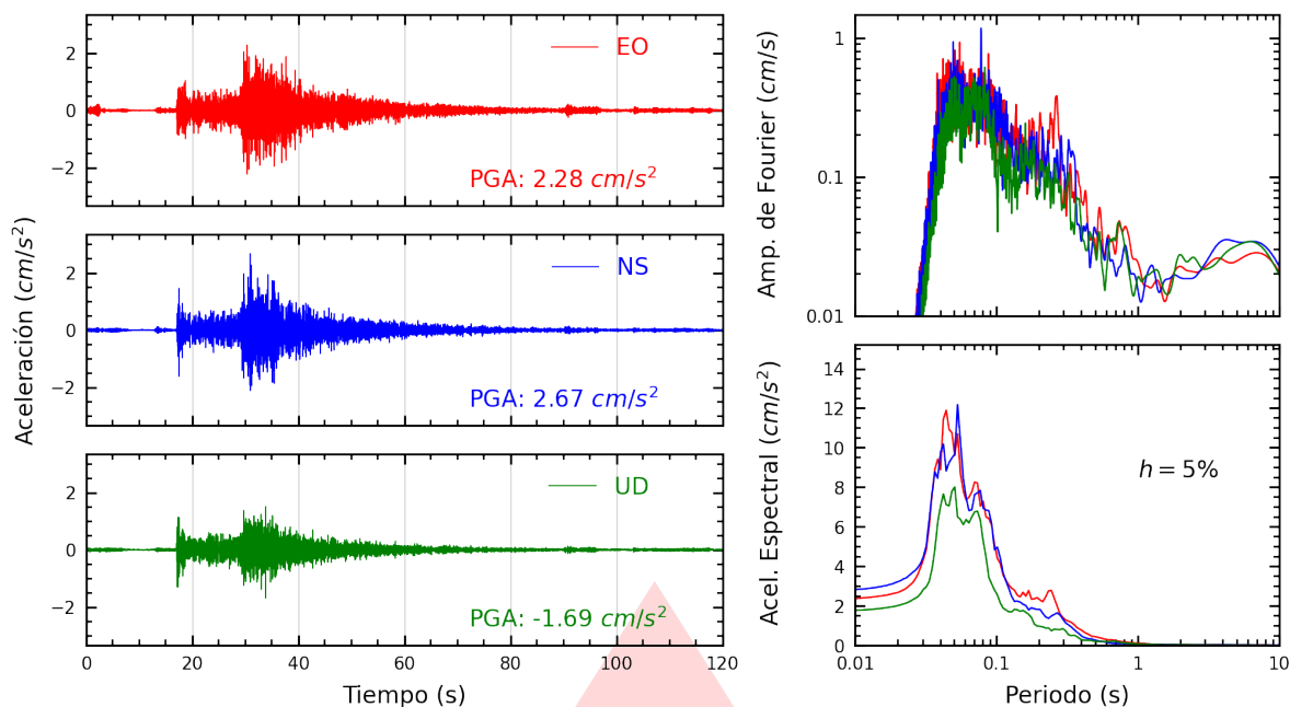
Figura A.25: Registros tiempo-historia, espectros de Fourier y de respuesta en las direcciones EO, NS y vertical de la estación UCSS. Sismo de Huacho, Huaura - Lima del 2026-09-24, 23:26:28 (Hora local)
