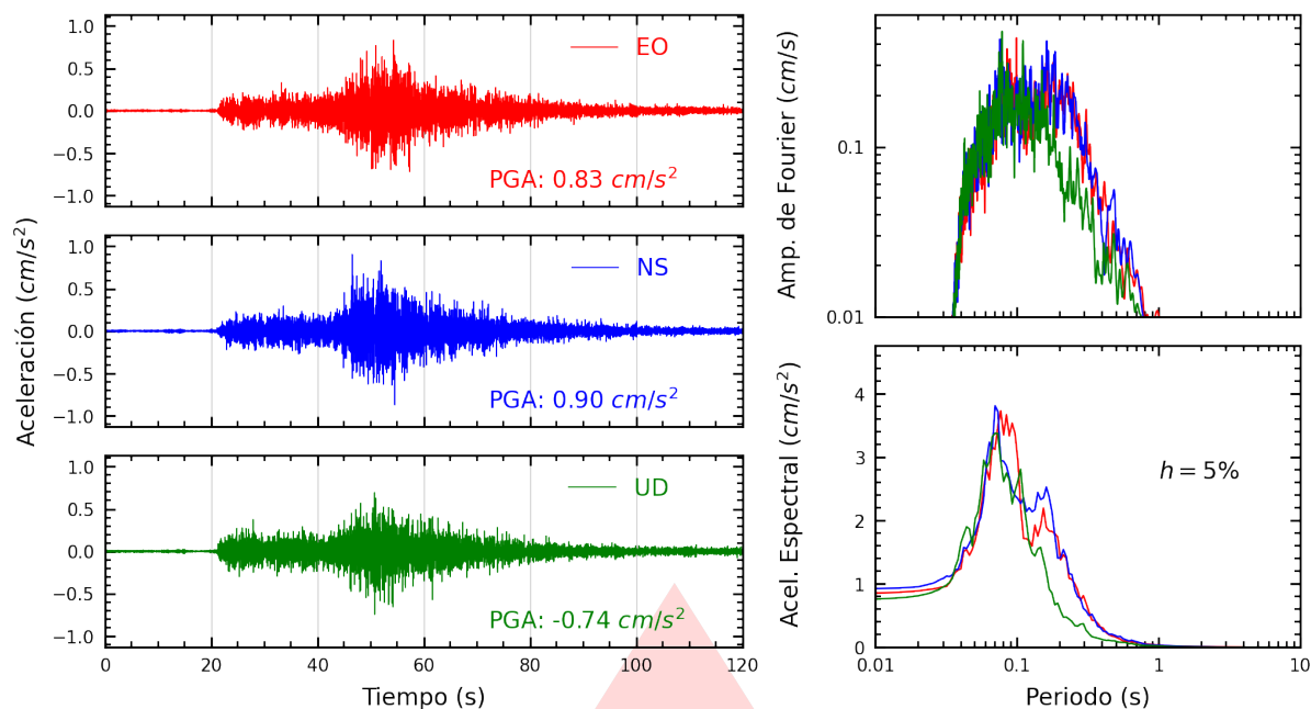
Figura A.41: Registros tiempo-historia, espectros de Fourier y de respuesta en las direcciones EO, NS y vertical de la estación ASIA. Sismo de Huacho, Huaura - Lima del 2026-09-24, 23:26:28 (Hora local)
