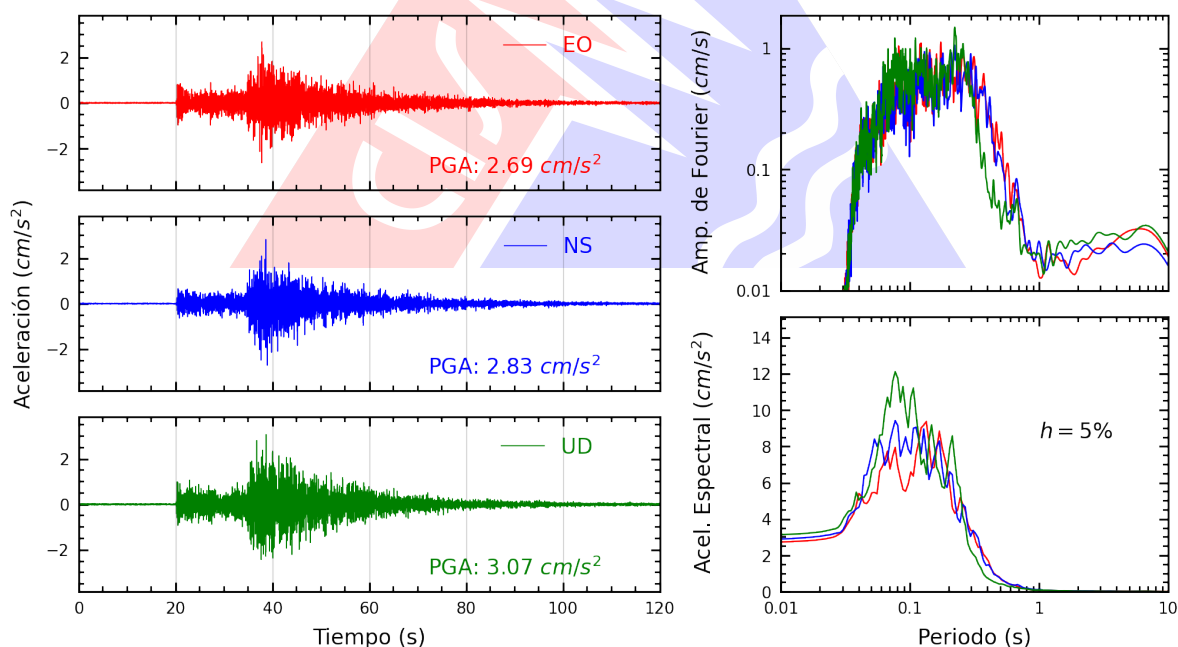
Figura A.20: Registros tiempo-historia, espectros de Fourier y de respuesta en las direcciones EO, NS y vertical de la estación SOVES. Sismo de Huacho, Huaura - Lima del 2026-09-24, 23:26:28 (Hora local)
