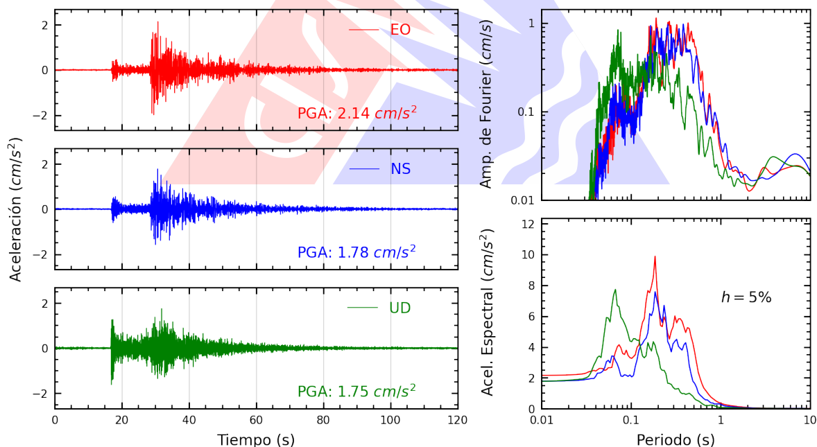
Figura A.30: Registros tiempo-historia, espectros de Fourier y de respuesta en las direcciones EO, NS y vertical de la estación ACAPU. Sismo de Huacho, Huaura - Lima del 2026-09-24, 23:26:28 (Hora local)
