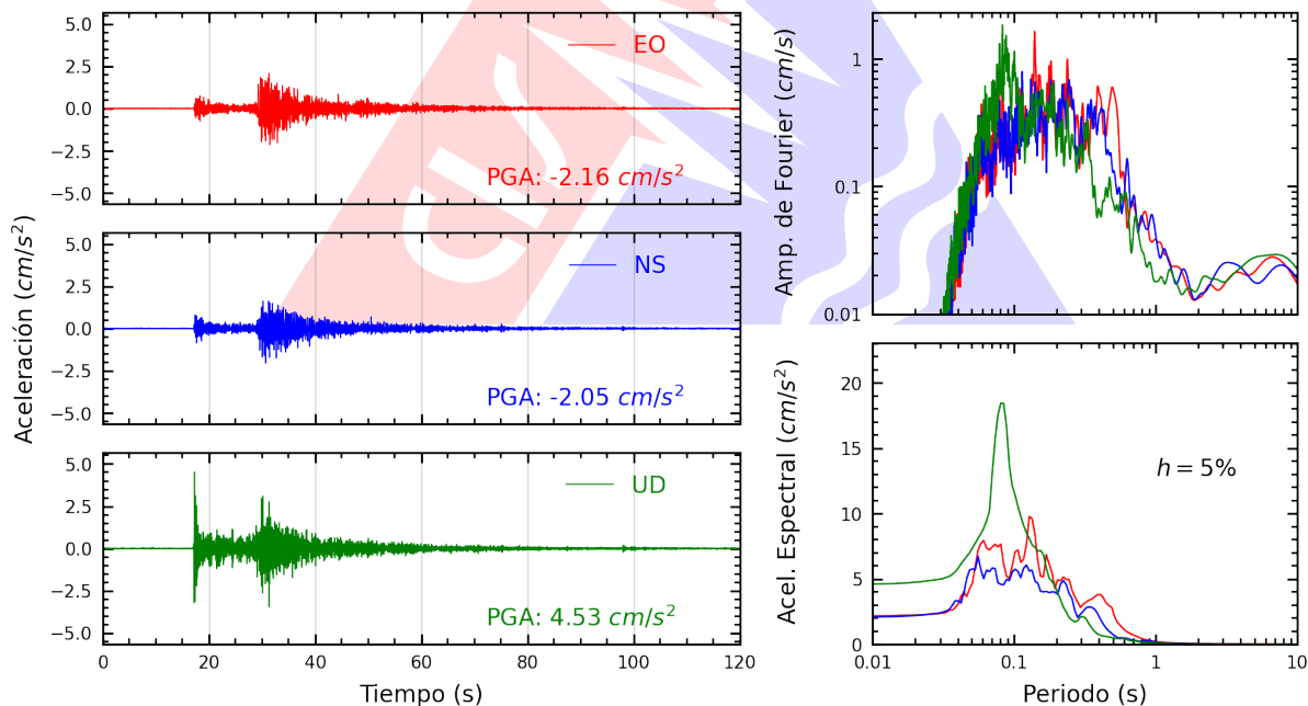
Figura A.10: Registros tiempo-historia, espectros de Fourier y de respuesta en las direcciones EO, NS y vertical de la estación RAMON. Sismo de Huacho, Huaura - Lima del 2026-09-24, 23:26:28 (Hora local)
