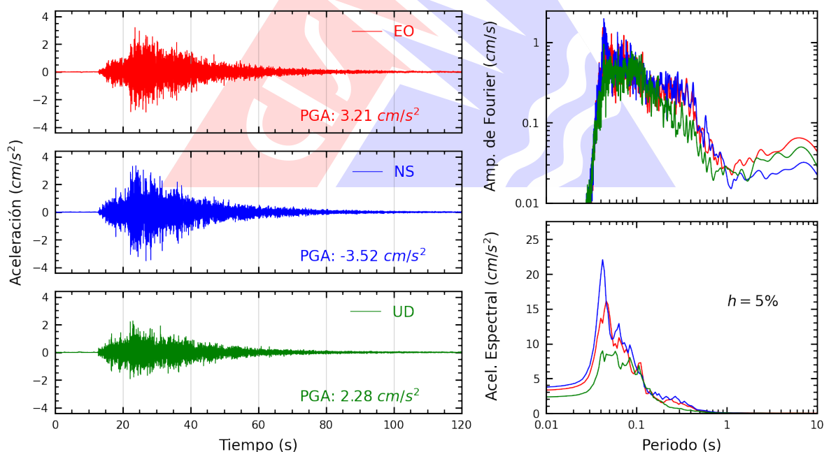
Figura A.16: Registros tiempo-historia, espectros de Fourier y de respuesta en las direcciones EO, NS y vertical de la estación UNAB. Sismo de Huacho, Huaura - Lima del 2026-09-24, 23:26:28 (Hora local)
