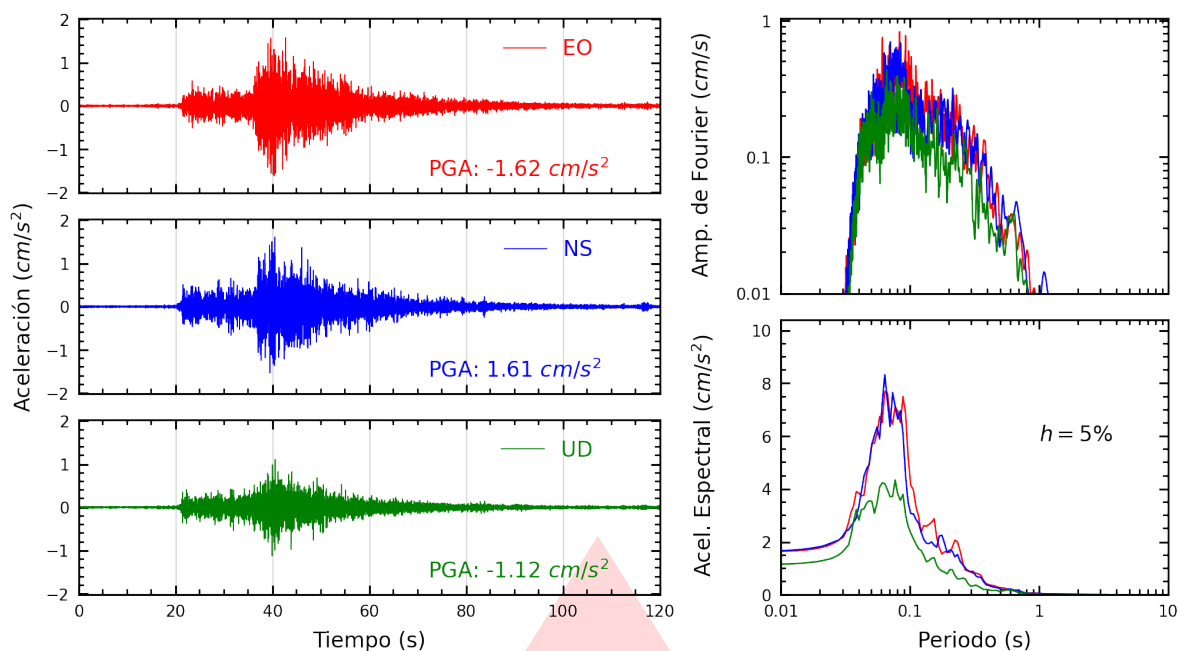
Figura A.35: Registros tiempo-historia, espectros de Fourier y de respuesta en las direcciones EO, NS y vertical de la estación PACHA. Sismo de Huacho, Huaura - Lima del 2026-09-24, 23:26:28 (Hora local)
