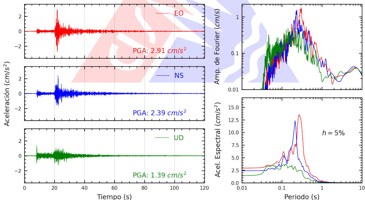
Figura A.22: Registros tiempo-historia, espectros de Fourier y de respuesta en las direcciones EO, NS y vertical de la estación DSMI. Sismo de Huacho, Huaura - Lima del 2026-09-24, 23:26:28 (Hora local)
