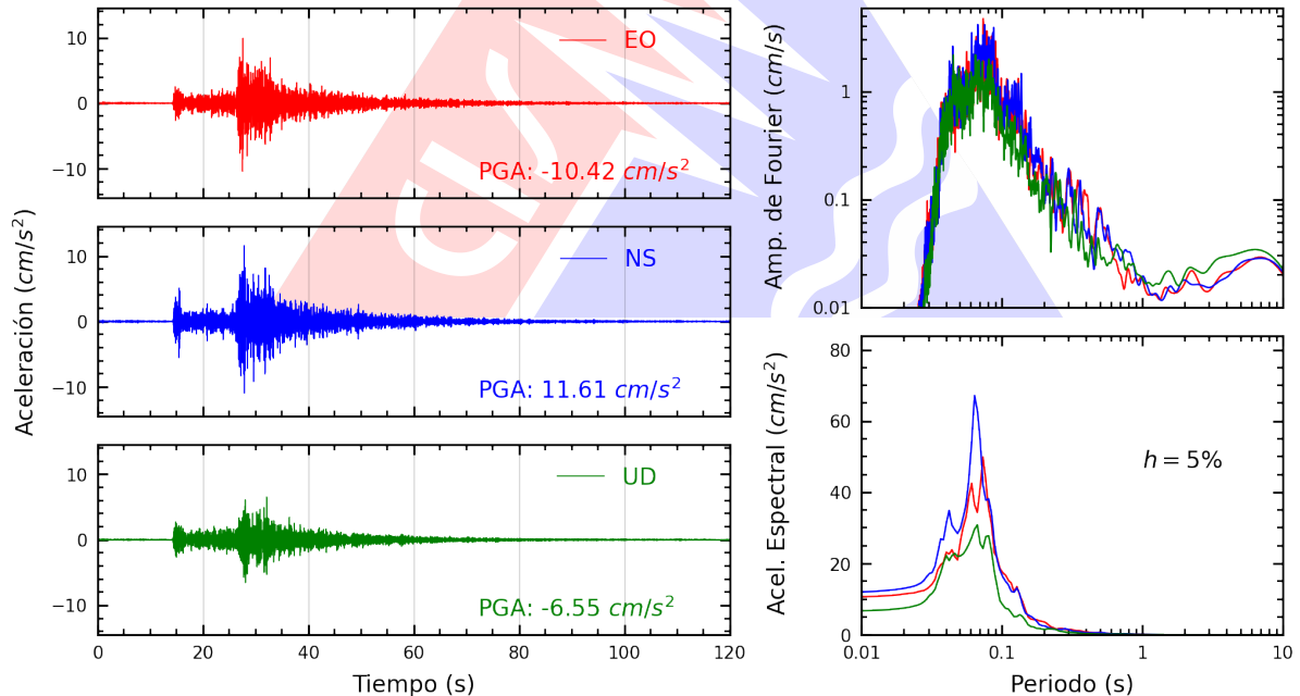
Figura A.2: Registros tiempo-historia, espectros de Fourier y de respuesta en las direcciones EO, NS y vertical de la estación JOSEO. Sismo de Huacho, Huaura - Lima del 2026-09-24, 23:26:28 (Hora local)
