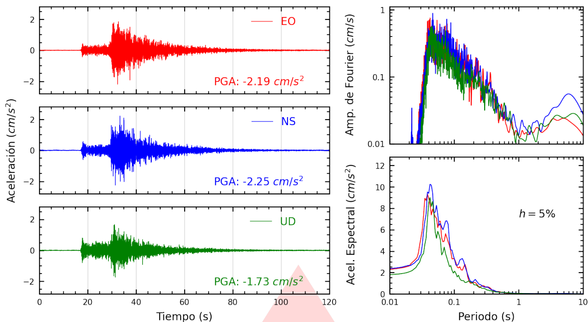
Figura A.29: Registros tiempo-historia, espectros de Fourier y de respuesta en las direcciones EO, NS y vertical de la estación SJLCE. Sismo de Huacho, Huaura - Lima del 2026-09-24, 23:26:28 (Hora local)
