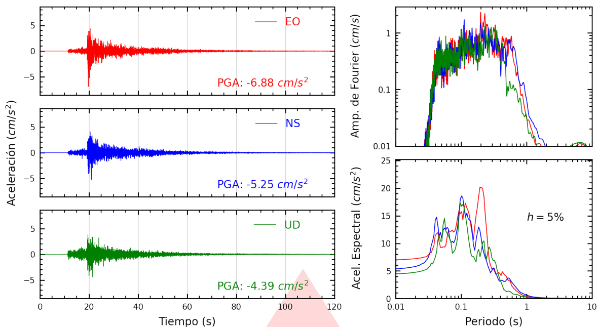
Figura A.7: Registros tiempo-historia, espectros de Fourier y de respuesta en las direcciones EO, NS y vertical de la estación CARAL. Sismo de Huacho, Huaura - Lima del 2026-09-24, 23:26:28 (Hora local)
