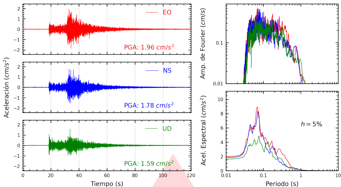
Figura A.31: Registros tiempo-historia, espectros de Fourier y de respuesta en las direcciones EO, NS y vertical de la estación BORJA. Sismo de Huacho, Huaura - Lima del 2026-09-24, 23:26:28 (Hora local)
