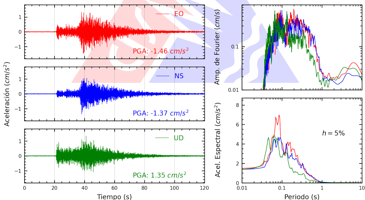
Figura A.38: Registros tiempo-historia, espectros de Fourier y de respuesta en las direcciones EO, NS y vertical de la estación USILP. Sismo de Huacho, Huaura - Lima del 2026-09-24, 23:26:28 (Hora local)
