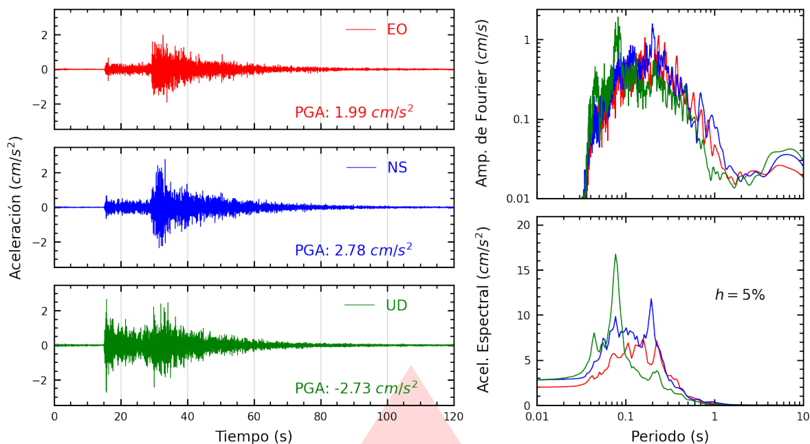
Figura A.23: Registros tiempo-historia, espectros de Fourier y de respuesta en las direcciones EO, NS y vertical de la estación SOCHO. Sismo de Huacho, Huaura - Lima del 2026-09-24, 23:26:28 (Hora local)
