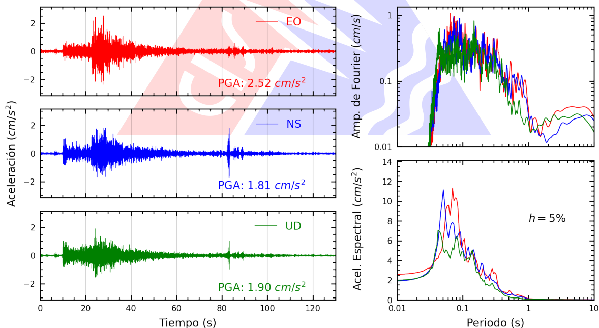
Figura A.28: Registros tiempo-historia, espectros de Fourier y de respuesta en las direcciones EO, NS y vertical de la estación UPCS. Sismo de Huacho, Huaura - Lima del 2026-09-24, 23:26:28 (Hora local)
