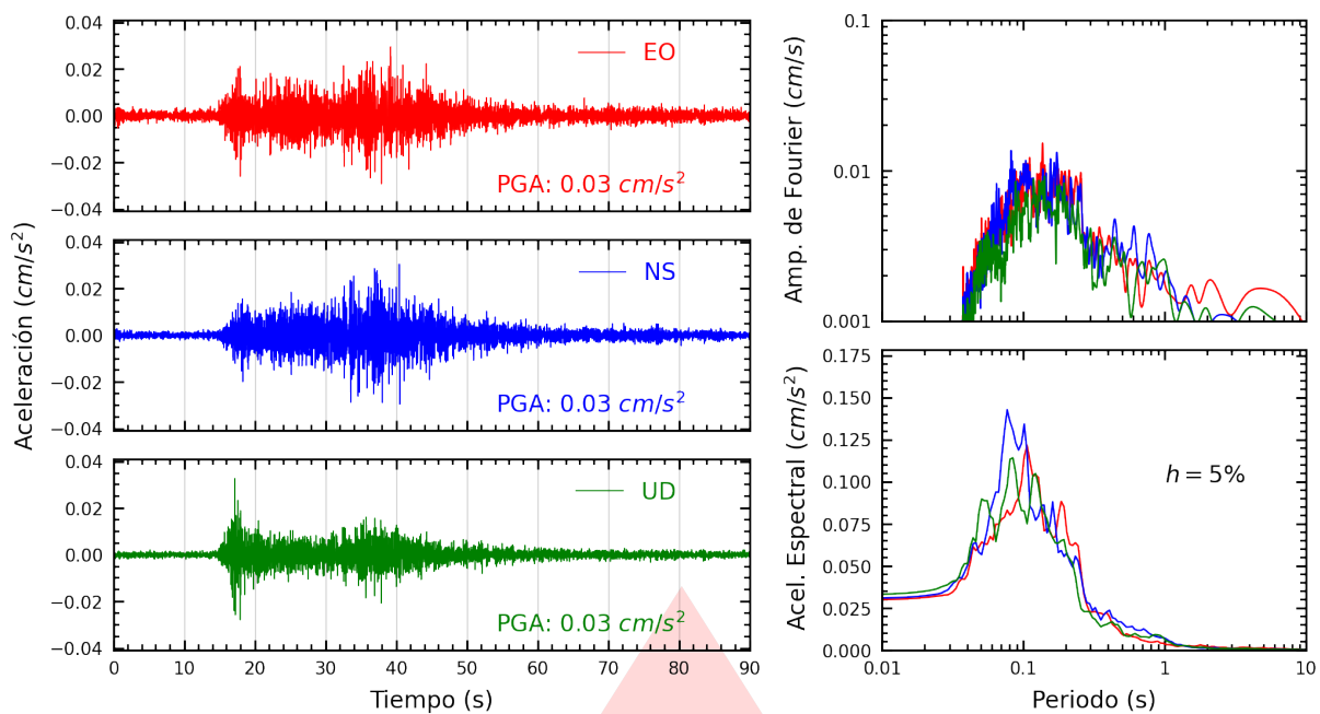
Figura A.1: Registros tiempo-historia, espectros de Fourier y de respuesta en las direcciones EO, NS y vertical de la estación UNSA2. Sismo de Cabanaconde, Caylloma - Arequipa del 2026-09-26, 16:44:41 (Hora local)
