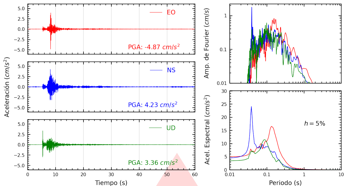
Figura A.1: Registros tiempo-historia, espectros de Fourier y de respuesta en las direcciones EO, NS y vertical de la estación UNJ. Sismo de Jaén, Jaén - Cajamarca del 2026-09-29, 13:01:39 (Hora local)
