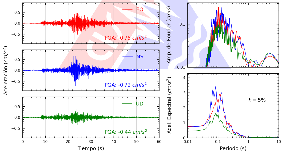
Figura A.2: Registros tiempo-historia, espectros de Fourier y de respuesta en las direcciones EO, NS y vertical de la estación UNTRM. Sismo de Jaén, Jaén - Cajamarca del 2026-09-29, 13:01:39 (Hora local)
