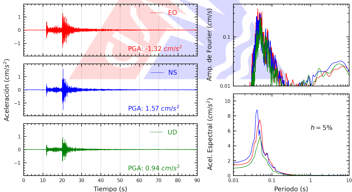
Figura A.12: Registros tiempo-historia, espectros de Fourier y de respuesta en las direcciones EO, NS y vertical de la estación UCSS. Sismo de Ancón, Lima - Lima del 2026-09-30, 03:52:59 (Hora local)
