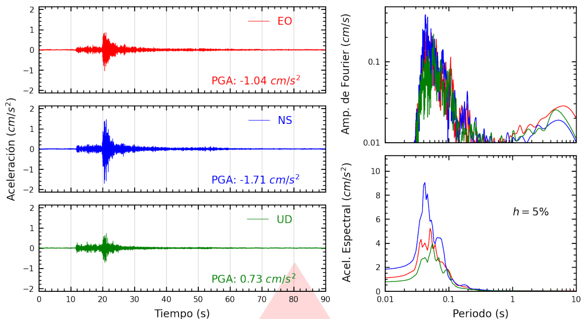
Figura A.9: Registros tiempo-historia, espectros de Fourier y de respuesta en las direcciones EO, NS y vertical de la estación COMAS. Sismo de Ancón, Lima - Lima del 2026-09-30, 03:52:59 (Hora local)
