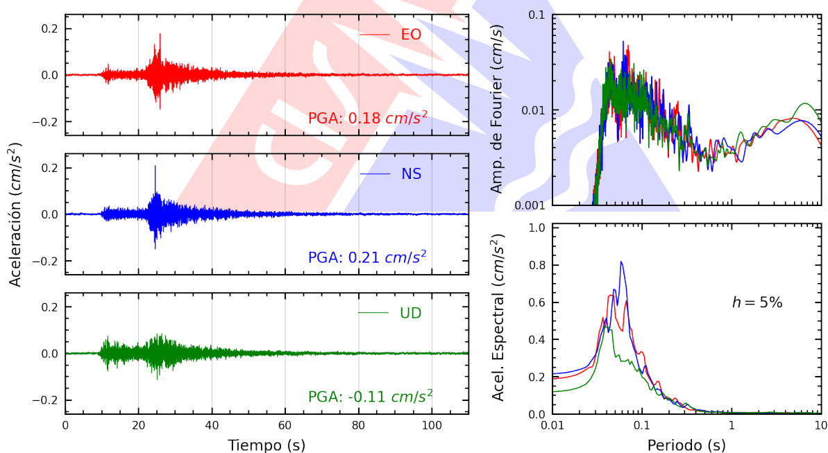
Figura A.34: Registros tiempo-historia, espectros de Fourier y de respuesta en las direcciones EO, NS y vertical de la estación CARAL. Sismo de Ancón, Lima - Lima del 2026-09-30, 03:52:59 (Hora local)
