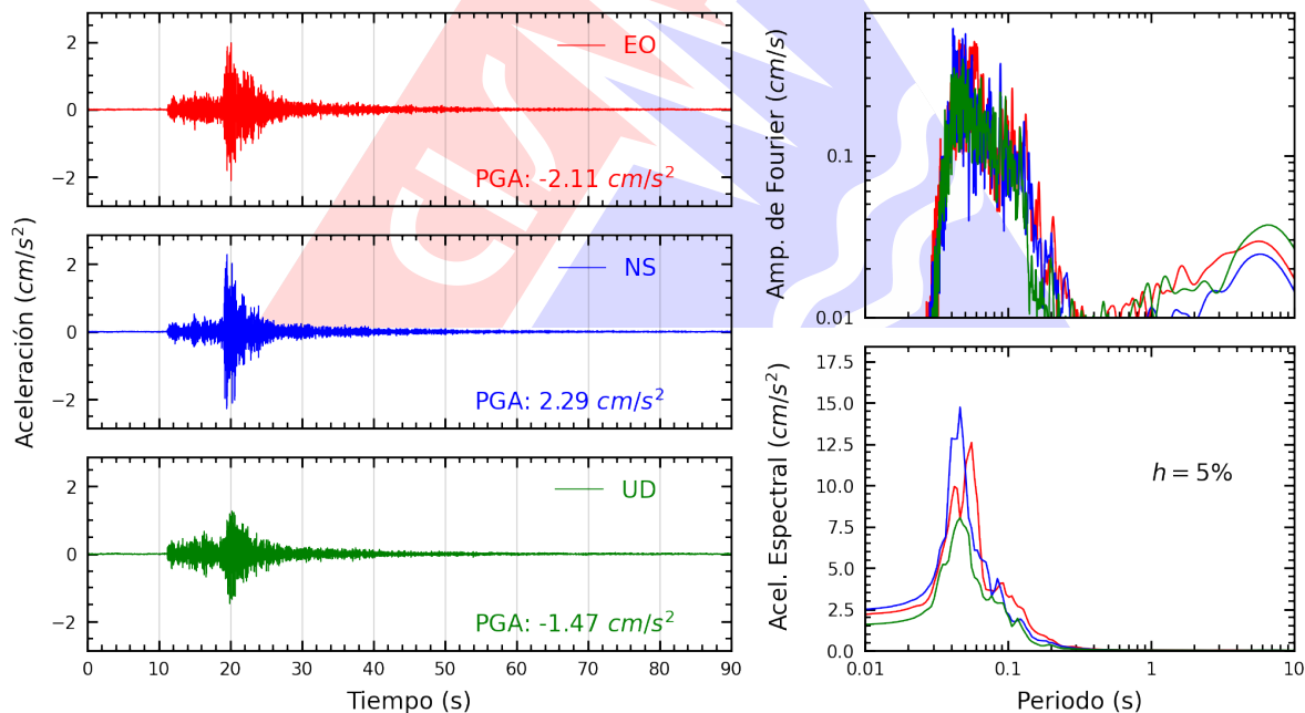
Figura A.6: Registros tiempo-historia, espectros de Fourier y de respuesta en las direcciones EO, NS y vertical de la estación AMORE. Sismo de Ancón, Lima - Lima del 2026-09-30, 03:52:59 (Hora local)
