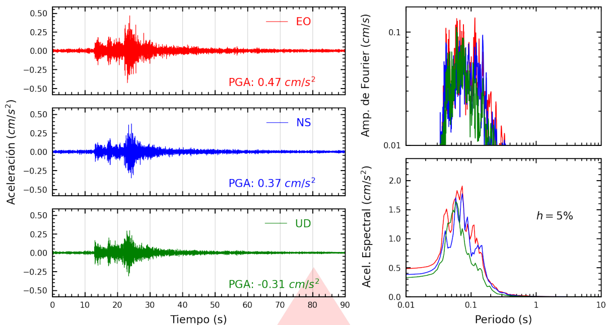
Figura A.27: Registros tiempo-historia, espectros de Fourier y de respuesta en las direcciones EO, NS y vertical de la estación SOBAR. Sismo de Ancón, Lima - Lima del 2026-09-30, 03:52:59 (Hora local)
