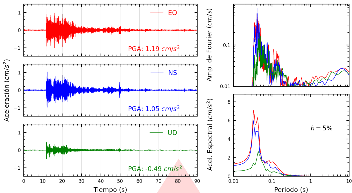
Figura A.17: Registros tiempo-historia, espectros de Fourier y de respuesta en las direcciones EO, NS y vertical de la estación DHNPE. Sismo de Ancón, Lima - Lima del 2026-09-30, 03:52:59 (Hora local)
