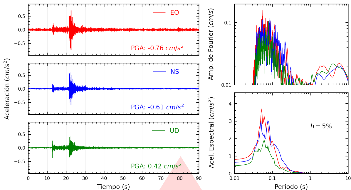
Figura A.23: Registros tiempo-historia, espectros de Fourier y de respuesta en las direcciones EO, NS y vertical de la estación INICT. Sismo de Ancón, Lima - Lima del 2026-09-30, 03:52:59 (Hora local)
