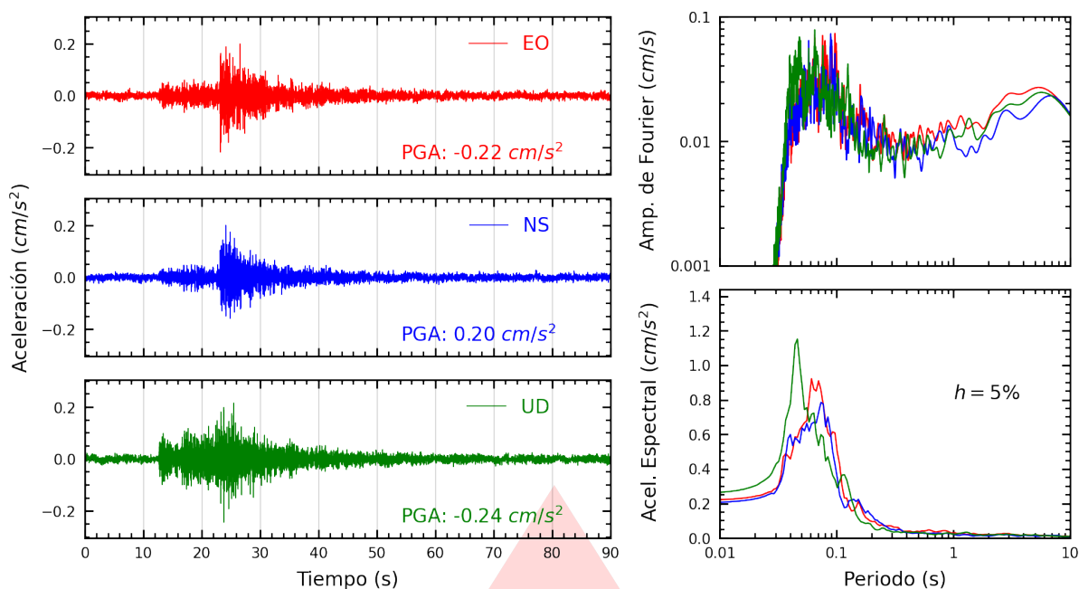
Figura A.33: Registros tiempo-historia, espectros de Fourier y de respuesta en las direcciones EO, NS y vertical de la estación USILP. Sismo de Ancón, Lima - Lima del 2026-09-30, 03:52:59 (Hora local)
