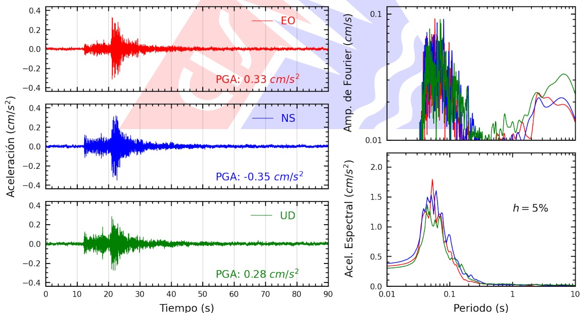
Figura A.30: Registros tiempo-historia, espectros de Fourier y de respuesta en las direcciones EO, NS y vertical de la estación UNFV. Sismo de Ancón, Lima - Lima del 2026-09-30, 03:52:59 (Hora local)
