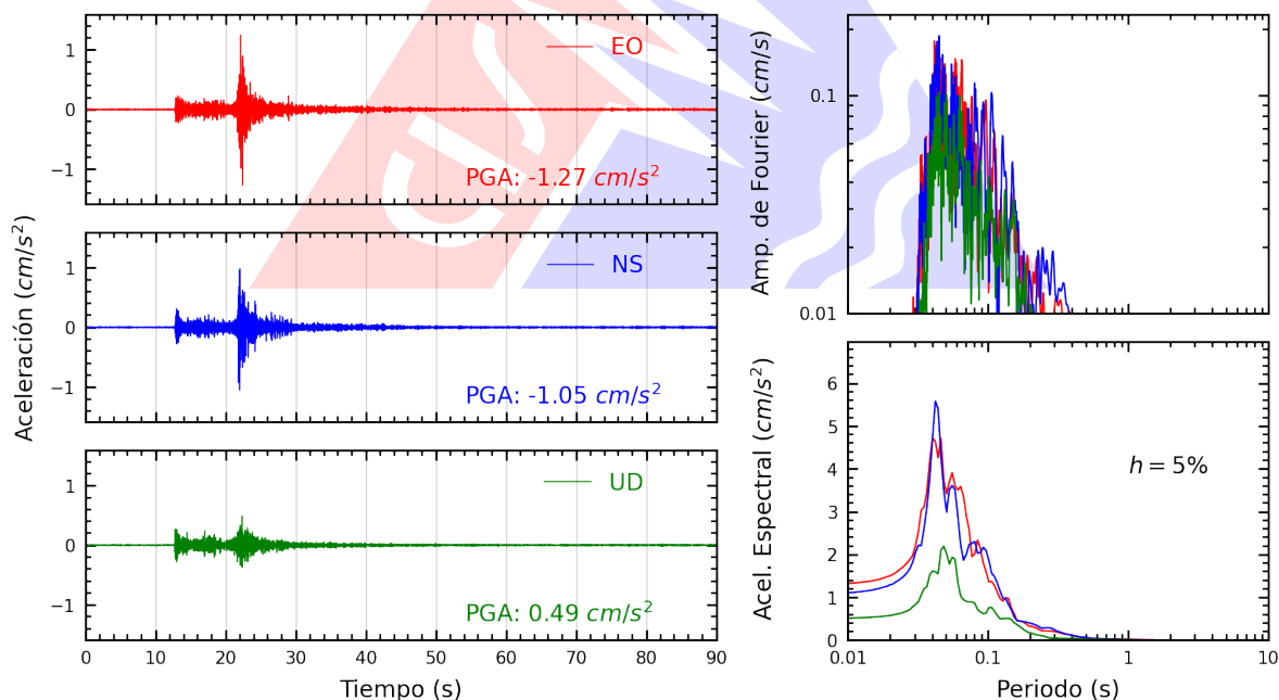
Figura A.16: Registros tiempo-historia, espectros de Fourier y de respuesta en las direcciones EO, NS y vertical de la estación BORJA. Sismo de Ancón, Lima - Lima del 2026-09-30, 03:52:59 (Hora local)
