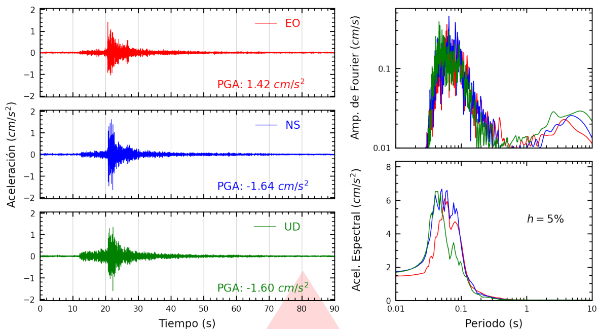
Figura A.11: Registros tiempo-historia, espectros de Fourier y de respuesta en las direcciones EO, NS y vertical de la estación SJLSC. Sismo de Ancón, Lima - Lima del 2026-09-30, 03:52:59 (Hora local)
