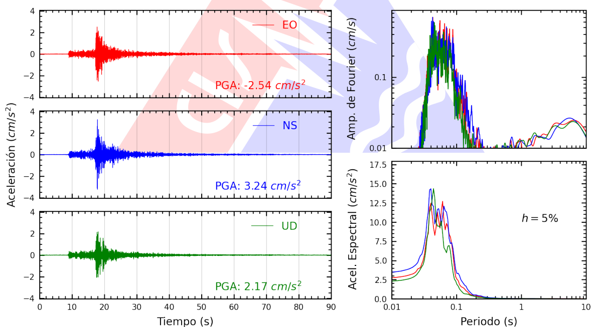
Figura A.2: Registros tiempo-historia, espectros de Fourier y de respuesta en las direcciones EO, NS y vertical de la estación JOSEO. Sismo de Ancón, Lima - Lima del 2026-09-30, 03:52:59 (Hora local)
