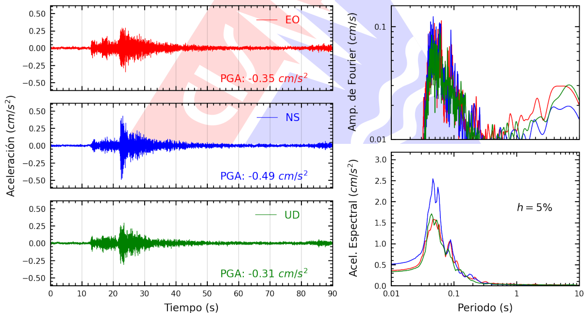
Figura A.24: Registros tiempo-historia, espectros de Fourier y de respuesta en las direcciones EO, NS y vertical de la estación IMCA. Sismo de Ancón, Lima - Lima del 2026-09-30, 03:52:59 (Hora local)
