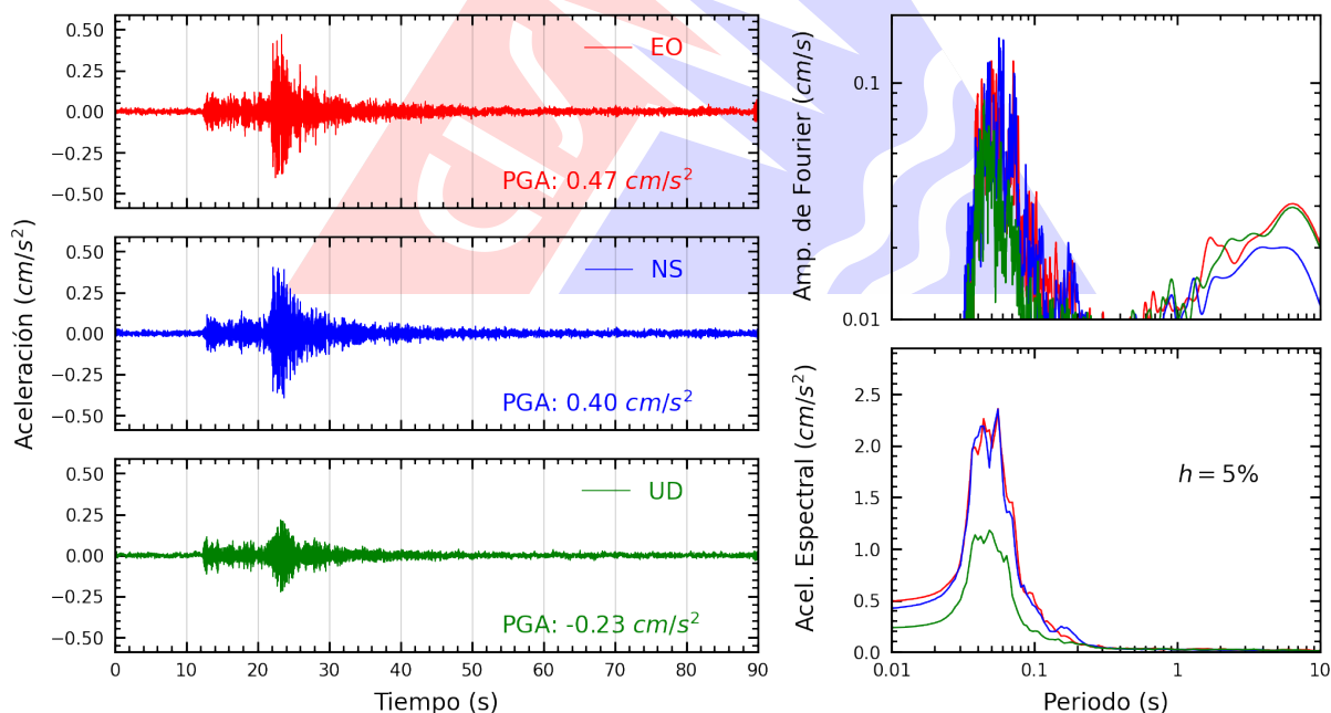
Figura A.26: Registros tiempo-historia, espectros de Fourier y de respuesta en las direcciones EO, NS y vertical de la estación UPCVI. Sismo de Ancón, Lima - Lima del 2026-09-30, 03:52:59 (Hora local)
