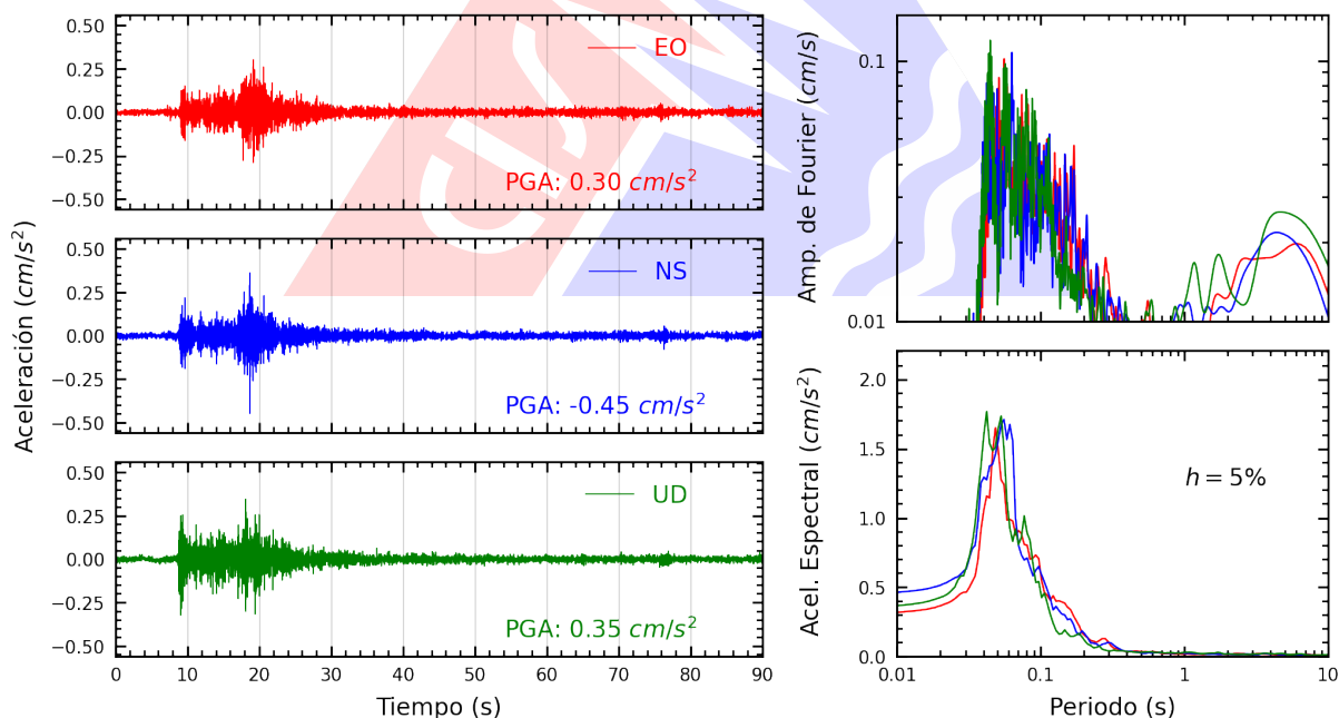
Figura A.28: Registros tiempo-historia, espectros de Fourier y de respuesta en las direcciones EO, NS y vertical de la estación PRADO. Sismo de Ancón, Lima - Lima del 2026-09-30, 03:52:59 (Hora local)
