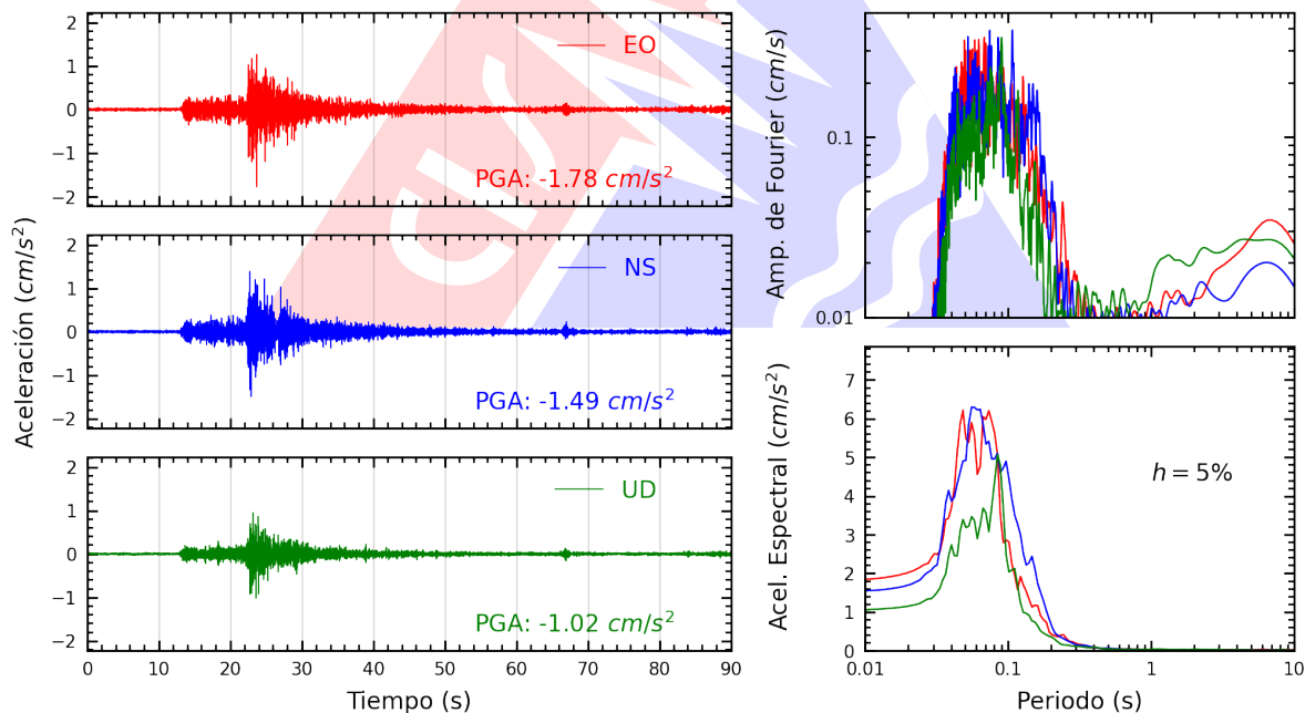
Figura A.8: Registros tiempo-historia, espectros de Fourier y de respuesta en las direcciones EO, NS y vertical de la estación USILM. Sismo de Ancón, Lima - Lima del 2026-09-30, 03:52:59 (Hora local)
