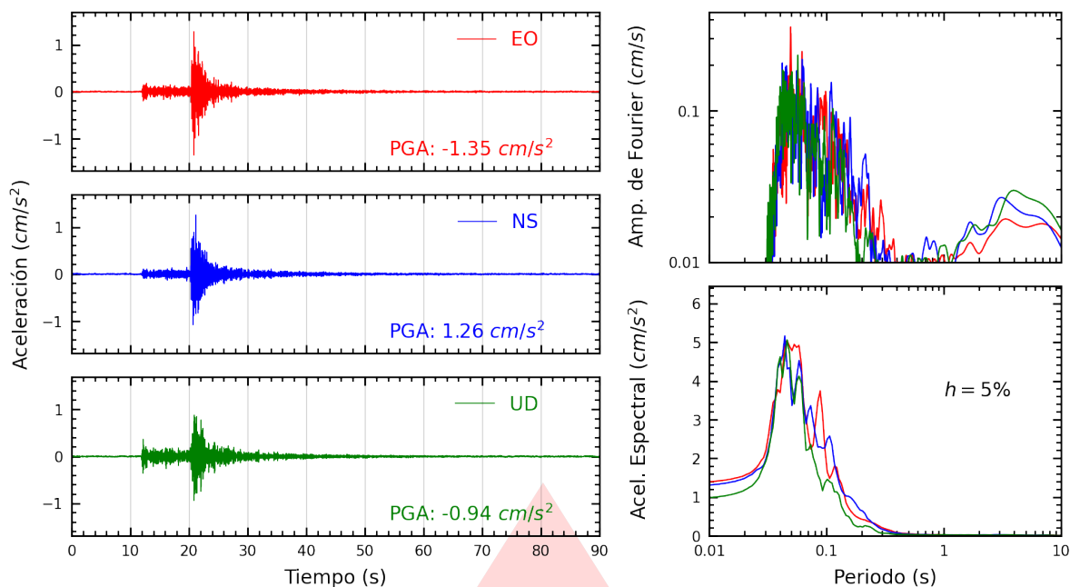
Figura A.15: Registros tiempo-historia, espectros de Fourier y de respuesta en las direcciones EO, NS y vertical de la estación JALVA. Sismo de Ancón, Lima - Lima del 2026-09-30, 03:52:59 (Hora local)
