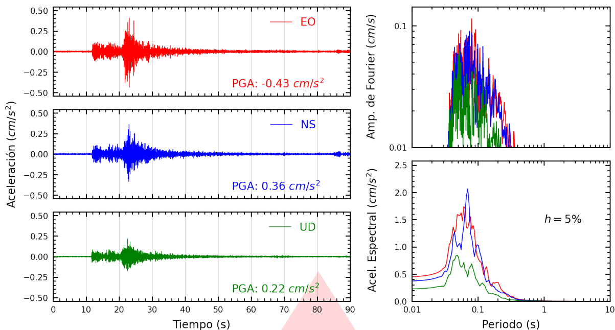
Figura A.29: Registros tiempo-historia, espectros de Fourier y de respuesta en las direcciones EO, NS y vertical de la estación BRISA. Sismo de Ancón, Lima - Lima del 2026-09-30, 03:52:59 (Hora local)
