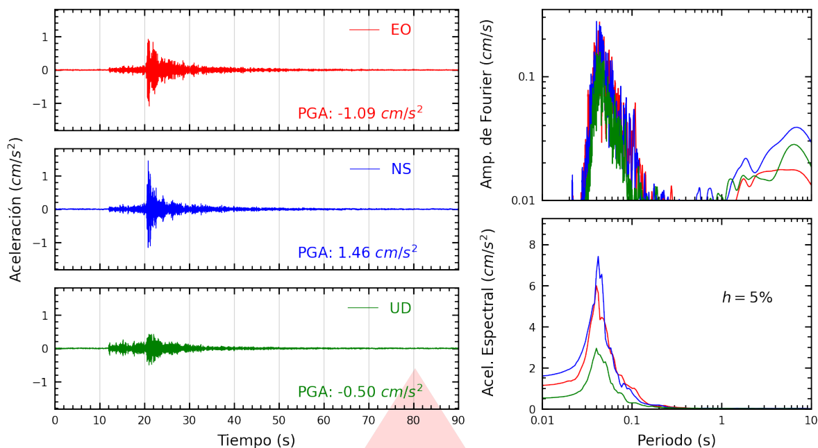
Figura A.13: Registros tiempo-historia, espectros de Fourier y de respuesta en las direcciones EO, NS y vertical de la estación SJLCE. Sismo de Ancón, Lima - Lima del 2026-09-30, 03:52:59 (Hora local)
