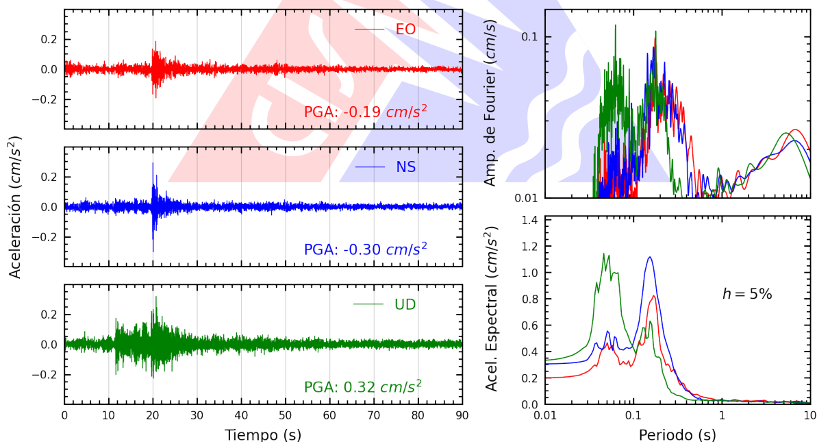
Figura A.32: Registros tiempo-historia, espectros de Fourier y de respuesta en las direcciones EO, NS y vertical de la estación ACAPU. Sismo de Ancón, Lima - Lima del 2026-09-30, 03:52:59 (Hora local)
