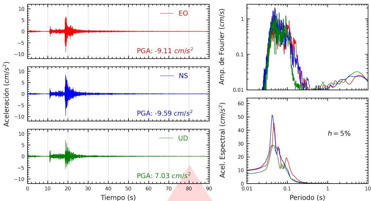
Figura A.1: Registros tiempo-historia, espectros de Fourier y de respuesta en las direcciones EO, NS y vertical de la estación SROSA. Sismo de Ancón, Lima - Lima del 2026-09-30, 03:52:59 (Hora local)
