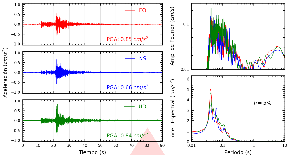
Figura A.21: Registros tiempo-historia, espectros de Fourier y de respuesta en las direcciones EO, NS y vertical de la estación SOVES. Sismo de Ancón, Lima - Lima del 2026-09-30, 03:52:59 (Hora local)
