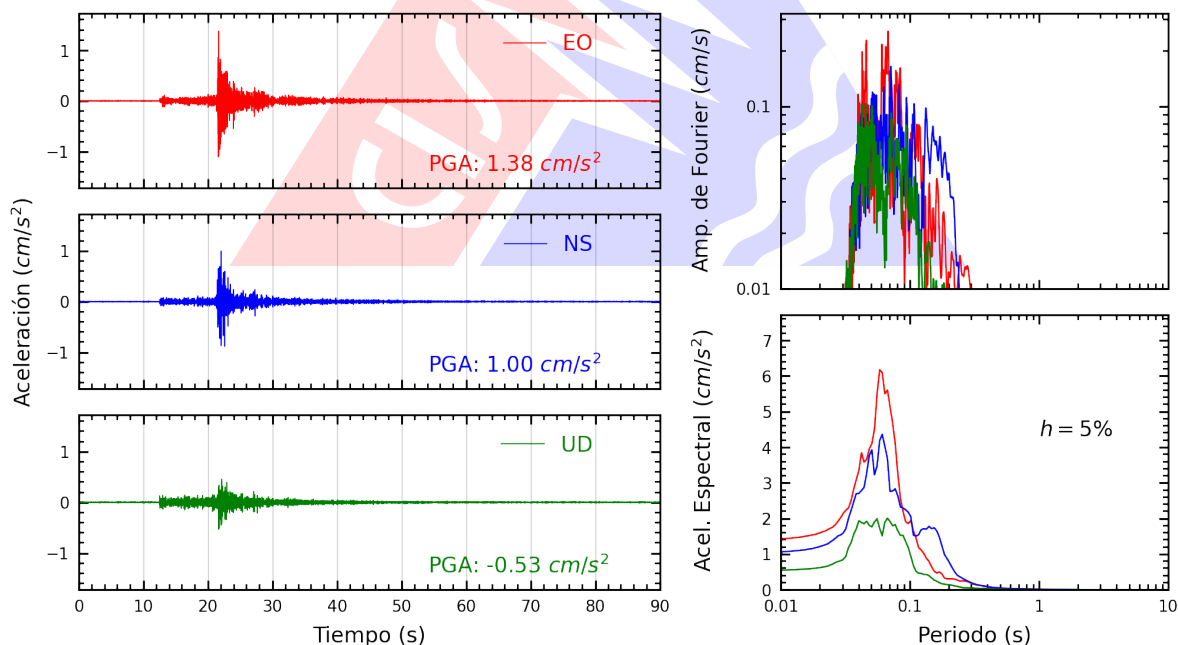
Figura A.14: Registros tiempo-historia, espectros de Fourier y de respuesta en las direcciones EO, NS y vertical de la estación ATARJ. Sismo de Ancón, Lima - Lima del 2026-09-30, 03:52:59 (Hora local)
