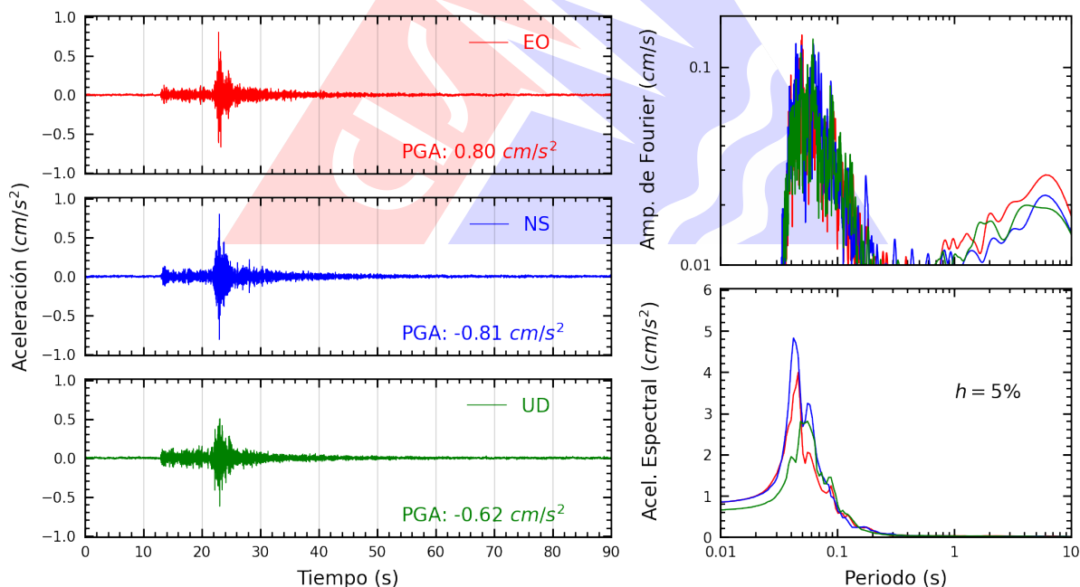
Figura A.22: Registros tiempo-historia, espectros de Fourier y de respuesta en las direcciones EO, NS y vertical de la estación SERVI. Sismo de Ancón, Lima - Lima del 2026-09-30, 03:52:59 (Hora local)
