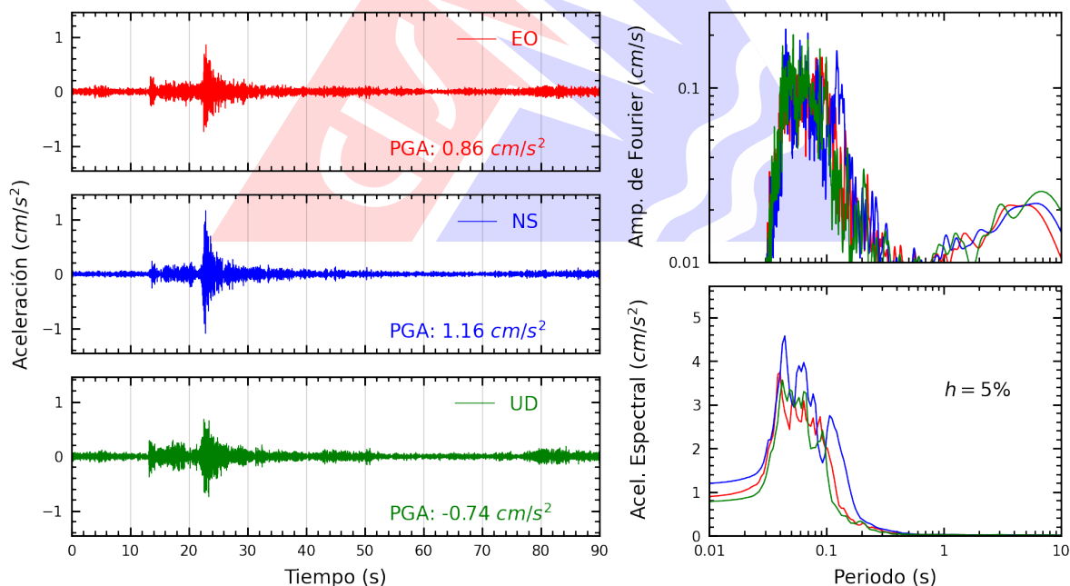
Figura A.18: Registros tiempo-historia, espectros de Fourier y de respuesta en las direcciones EO, NS y vertical de la estación URPPE. Sismo de Ancón, Lima - Lima del 2026-09-30, 03:52:59 (Hora local)
