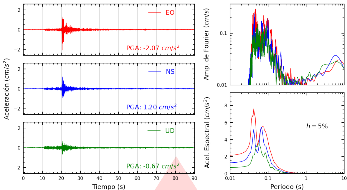
Figura A.7: Registros tiempo-historia, espectros de Fourier y de respuesta en las direcciones EO, NS y vertical de la estación UCVAT. Sismo de Ancón, Lima - Lima del 2026-09-30, 03:52:59 (Hora local)
