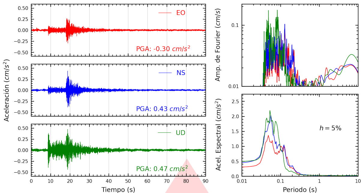
Figura A.25: Registros tiempo-historia, espectros de Fourier y de respuesta en las direcciones EO, NS y vertical de la estación SOCHO. Sismo de Ancón, Lima - Lima del 2026-09-30, 03:52:59 (Hora local)
