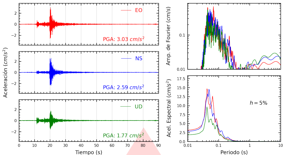
Figura A.3: Registros tiempo-historia, espectros de Fourier y de respuesta en las direcciones EO, NS y vertical de la estación INDEP. Sismo de Ancón, Lima - Lima del 2026-09-30, 03:52:59 (Hora local)
