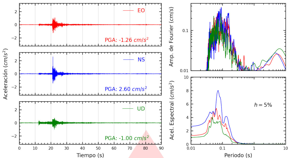
Figura A.5: Registros tiempo-historia, espectros de Fourier y de respuesta en las direcciones EO, NS y vertical de la estación SJLSV. Sismo de Ancón, Lima - Lima del 2026-09-30, 03:52:59 (Hora local)
