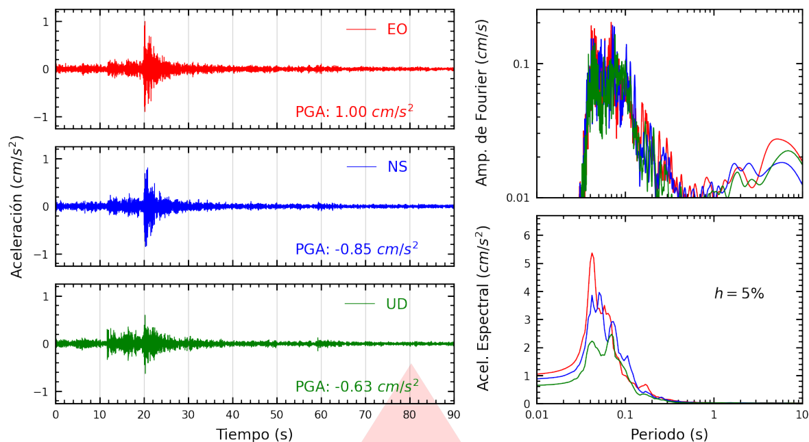
Figura A.19: Registros tiempo-historia, espectros de Fourier y de respuesta en las direcciones EO, NS y vertical de la estación MADRE. Sismo de Ancón, Lima - Lima del 2026-09-30, 03:52:59 (Hora local)
