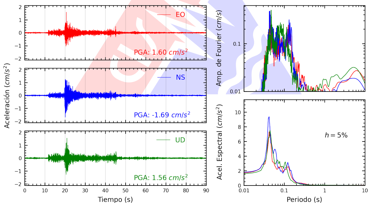
Figura A.10: Registros tiempo-historia, espectros de Fourier y de respuesta en las direcciones EO, NS y vertical de la estación CARAB. Sismo de Ancón, Lima - Lima del 2026-09-30, 03:52:59 (Hora local)
