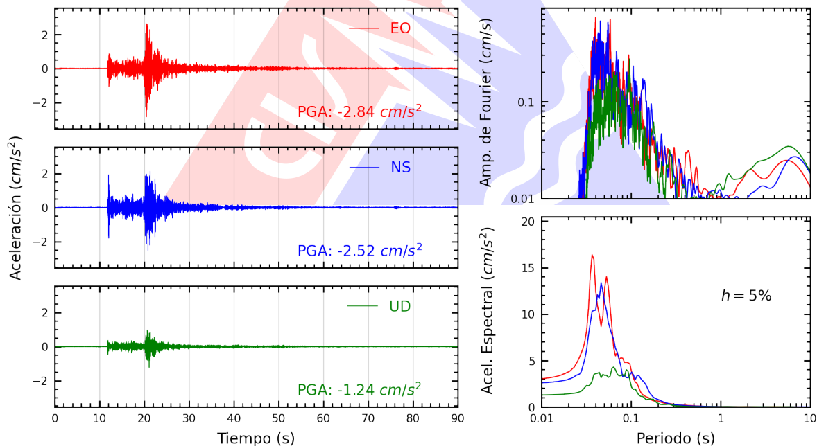
Figura A.4: Registros tiempo-historia, espectros de Fourier y de respuesta en las direcciones EO, NS y vertical de la estación OLIVO. Sismo de Ancón, Lima - Lima del 2026-09-30, 03:52:59 (Hora local)
