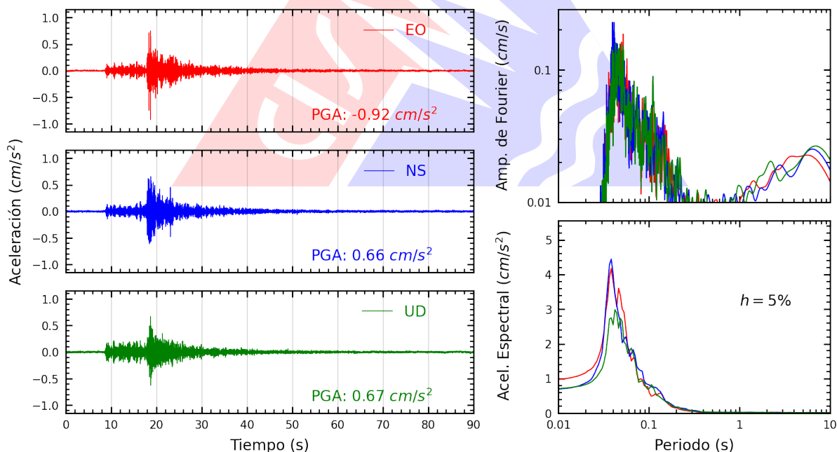
Figura A.20: Registros tiempo-historia, espectros de Fourier y de respuesta en las direcciones EO, NS y vertical de la estación USMP. Sismo de Ancón, Lima - Lima del 2026-09-30, 03:52:59 (Hora local)
