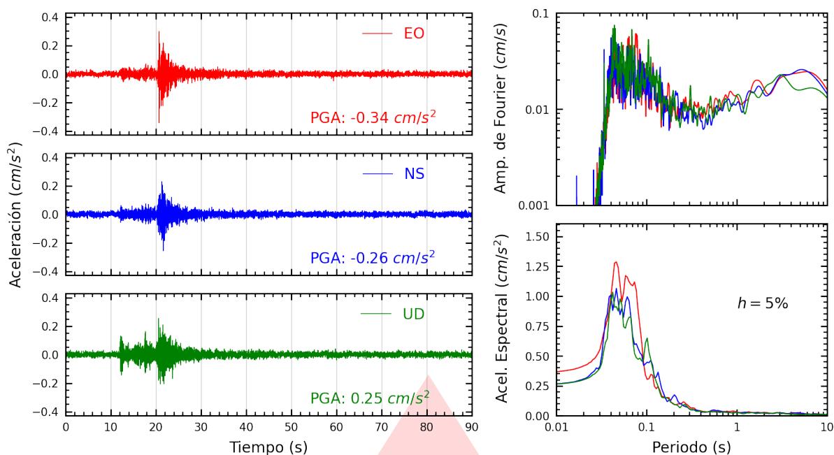
Figura A.31: Registros tiempo-historia, espectros de Fourier y de respuesta en las direcciones EO, NS y vertical de la estación BONDY. Sismo de Ancón, Lima - Lima del 2026-09-30, 03:52:59 (Hora local)
