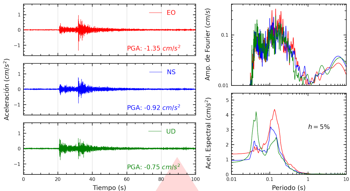
Figura A.13: Registros tiempo-historia, espectros de Fourier y de respuesta en las direcciones EO, NS y vertical de la estación USMP. Sismo de Callao, Provincia Constitucional del Callao del 2026-09-30, 11:12:38 (Hora local)
