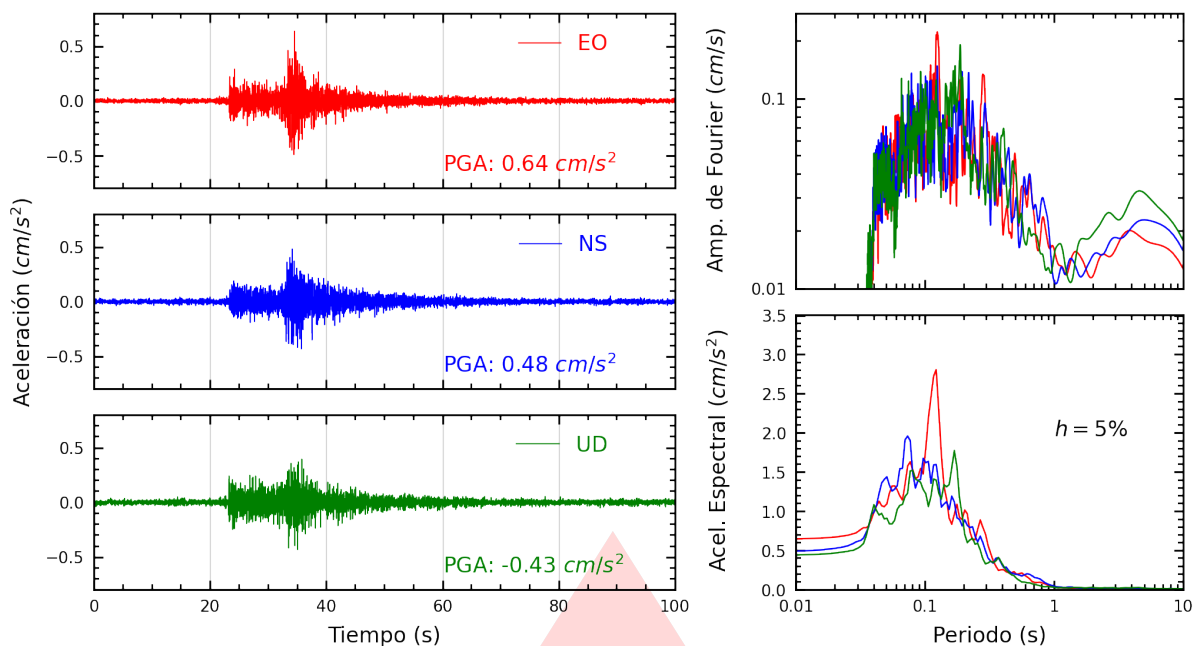
Figura A.33: Registros tiempo-historia, espectros de Fourier y de respuesta en las direcciones EO, NS y vertical de la estación UNFV. Sismo de Callao, Provincia Constitucional del Callao del 2026-09-30, 11:12:38 (Hora local)
