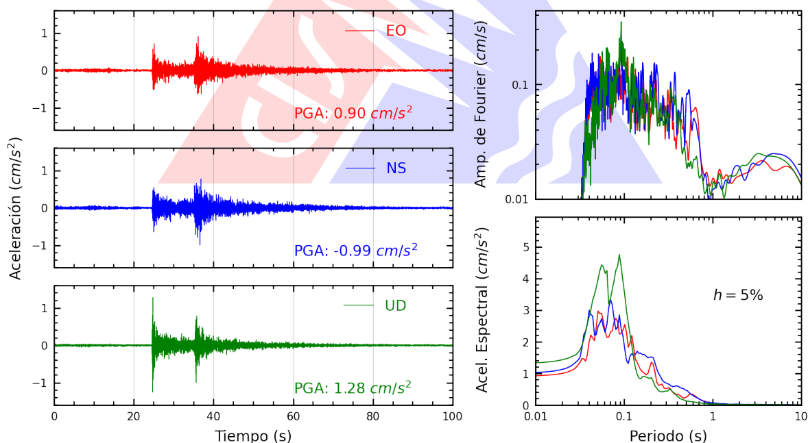
Figura A.16: Registros tiempo-historia, espectros de Fourier y de respuesta en las direcciones EO, NS y vertical de la estación COMAS. Sismo de Callao, Provincia Constitucional del Callao del 2026-09-30, 11:12:38 (Hora local)
