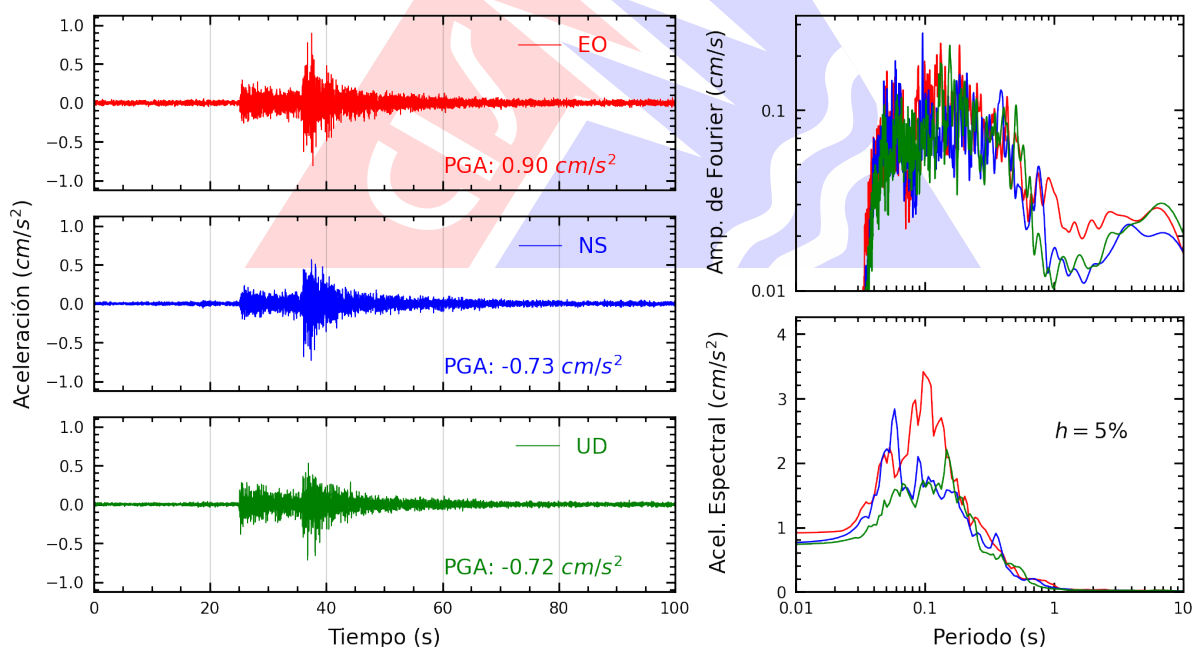
Figura A.26: Registros tiempo-historia, espectros de Fourier y de respuesta en las direcciones EO, NS y vertical de la estación IMCA. Sismo de Callao, Provincia Constitucional del Callao del 2026-09-30, 11:12:38 (Hora local)
