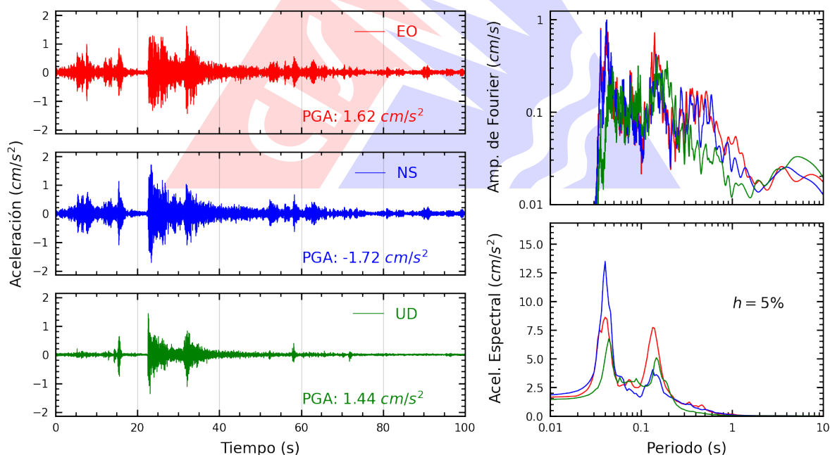
Figura A.8: Registros tiempo-historia, espectros de Fourier y de respuesta en las direcciones EO, NS y vertical de la estación DHNPE. Sismo de Callao, Provincia Constitucional del Callao del 2026-09-30, 11:12:38 (Hora local)
