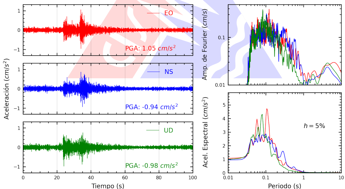
Figura A.20: Registros tiempo-historia, espectros de Fourier y de respuesta en las direcciones EO, NS y vertical de la estación MADRE. Sismo de Callao, Provincia Constitucional del Callao del 2026-09-30, 11:12:38 (Hora local)
