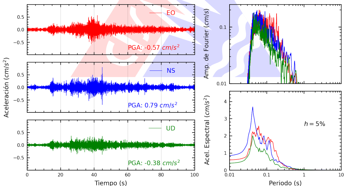
Figura A.28: Registros tiempo-historia, espectros de Fourier y de respuesta en las direcciones EO, NS y vertical de la estación PACHA. Sismo de Callao, Provincia Constitucional del Callao del 2026-09-30, 11:12:38 (Hora local)
