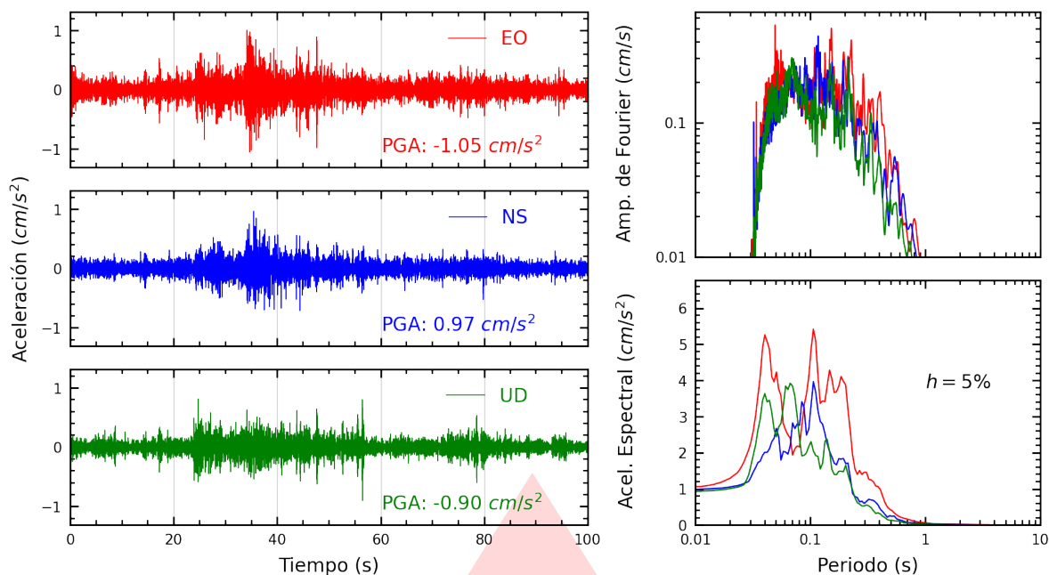
Figura A.21: Registros tiempo-historia, espectros de Fourier y de respuesta en las direcciones EO, NS y vertical de la estación SOBAR. Sismo de Callao, Provincia Constitucional del Callao del 2026-09-30, 11:12:38 (Hora local)
