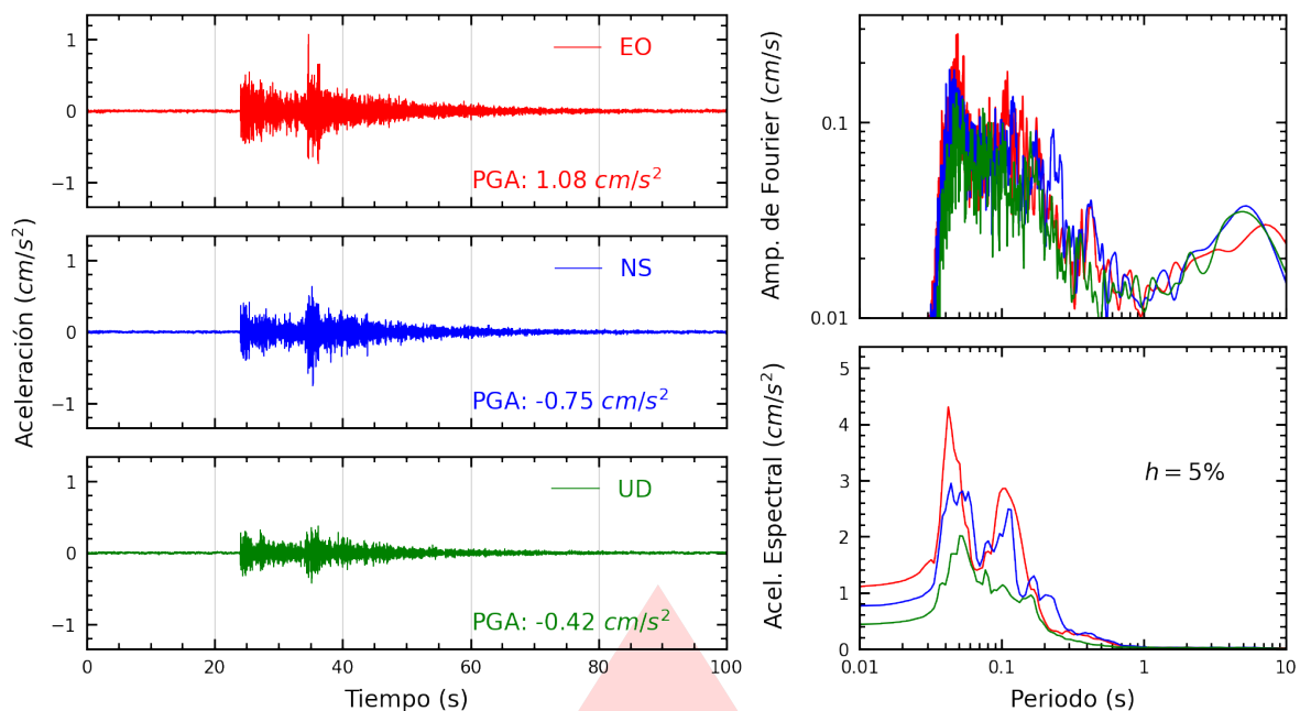
Figura A.19: Registros tiempo-historia, espectros de Fourier y de respuesta en las direcciones EO, NS y vertical de la estación UCSS. Sismo de Callao, Provincia Constitucional del Callao del 2026-09-30, 11:12:38 (Hora local)
