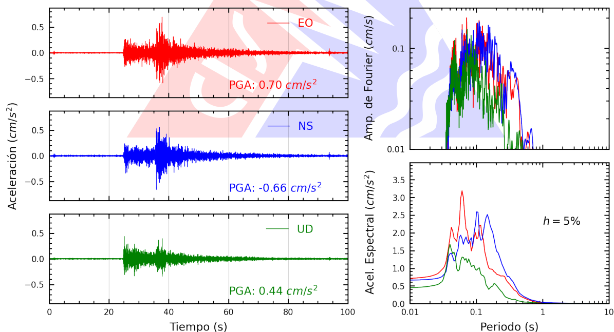
Figura A.30: Registros tiempo-historia, espectros de Fourier y de respuesta en las direcciones EO, NS y vertical de la estación ATARJ. Sismo de Callao, Provincia Constitucional del Callao del 2026-09-30, 11:12:38 (Hora local)
