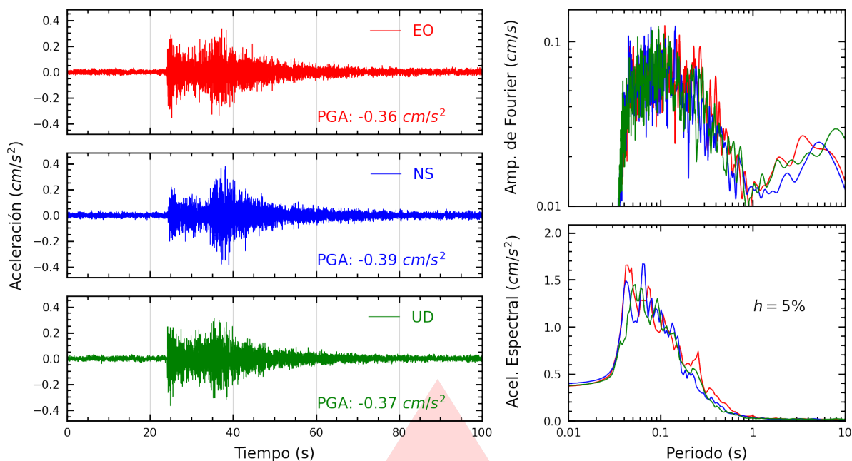
Figura A.35: Registros tiempo-historia, espectros de Fourier y de respuesta en las direcciones EO, NS y vertical de la estación SERVI. Sismo de Callao, Provincia Constitucional del Callao del 2026-09-30, 11:12:38 (Hora local)
