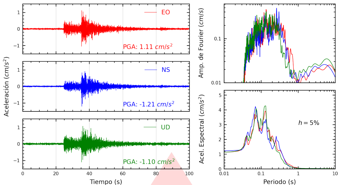
Figura A.17: Registros tiempo-historia, espectros de Fourier y de respuesta en las direcciones EO, NS y vertical de la estación SOVES. Sismo de Callao, Provincia Constitucional del Callao del 2026-09-30, 11:12:38 (Hora local)
