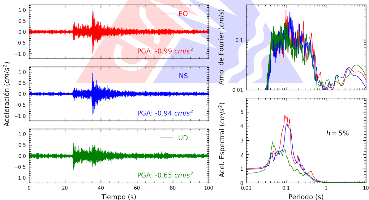
Figura A.24: Registros tiempo-historia, espectros de Fourier y de respuesta en las direcciones EO, NS y vertical de la estación URPE. Sismo de Callao, Provincia Constitucional del Callao del 2026-09-30, 11:12:38 (Hora local)
