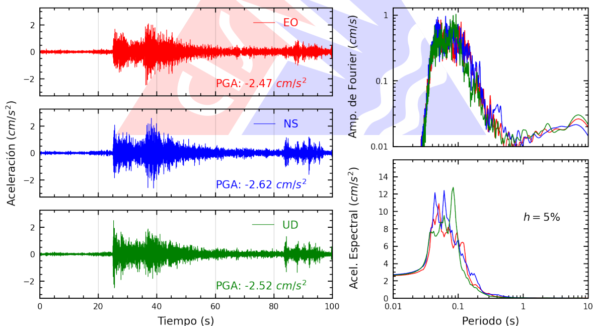
Figura A.4: Registros tiempo-historia, espectros de Fourier y de respuesta en las direcciones EO, NS y vertical de la estación SROSA. Sismo de Callao, Provincia Constitucional del Callao del 2026-09-30, 11:12:38 (Hora local)
