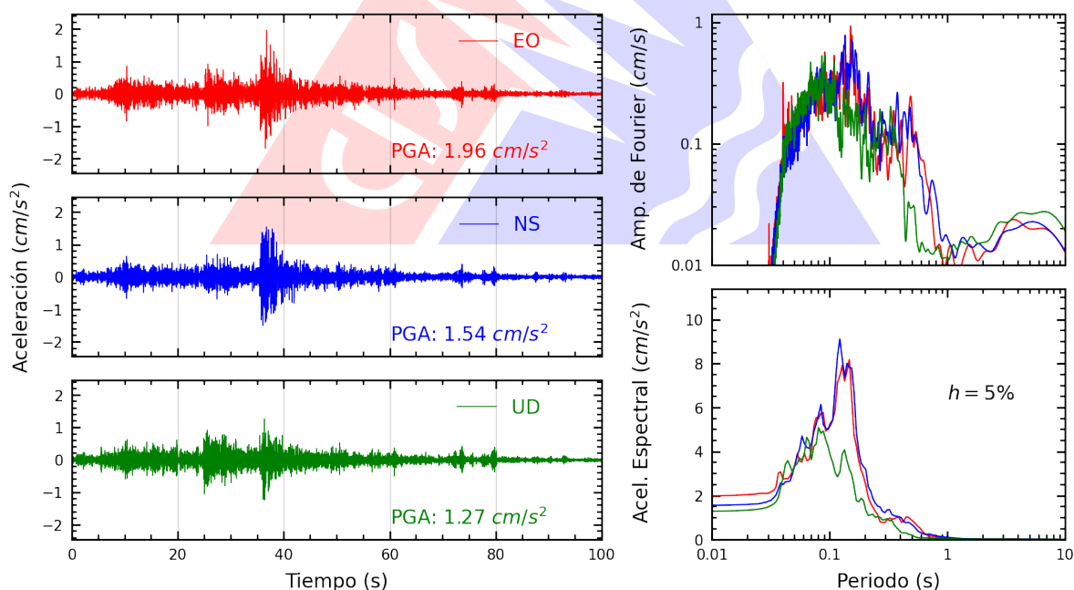
Figura A.6: Registros tiempo-historia, espectros de Fourier y de respuesta en las direcciones EO, NS y vertical de la estación SJLSV. Sismo de Callao, Provincia Constitucional del Callao del 2026-09-30, 11:12:38 (Hora local)
