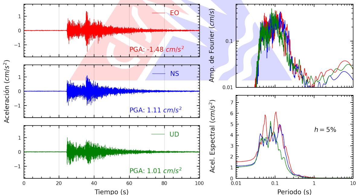
Figura A.10: Registros tiempo-historia, espectros de Fourier y de respuesta en las direcciones EO, NS y vertical de la estación AMORE. Sismo de Callao, Provincia Constitucional del Callao del 2026-09-30, 11:12:38 (Hora local)
