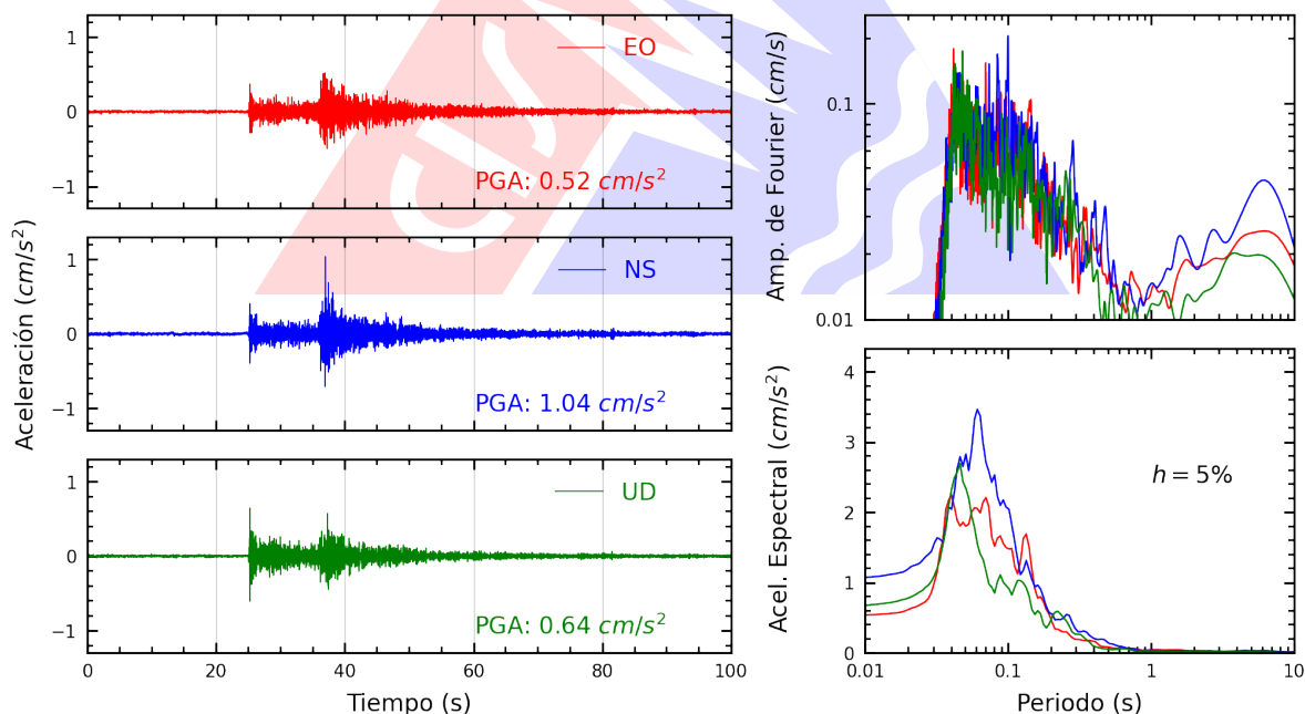
Figura A.22: Registros tiempo-historia, espectros de Fourier y de respuesta en las direcciones EO, NS y vertical de la estación SJLCE. Sismo de Callao, Provincia Constitucional del Callao del 2026-09-30, 11:12:38 (Hora local)
