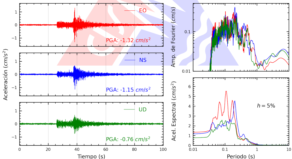
Figura A.14: Registros tiempo-historia, espectros de Fourier y de respuesta en las direcciones EO, NS y vertical de la estación UCVAT. Sismo de Callao, Provincia Constitucional del Callao del 2026-09-30, 11:12:38 (Hora local)
