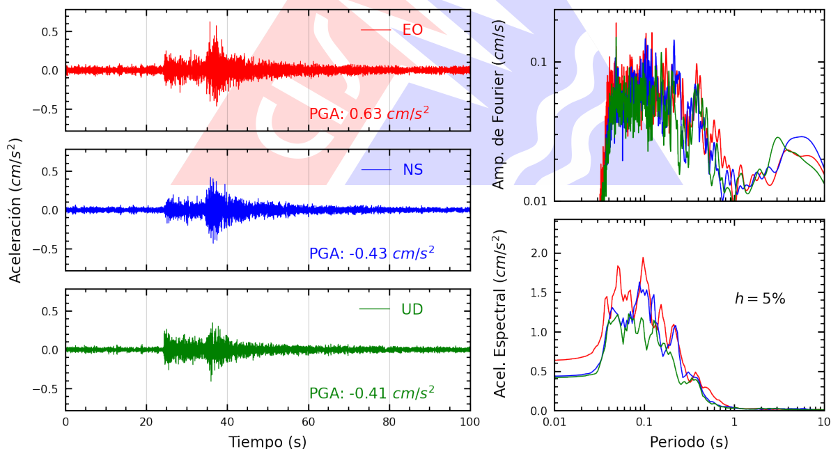
Figura A.34: Registros tiempo-historia, espectros de Fourier y de respuesta en las direcciones EO, NS y vertical de la estación INICT. Sismo de Callao, Provincia Constitucional del Callao del 2026-09-30, 11:12:38 (Hora local)
