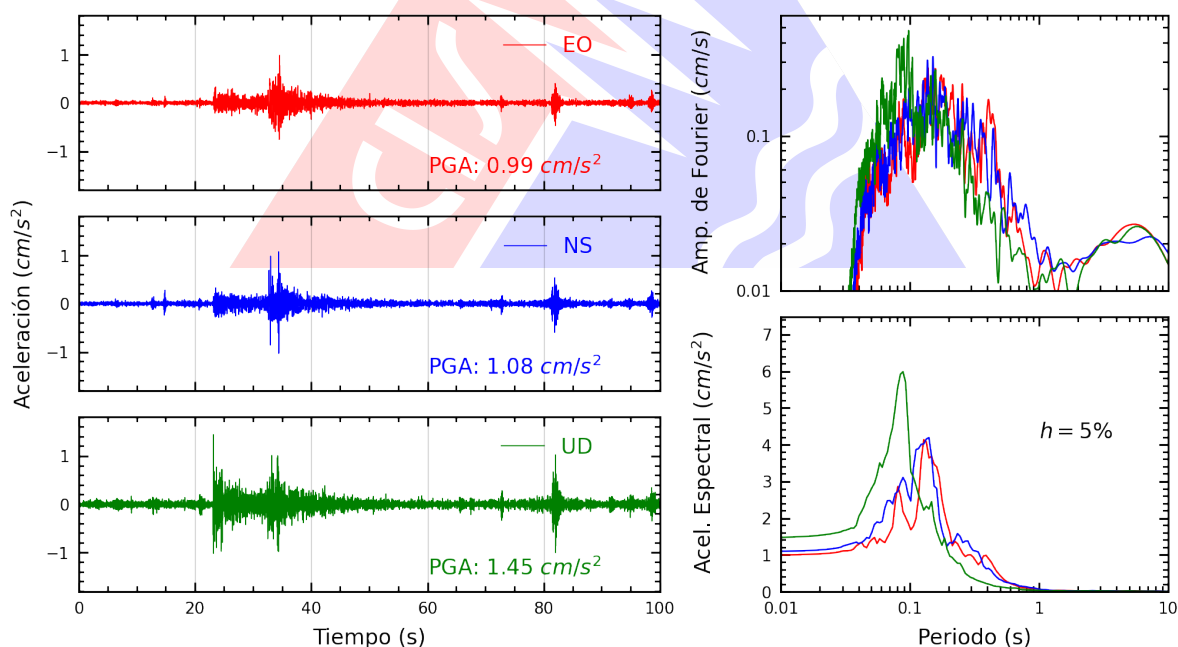
Figura A.12: Registros tiempo-historia, espectros de Fourier y de respuesta en las direcciones EO, NS y vertical de la estación RAMON. Sismo de Callao, Provincia Constitucional del Callao del 2026-09-30, 11:12:38 (Hora local)
