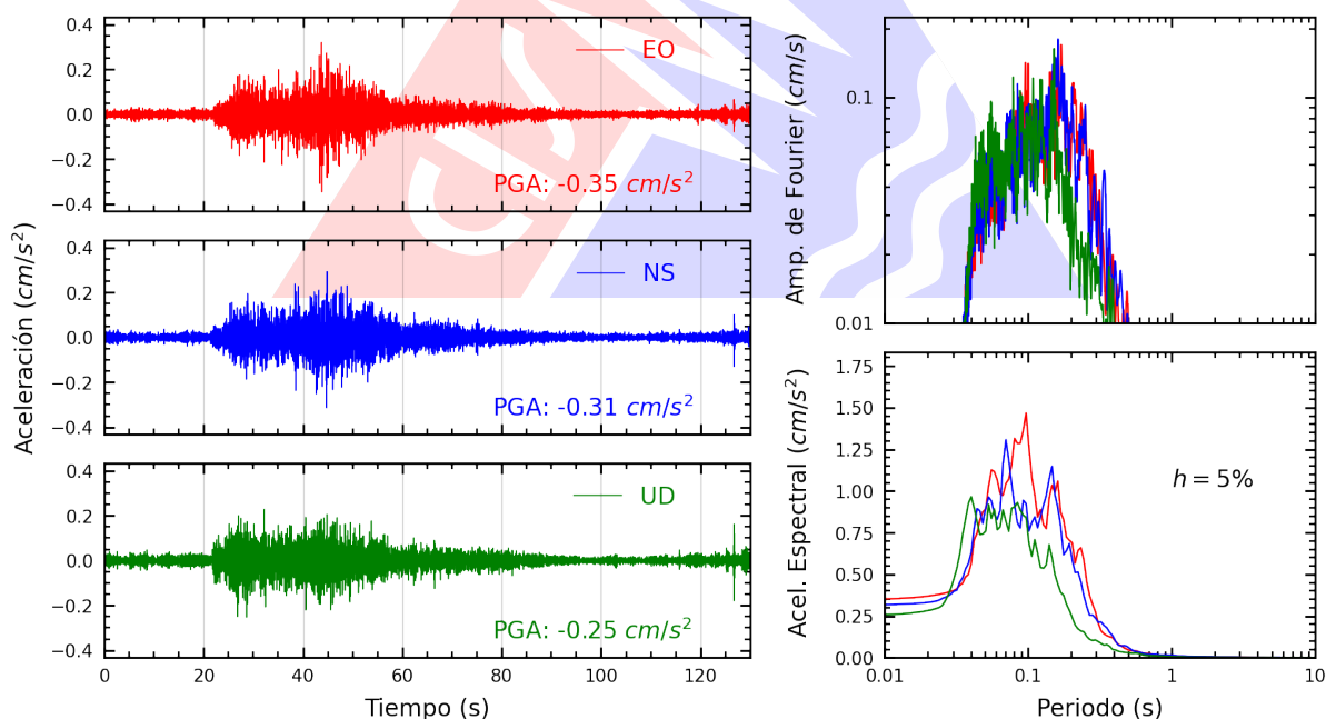
Figura A.36: Registros tiempo-historia, espectros de Fourier y de respuesta en las direcciones EO, NS y vertical de la estación ASIA. Sismo de Callao, Provincia Constitucional del Callao del 2026-09-30, 11:12:38 (Hora local)
