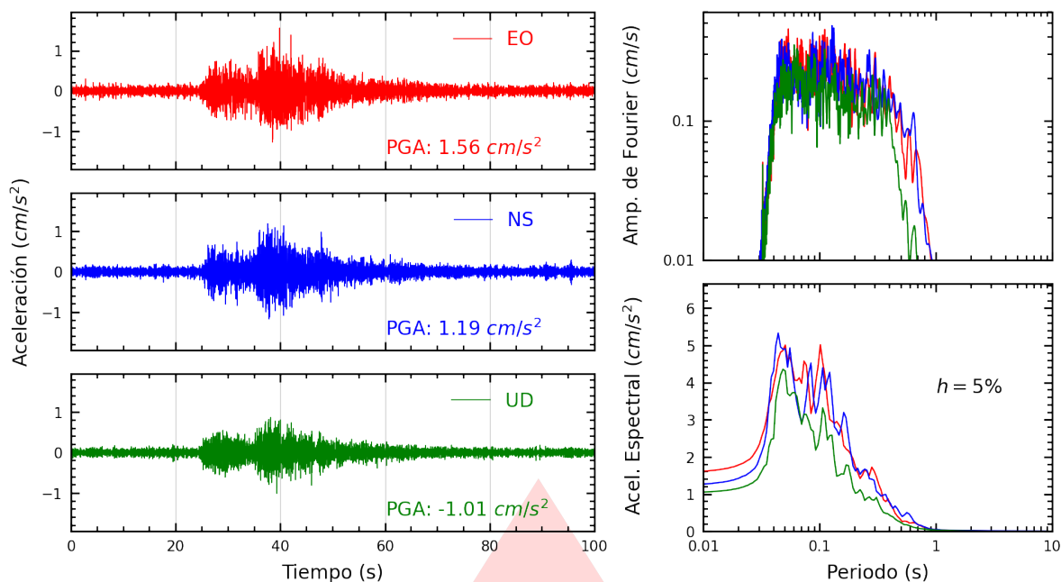
Figura A.9: Registros tiempo-historia, espectros de Fourier y de respuesta en las direcciones EO, NS y vertical de la estación UNTEL. Sismo de Callao, Provincia Constitucional del Callao del 2026-09-30, 11:12:38 (Hora local)
