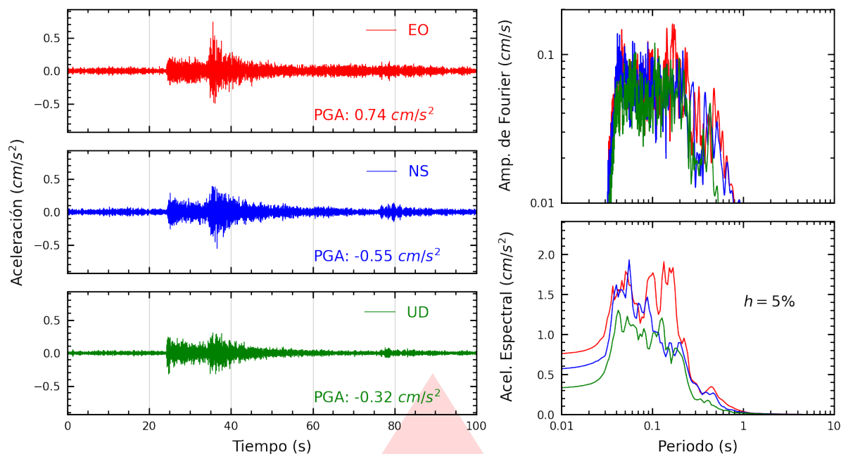
Figura A.29: Registros tiempo-historia, espectros de Fourier y de respuesta en las direcciones EO, NS y vertical de la estación BORJA. Sismo de Callao, Provincia Constitucional del Callao del 2026-09-30, 11:12:38 (Hora local)
