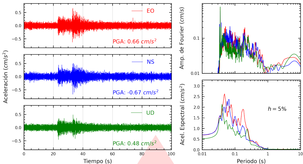
Figura A.31: Registros tiempo-historia, espectros de Fourier y de respuesta en las direcciones EO, NS y vertical de la estación UPCVI. Sismo de Callao, Provincia Constitucional del Callao del 2026-09-30, 11:12:38 (Hora local)
