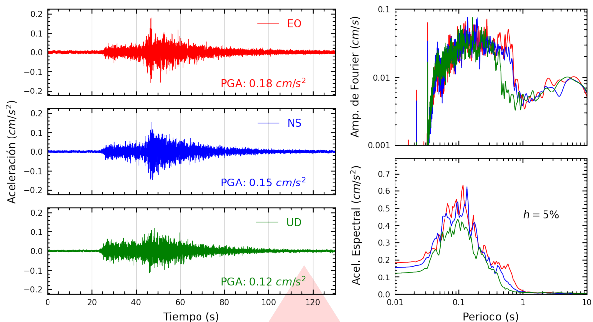
Figura A.37: Registros tiempo-historia, espectros de Fourier y de respuesta en las direcciones EO, NS y vertical de la estación CARAL. Sismo de Callao, Provincia Constitucional del Callao del 2026-09-30, 11:12:38 (Hora local)
