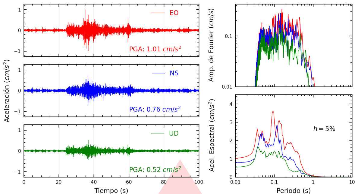
Figura A.23: Registros tiempo-historia, espectros de Fourier y de respuesta en las direcciones EO, NS y vertical de la estación BRISA. Sismo de Callao, Provincia Constitucional del Callao del 2026-09-30, 11:12:38 (Hora local)
