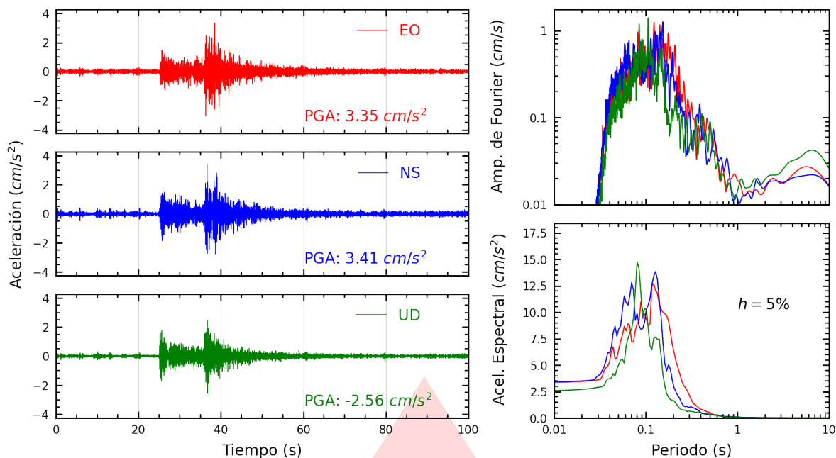
Figura A.1: Registros tiempo-historia, espectros de Fourier y de respuesta en las direcciones EO, NS y vertical de la estación USILM. Sismo de Callao, Provincia Constitucional del Callao del 2026-09-30, 11:12:38 (Hora local)
