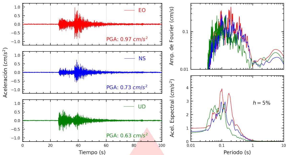
Figura A.25: Registros tiempo-historia, espectros de Fourier y de respuesta en las direcciones EO, NS y vertical de la estación USILP. Sismo de Callao, Provincia Constitucional del Callao del 2026-09-30, 11:12:38 (Hora local)
