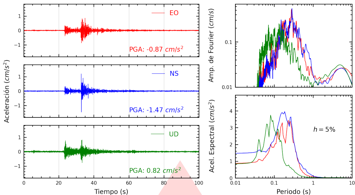
Figura A.11: Registros tiempo-historia, espectros de Fourier y de respuesta en las direcciones EO, NS y vertical de la estación ACAPU. Sismo de Callao, Provincia Constitucional del Callao del 2026-09-30, 11:12:38 (Hora local)
