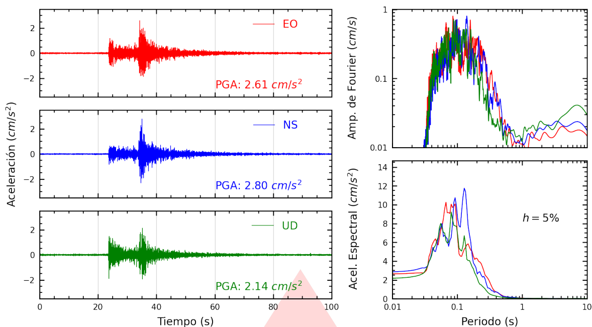
Figura A.3: Registros tiempo-historia, espectros de Fourier y de respuesta en las direcciones EO, NS y vertical de la estación INDEP. Sismo de Callao, Provincia Constitucional del Callao del 2026-09-30, 11:12:38 (Hora local)
