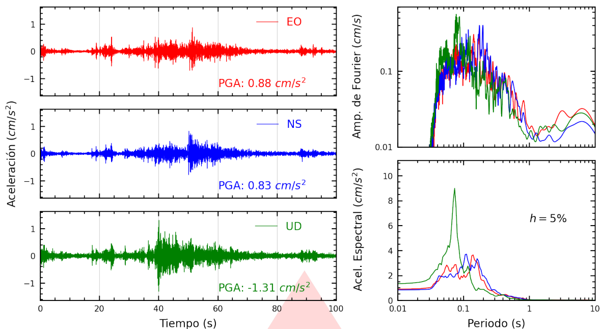
Figura A.15: Registros tiempo-historia, espectros de Fourier y de respuesta en las direcciones EO, NS y vertical de la estación SOCHO. Sismo de Callao, Provincia Constitucional del Callao del 2026-09-30, 11:12:38 (Hora local)
