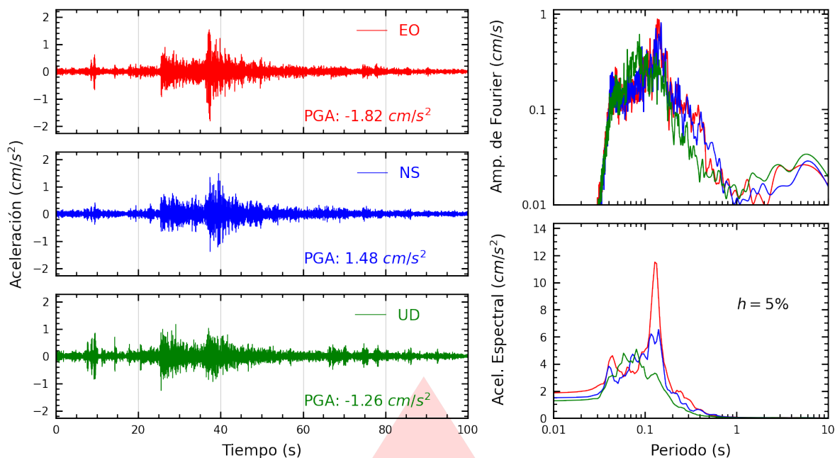
Figura A.7: Registros tiempo-historia, espectros de Fourier y de respuesta en las direcciones EO, NS y vertical de la estación CARAB. Sismo de Callao, Provincia Constitucional del Callao del 2026-09-30, 11:12:38 (Hora local)
