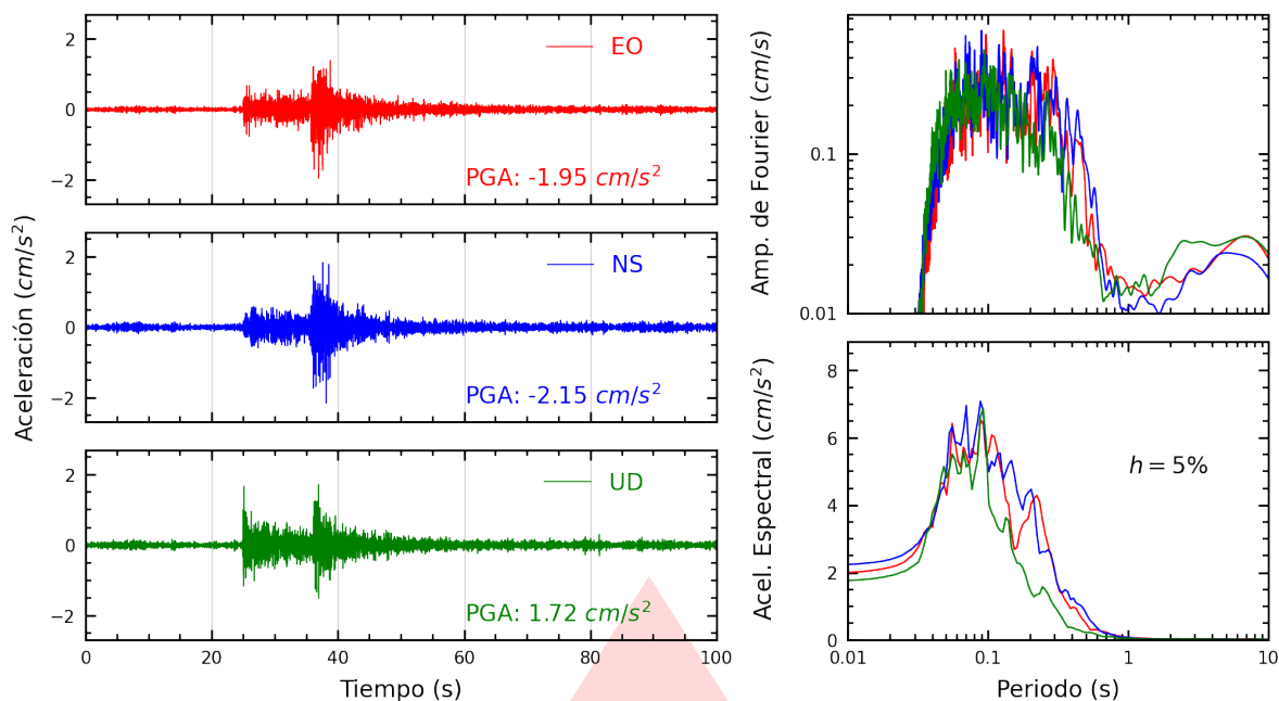
Figura A.5: Registros tiempo-historia, espectros de Fourier y de respuesta en las direcciones EO, NS y vertical de la estación SJLSC. Sismo de Callao, Provincia Constitucional del Callao del 2026-09-30, 11:12:38 (Hora local)
