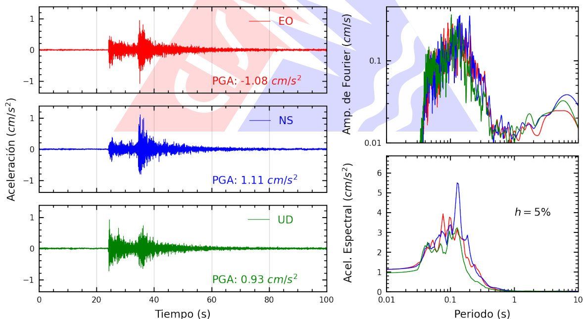
Figura A.18: Registros tiempo-historia, espectros de Fourier y de respuesta en las direcciones EO, NS y vertical de la estación JALVA. Sismo de Callao, Provincia Constitucional del Callao del 2026-09-30, 11:12:38 (Hora local)
