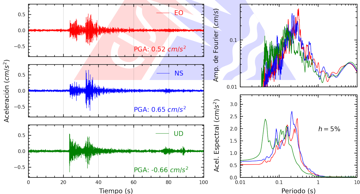
Figura A.32: Registros tiempo-historia, espectros de Fourier y de respuesta en las direcciones EO, NS y vertical de la estación DSML. Sismo de Callao, Provincia Constitucional del Callao del 2026-09-30, 11:12:38 (Hora local)
