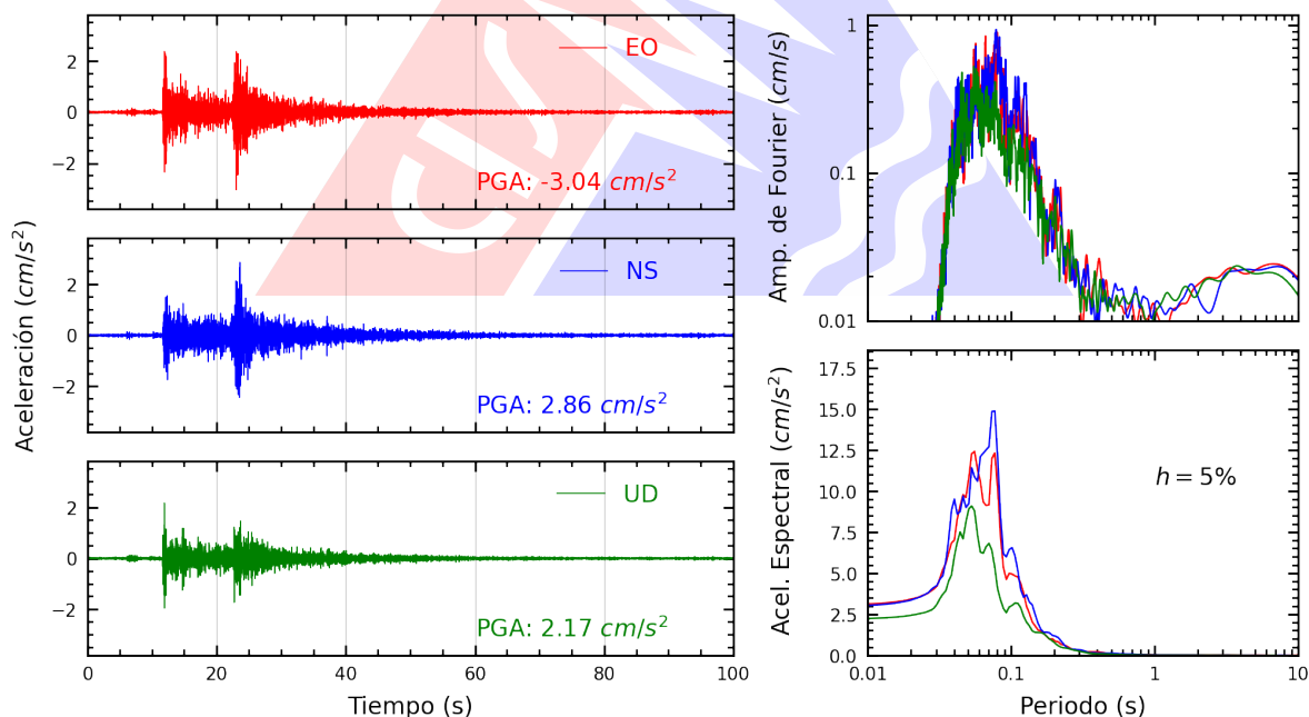
Figura A.2: Registros tiempo-historia, espectros de Fourier y de respuesta en las direcciones EO, NS y vertical de la estación JOSEO. Sismo de Callao, Provincia Constitucional del Callao del 2026-09-30, 11:12:38 (Hora local)
