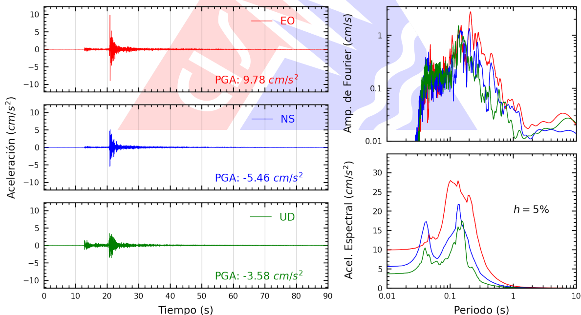
Figura A.2: Registros tiempo-historia, espectros de Fourier y de respuesta en las direcciones EO, NS y vertical de la estación UPAOT. Sismo de Trujillo, Trujillo - La Libertad del 2026-10-02, 05:13:19 (Hora local)
