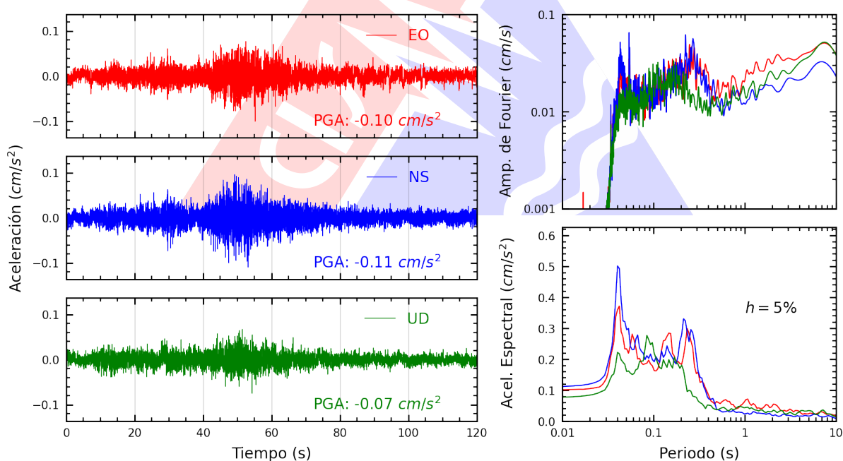
Figura A.4: Registros tiempo-historia, espectros de Fourier y de respuesta en las direcciones EO, NS y vertical de la estación UNAB. Sismo de Trujillo, Trujillo - La Libertad del 2026-10-02, 05:13:19 (Hora local)
