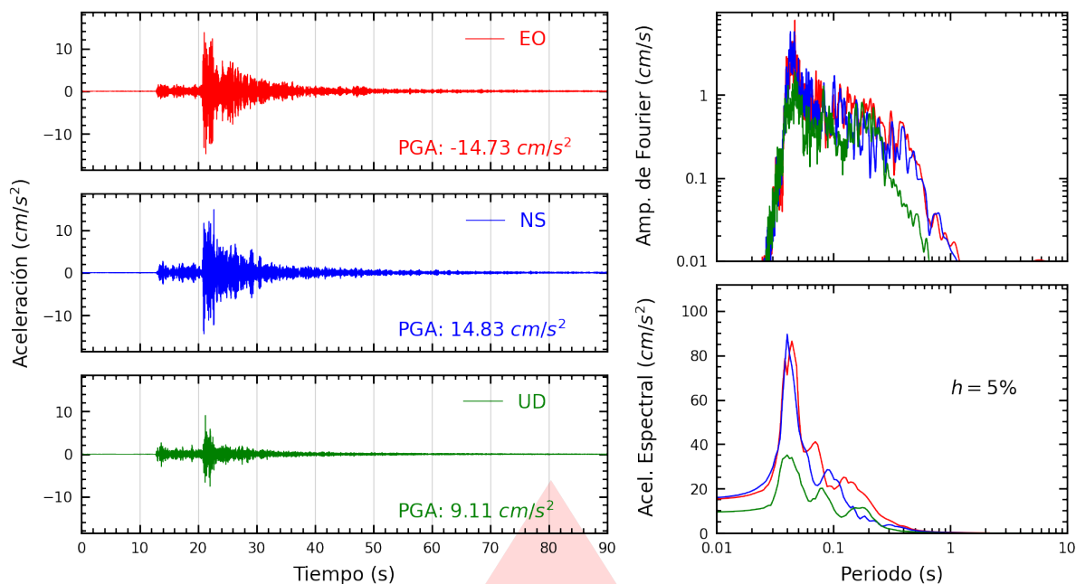
Figura A.1: Registros tiempo-historia, espectros de Fourier y de respuesta en las direcciones EO, NS y vertical de la estación SCTR. Sismo de Trujillo, Trujillo - La Libertad del 2026-10-02, 05:13:19 (Hora local)
