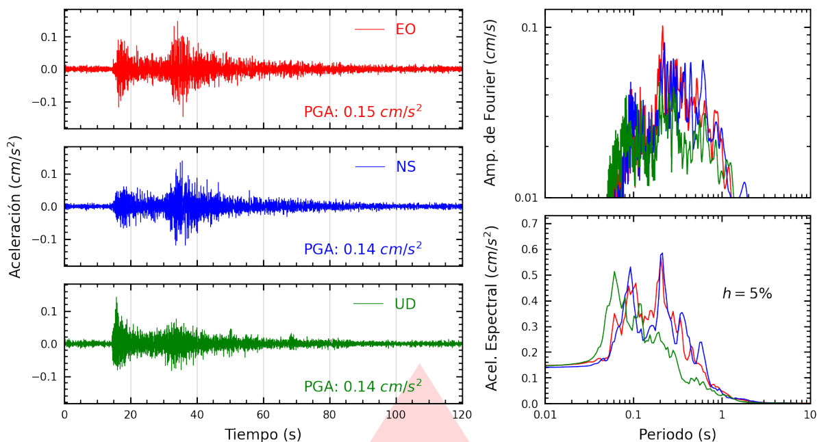
Figura A.3: Registros tiempo-historia, espectros de Fourier y de respuesta en las direcciones EO, NS y vertical de la estación UNC. Sismo de Trujillo, Trujillo - La Libertad del 2026-10-02, 05:13:19 (Hora local)
