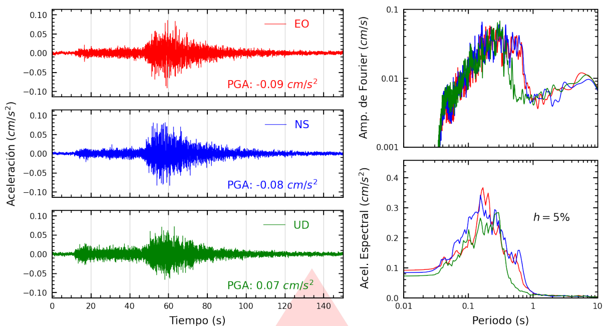
Figura A.5: Registros tiempo-historia, espectros de Fourier y de respuesta en las direcciones EO, NS y vertical de la estación CARAL. Sismo de Trujillo, Trujillo - La Libertad del 2026-10-02, 05:13:19 (Hora local)
