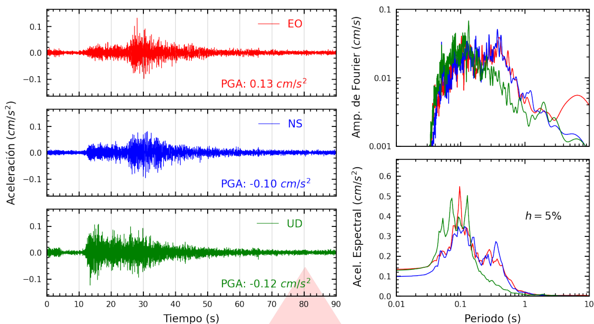
Figura A.1: Registros tiempo-historia, espectros de Fourier y de respuesta en las direcciones EO, NS y vertical de la estación SCPIU. Sismo de Talara, Talara - Piura del 2026-10-04, 03:14:10 (Hora local)
