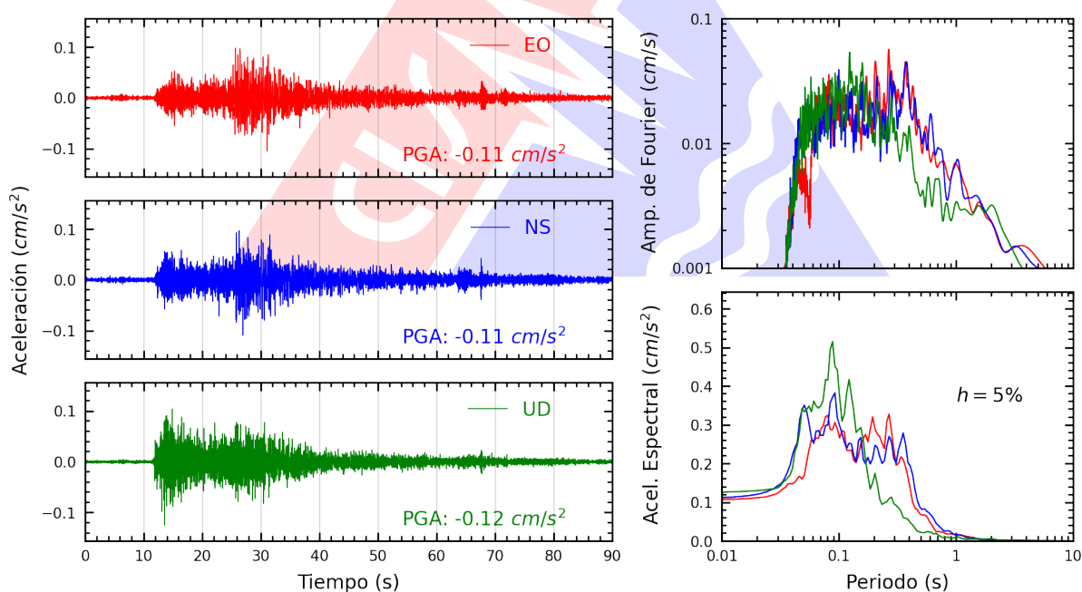
Figura A.2: Registros tiempo-historia, espectros de Fourier y de respuesta en las direcciones EO, NS y vertical de la estación UPAOP. Sismo de Talara, Talara - Piura del 2026-10-04, 03:14:10 (Hora local)
