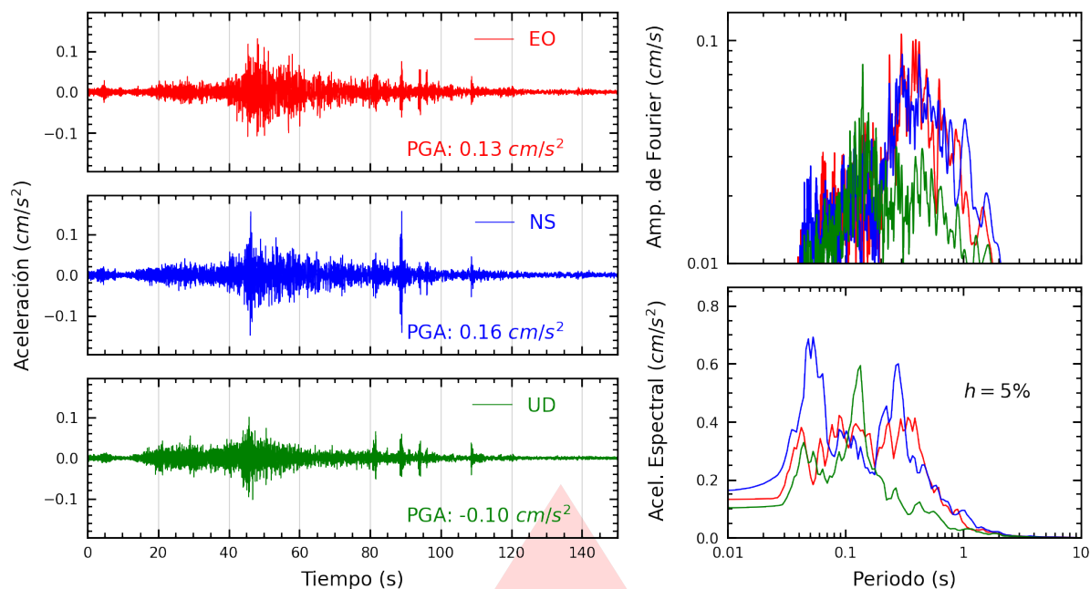
Figura A.1: Registros tiempo-historia, espectros de Fourier y de respuesta en las direcciones EO, NS y vertical de la estación UPAOP. Sismo de Zarumilla, Zarumilla - Tumbes del 2026-10-04, 03:57:19 (Hora local)
