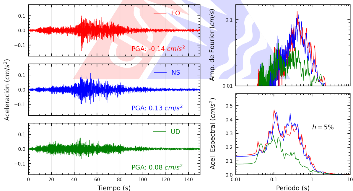
Figura A.2: Registros tiempo-historia, espectros de Fourier y de respuesta en las direcciones EO, NS y vertical de la estación SCPIU. Sismo de Zarumilla, Zarumilla - Tumbes del 2026-10-04, 03:57:19 (Hora local)
