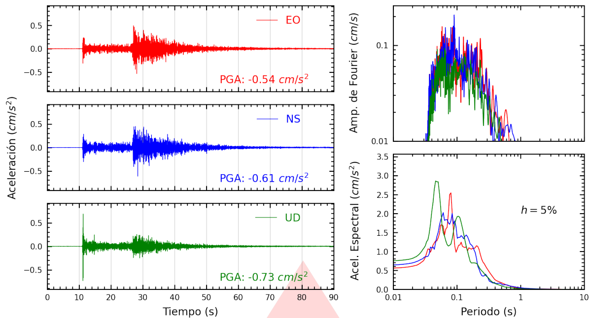
Figura A.1: Registros tiempo-historia, espectros de Fourier y de respuesta en las direcciones EO, NS y vertical de la estación UNSA2. Sismo de Aplao, Castilla - Arequipa del 2026-10-05, 05:32:49 (Hora local)
